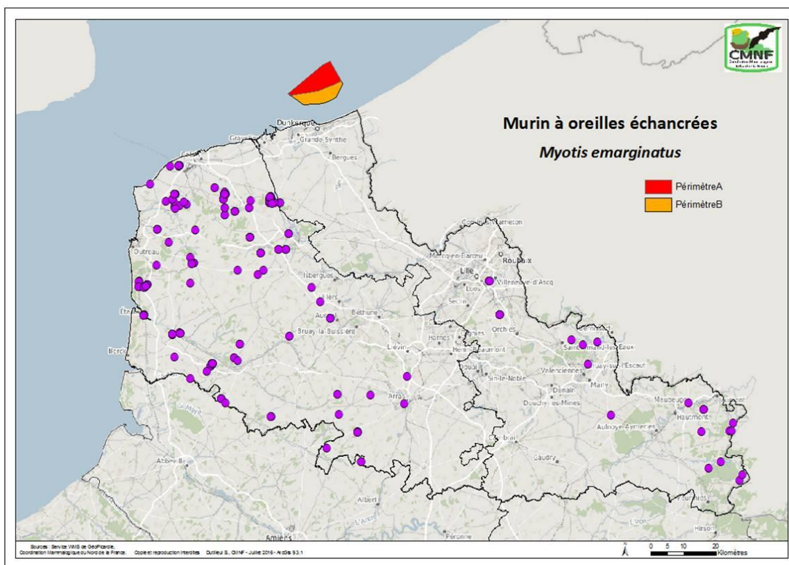
Figure 3.6 : Répartition du Murin à oreilles échanquées en Nord – Pas-de-Calais en 2015 (source : CMNF, Groupe Chiroptères)
