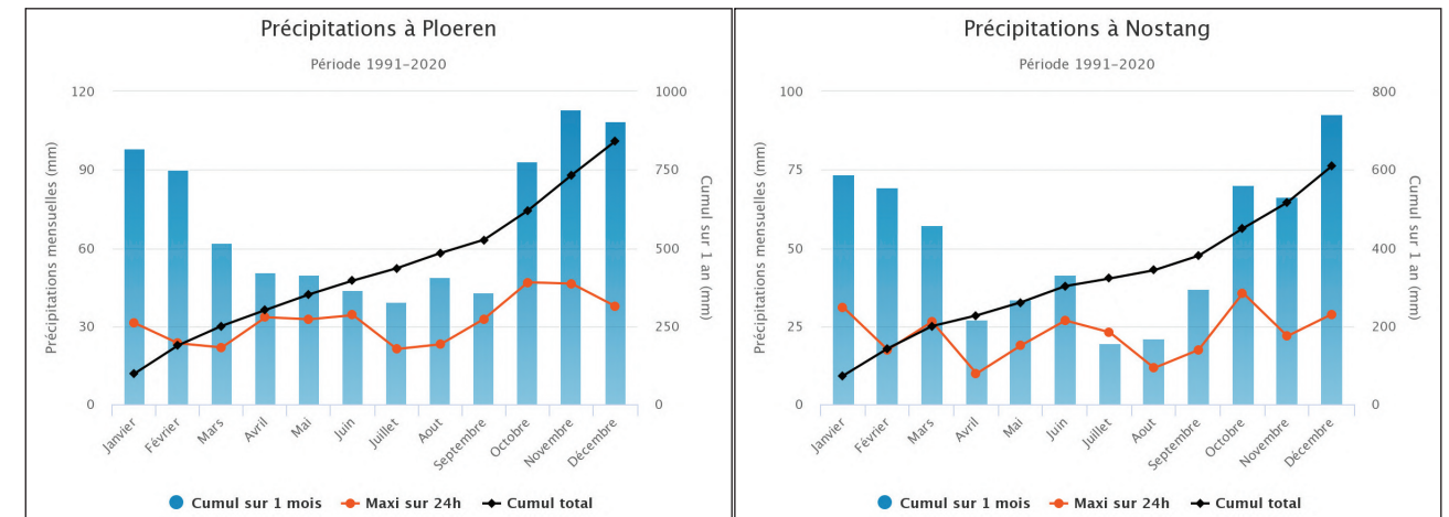
Moyenne mensuelle des précipitations sur la période de 1991-2020 à Ploeren
