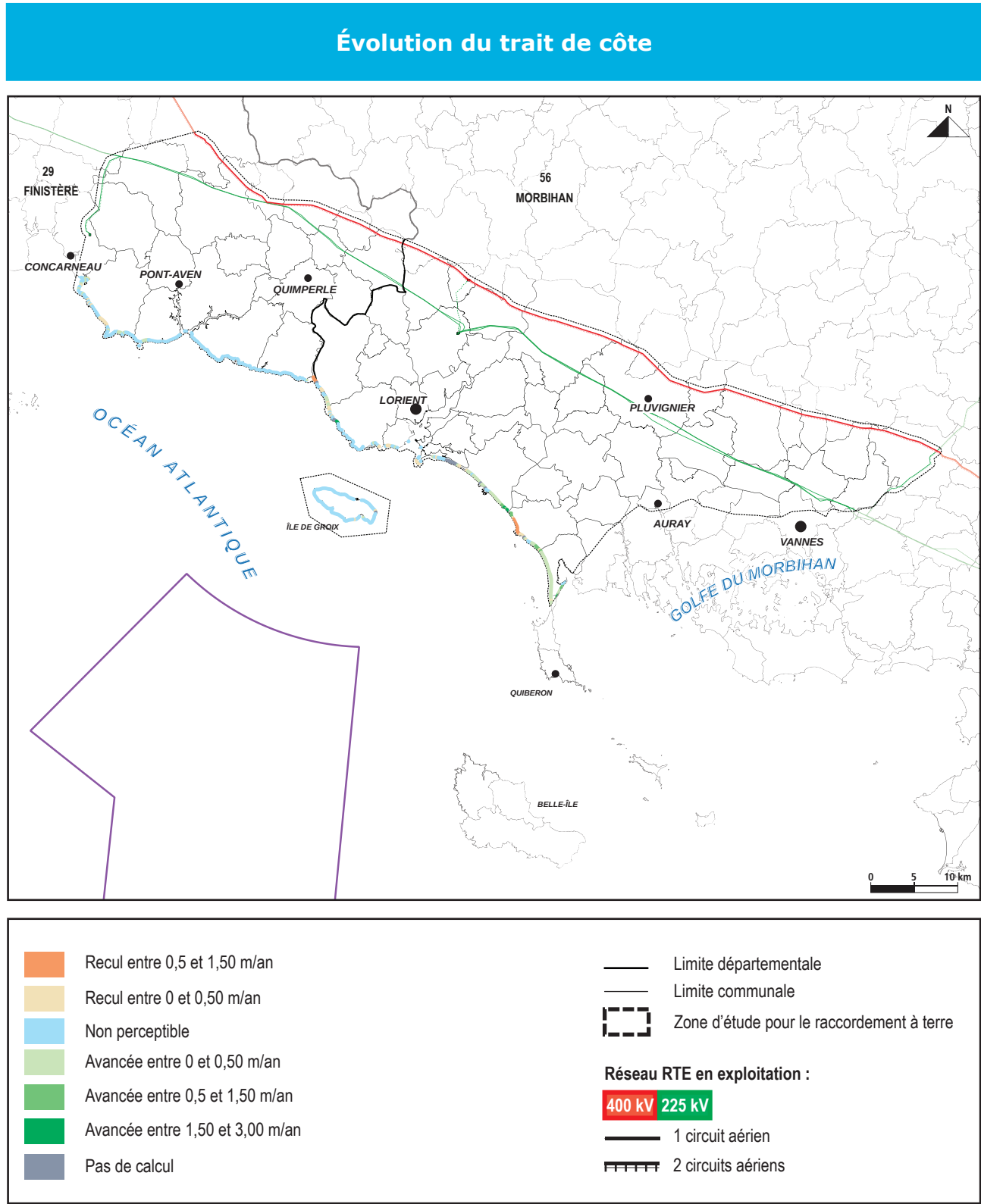
Figure 100 : Carte de l'évolution du trait de côte
