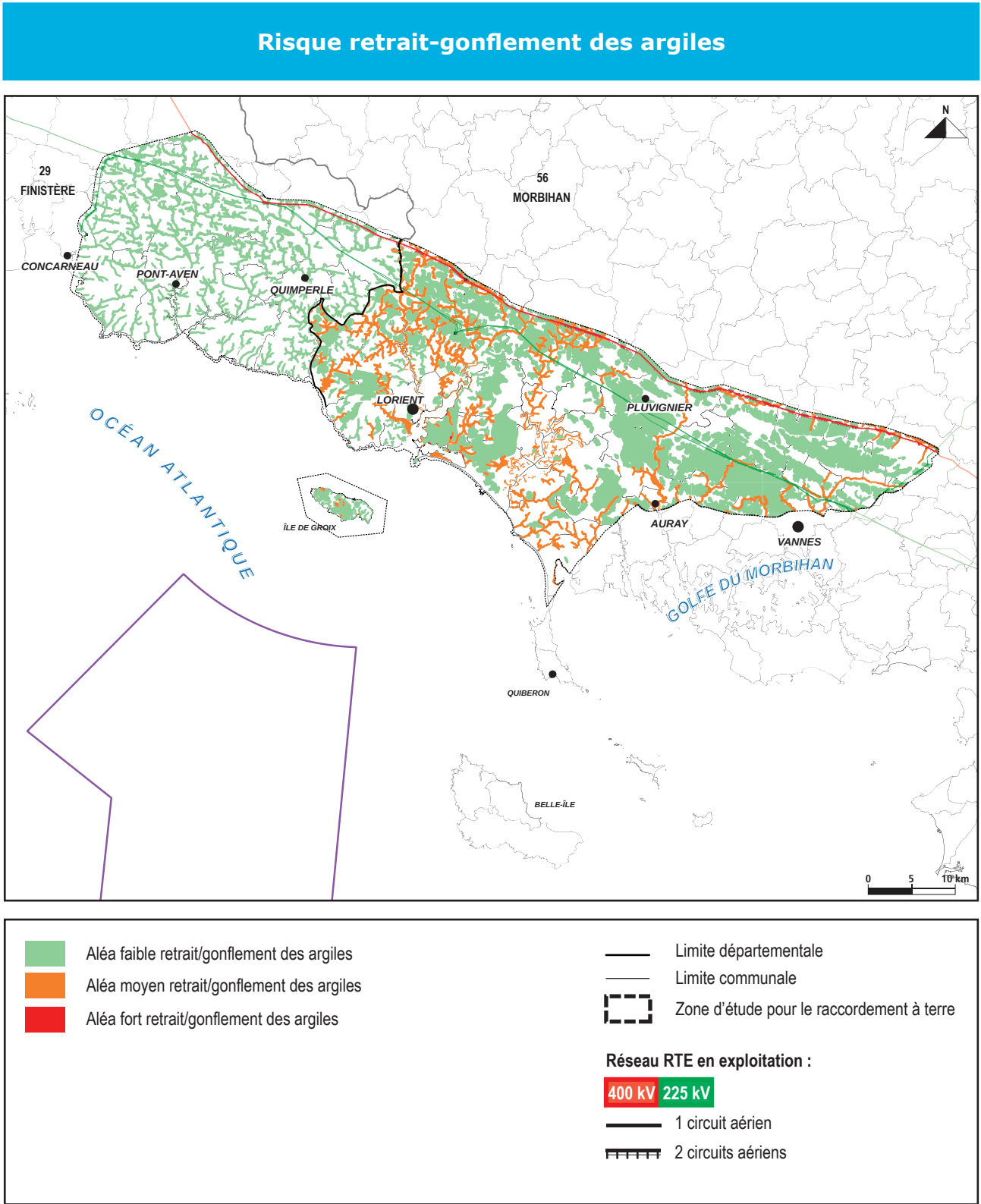
Figure 98 : Carte du risque retrait-gonflement des argiles
