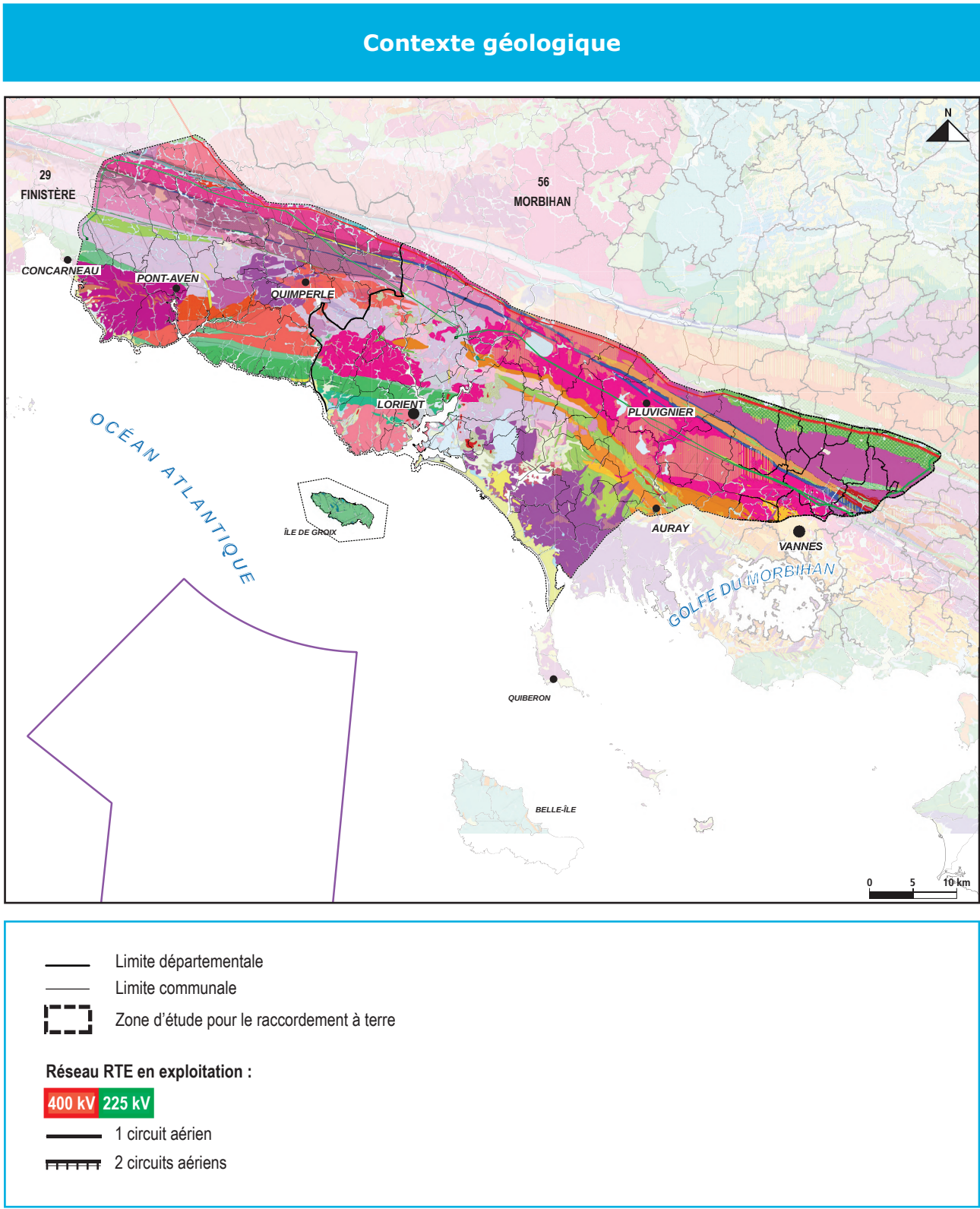
Figure 90 : Carte du contexte géologique
