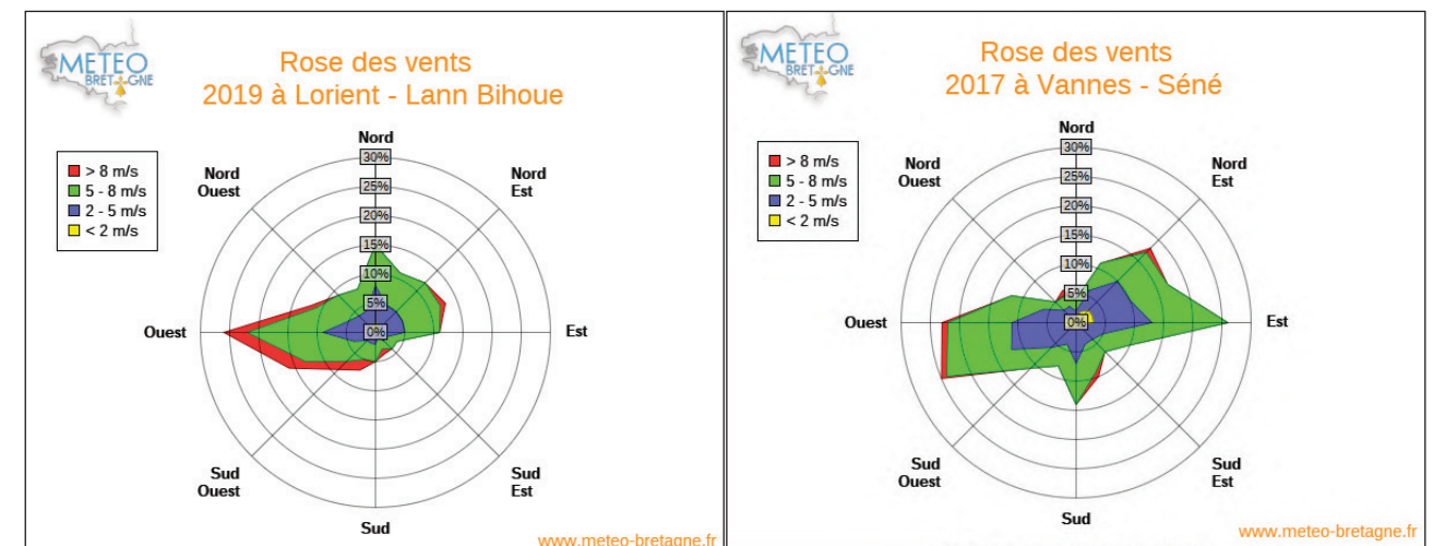
Rose des vents 2019 à Lorient Lann Bihoué
