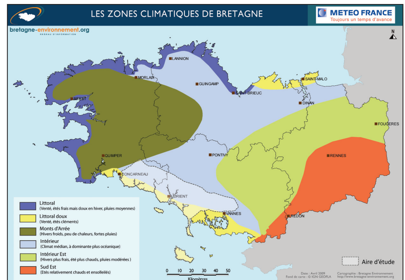
Les zones climatiques de la zone d'étude du raccordement à terre
