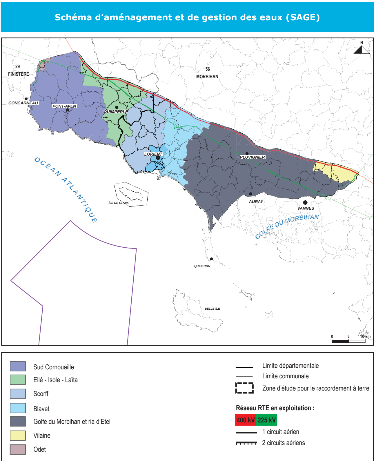
Figure 93 : Carte des Schéma d'aménagement et de gestion des eaux (SAGE)
