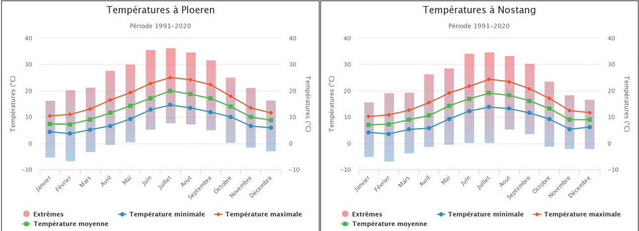
Températures sur la période de 1991-2020 à Ploeren
