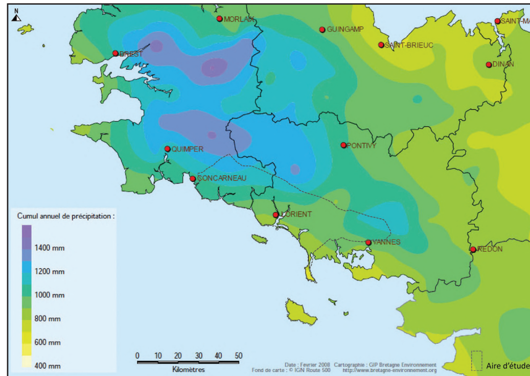
Cumul annuel de précipitation de la zone d'étude du raccordement à terre
