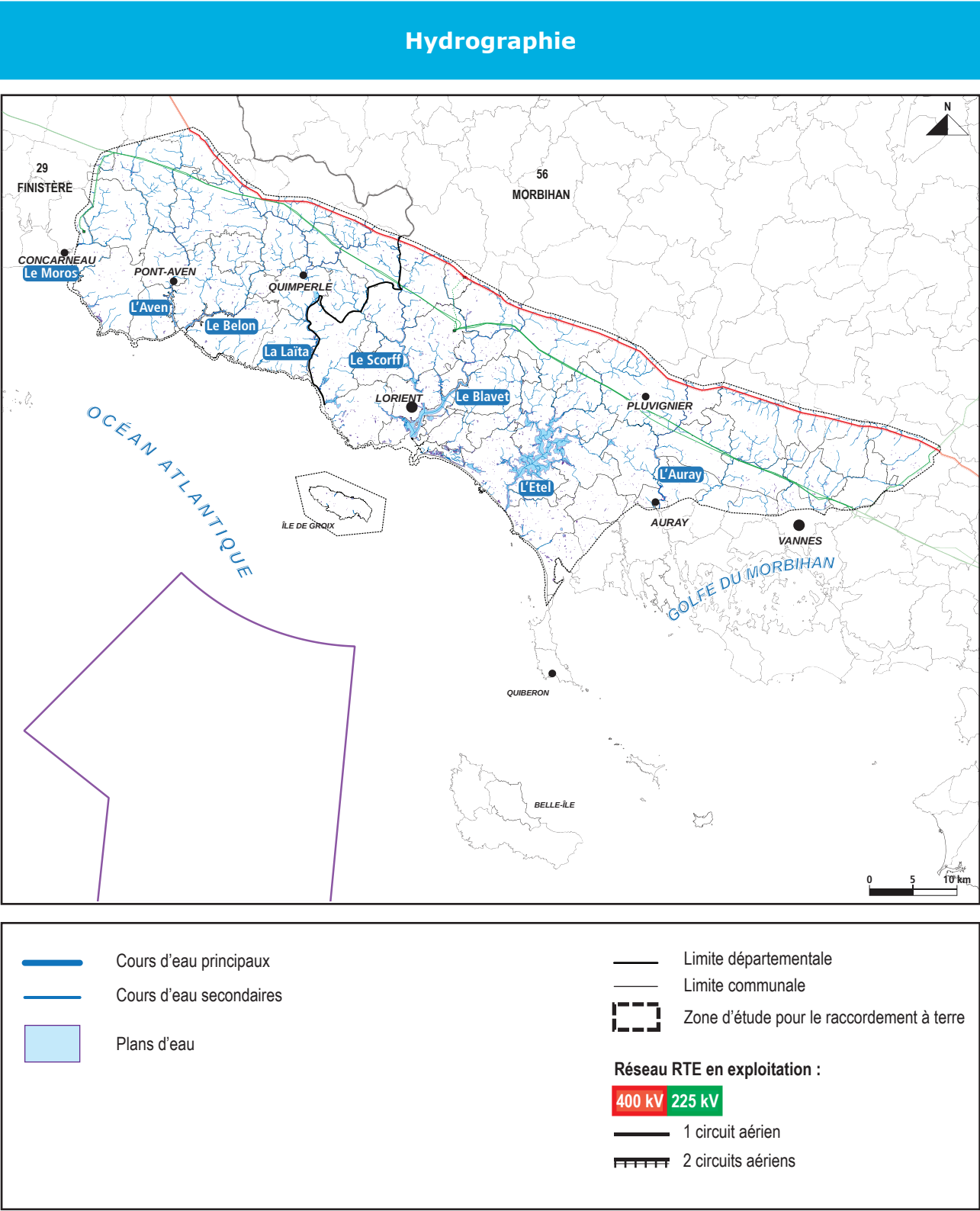
Figure 92 : Carte du réseau hydrographique
