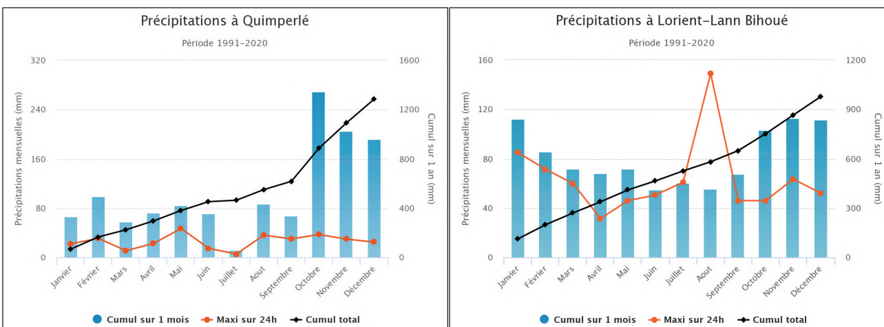
Moyenne mensuelle des précipitations sur la période de 1991-2020 à Quimperlé
