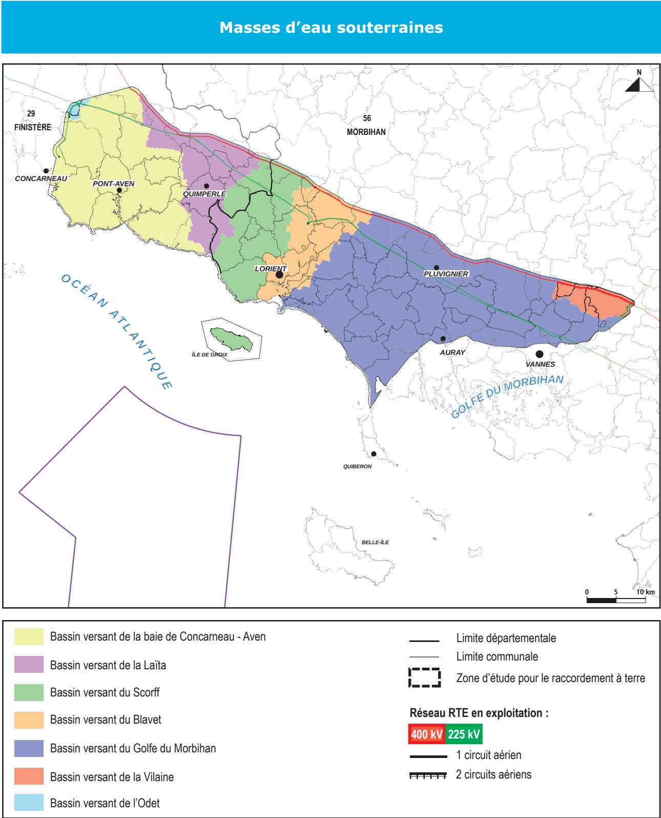
Figure 95 : Carte des masses d'eau souterraines
