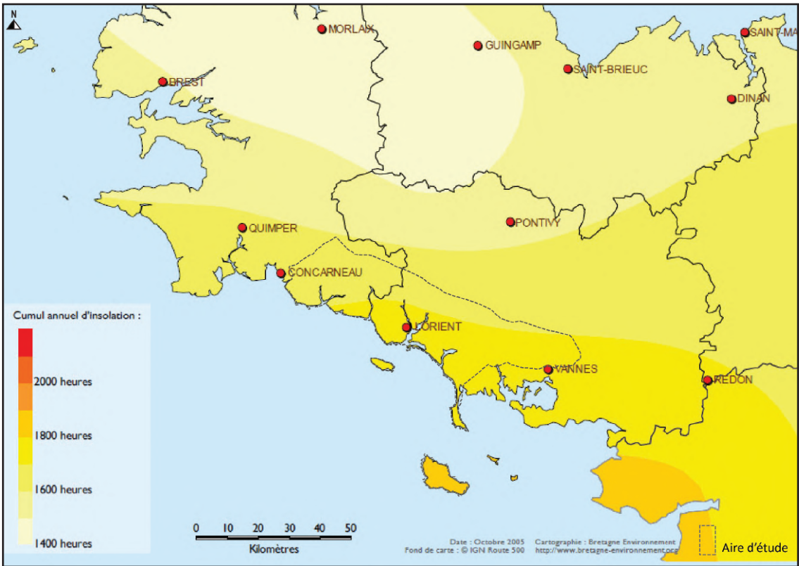
Cumul annuel d'insolation de la zone d'étude du raccordement à terre
