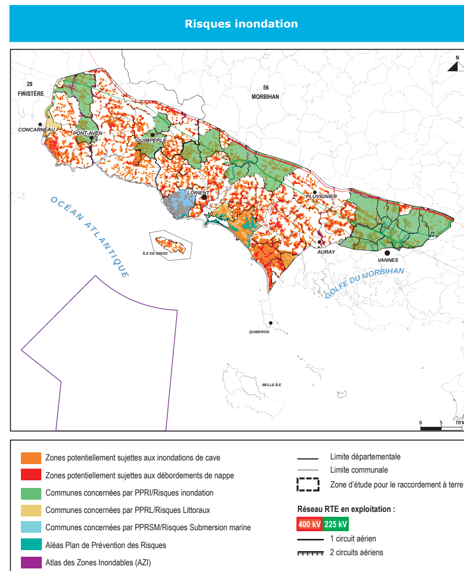
Figure 97 : Carte du risque inondation
