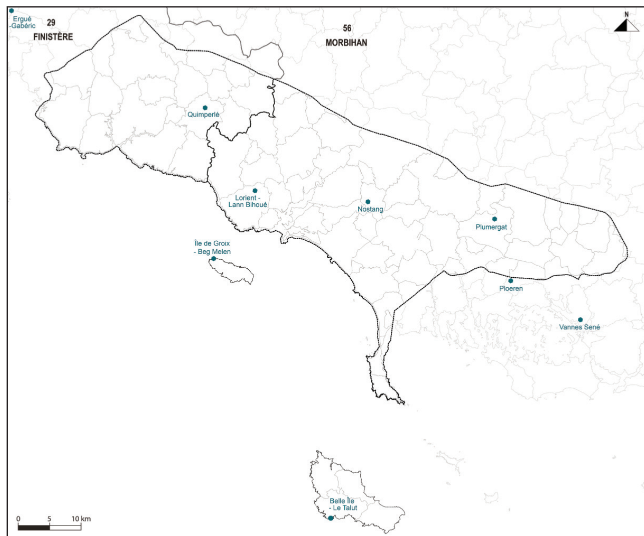
Localisation des stations météorologiques de la zone d'étude du raccordement à terre
