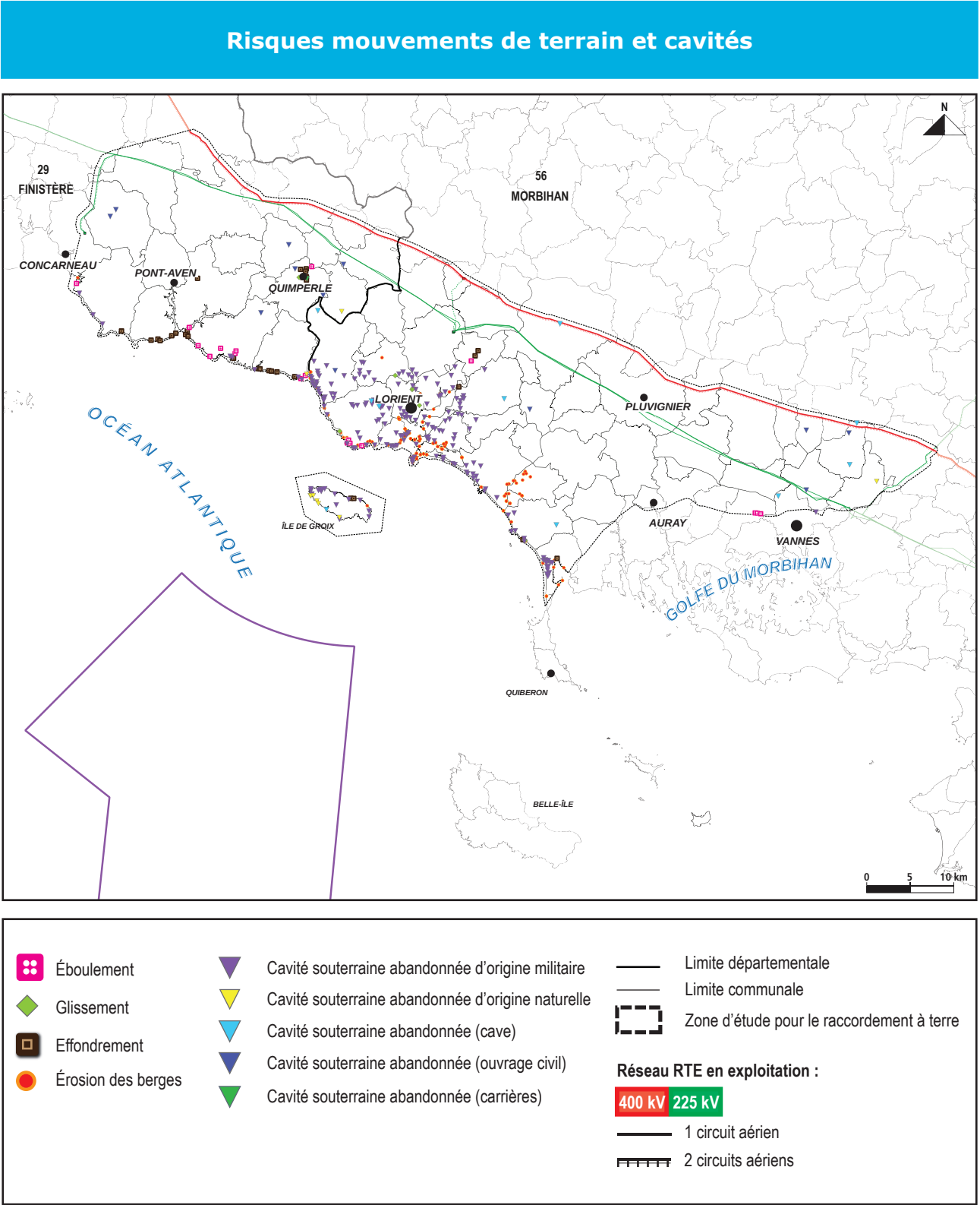
Figure 99 : Carte des mouvements de terrain et cavités
