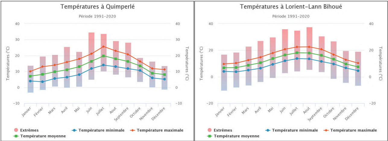
Températures sur la période de 1991-2020 à Quimperlé
