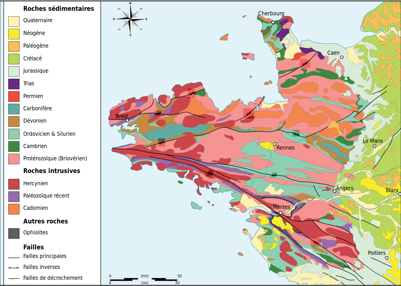
Géologie du Massif armoricain (BRGM)
