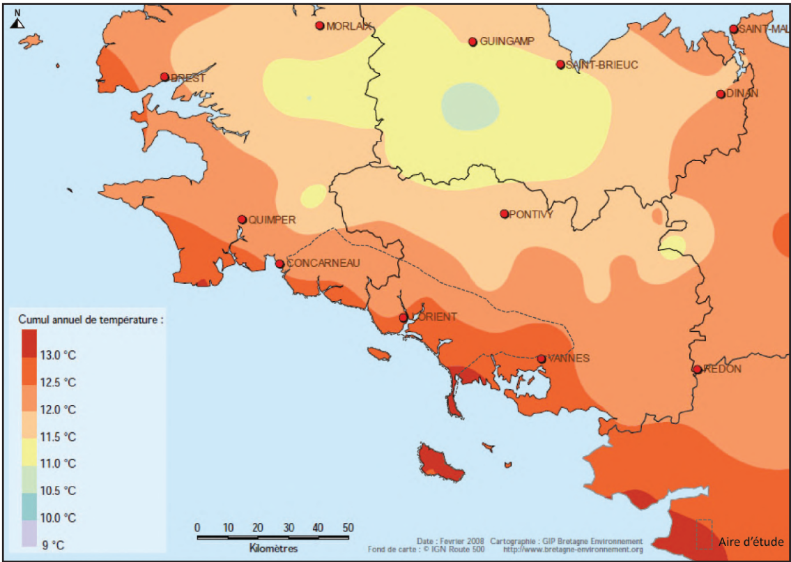
Cumul annuel de températures
