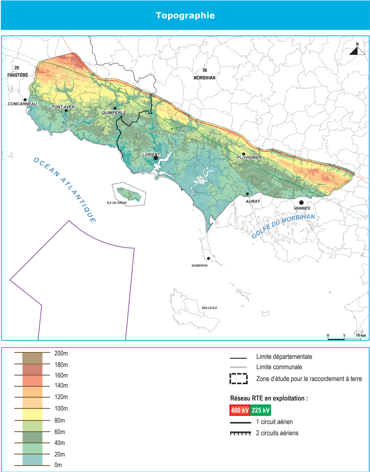
Figure 91 : Carte de la topographie
