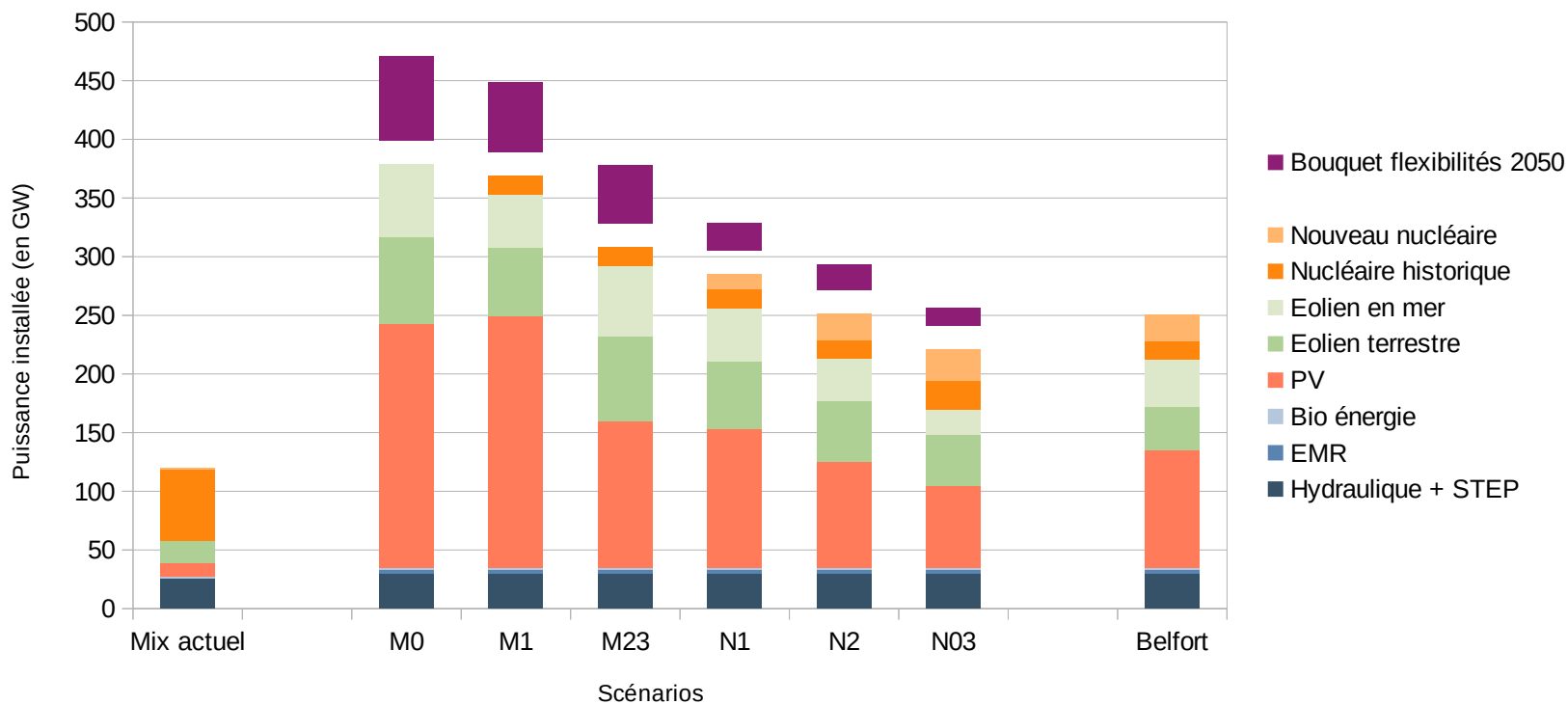
Puissance installée par filière selon les scénarios
