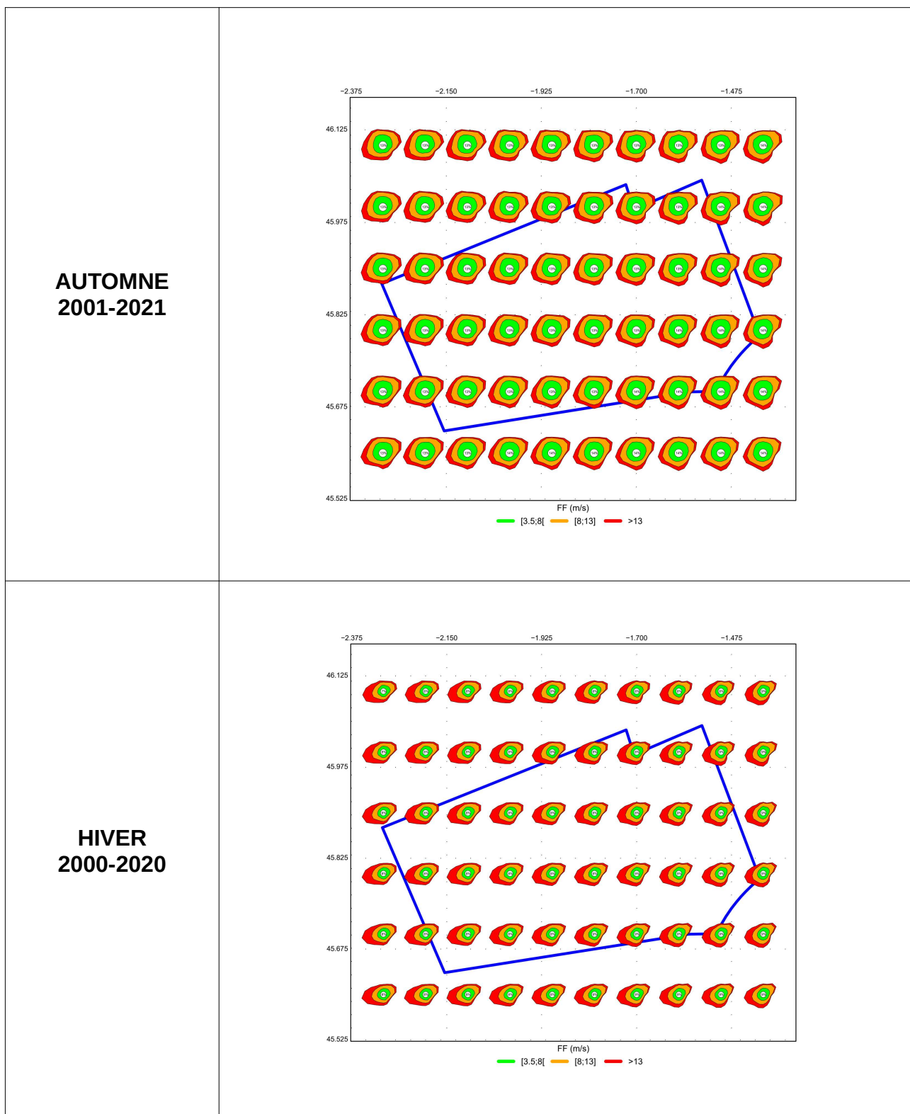
Illustration 4.39 Roses saisonnières simulées au niveau 250 m sur la zone d'intérêt
