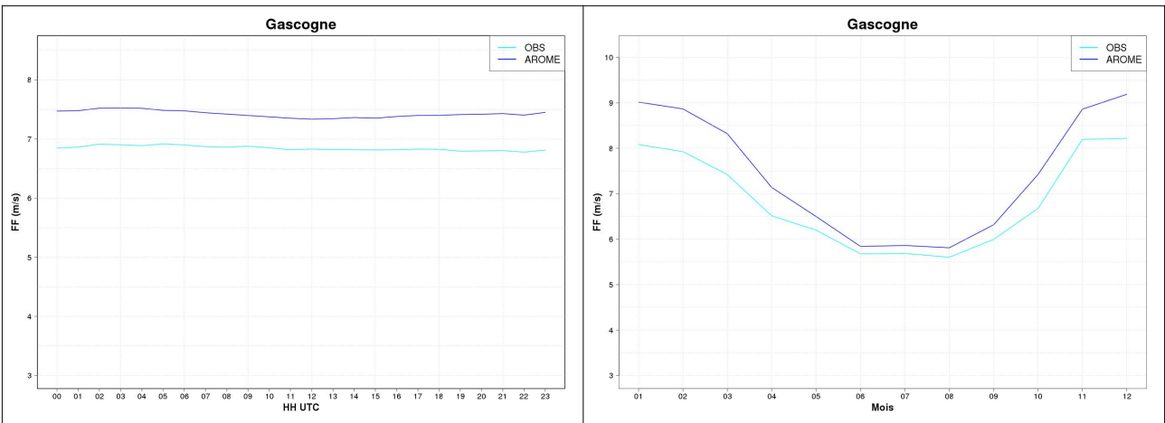
Illustration 4.25 : Forces moyennes des vents horaires en m/s du point d'observation et du point AROME 10 m par heure UTC sur le graphique de gauche et par mois sur le graphique de droite sur la période 2000-2021 (seuil plafond des forces : 25 m/s)
