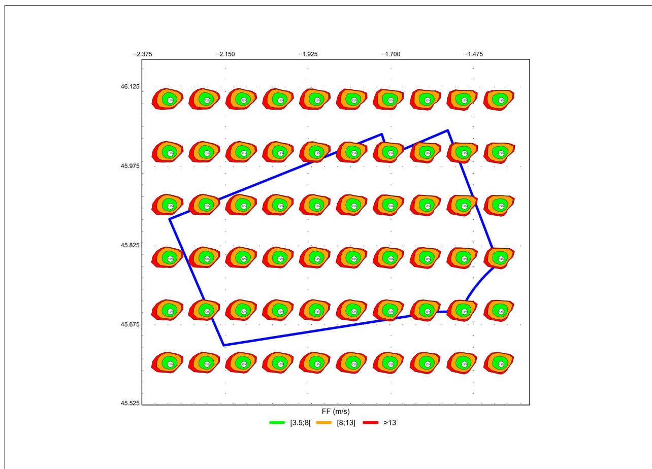
Illustration 4.38 : Roses annuelles simulées au niveau 250 m sur la zone d'intérêt (2000-2020)
