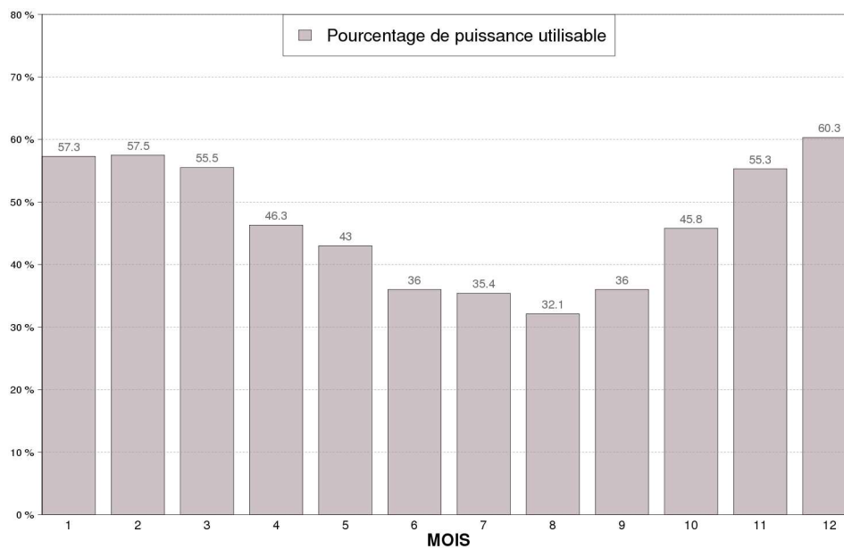
Illustration 5.3 : Facteurs de charge mensuels sur la période 2000-2021 au niveau 140 m
