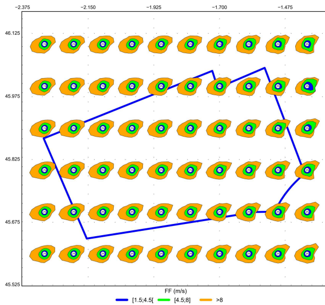
Illustration 4.30 : Roses saisonnières simulées au niveau 10 m sur la zone d'intérêt
