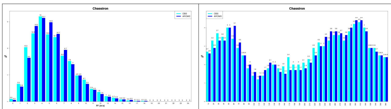
Illustration 4.6 : Comparaison des forces de vent (fréquences par m/s) à gauche et des directions (fréquences par secteur) à droite du point d'observation et du point AROME 10 m sur la période 2000-2021
