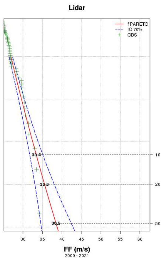
Illustration 6.3 : Graphe de durées de retour (10, 20 et 50 ans) du vent pour le point AROME Lidar à 100 m.
