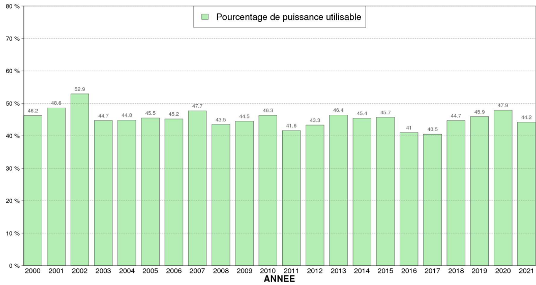
Illustration 5.4 : Facteurs de charge annuels sur la période 2000-2021 au niveau 100 m
