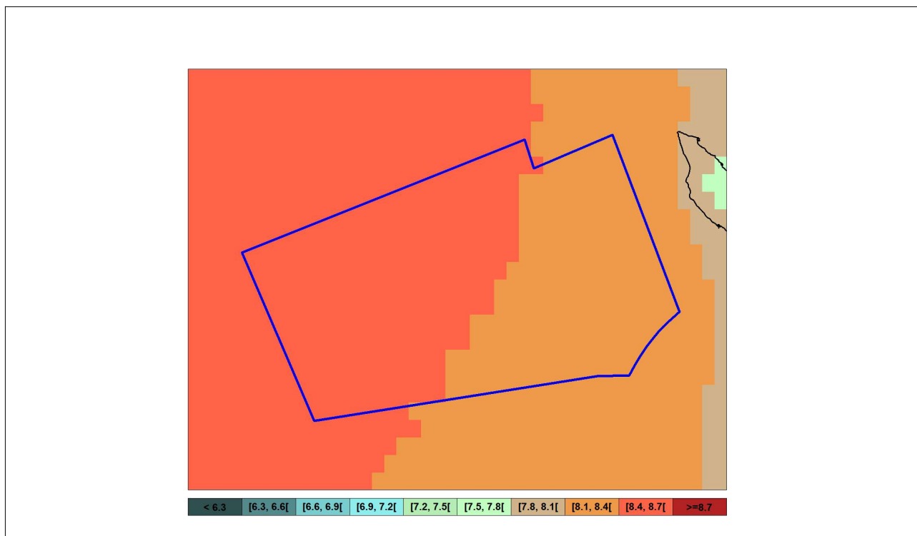
Illustration 4.37 : Forces moyennes du vent sur la zone d'intérêt au niveau 160 m sur la période 2000-2019
