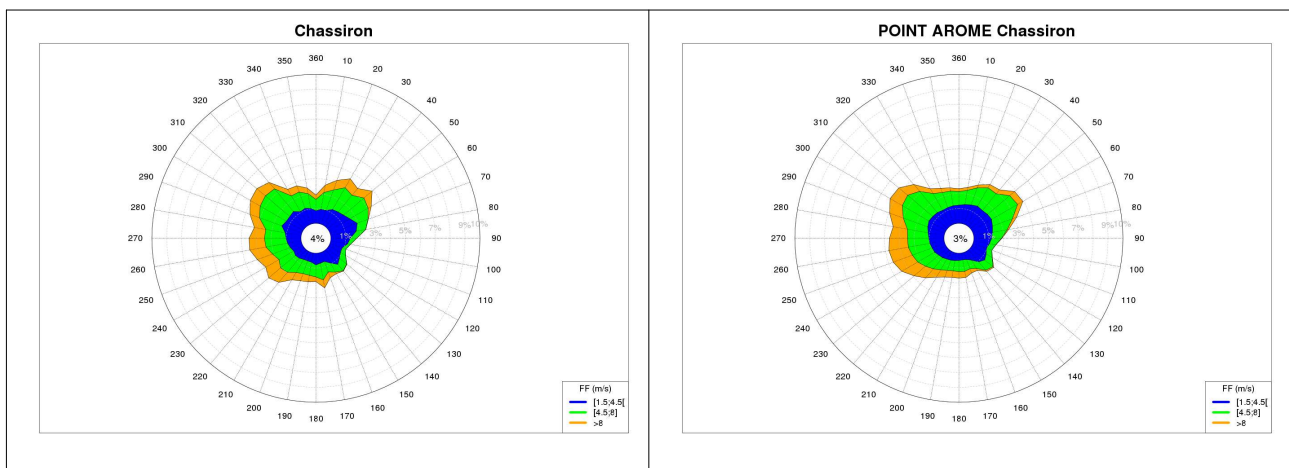
Illustration 4.4 : Roses annuelles des vents horaires du point d'observation (à gauche) et du point AROME 10 m (à droite) sur la période 2000-2021
