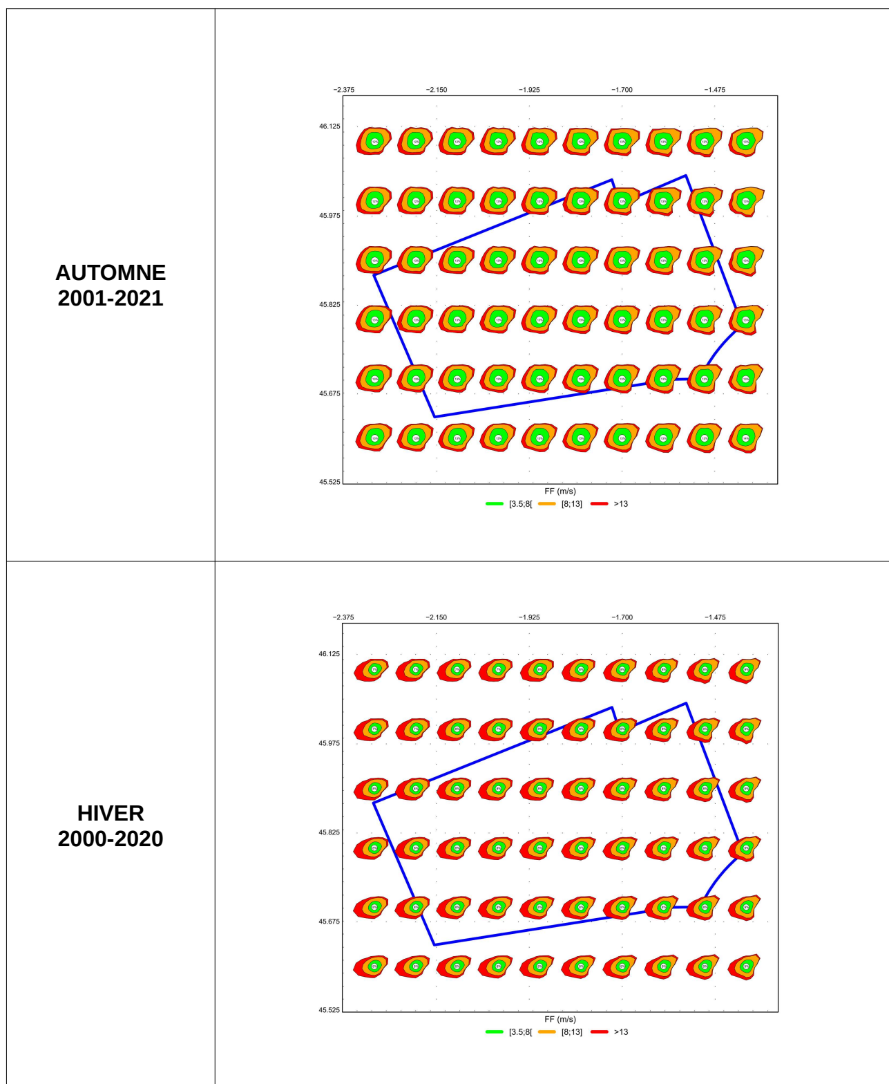
Illustration 4.36 : Roses saisonnières simulées au niveau 160 m sur la zone d'intérêt
