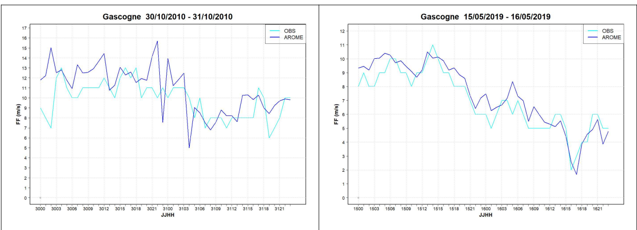
Illustration 4.26 : Forces horaires en m/s du point d'observation et du point AROME 10 m sur les périodes du 30 octobre 2010 à 00 h UTC au 31 octobre 2010 à 23 h UTC (graphique gauche) et du 15 mai 2019 à 00 h UTC au 16 mai 2019 à 23 h UTC (graphique droit)
