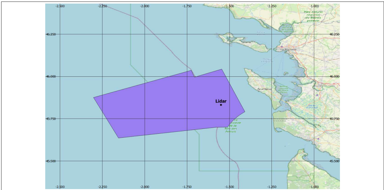
Illustration 1.3 : Localisation du lidar sur la zone offshore de l'AO7
