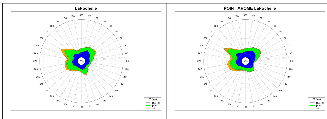
Illustration 4.10 : Roses annuelles des vents horaires du point d'observation (à gauche) et du point AROME 10 m (à droite) sur la période 2000-2021
