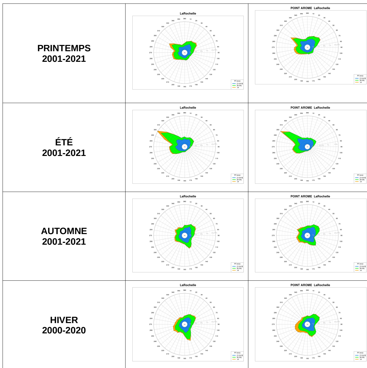
Illustration 4.11 : Roses saisonnières des vents horaires du point d'observation (à gauche) et du point AROME (à droite) sur la période 2000-2021
