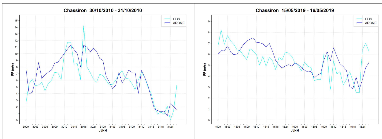
Illustration 4.8 : Forces horaires en m/s du point d'observation et du point AROME 10 m sur les périodes du 30 octobre 2010 à 00 h UTC au 31 octobre 2010 à 23 h UTC (graphique gauche) et du 15 mai 2019 à 00 h UTC au 16 mai 2019 à 23 h UTC (graphique droit)
