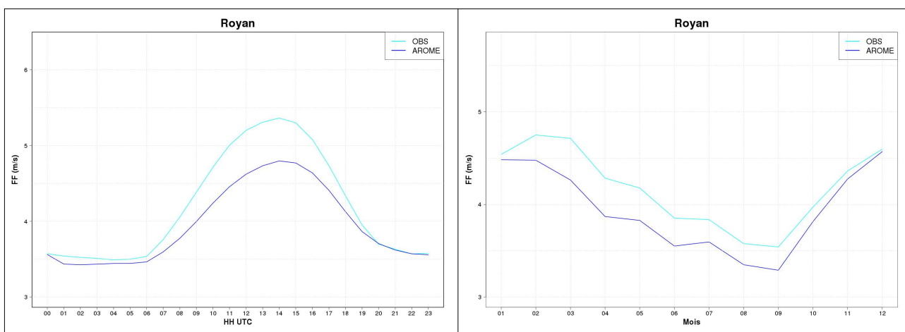
Illustration 4.19 : Forces moyennes des vents horaires en m/s du point d'observation et du point AROME 10 m par heure UTC sur le graphique de gauche et par mois sur le graphique de droite sur la période 2000-2021 (seuil plafond des forces : 25 m/s)
