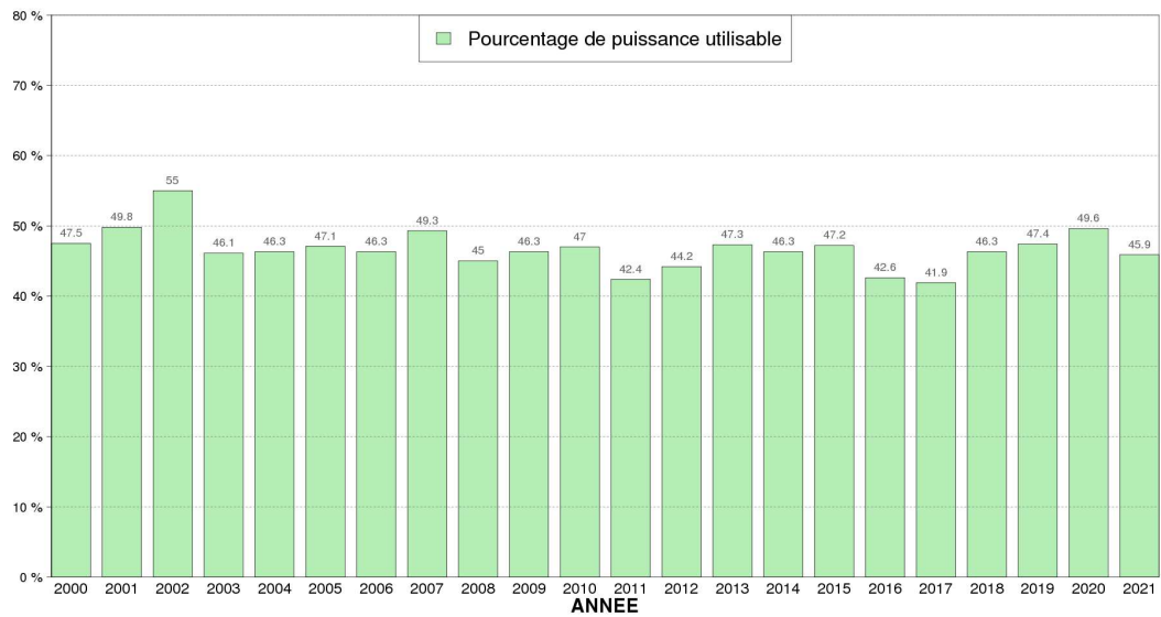
Illustration 5.5 : Facteurs de charge annuels sur la période 2000-2021 au niveau 140 m
