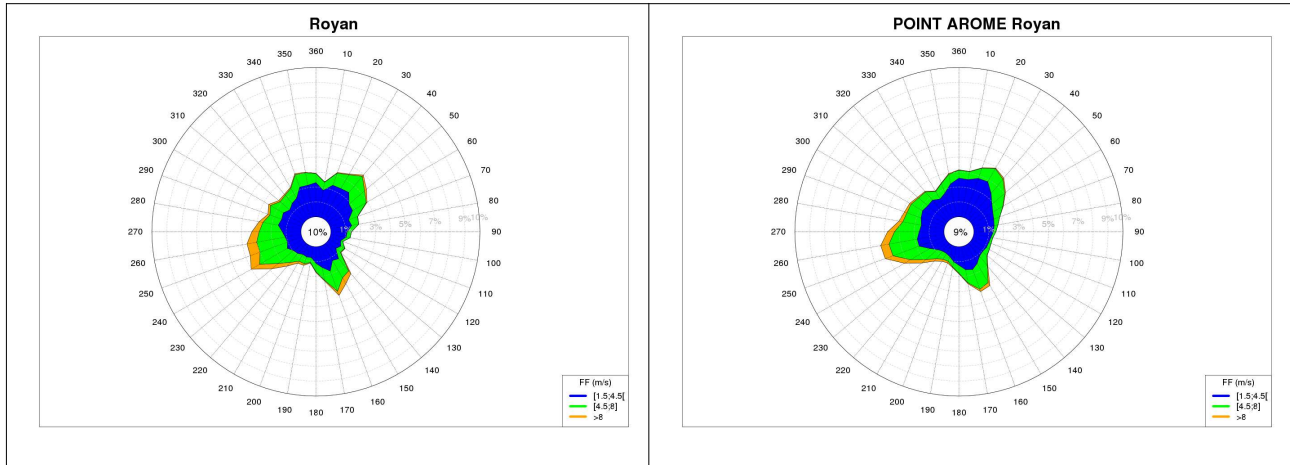
Illustration 4.16 : Roses annuelles des vents horaires du point d'observation (à gauche) et du point AROME 10 m (à droite) sur la période 2000-2021
