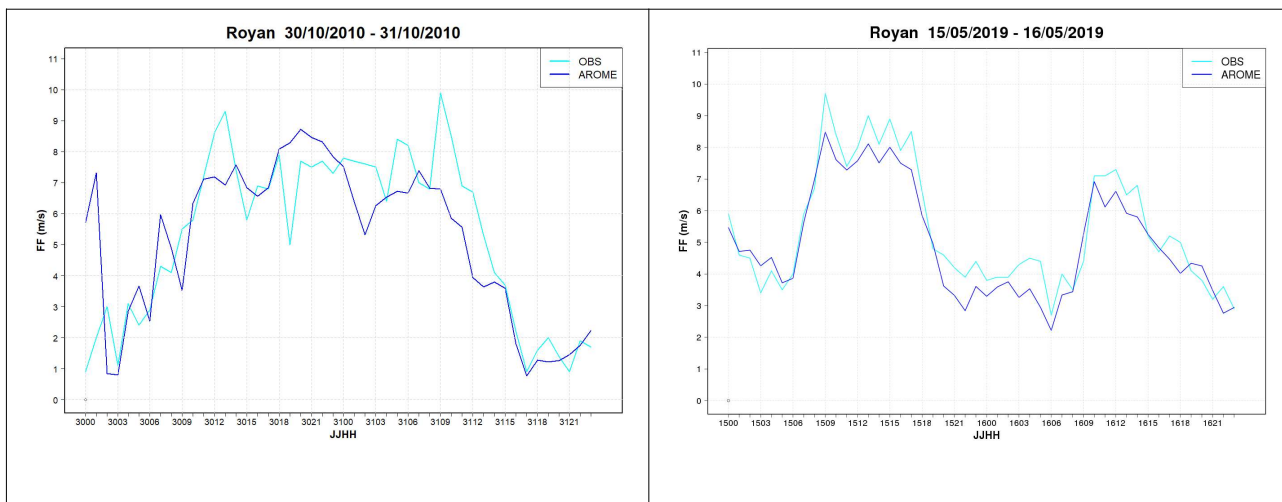
Illustration 4.20 : Forces horaires en m/s du point d'observation et du point AROME 10 m sur les périodes du 30 octobre 2010 à 00 h UTC au 31 octobre 2010 à 23 h UTC (graphique gauche) et du 15 mai 2019 à 00 h UTC au 16 mai 2019 à 23 h UTC (graphique droit)
