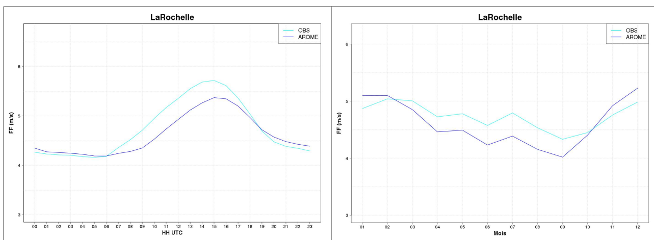
Illustration 4.13 : Forces moyennes des vents horaires en m/s du point d'observation et du point AROME 10 m par heure UTC sur le graphique de gauche et par mois sur le graphique de droite sur la période 2000-2021 (seuil plafond des forces : 25 m/s)
