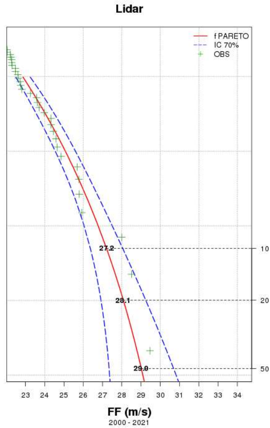
Illustration 6.2 : Graphe de durées de retour (10, 20 et 50 ans) du vent pour le point AROME Lidar à 10 m.
