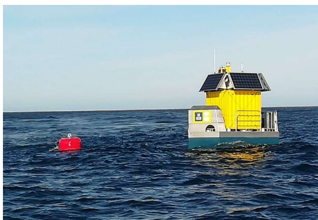
Illustration 1.2 : Photo d'une bouée exploitée par Akrocéan du même type que celle installée sur le site de l'AO7. Cette bouée embarque notamment un LIDAR, une station météorologique et des capteurs océanographiques.
