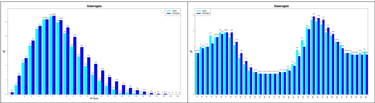
Illustration 4.24 : Comparaison des forces de vent (fréquences par m/s) à gauche et des directions (fréquences par secteur) à droite du point d'observation et du point AROME 10 m sur la période 2000-2021
