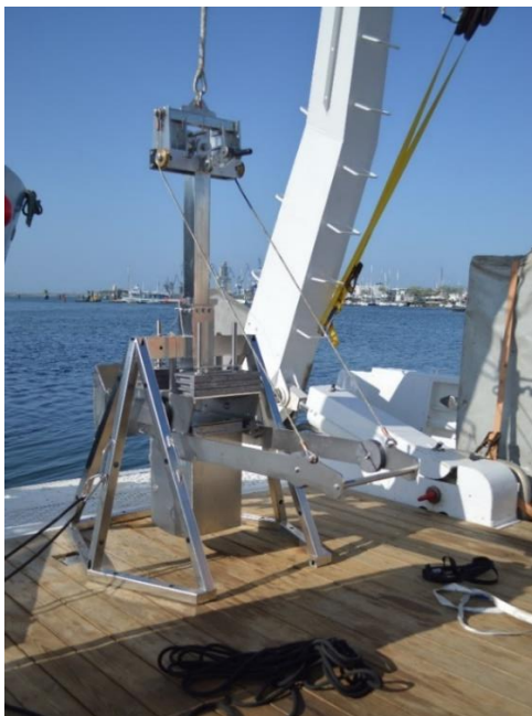
Photo 2 : Carottier boîte (source : setec énergie environnement, 2023)
