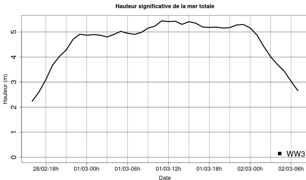
Illustration 3.16: Evolution temporelle de Hs au point de grille 43,02° N et 3,55° E – tempête du 01 et 02/03/18
