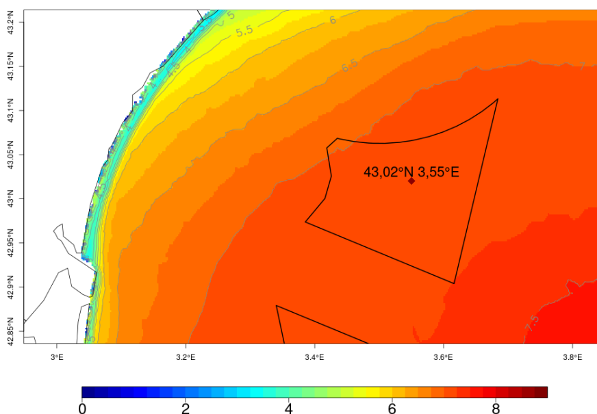
Illustration 3.5: Hauteur significative de la mer totale ( H_s , en mètres) lors de la tempête des 3 et 4/12/03 (valeur maximale intégrée sur la période comprise entre le 3 déc. à 09 UTC et le 04 déc. à 21 UTC)
