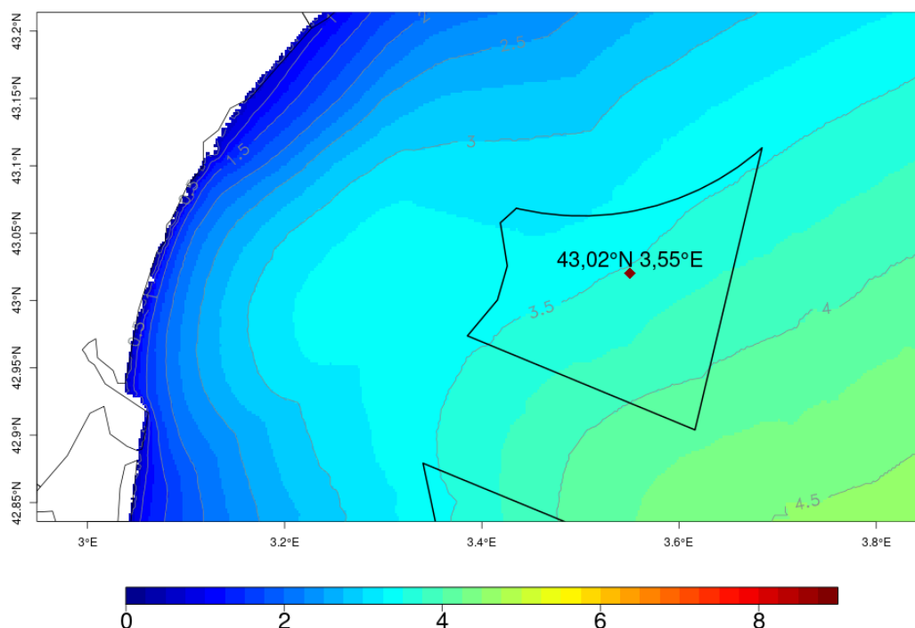
Illustration 3.11: Hauteur significative de la mer totale (Hs, en mètres) lors de la tempête du 24/01/09 (valeur maximale intégrée sur la période comprise entre le 24 jan. à 03 UTC et le 25 jan. à 06 UTC)
