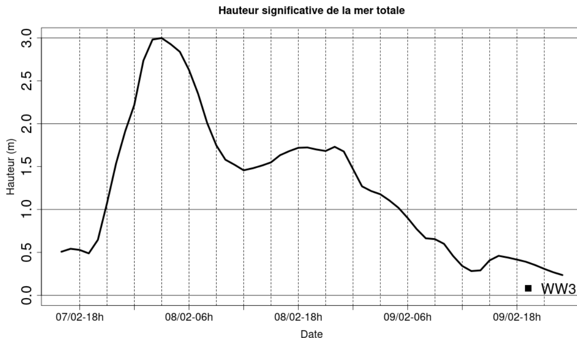
Illustration 3.2: Evolution temporelle de Hs au point de grille 43,02° N et 3,55° E – tempête du 08/02/96
