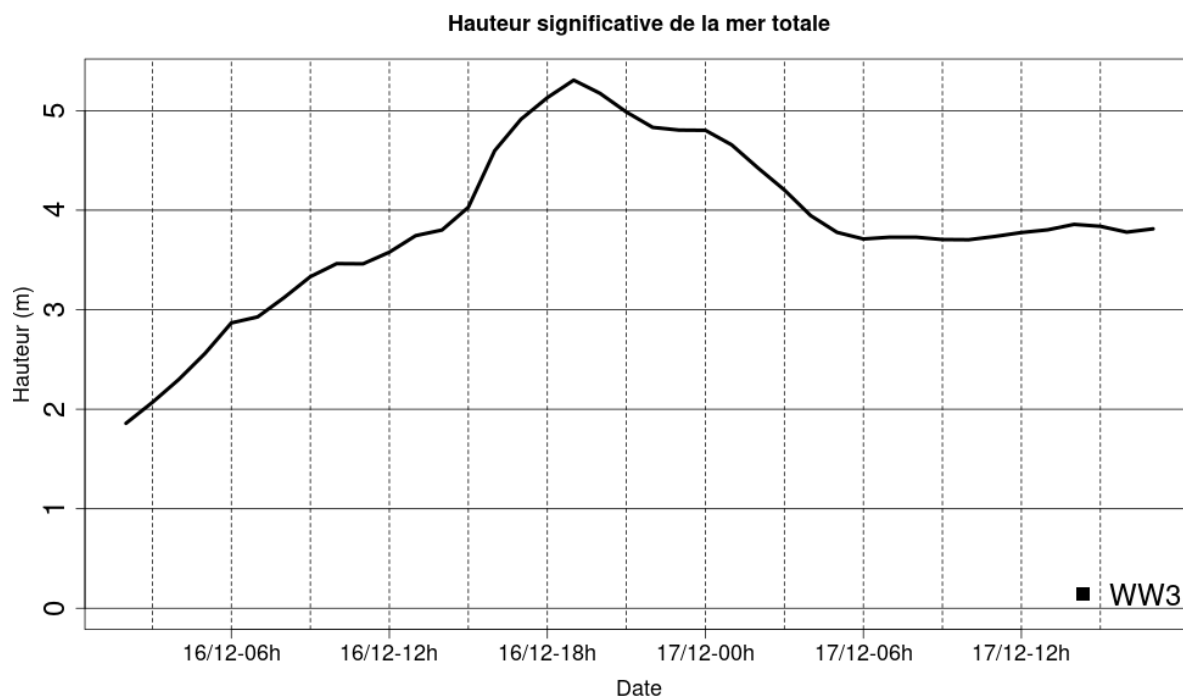
Illustration 3.4: Evolution temporelle de Hs au point de grille 43,02° N et 3,55° E – tempête des 16 et 17/12/97
