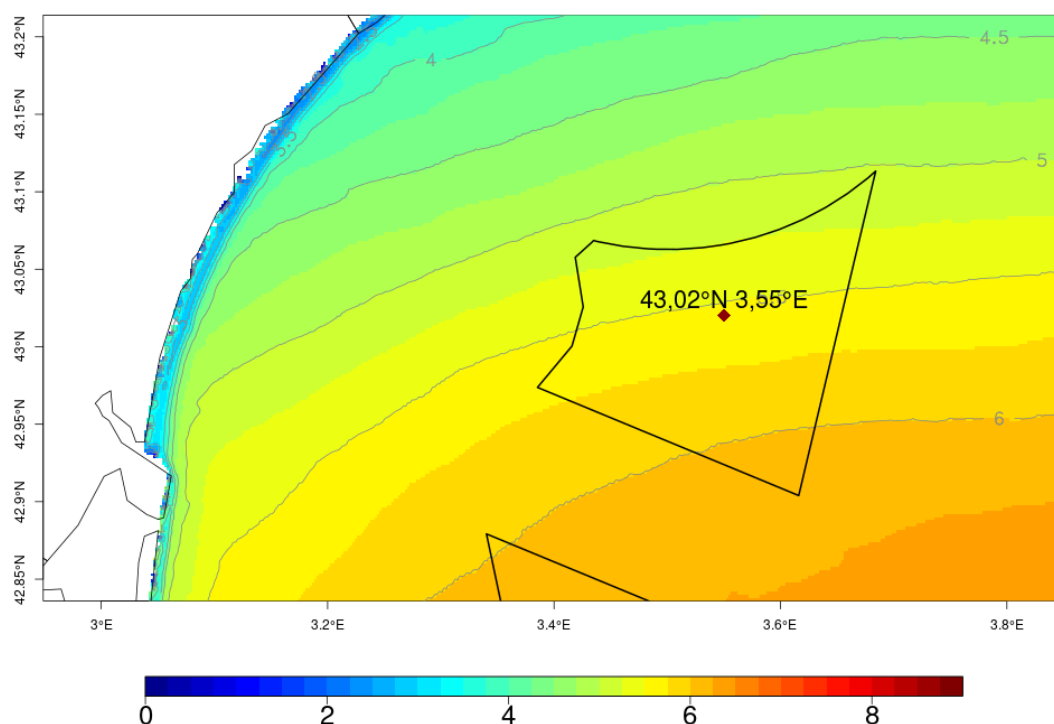
Illustration 3.9: Hauteur significative de la mer totale ( H_s , en mètres) lors de la tempête des 26 et 27/12/08 (valeur maximale intégrée sur la période comprise entre le 26 déc. à 03 UTC et le 27 déc. à 21 UTC)
