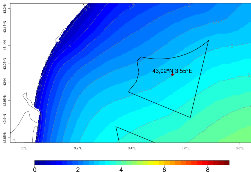
Illustration 3.1: Hauteur significative de la mer totale (Hs, en mètres) lors de la tempête du 08/02/96 (valeur maximale intégrée sur la période comprise entre le 07 fév. à 18 UTC et le 09 fév. à 21 UTC)
