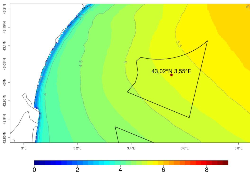
Illustration 3.3: Hauteur significative de la mer totale (Hs, en mètres) lors de la tempête des 16 et 17/12/97 (valeur maximale intégrée sur la période comprise entre le 16 déc. à 03 UTC et le 17 déc. à 15 UTC)
