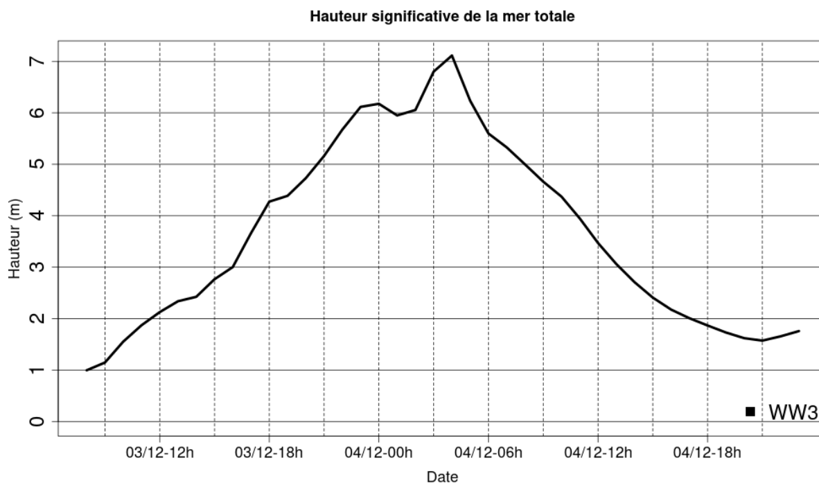
Illustration 3.6: Evolution temporelle de Hs au point de grille 43,02° N et 3,55° E – tempête des 3 et 4/12/03
