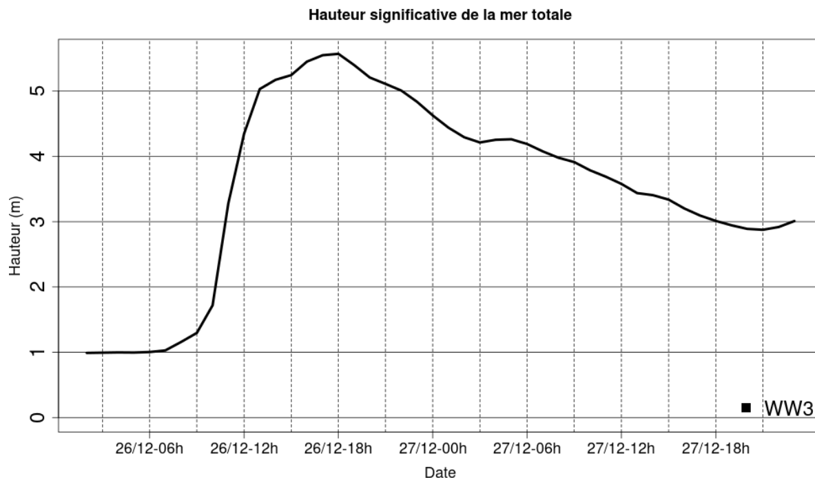
Illustration 3.10: Evolution temporelle de Hs au point de grille 43,02° N et 3,55° E – tempête des 26 et 27/12/08
