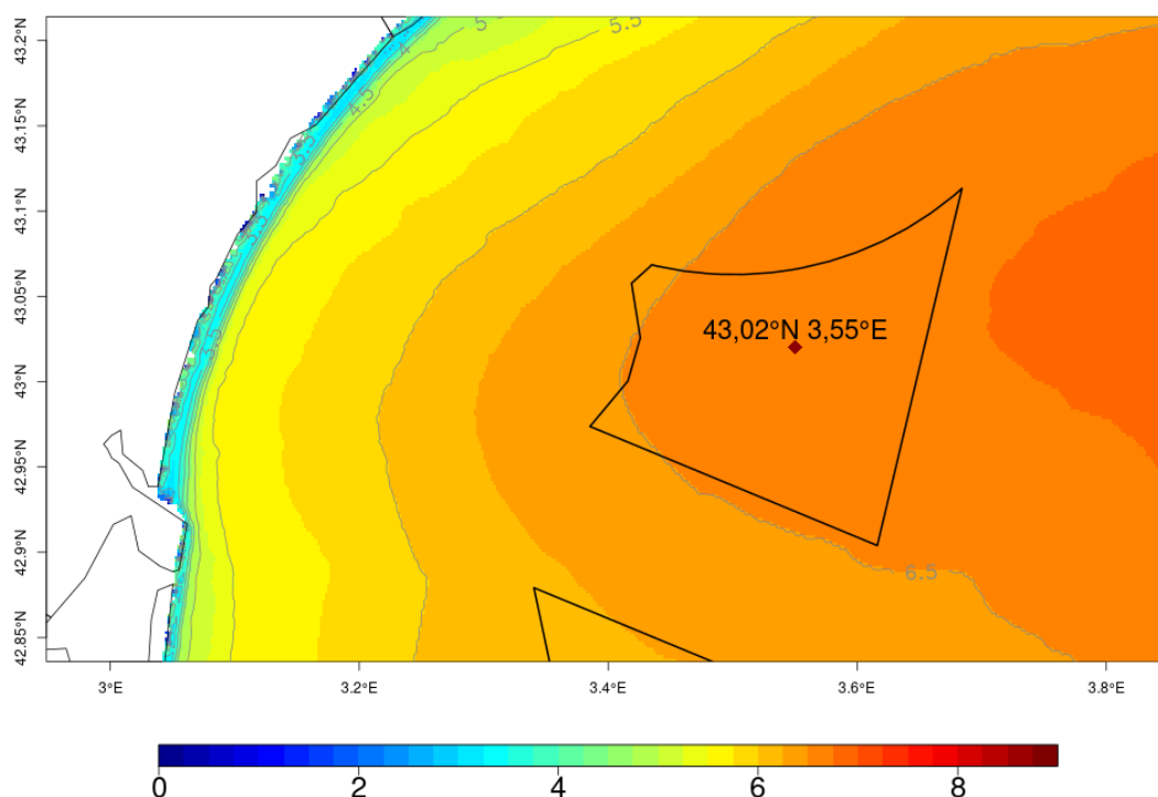
Illustration 3.13: Hauteur significative de la mer totale (Hs, en mètres) lors de la tempête du 06/03/13 (valeur maximale intégrée sur la période comprise entre le 5 mars à 15 UTC et le 07 mars à 03 UTC)
