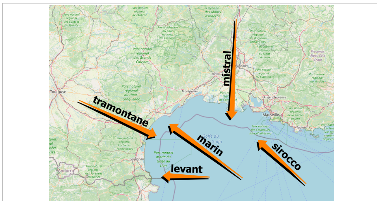
Illustration 2.1 : Principaux régimes de vent sur le bassin méditerranéen occidental
