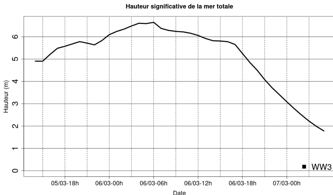
Illustration 3.14: Evolution temporelle de Hs au point de grille 43,02° N et 3,55° E – tempête du 06/03/13
