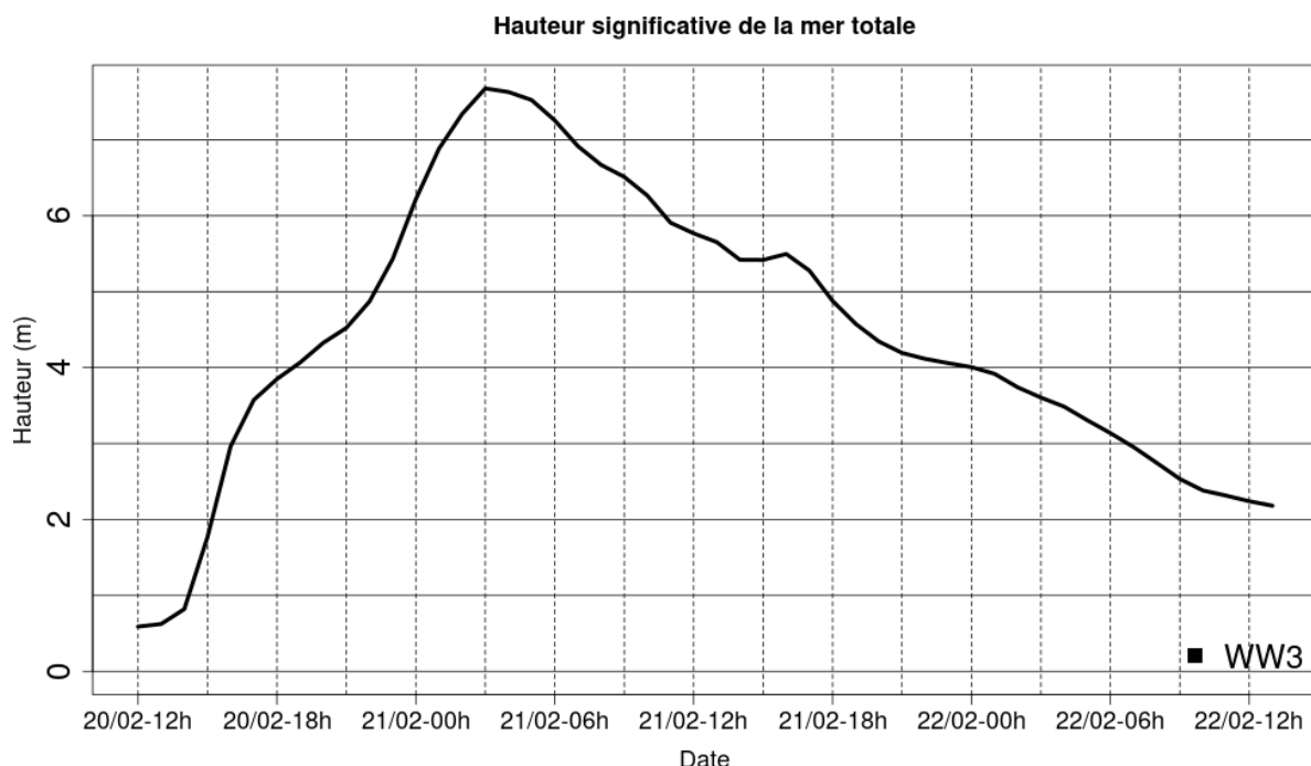
Illustration 3.8: Evolution temporelle de Hs au point de grille 43,02° N et 3,55° E – tempête des 20 et 21/02/04
