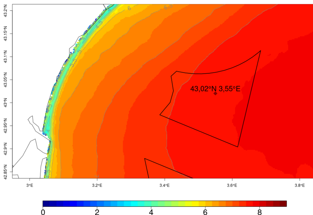
Illustration 3.7: Hauteur significative de la mer totale ( H_s , en mètres) lors de la tempête des 20 et 21/02/04 (valeur maximale intégrée sur la période comprise entre le 20 déc. à 12UTC et le 22 déc. à 12 UTC)
