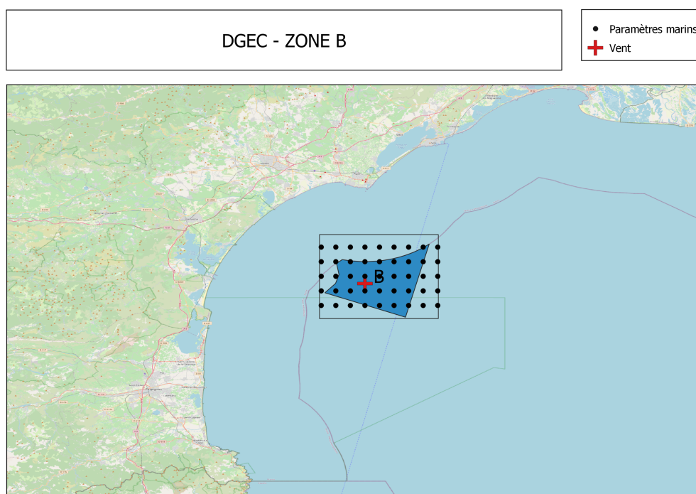
Illustration 2.2: Localisation de la zone d'étude B (zone bleue) par rapport aux points de grille des deux réanalyses : ERA5 (croix rouge) et Med-WAV (points noirs).
