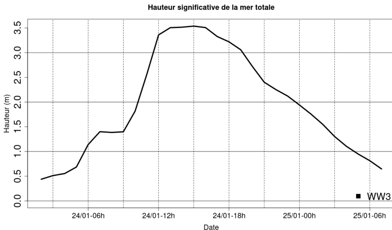
Illustration 3.12: Evolution temporelle de Hs au point de grille 43,02° N et 3,55° E – tempête du 24/01/09
