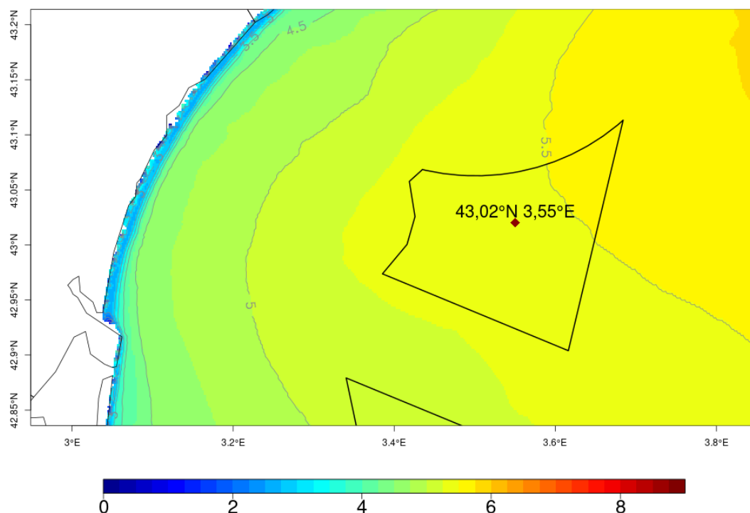
Illustration 3.15: Hauteur significative de la mer totale (Hs, en mètres) lors de la tempête du 01 et 02/03/18 (valeur maximale intégrée sur la période comprise entre le 28 fév. à 18 UTC et le 02 mars à 06 UTC)
