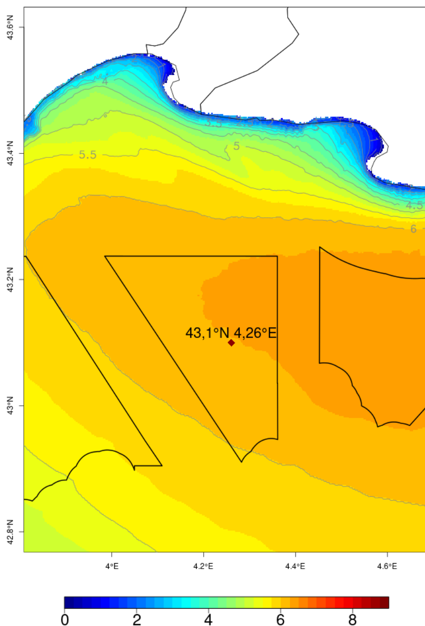
Illustration 3.1: Hauteur significative de la mer totale (Hs, en mètres) lors de la tempête des 16 et 17/12/97 (valeur maximale intégrée sur la période comprise entre le 16 déc. à 03 UTC et le 17 déc. à 15 UTC)
