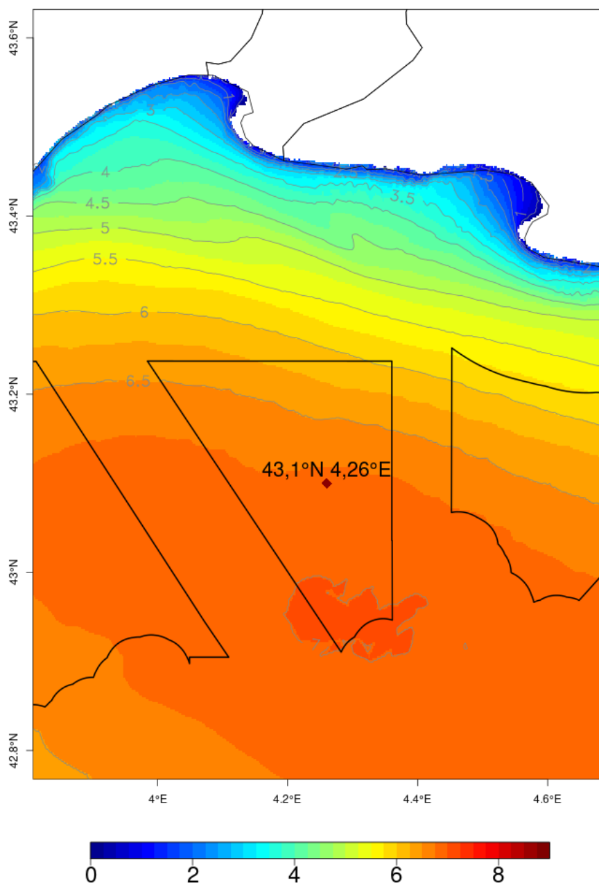
Illustration 3.9: Hauteur significative de la mer totale ( H_s , en mètres) lors de la tempête du 06/03/13 (valeur maximale intégrée sur la période comprise entre le 05 mars à 15UTC et le 07 mars à 03 UTC)
