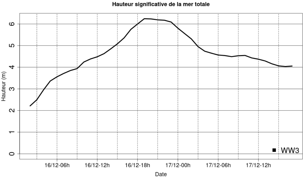
Illustration 3.2: Evolution temporelle de Hs au point de grille 43,10° N et 4,26° E – tempête des 16 et 17/12/97
