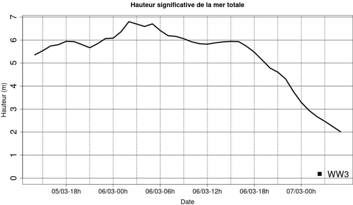
Illustration 3.10: Evolution temporelle de Hs au point de grille 43,10° N et 4,26° E – tempête du 06/03/13
