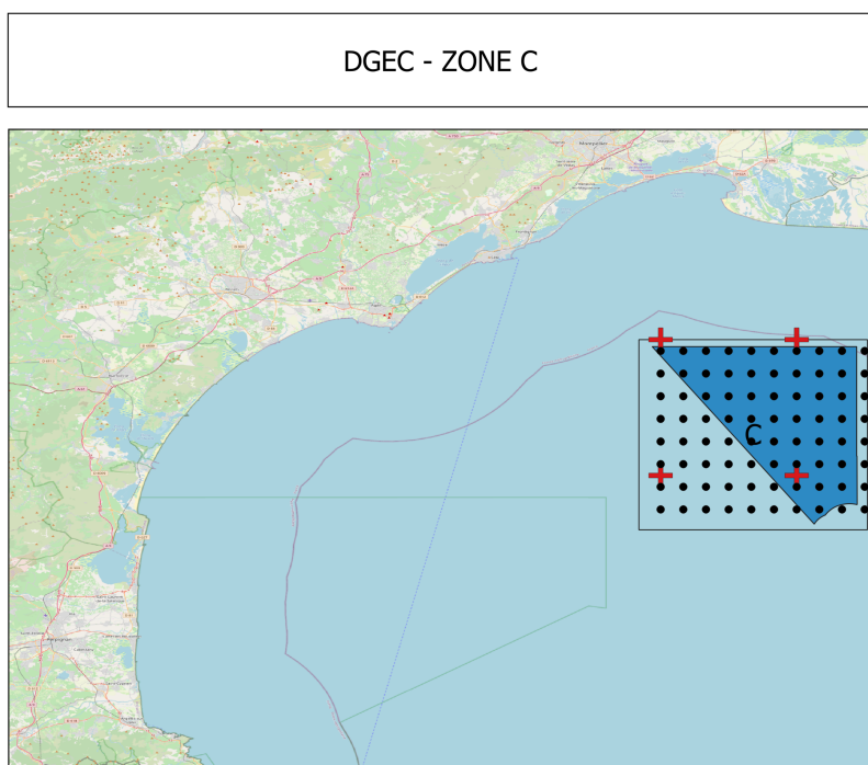
Illustration 2.2: Localisation de la zone d'étude C (zone bleue) par rapport aux points de grille des deux réanalyses : ERA5 (croix rouge) et Med-WAV (points noirs).
