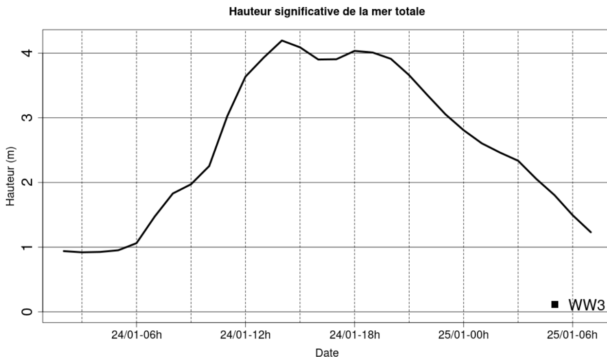
Illustration 3.8: Evolution temporelle de Hs au point de grille 43,10° N et 4,26° E – tempête du 24/01/09
