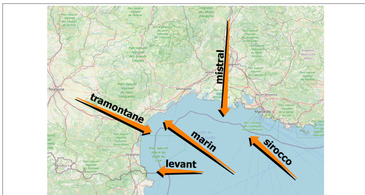
Illustration 2.1 : Principaux régimes de vent sur le bassin méditerranéen occidental
