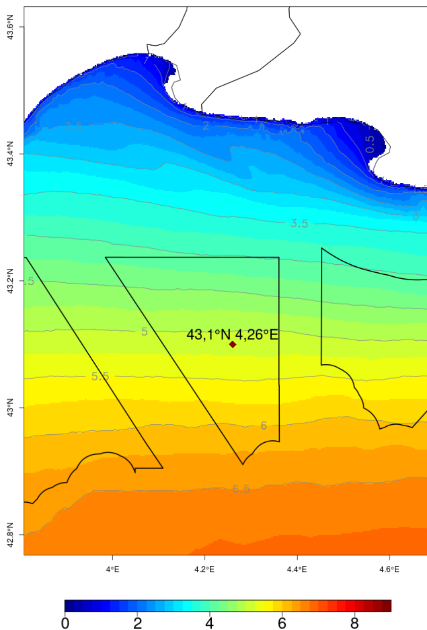
Illustration 3.5: Hauteur significative de la mer totale ( H_s , en mètres) lors de la tempête des 26 et 27/12/08 (valeur maximale intégrée sur la période comprise entre le 26 déc. à 03 UTC et le 27 déc. à 21 UTC)
