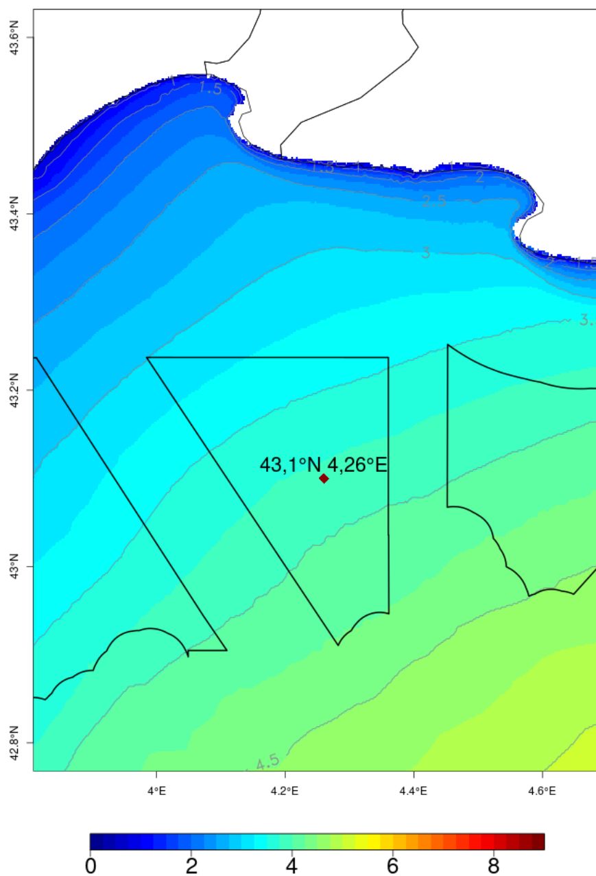
Illustration 3.11: Hauteur significative de la mer totale ( H_s , en mètres) lors de la tempête du 06/03/17 (valeur maximale intégrée sur la période comprise entre le 06 mars à 00 UTC et le 07 mars à 03 UTC)
