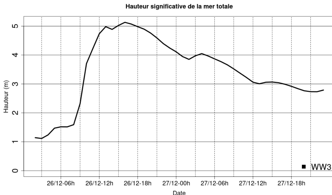
Illustration 3.6: Evolution temporelle de Hs au point de grille 43,10° N et 4,26° E – tempête des 26 et 27/12/08
