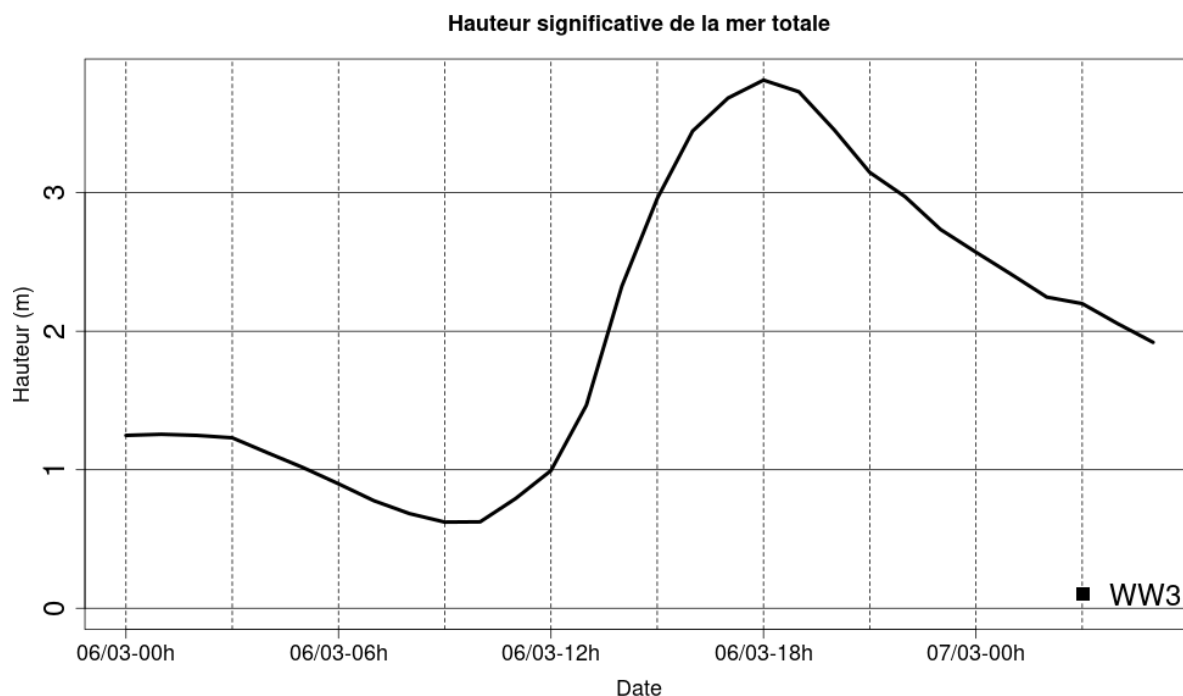
Illustration 3.12: Evolution temporelle de IHS au point de grille 43,10° N et 4,26° E – tempête du 06/03/17
