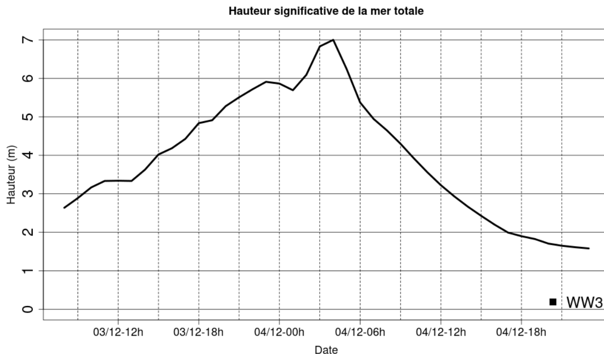
Illustration 3.4: Evolution temporelle de Hs au point de grille 43,10° N et 4,26° E – tempête des 3 et 4/12/03
