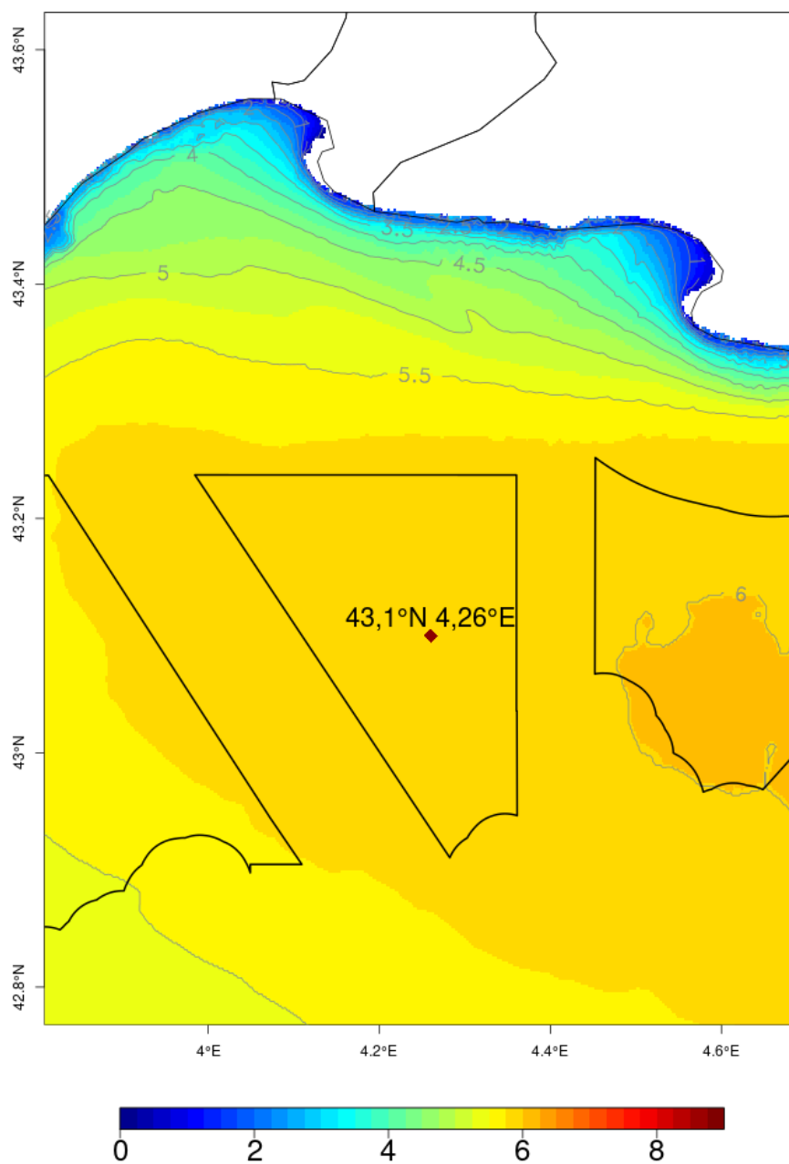
Illustration 3.13: Hauteur significative de la mer totale ( H_s , en mètres) lors de la tempête du 01 et 02/03/18 (valeur maximale intégrée sur la période comprise entre le 28 fév. à 18 UTC et le 02 mars à 06 UTC)
