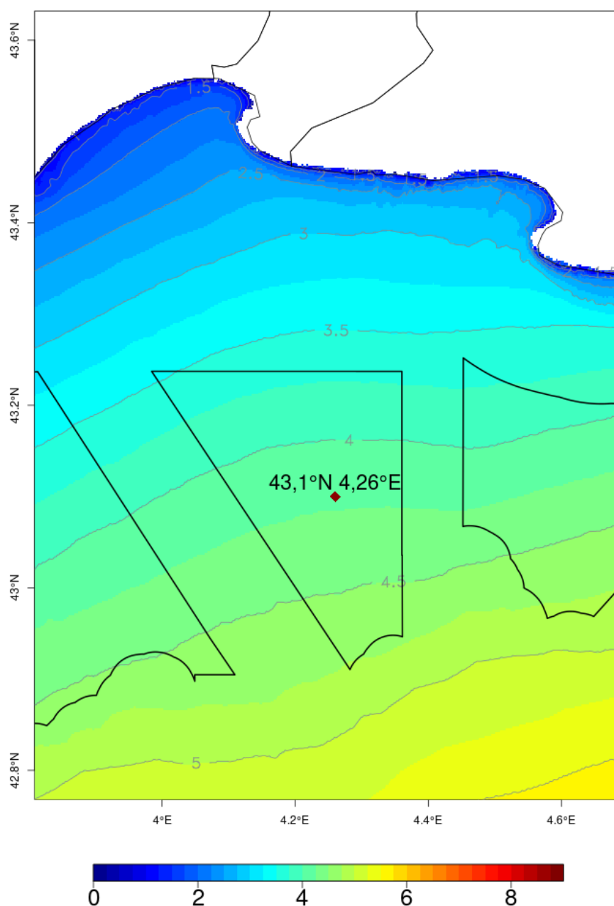
Illustration 3.7: Hauteur significative de la mer totale ( H_s , en mètres) lors de la tempête du 24/01/09 (valeur maximale intégrée sur la période comprise entre le 24 jan. à 03 UTC et le 25 jan. à 06 UTC)
