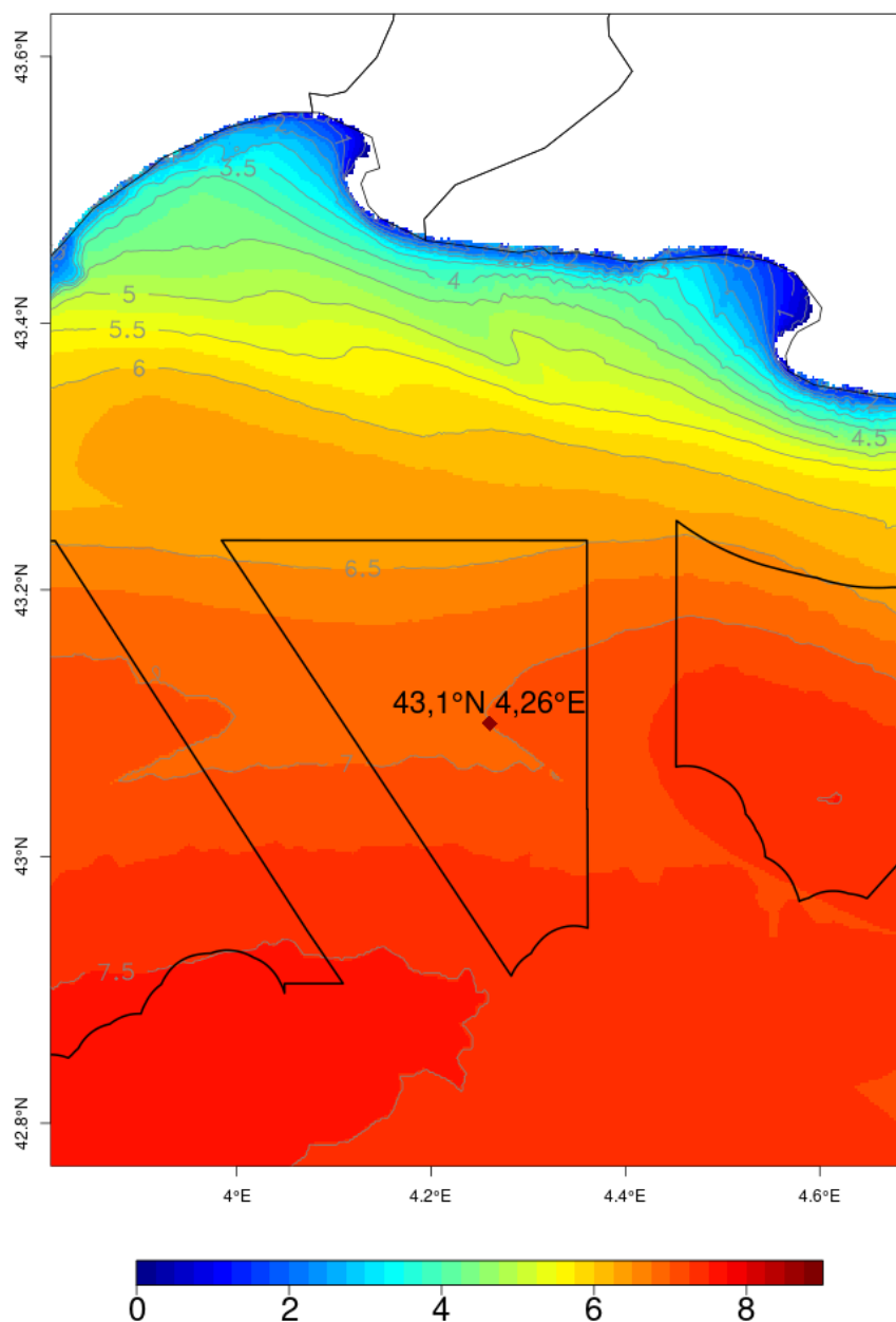
Illustration 3.3: Hauteur significative de la mer totale (Hs, en mètres) lors de la tempête des 3 et 4/12/03 (valeur maximale intégrée sur la période comprise entre le 03 déc. à 09 UTC et le 04 déc. à 21 UTC)
