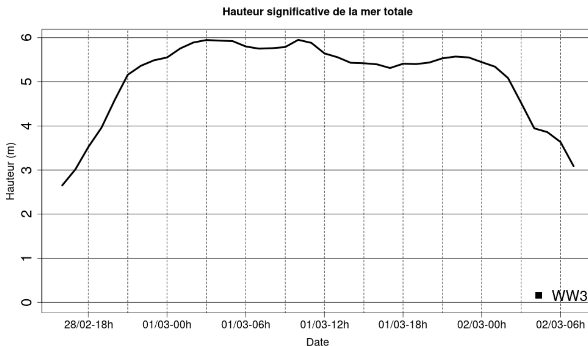
Illustration 3.14: Evolution temporelle de Hs au point de grille 43,10° N et 4,26° E – tempête du 01 et 02/03/18
