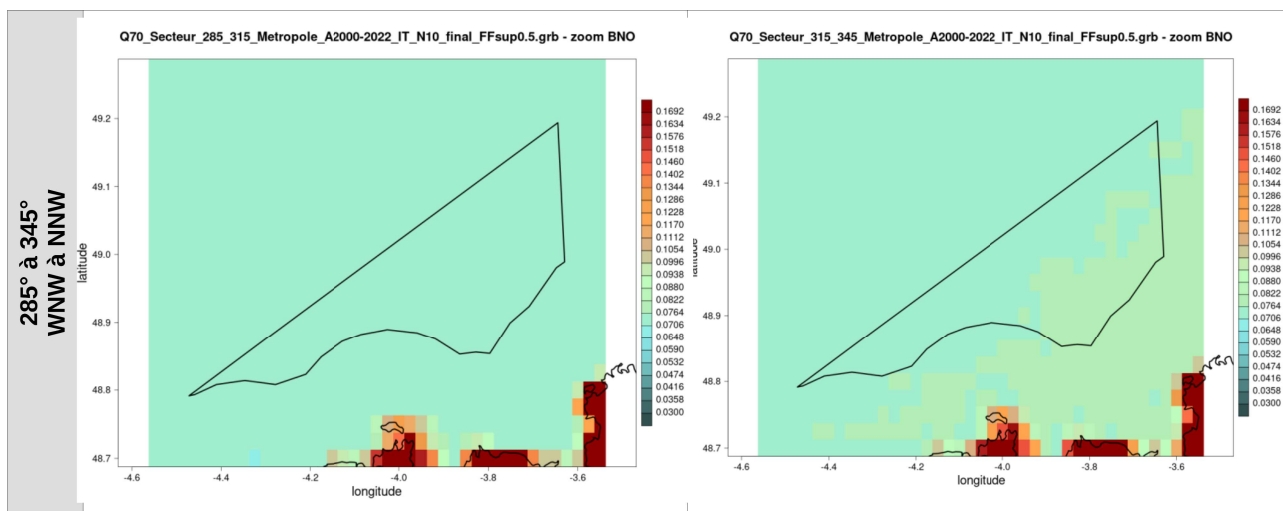
Illustration 18 : cartes des Q70 de l'intensité de turbulence au niveau 10 m par secteur de direction de 30° pour la zone BNO, calculés à partir des données AROME (2000-2022)
