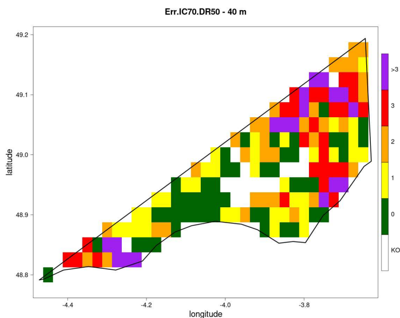
Illustration 34 : carte des quantiles de durées de retour 50 ans des rafales estimées à 40 m pour la zone BNO, calculés à partir des données AROME (2000-2022)
