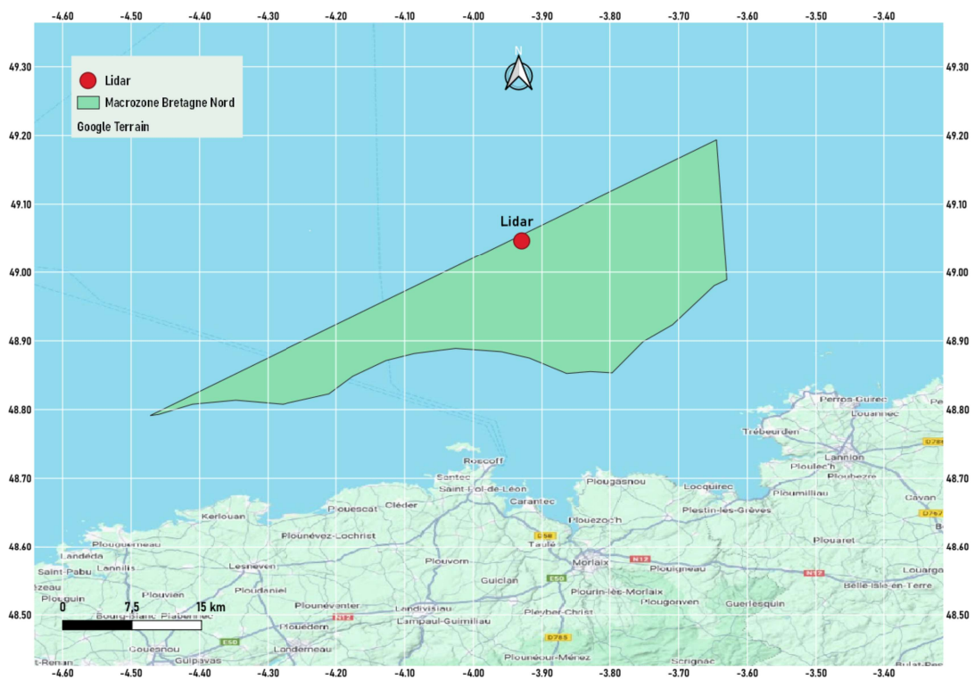
Illustration 1 : localisation de la zone Bretagne nord-ouest (BNO)
