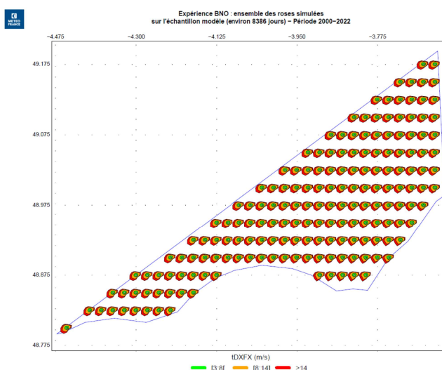
Illustration 27 : roses des vents de rafales estimées à 40 m sur la zone BNO sur la période 2000-2022
