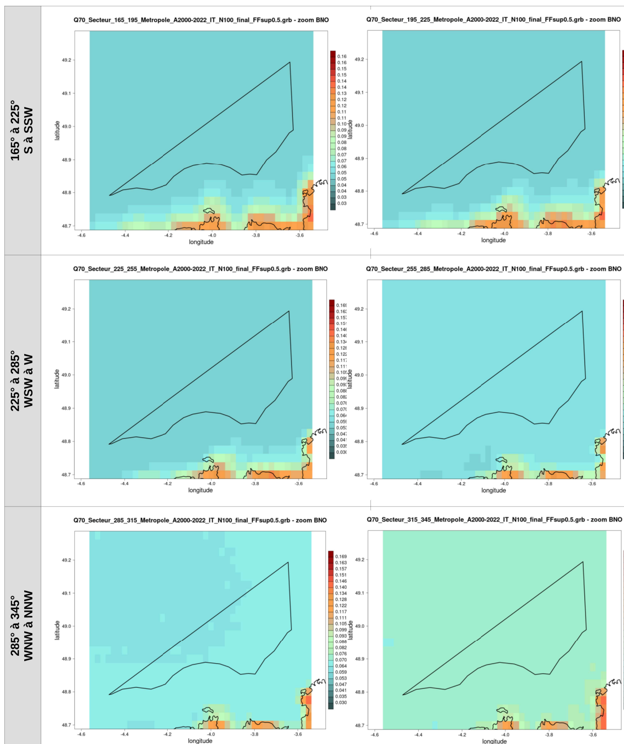
Illustration 4 : cartes des Q70 de l'intensité de turbulence au niveau 100 m par secteur de direction de 30° pour la zone BNO, calculés à partir des données AROME (2000-2022)
