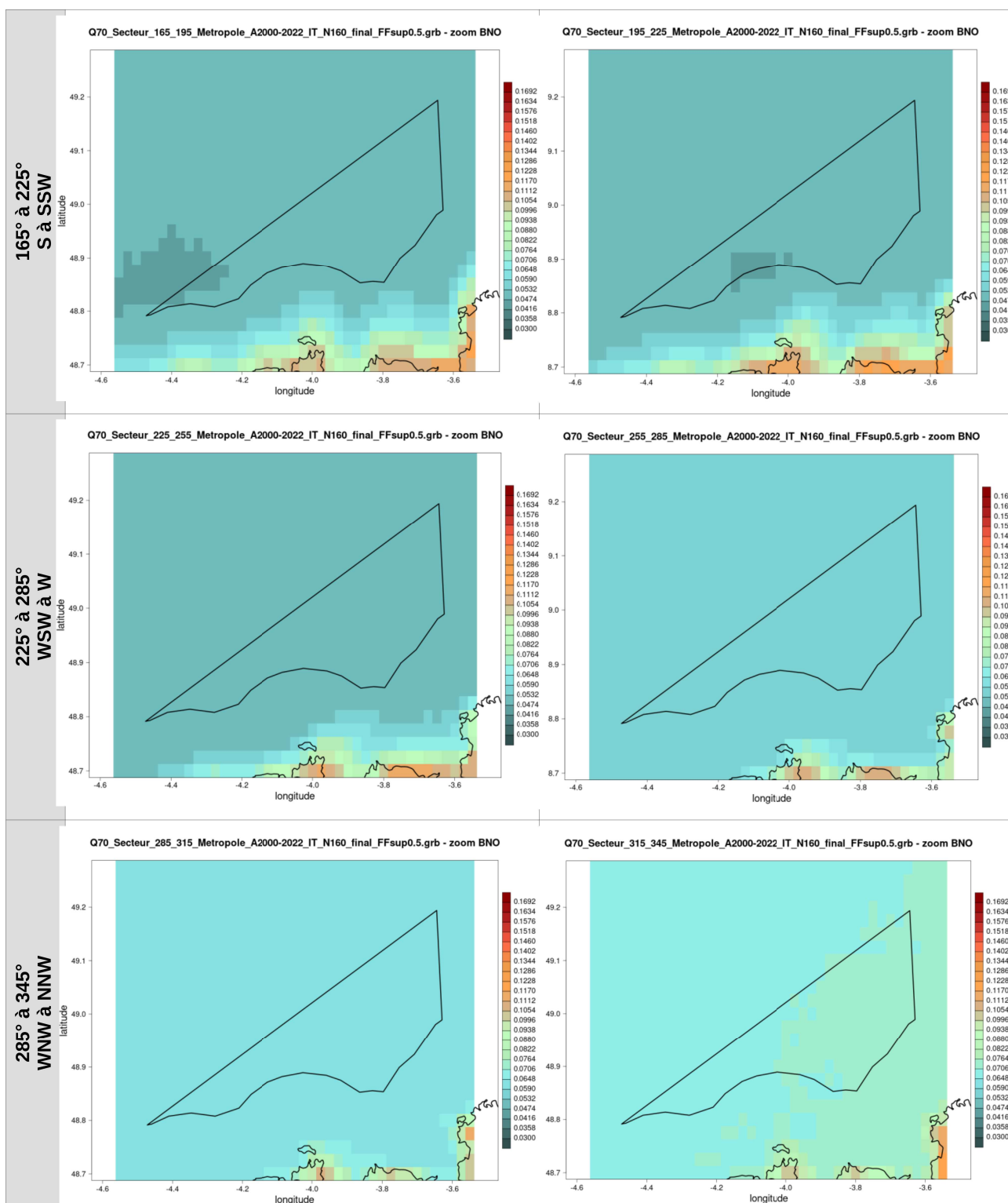
Illustration 20 : cartes des Q70 de l'intensité de turbulence au niveau 160 m par secteur de direction de 30° pour la zone BNO, calculés à partir des données AROME (2000-2022)
