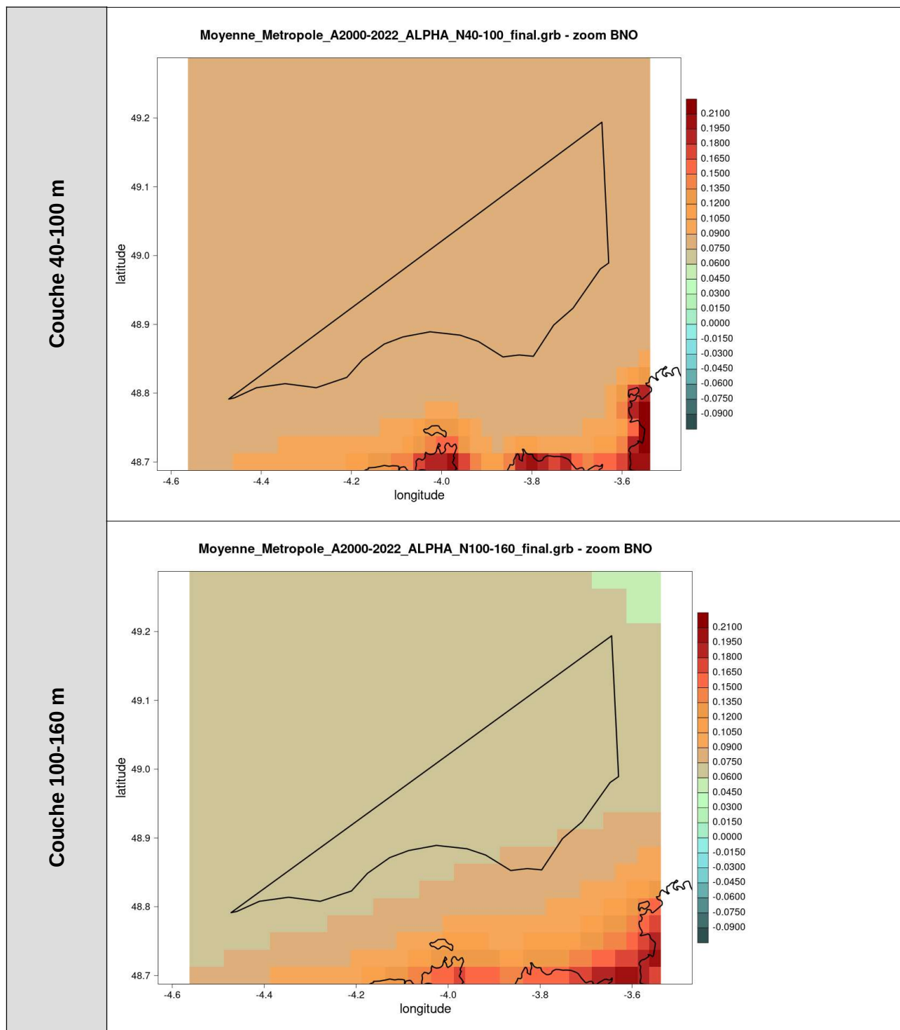
Illustration 12 : carte du coefficient \alpha de cisaillement de vent pour les couches 10-40, 10-160, 40-100 et 100-160 m tous secteurs confondus pour la zone BNO, calculé à partir des forces du vent AROME (2000-2022)
