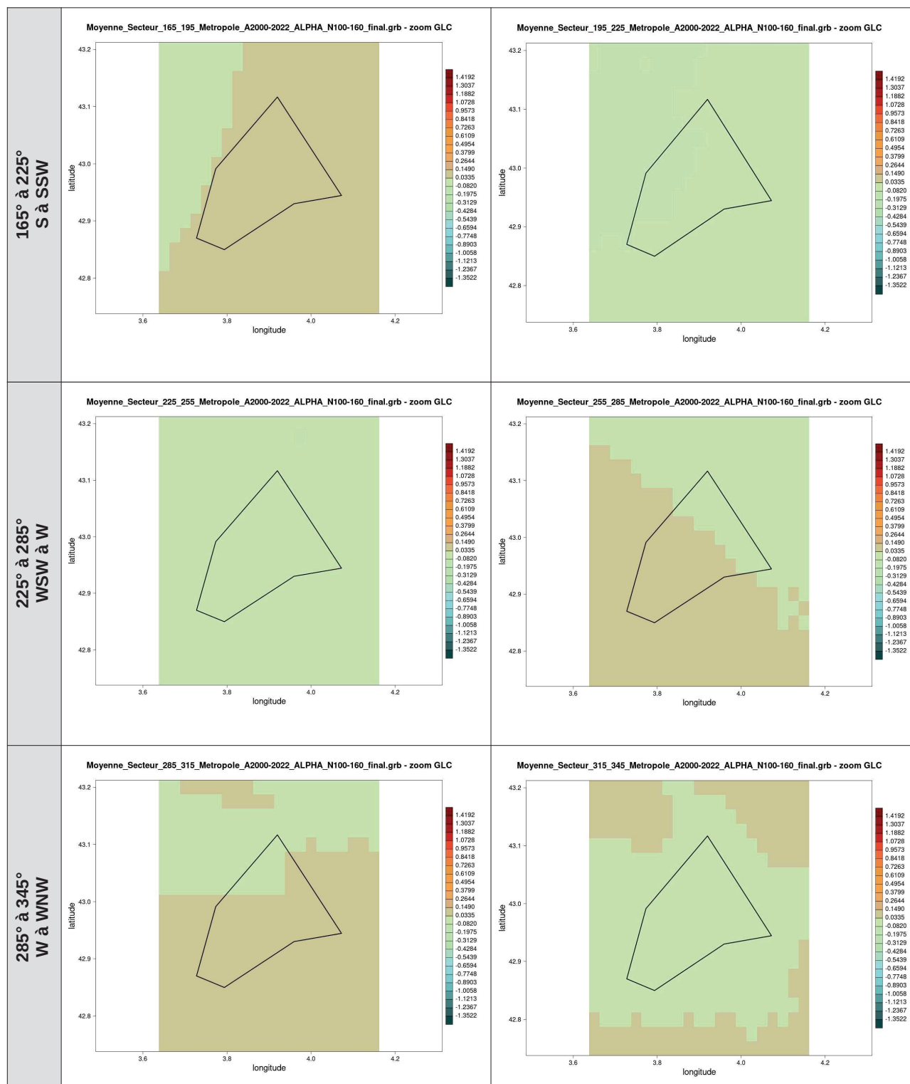
Illustration 37 : cartes du coefficient \alpha de cisaillement de vent pour la couche 100-160 m par secteur de direction de 30° pour la zone GLC calculé à partir du vent AROME (2000-2022)
