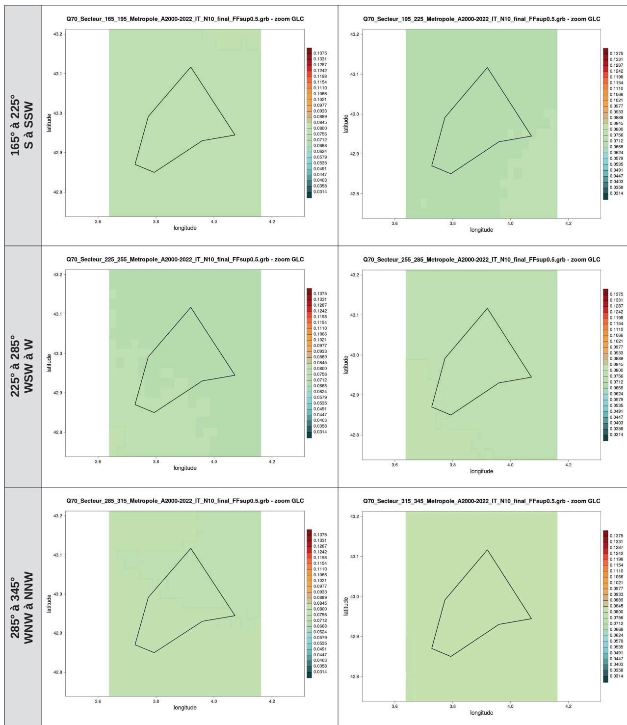
Illustration 17 : cartes des Q70 de l'intensité de turbulence au niveau 10 m par secteur de direction de 30° pour la zone GLC, calculés à partir des données AROME (2000-2022)
