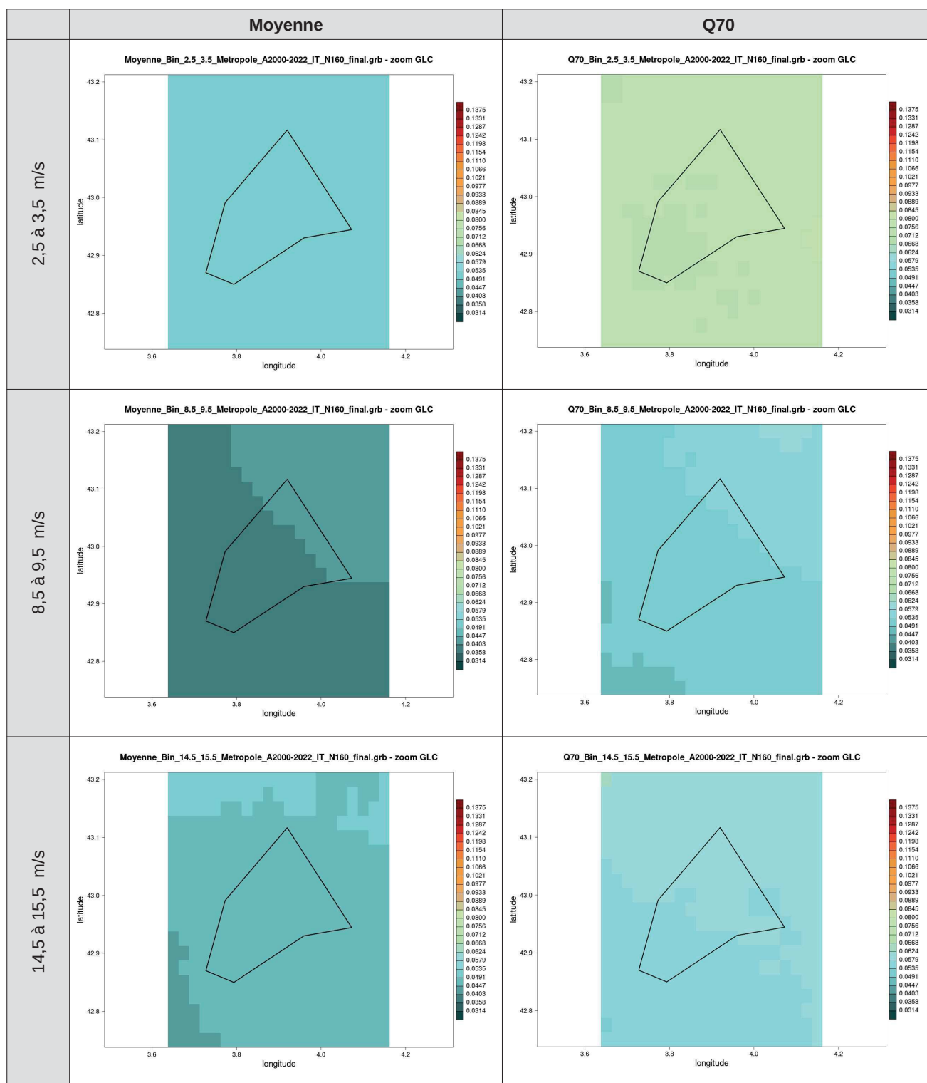
Illustration 22 : cartes des moyennes à gauche et du Q70 à droite de l'intensité de turbulence au niveau 160 m par bin de 1 m/s pour la zone GLC, calculées à partir des données AROME (2000-2022)
