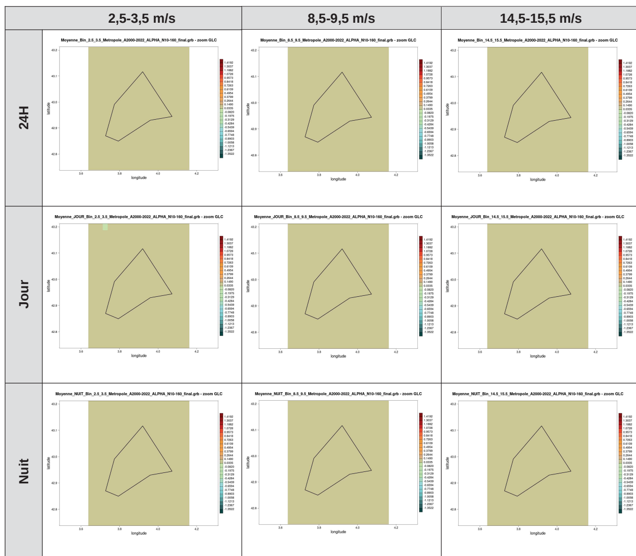
Illustration 13 : coefficient \alpha du cisaillement moyen du vent sur la couche 10-160 mètres pour les bins 2,5-3,5, 8,5-9,5 et 14,5-15,5 m/s avec et sans différenciation jour/nuit sur la zone GLC
