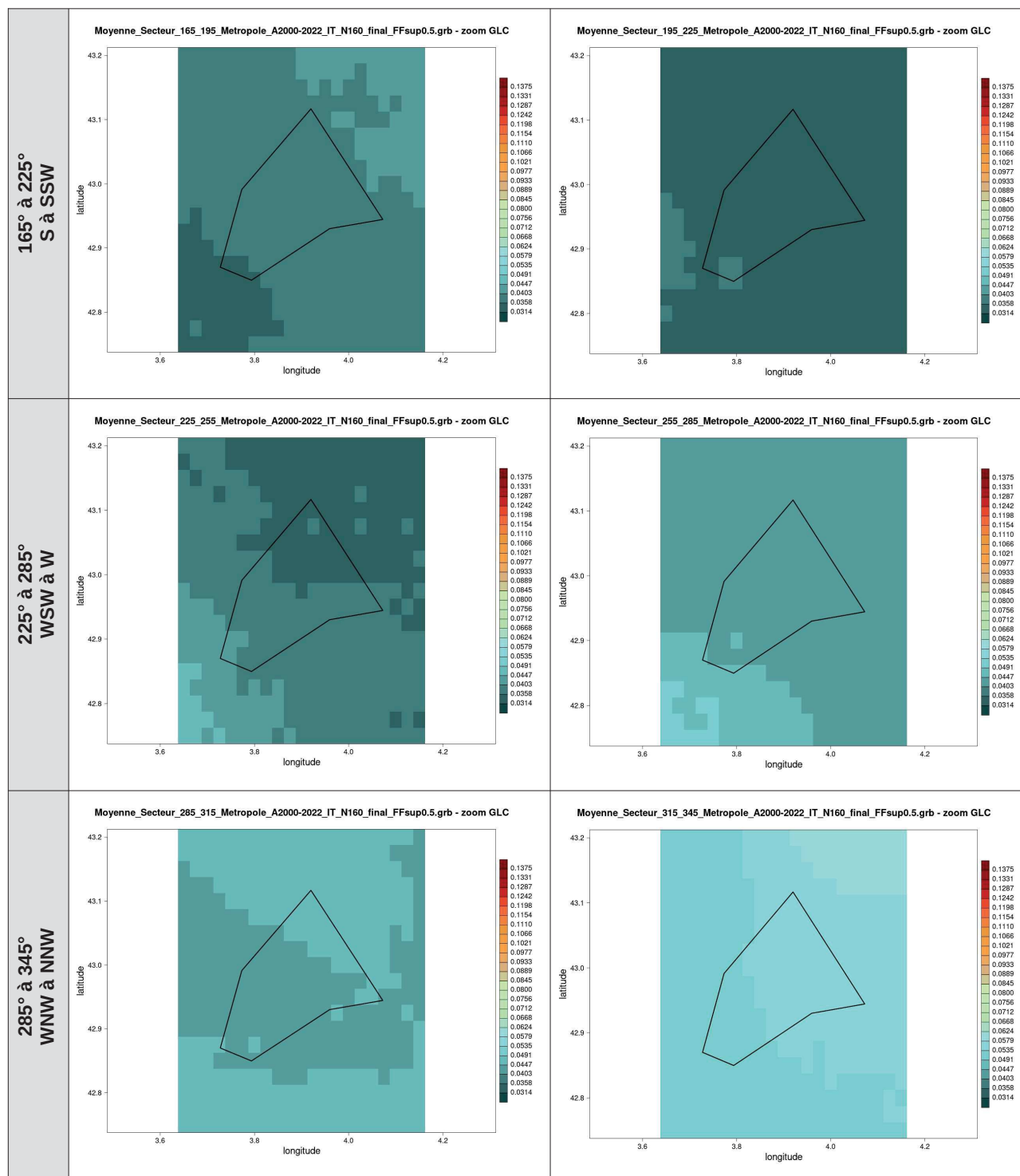
Illustration 16 : cartes des moyennes de l'intensité de turbulence au niveau 160 m par secteur de direction de 30° pour la zone GLC, calculées à partir des données AROME (2000-2022)
