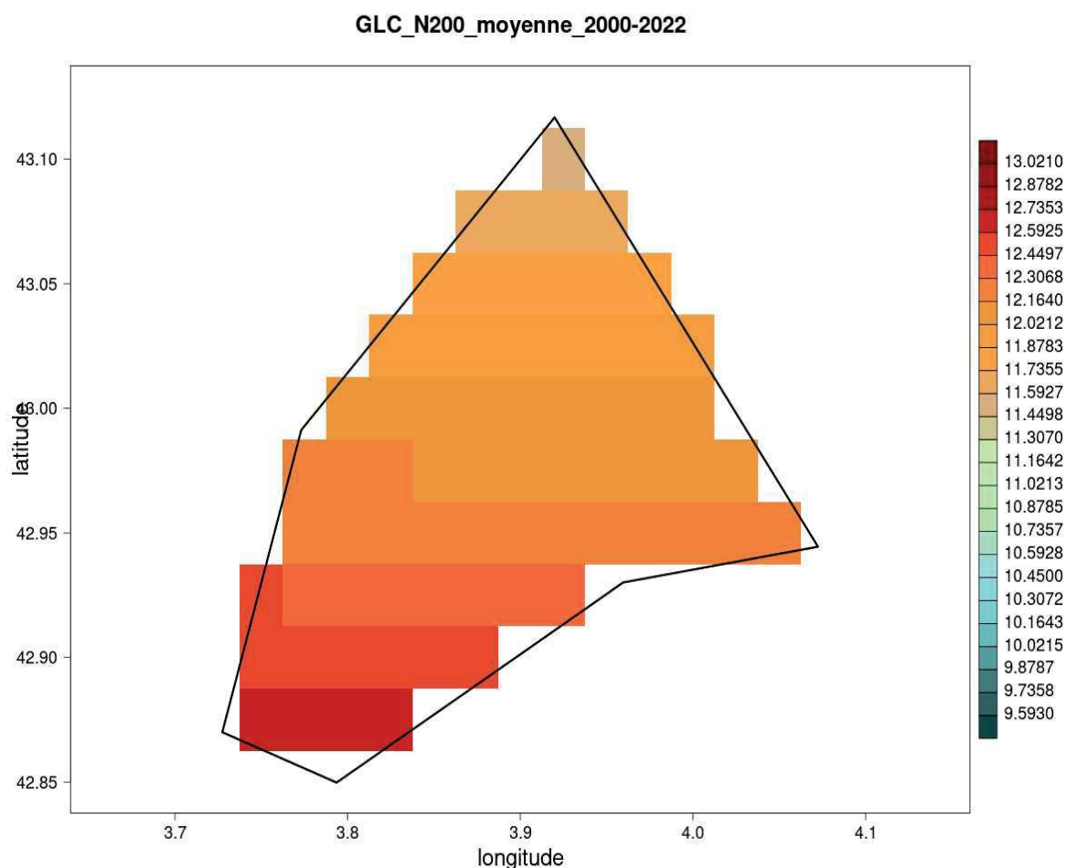
Illustration 29 : forces moyennes du vent de rafale sur la zone GLC au niveau 200 m sur la période 2000-2022
