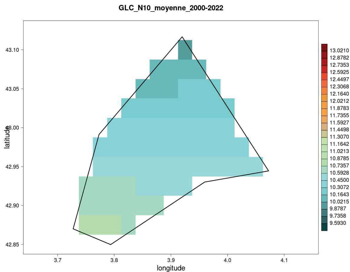
Illustration 23 : forces moyennes du vent de rafale sur la zone GLC au niveau 10 m sur la période 2000-2022
