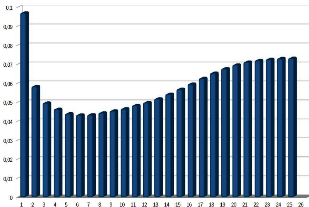
Illustration 6 : moyenne sur la zone GLC de la moyenne de l'intensité de turbulence, en fonction de la force du vent (m/s) en abscisse. Période 2000-2022 à 100 mètres
