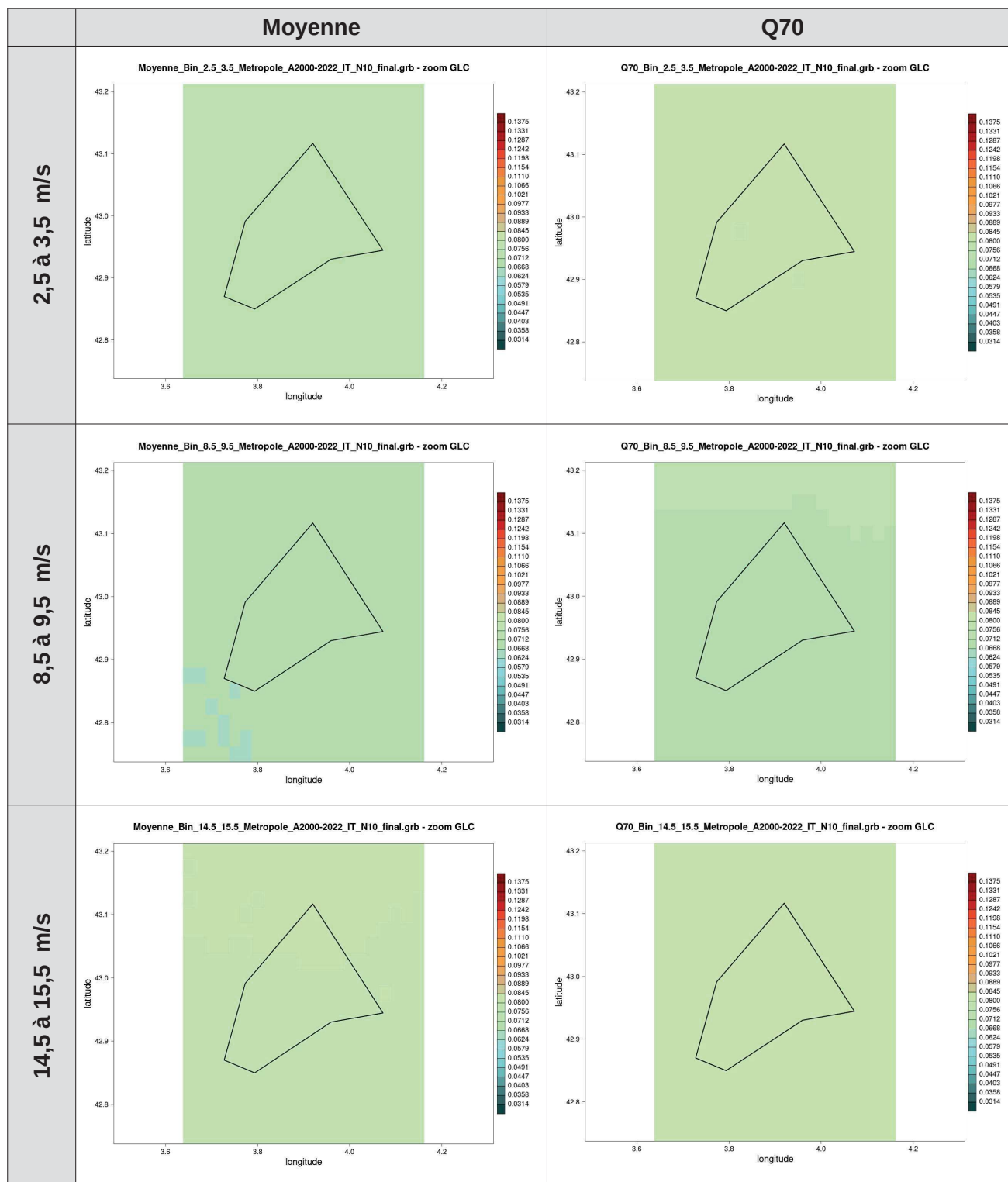
Illustration 20 : cartes des moyennes à gauche et du Q70 à droite de l'intensité de turbulence au niveau 10 m par bin de 1 m/s pour la zone GLC, calculées à partir des données AROME (2000-2022)
