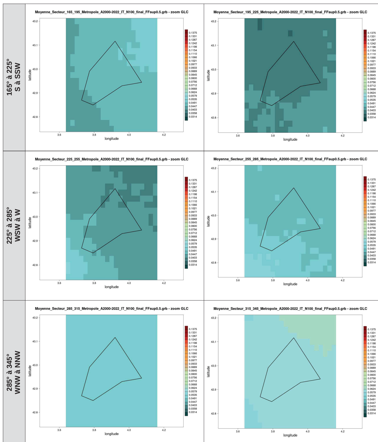
Illustration 3 : cartes des moyennes de l'intensité de turbulence au niveau 100 m par secteur de direction de 30° pour la zone GLC, calculées à partir des données AROME (2000-2022)
