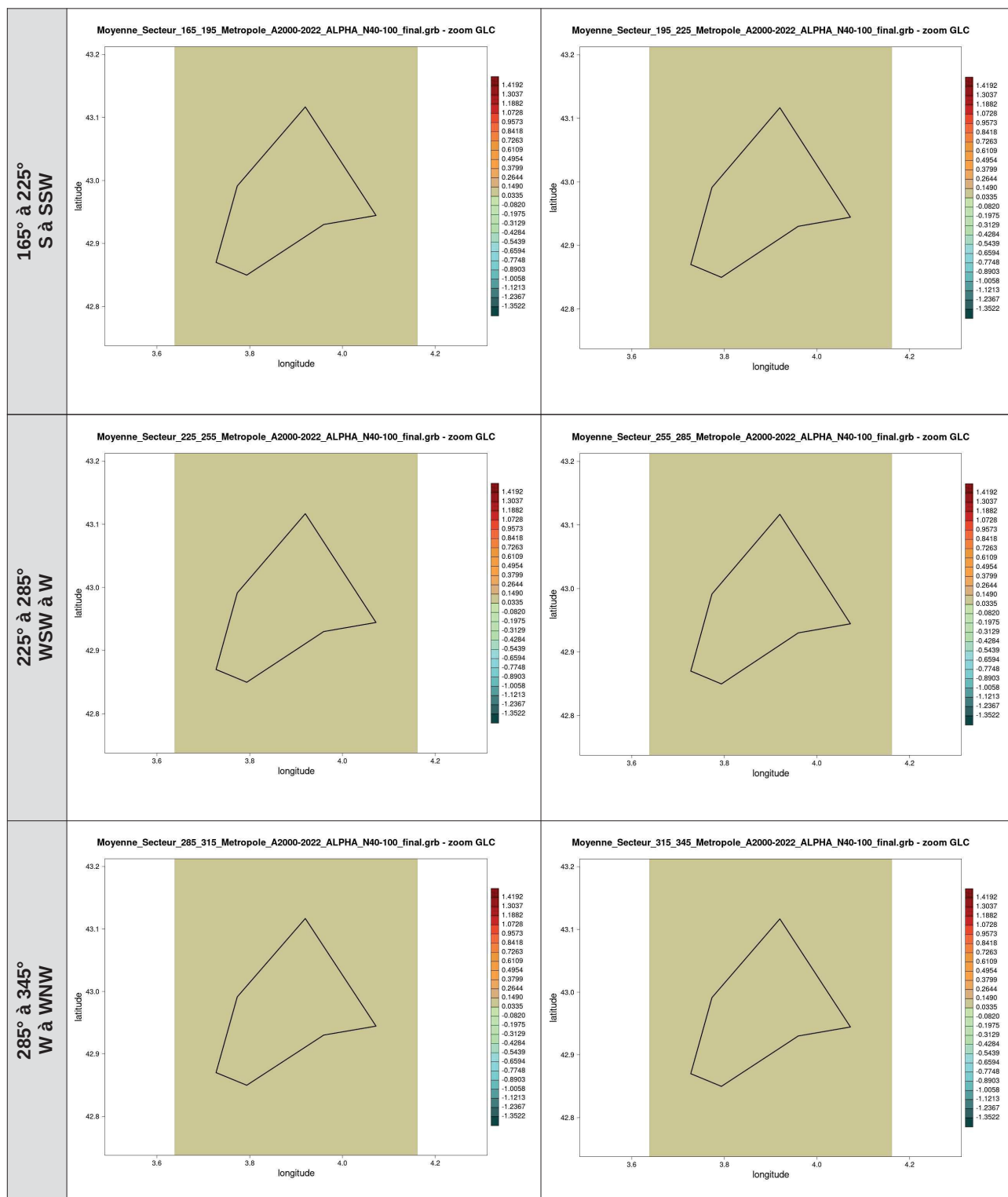
Illustration 36 : cartes du coefficient \alpha de cisaillement de vent pour la couche 40-100 m par secteur de direction de 30° pour la zone GLC calculé à partir du vent AROME (2000-2022)
