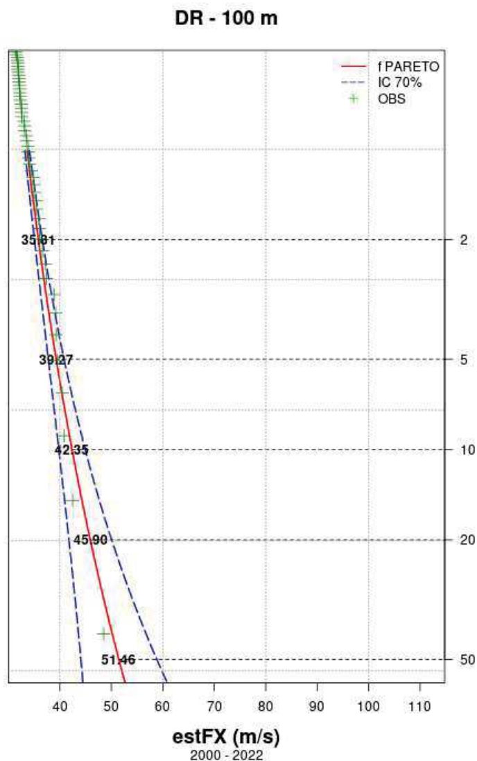
Illustration 10 : courbe des quantiles pour le point 51, positionné à 43,025 Nord et 43,95 Est, situé à l'intérieur du domaine de la zone GLC (à 100 m)
