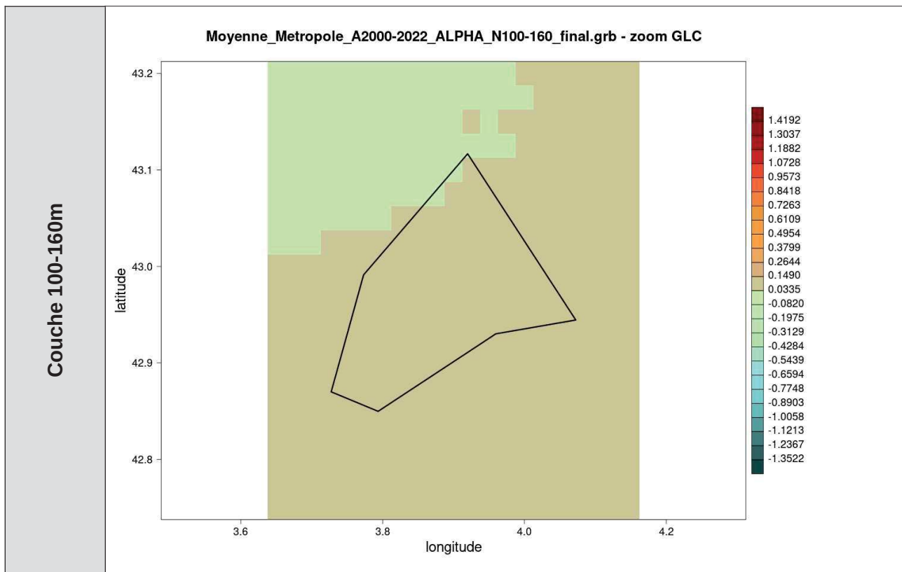
Illustration 11 : cartes du coefficient \alpha de cisaillement de vent pour les couches 10-40, 10-160, 40-100 et 100-160 m tous secteurs confondus pour la zone GLC, calculé à partir des forces du vent AROME (2000-2022)
