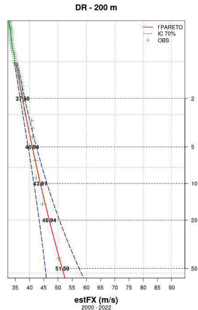
Illustration 34 : courbe des quantiles pour le point 51, positionné à 43,025 Nord et 3,95 Est, situé à l'intérieur du domaine de la zone GLC (à 200 m)
