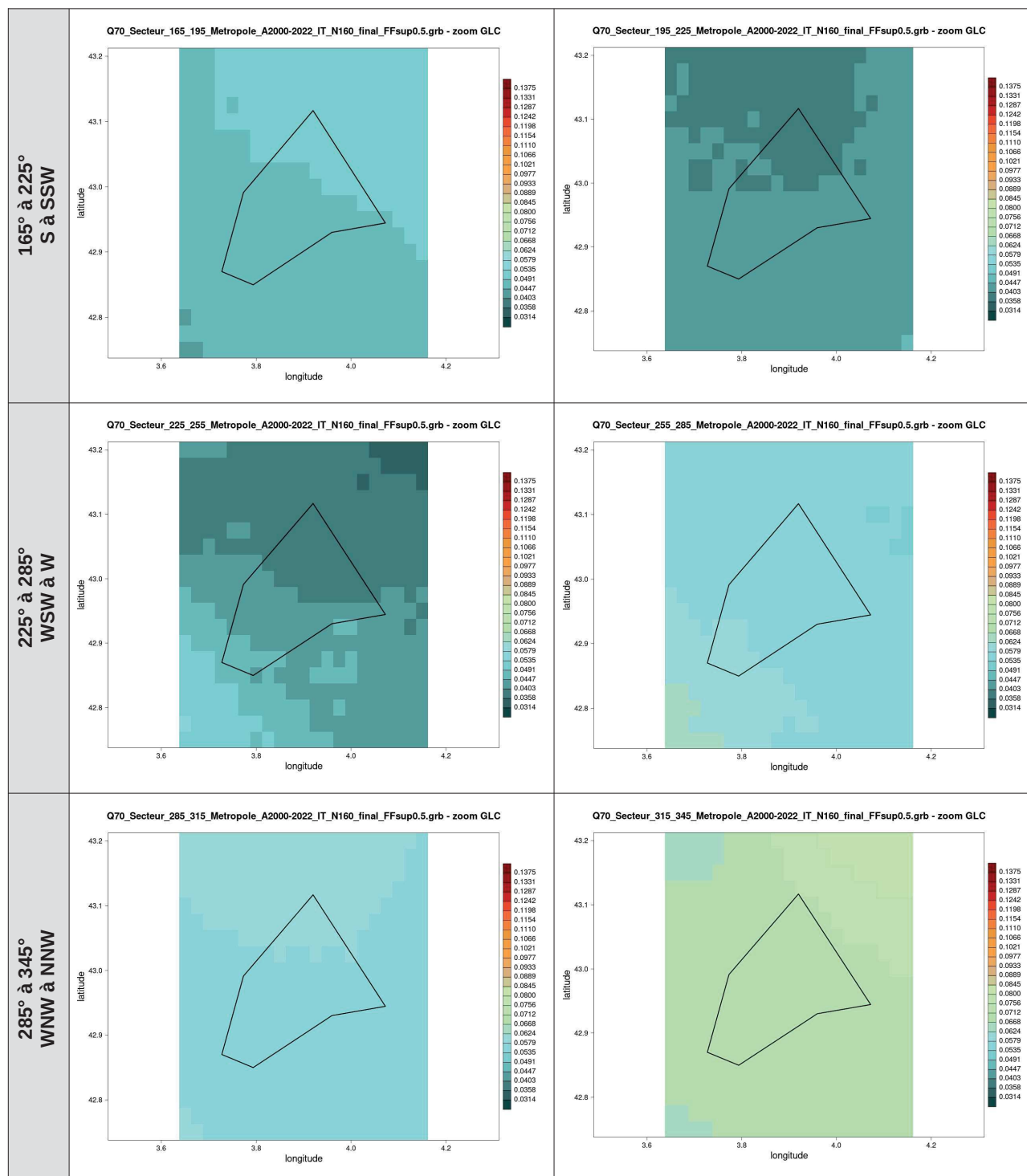
Illustration 19 : cartes des Q70 de l'intensité de turbulence au niveau 160 m par secteur de direction de 30° pour la zone GLC, calculés à partir des données AROME (2000-2022)
