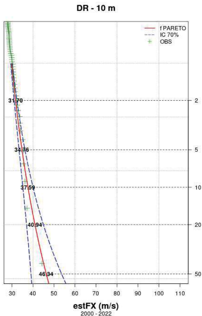
Illustration 31 : courbe des quantiles pour le point 51, positionné à 43,025 Nord et 3,95 Est, situé à l'intérieur du domaine de la zone GLC (à 10 m)
