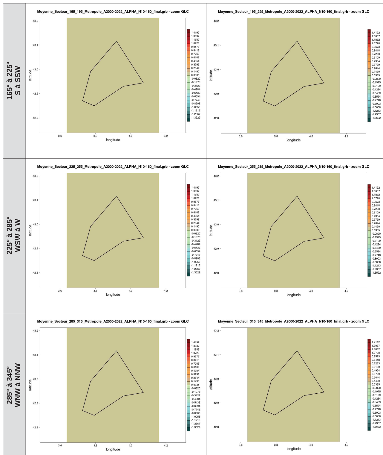
Illustration 12 : cartes du coefficient \alpha de cisaillement de vent pour la couche 10-160 m par secteur de direction de 30° pour la zone GLC, calculé à partir du vent AROME (2000-2022)
