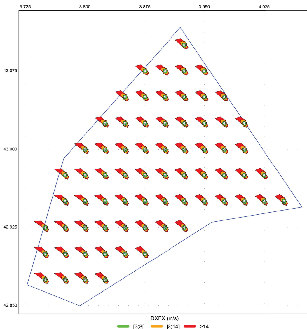
Illustration 28 : roses des vents de rafales estimées à 160 m sur la période 2000-2022
