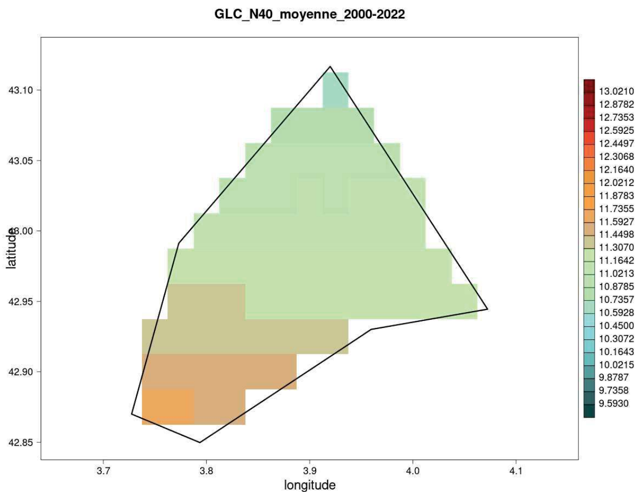
Illustration 25 : forces moyennes du vent de rafale sur la zone GLC au niveau 40 m sur la période 2000-2022
