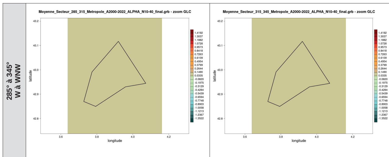
Illustration 35 : cartes du coefficient \alpha de cisaillement de vent pour la couche 10-40 m par secteur de direction de 30° pour la zone GLC, calculé à partir du vent AROME (2000-2022)
