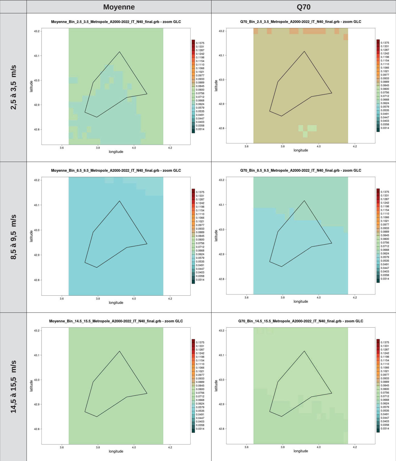
Illustration 21 : cartes des moyennes à gauche et du Q70 à droite de l'intensité de turbulence au niveau 40 m par bin de 1 m/s pour la zone GLC, calculées à partir des données AROME (2000-2022)
