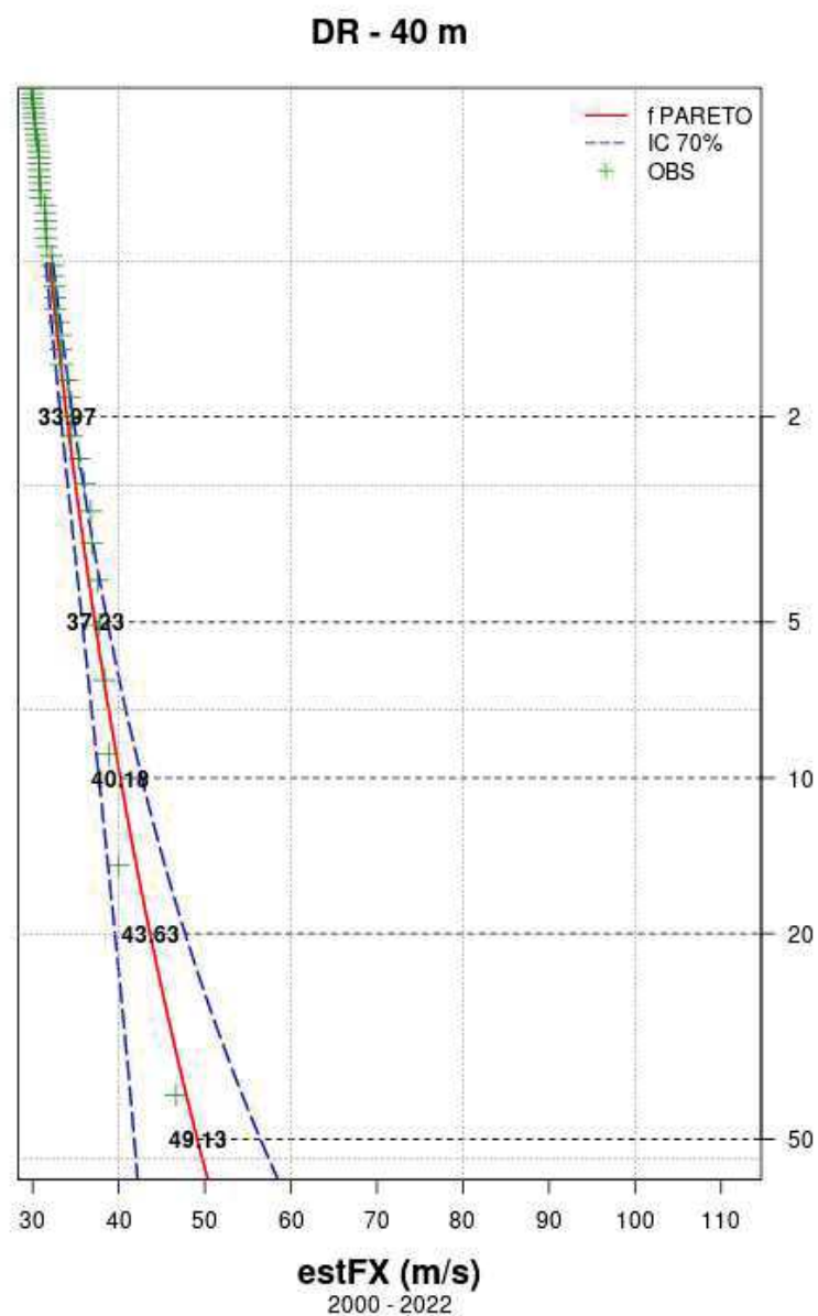
Illustration 32 : courbe des quantiles pour le point 51, positionné à 43,025 Nord et 3,95 Est, situé à l'intérieur du domaine de la zone GLC (à 40 m)
