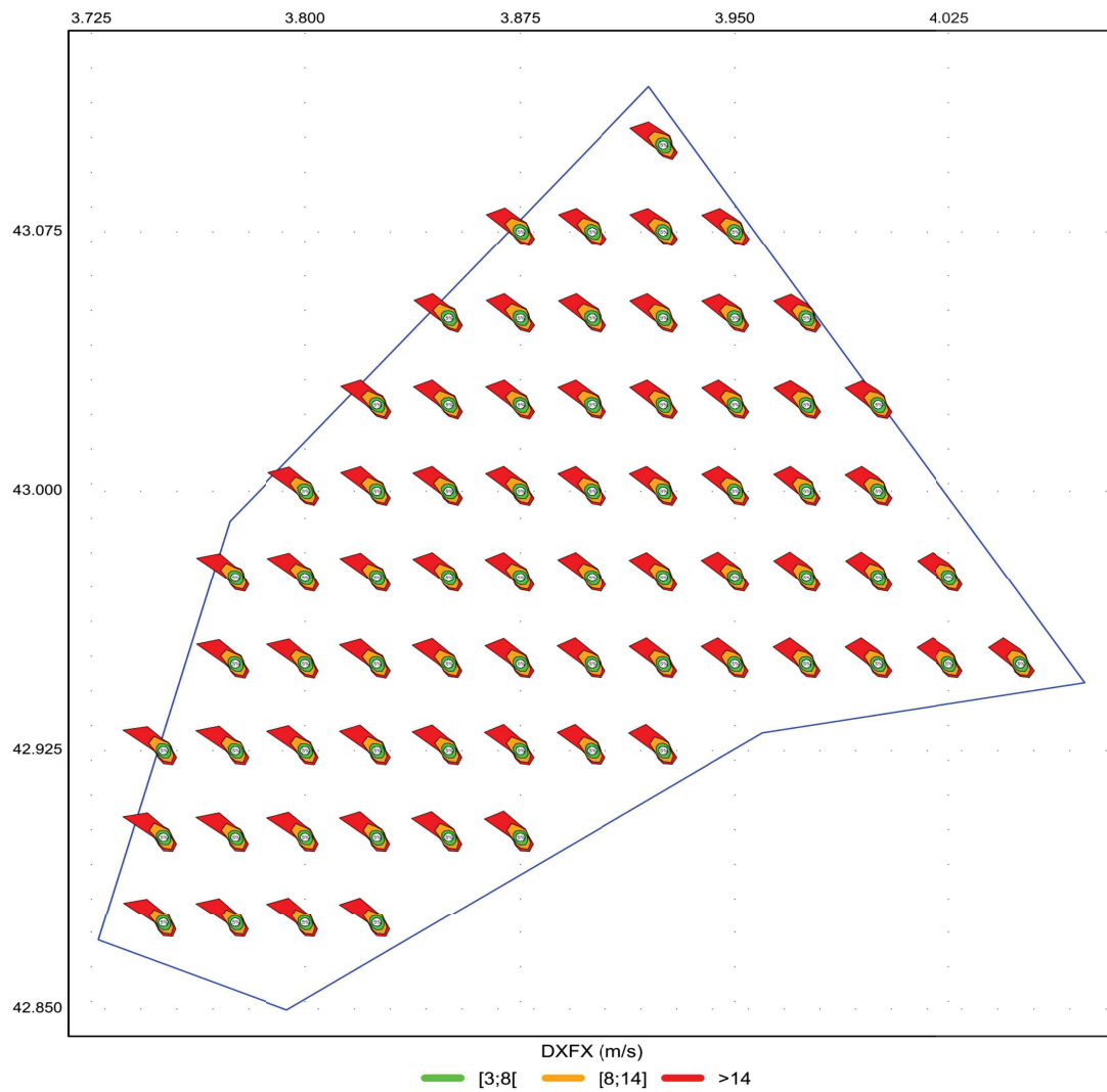
Illustration 30 : roses des vents de rafales estimées à 200 m sur la période 2000-2022
