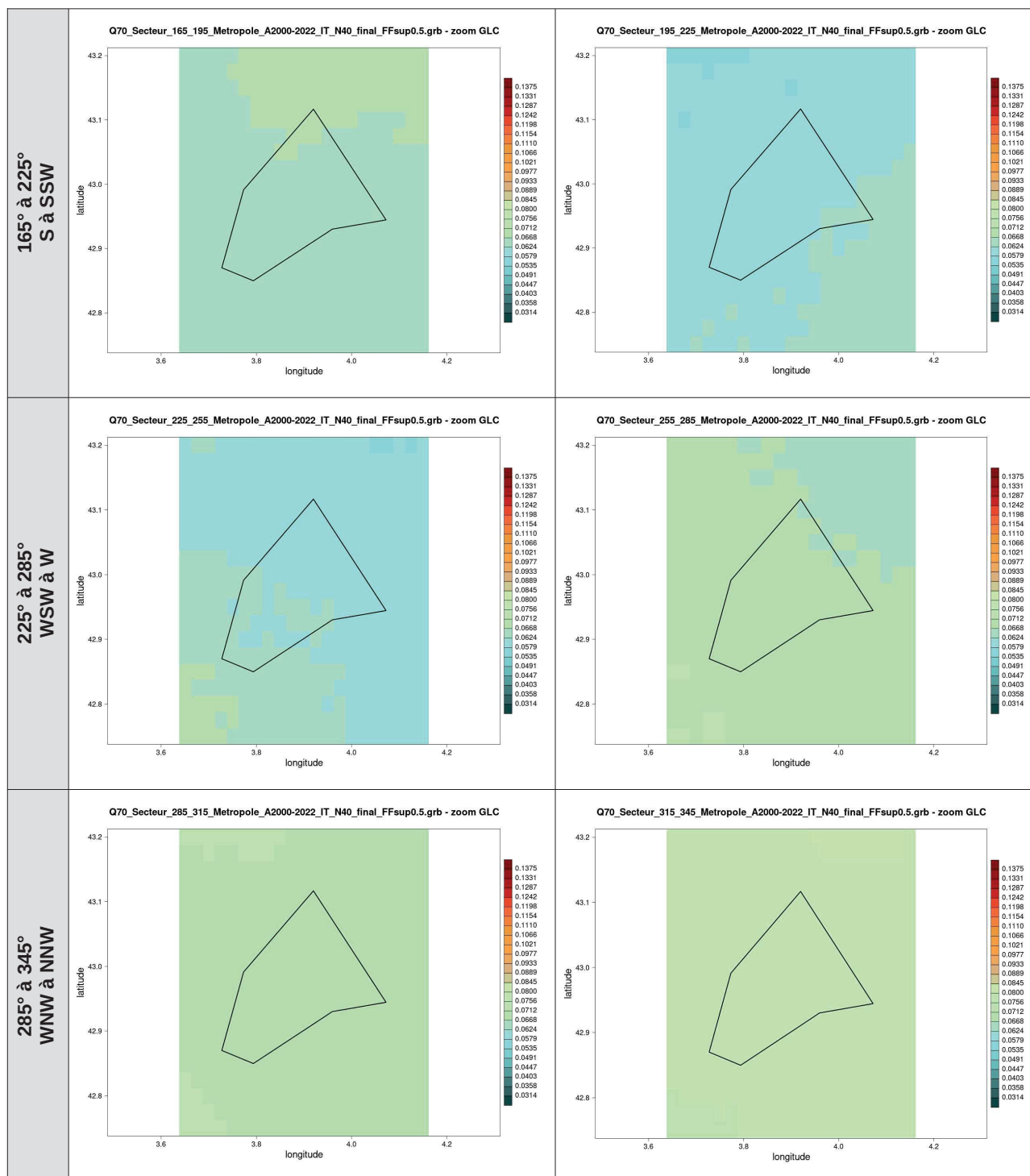
Illustration 18 : cartes des Q70 de l'intensité de turbulence au niveau 40 m par secteur de direction de 30° pour la zone GLC, calculés à partir des données AROME (2000-2022)
