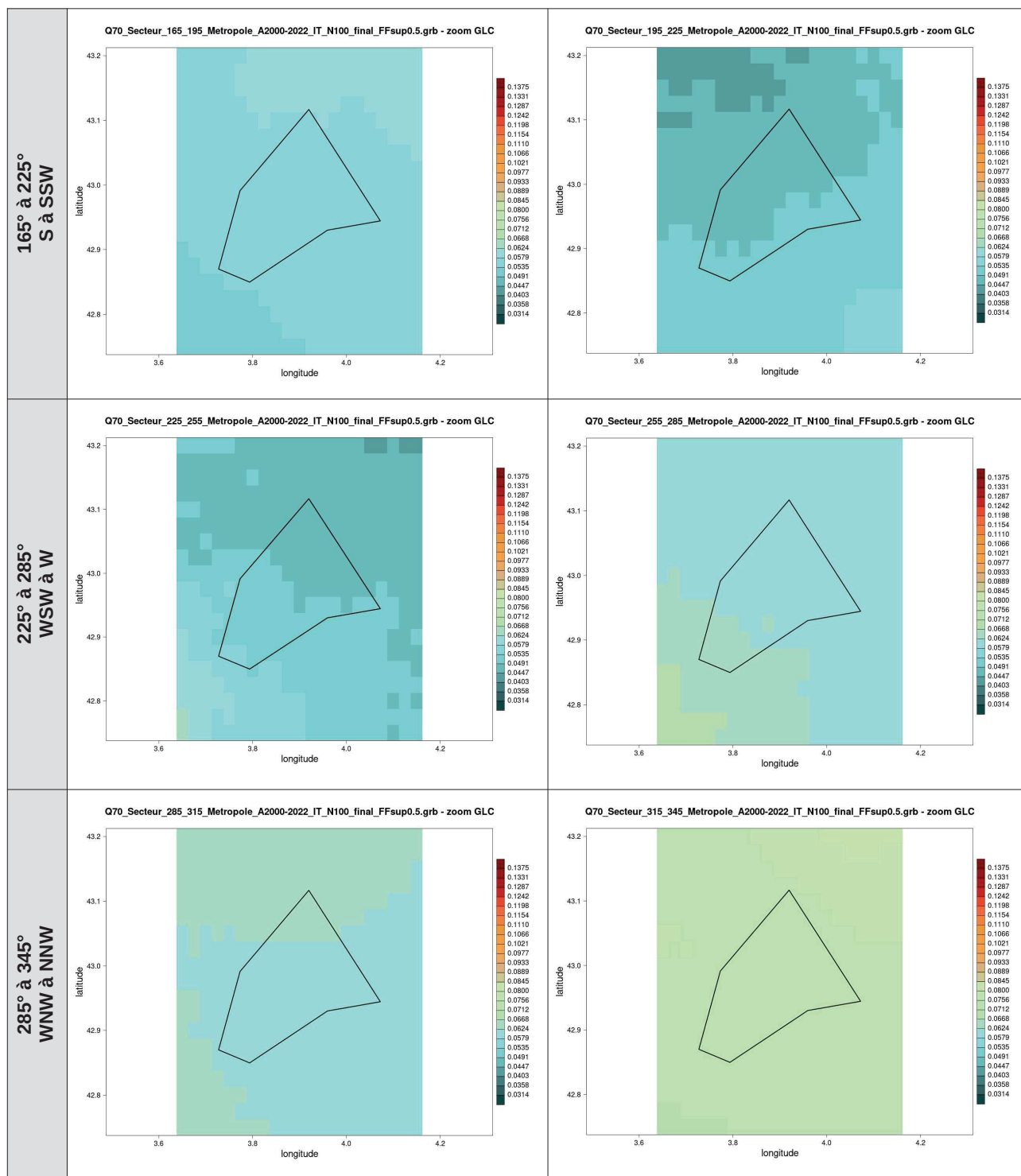
Illustration 4 : cartes des Q70 de l'intensité de turbulence au niveau 100 m par secteur de direction de 30° pour la zone GLC, calculés à partir des données AROME (2000-2022)
