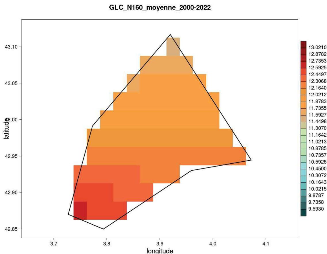
Illustration 27 : forces moyennes du vent de rafale sur la zone GLC au niveau 160 m sur la période 2000-2022
