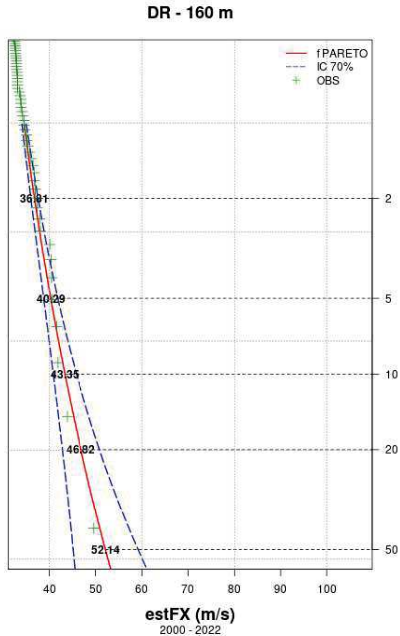
Illustration 33 : courbe des quantiles pour le point 51, positionné à 43,025 Nord et 3,95 Est, situé à l'intérieur du domaine de la zone GLC (à 160 m)
