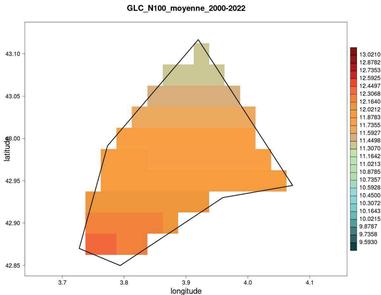
Illustration 8 : forces moyennes du vent de rafale sur la zone GLC au niveau 100 m sur la période 2000-2022
