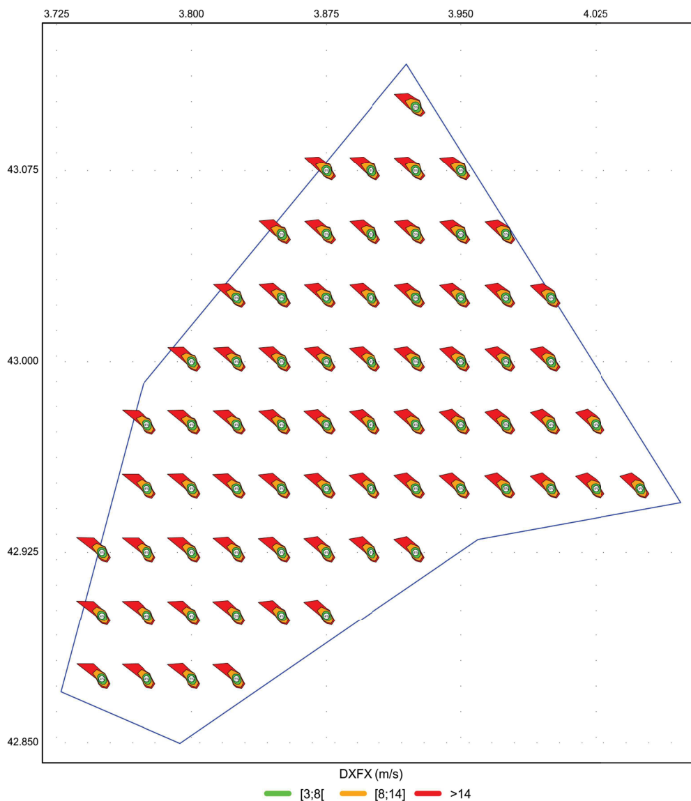
Illustration 9 : roses des vents de rafales estimées à 100 m sur la période 2000-2022
