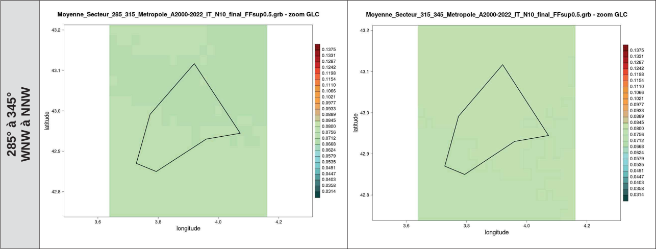
Illustration 14 : cartes des moyennes de l'intensité de turbulence au niveau 10 m par secteur de direction de 30° pour la zone GLC, calculées à partir des données AROME (2000-2022)
