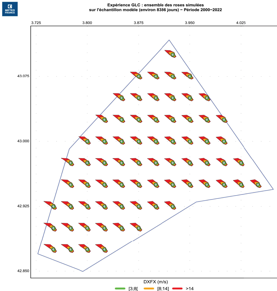
Illustration 26 : roses des vents de rafales estimées à 40 m sur la zone GLC sur la période 2000-2022
