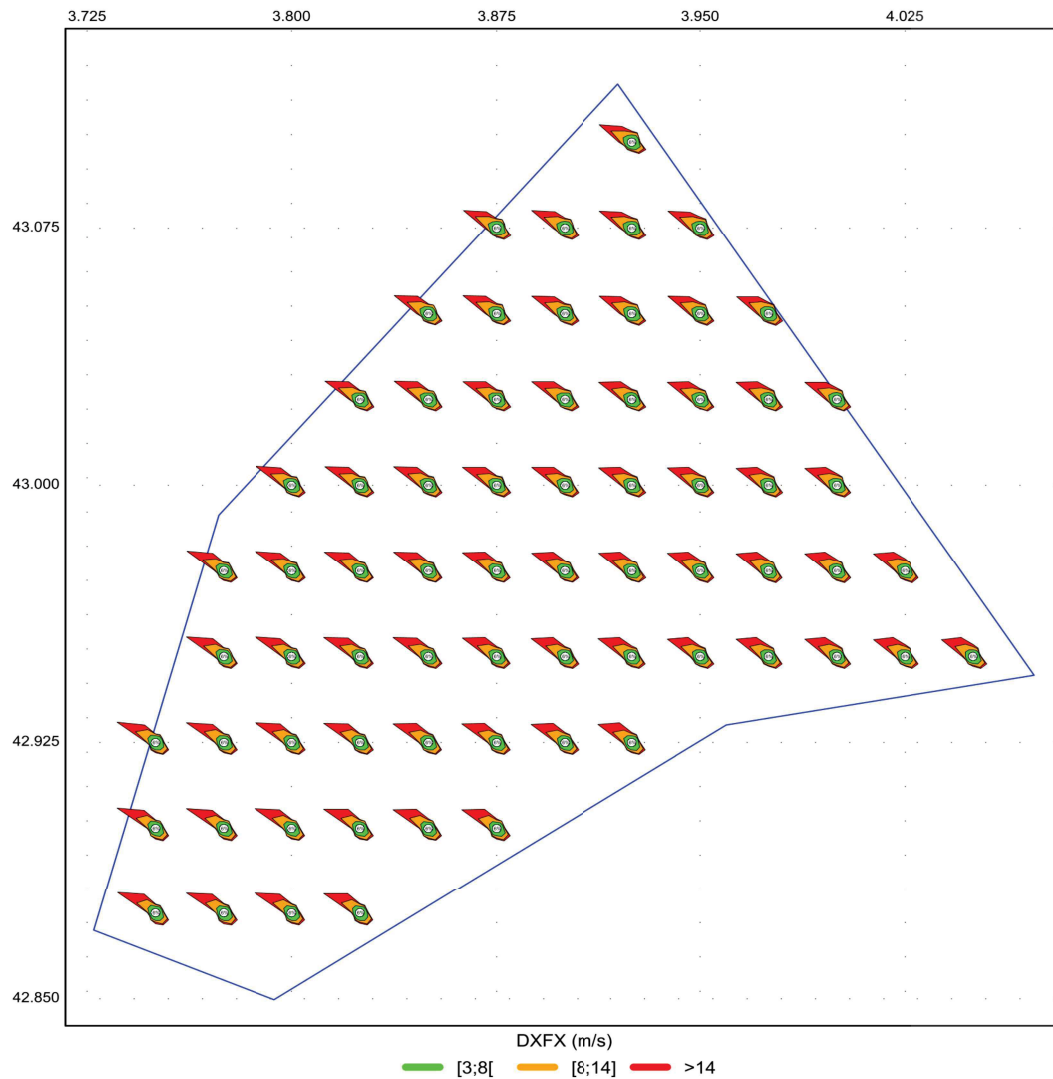
Illustration 24 : roses des vents de rafales estimées à 10 m sur la zone GLC sur la période 2000-2022
