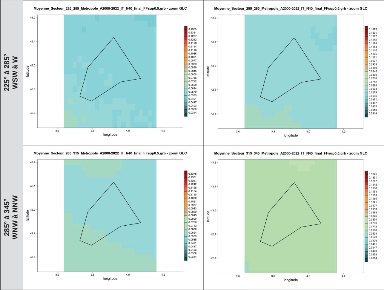
Illustration 15 : cartes des moyennes de l'intensité de turbulence au niveau 40 m par secteur de direction de 30° pour la zone GLC, calculées à partir des données AROME (2000-2022)
