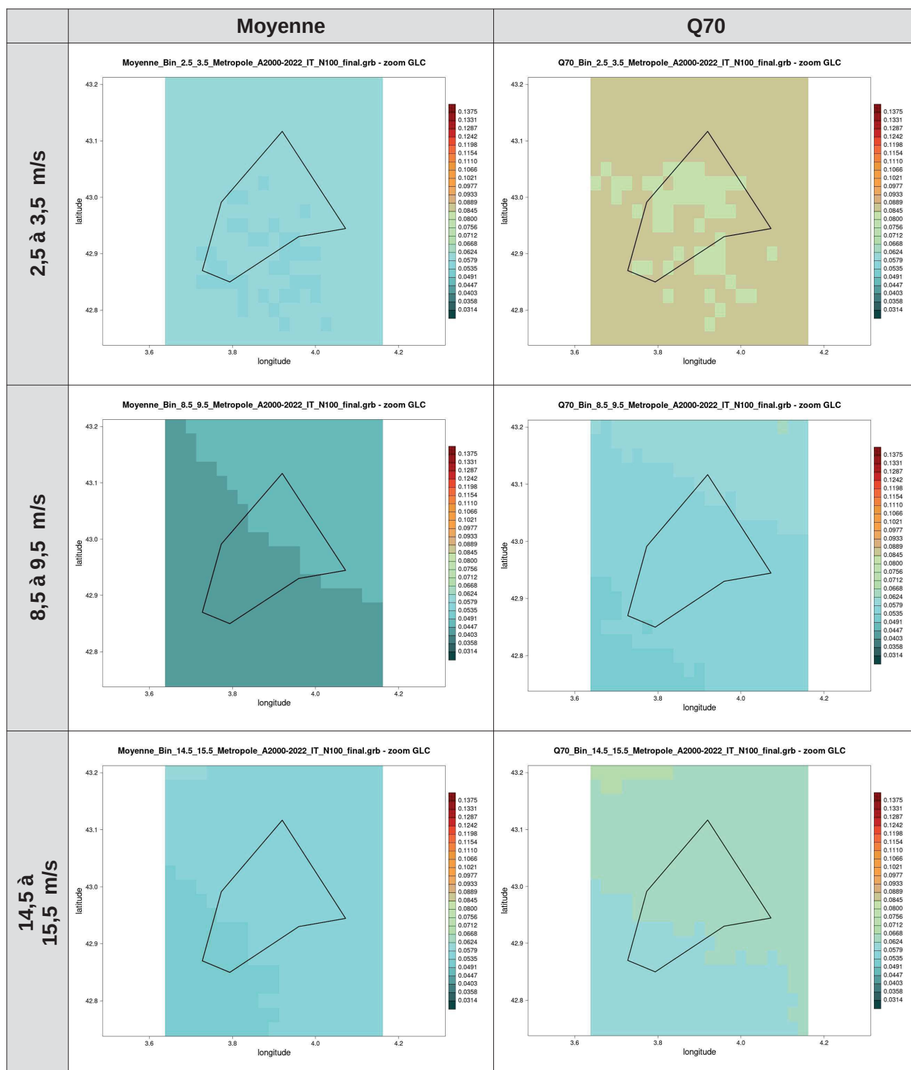
Illustration 5 : cartes des moyennes à gauche et du Q70 à droite de l'intensité de turbulence au niveau 100 m pour 3 bins de 1 m/s pour la zone GLC, calculés à partir des données AROME (2000-2022)
