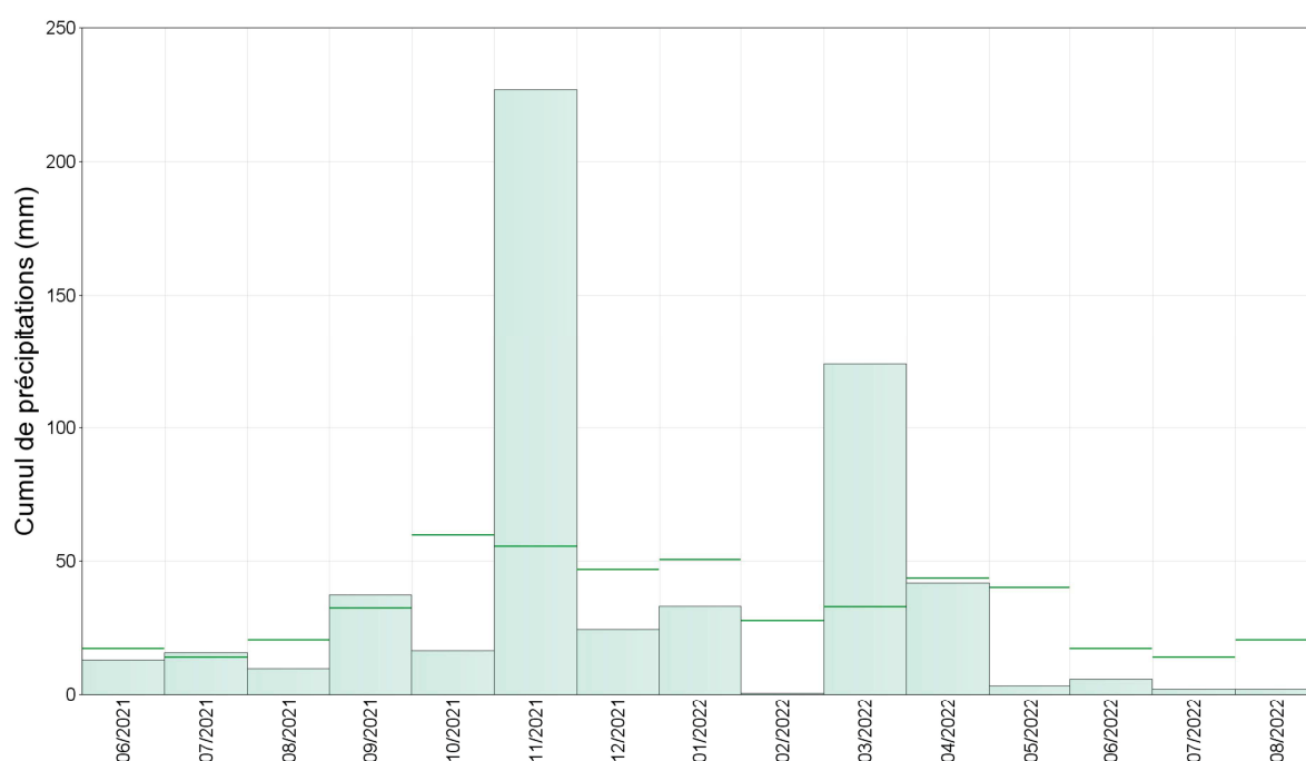
Illustration 37 : Cumuls mensuels de précipitations de juin 2021 à août 2022 à la station de Leucate (11) (histogrammes en bleu) et normale de précipitations (segments en vert) - Période de référence : 1991 - 2020
