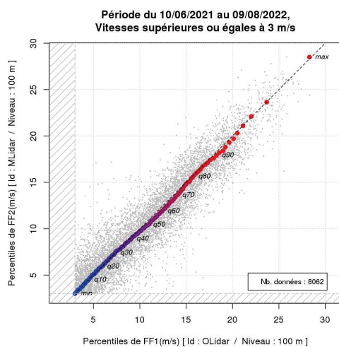
Illustration 12 : Diagramme « quantile-quantile »
