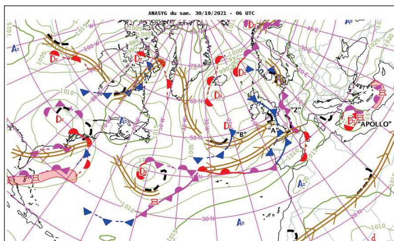
Illustration 27 : Anasyg du samedi 30 octobre à 06 UTC
