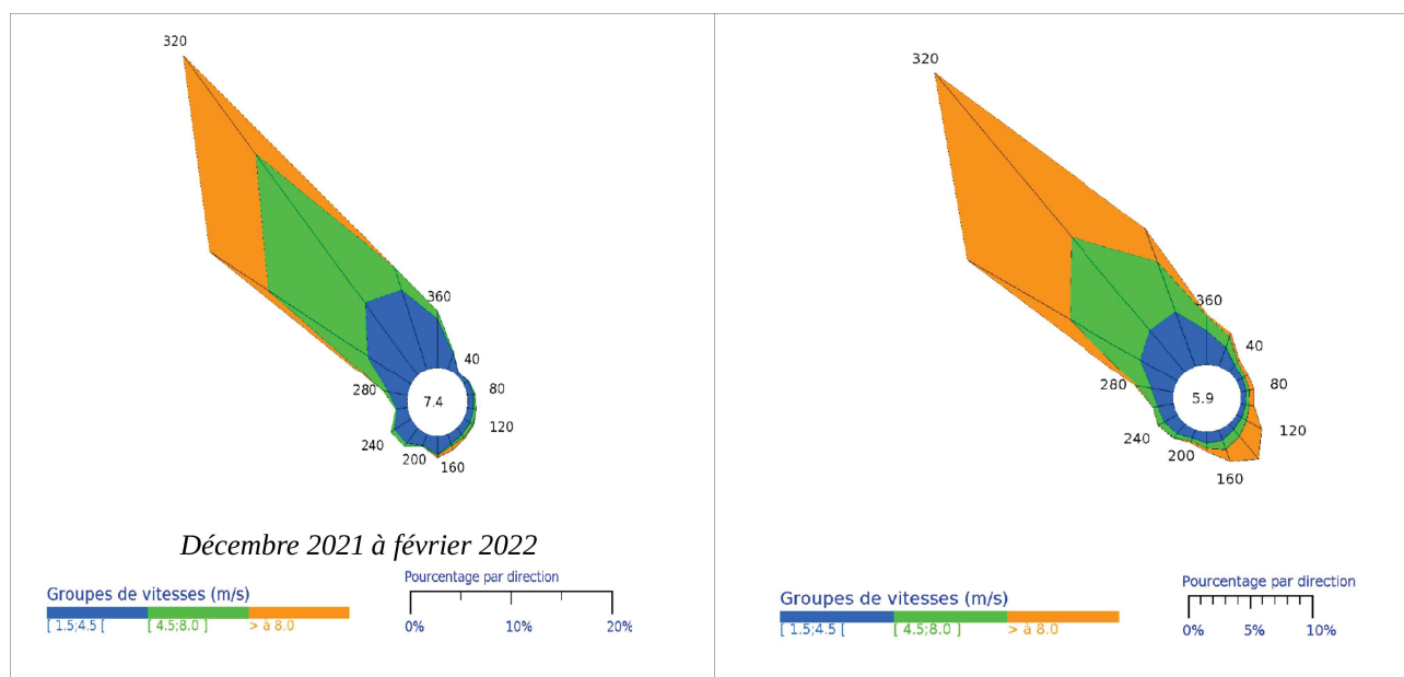
Illustration 33 : Roses des vents de l'hiver 2021-2022 et en moyenne sur la période 2001-2020 pour la station de Leucate
