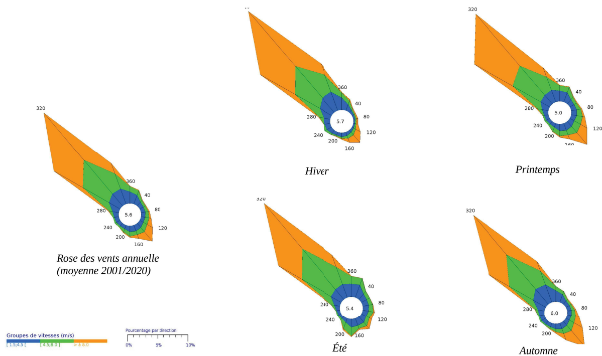
Illustration 2 : Roses des vents annuelle et saisonnières de la station de Leucate (numéro INSEE : 11202001) sur la période 2001/2020
