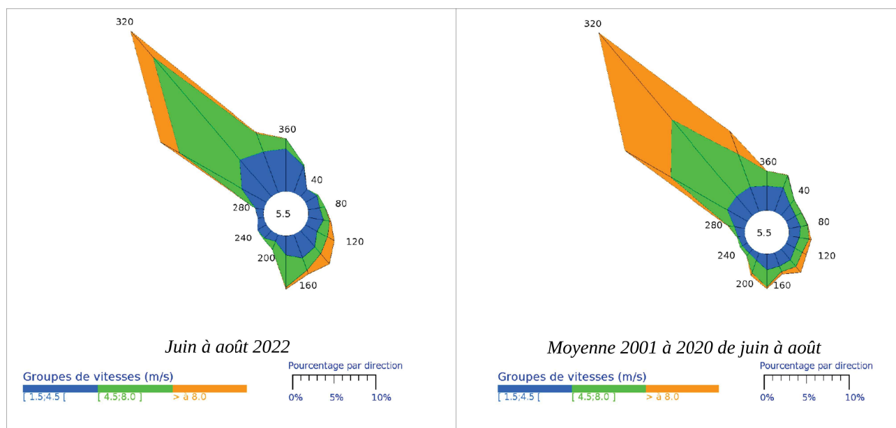
Illustration 35 : Roses des vents en été 2022 et en moyenne sur la période 2001-2020 pour la station de Leucate
