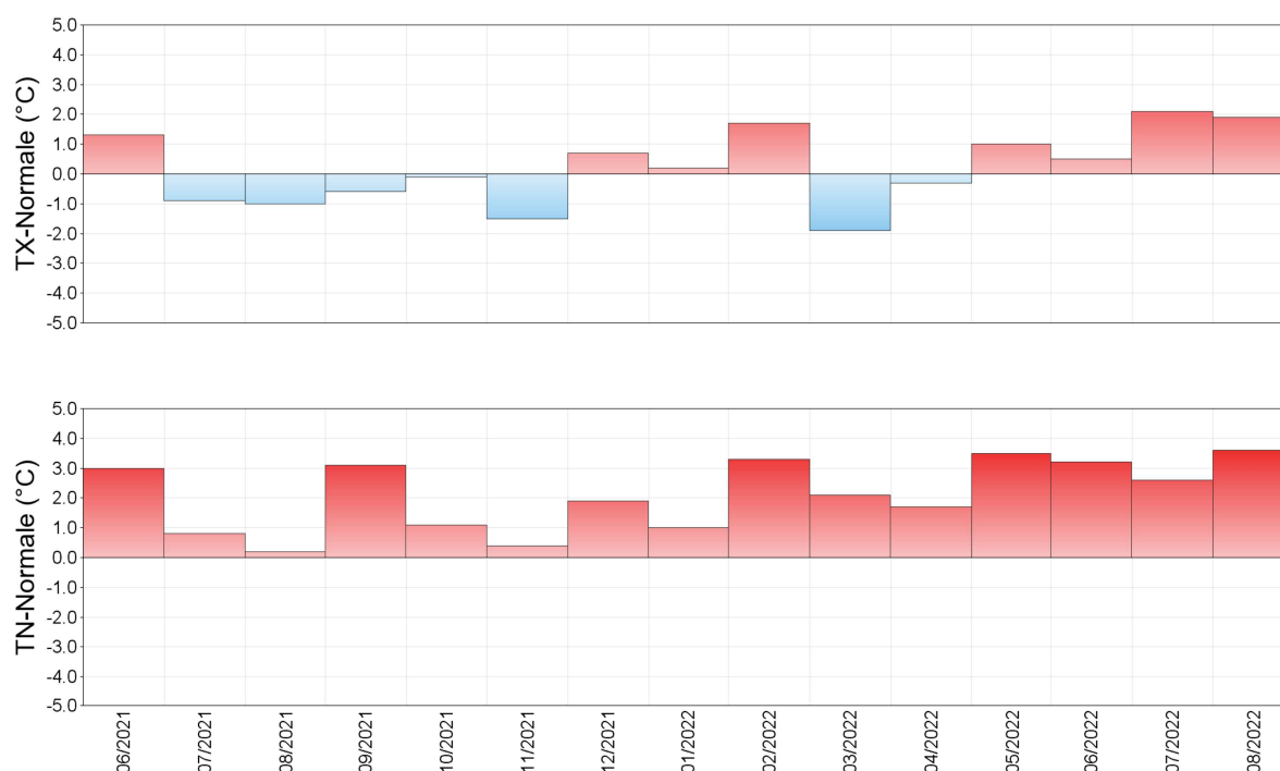
Illustration 36 : Anomalies mensuelles de températures minimales et maximales de juin 2021 à août 2022 à la station de Leucate (11) - Période de référence : 1991 - 2020
