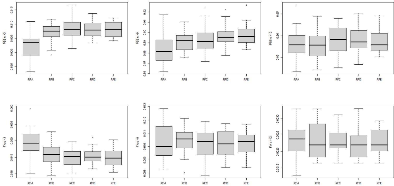
Illustration 8.16: Station de test 1 – FF – Modèles de forêt aléatoire à 20, 50, 100, 200 et 500 arbres - Box-plot PSS (première ligne pss > 3 m/s, pss > 9 m/s et pss > 12 m/s) et FA (deuxième ligne fa > 3 m/s, fa > 9 m/s et fa > 12 m/s) pour l'échantillon d'apprentissage
