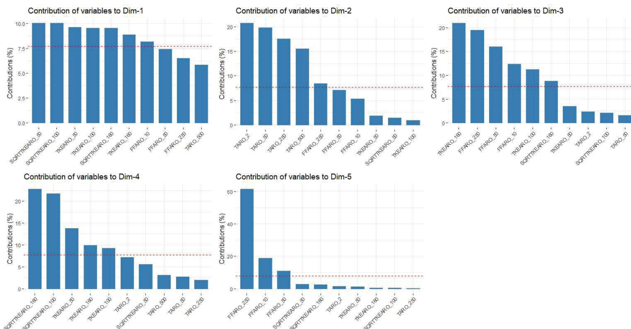
Illustration 3.15: AO6 Méditerranée zone 1 – FF – Contribution des variables à l'ACP (une figure pour chaque dimension)
