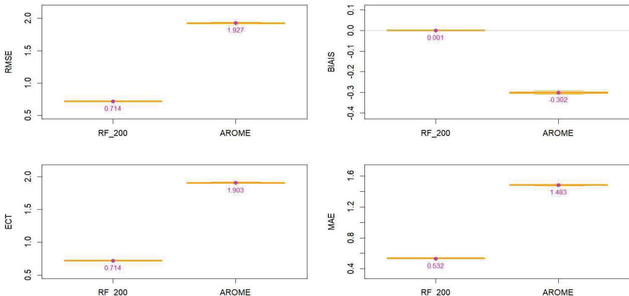
Illustration 3.17: AO6 Méditerranée zone 1 – U – Modèle de forêt aléatoire à 200 arbres - Box-plot RMSE (haut gauche), ECT (bas gauche), BIAIS (haut droite) et MAE (bas droite) pour l'échantillon d'apprentissage. La valeur en magenta sur chaque boîte à moustaches correspond à la moyenne des 20 échantillons.
