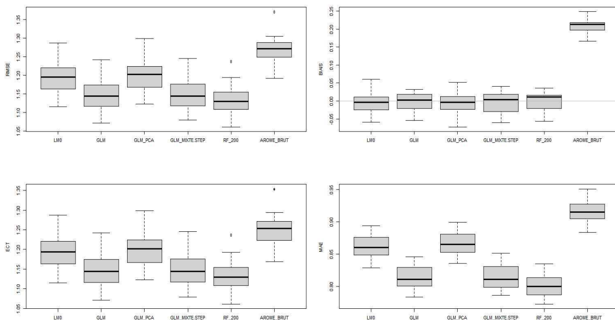
Illustration 8.45: Station de test 1 – U – Modèles linéaires, forêt et AROME - Box-plot RMSE, ECT, BIAIS et MAE pour l'échantillon de test
