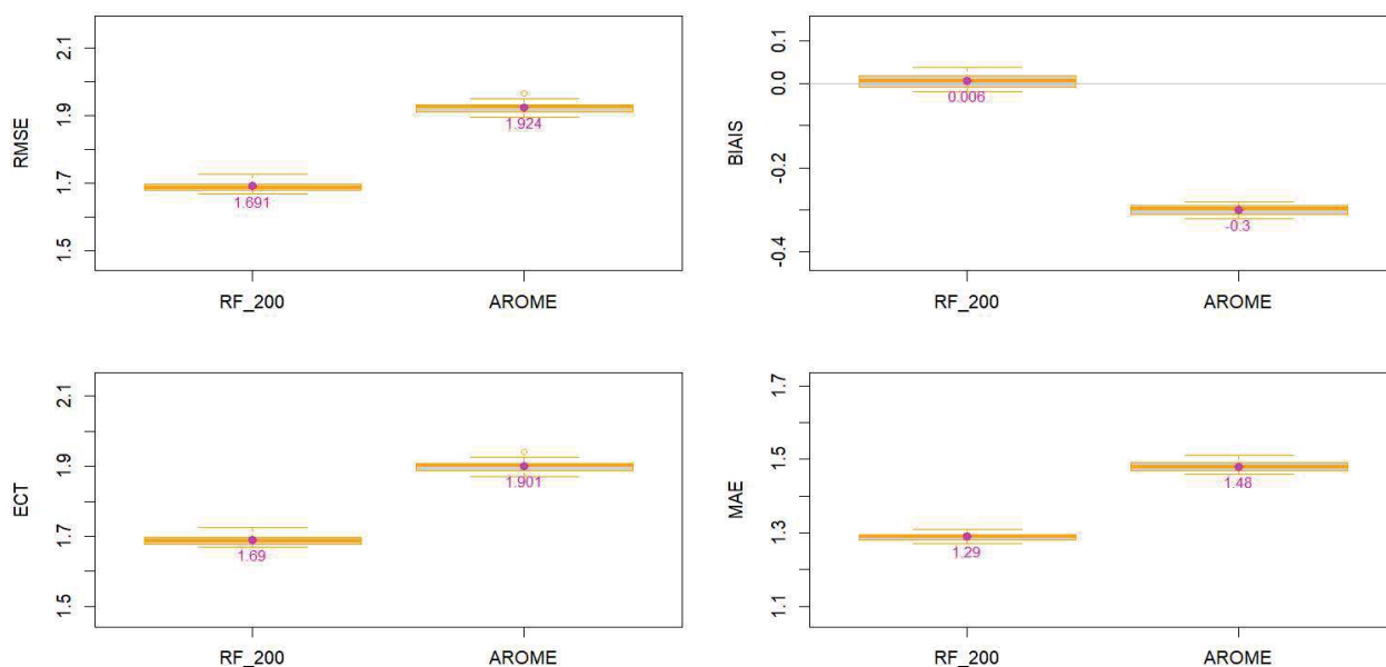
Illustration 3.19: AO6 Méditerranée zone 1 – U – Modèle de forêt aléatoire à 200 arbres - Box-plot RMSE, ECT, BIAIS et MAE pour l'échantillon de test. La valeur en magenta sur chaque boîte à moustaches correspond à la moyenne des 20 échantillons.
