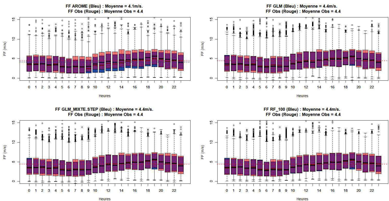
Illustration 8.34: Station de test 1 – FF – Cycle diurne des modèles statistiques (bleu) superposé aux observations (rouge)
