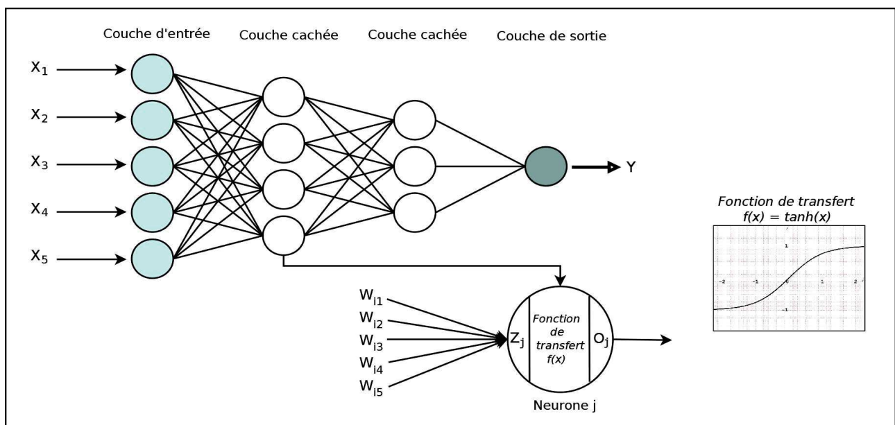
Illustration 7.1: Réseau de neurones multi-couches
