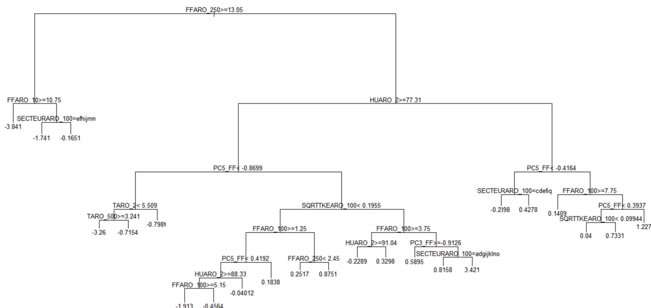
Illustration 8.10: Station de test 1 – FF –Modèle d'arbre de décision (arbre optimal)
