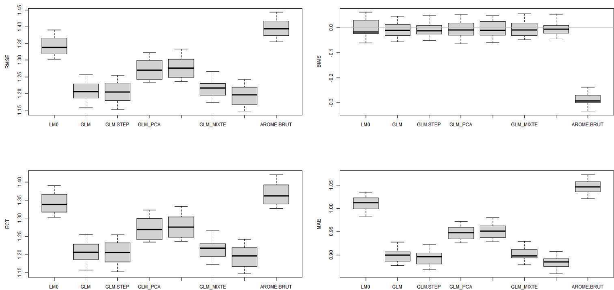
Illustration 8.13: Station de test 1 – FF – Modèles linéaires et AROME.BRUT - Box-plot RMSE, ECT, BIAIS et MAE pour l'échantillon de test
