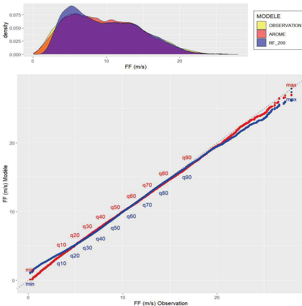
Illustration 3.16: AO6 Méditerranée zone 1 – FF – QQ-Plots sur l'échantillon de test concaténé.
