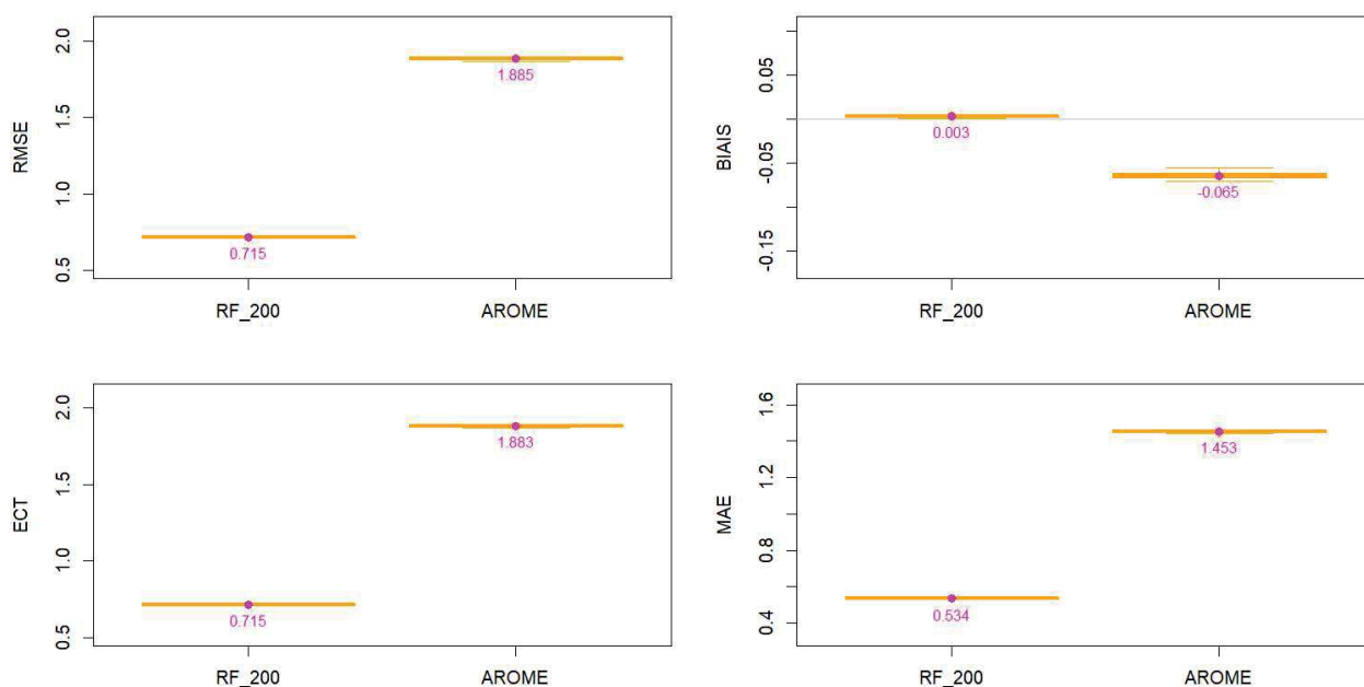
Illustration 3.11: AO6 Méditerranée zone 1 – FF – Modèle de forêt aléatoire à 200 arbres - Box-plot RMSE (haut gauche), ECT (bas gauche), BIAIS (haut droite) et MAE (bas droite) pour l'échantillon d'apprentissage. La valeur en magenta sur chaque boîte à moustaches correspond à la moyenne des 20 échantillons.
