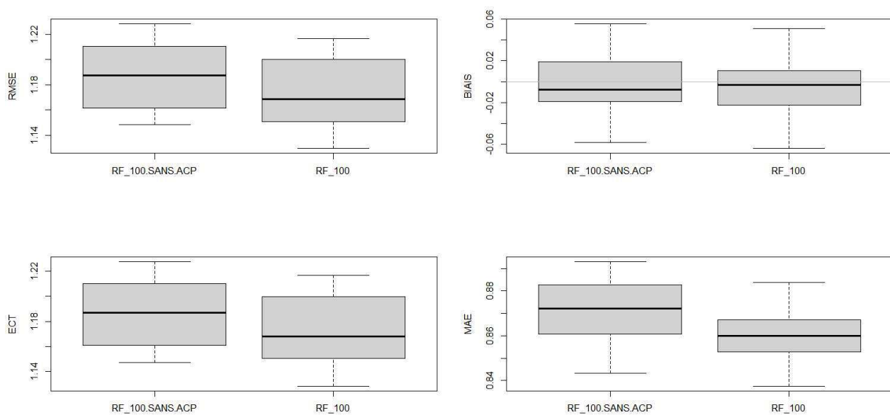
Illustration 8.21: Station de test 1 – FF – Modèles de forêt aléatoire à 100 arbres avec et sans ACP - Box-plot RMSE (haut gauche), ECT (bas gauche), BIAIS (haut droite) et MAE (bas droite) pour l'échantillon de test
