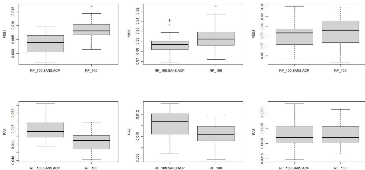
Illustration 8.20: Station de test 1 – FF – Modèles de forêt aléatoire à 100 arbres avec et sans ACP - Box-plot PSS (première ligne pss > 3 m/s, pss > 9 m/s et pss > 12 m/s) et FA (deuxième ligne fa > 3 m/s, fa > 9 m/s et fa > 12 m/s) pour l'échantillon d'apprentissage
