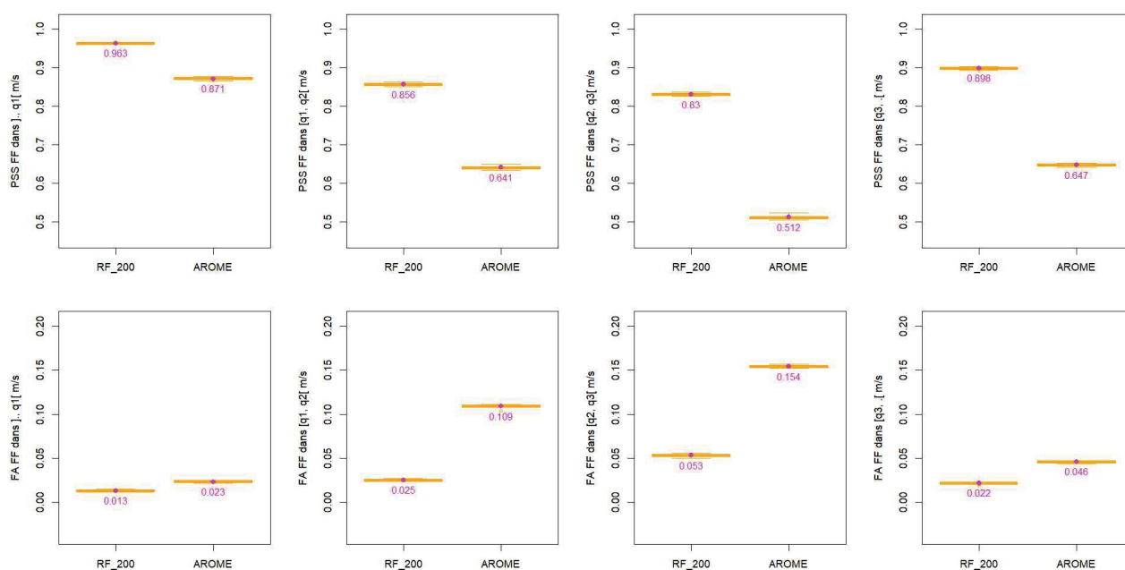
Illustration 3.22: AO6 Méditerranée zone 1 – V – Modèle de forêt aléatoire à 200 arbres - Box-plot PSS (première ligne PSS V \in ]q_1, q_2[ m/s , PSS V \in [q_2, q_3[ m/s et PSS V \in [q_3, .[ m/s ) et FA (deuxième ligne FA V \in ]q_1, q_2[ m/s , FA V \in [q_2, q_3[ m/s et FA V \in [q_3, .[ m/s ) pour l'échantillon d'apprentissage. La valeur en magenta sur chaque boîte à moustaches correspond à la moyenne des 20 échantillons.
