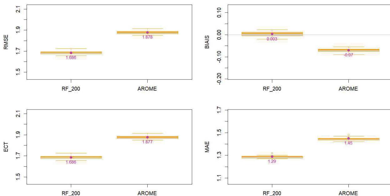
Illustration 3.13: AO6 Méditerranée zone 1 – FF – Modèle de forêt aléatoire - Box-plot RMSE, ECT, BIAIS et MAE pour l'échantillon de test. La valeur en magenta sur chaque boîte à moustaches correspond à la moyenne des 20 échantillons.
