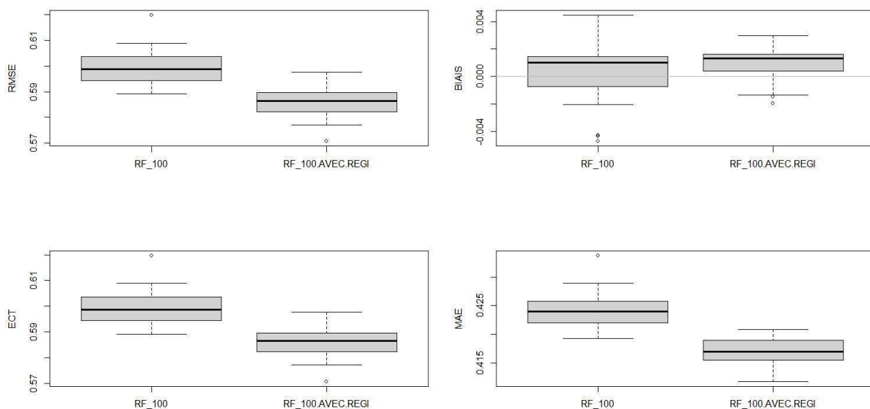
Illustration 8.36: Station de test 2 – FF – Modèles de forêt aléatoire à 100 arbres avec et sans prédicteurs de régimes de temps - Box-plot RMSE (haut gauche), ECT (bas gauche), BIAIS (haut droite) et MAE (bas droite) pour l'échantillon d'apprentissage
