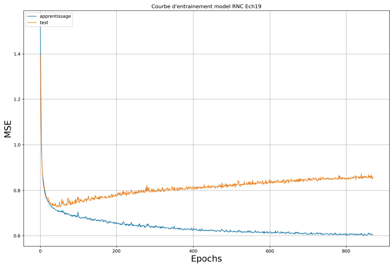
Illustration 8.26: Station de test 1 – FF – Courbe d'entraînement - modèles RNC avec l'optimizer RAdam
