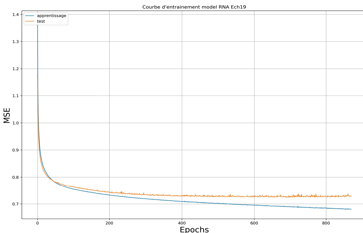
Illustration 8.24: Station de test 1 – FF – Courbe d'entraînement - modèles RNA avec l'optimizer SGD
