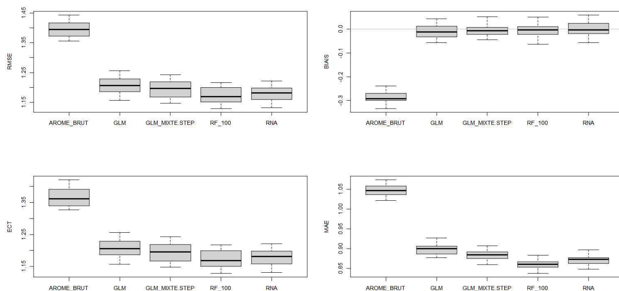
Illustration 8.31: Station de test 1 – FF – Comparaison inter-modèles - Box-plot RMSE (haut gauche), ECT (bas gauche), BIAIS (haut droite) et MAE (bas droite) pour l'échantillon de test
