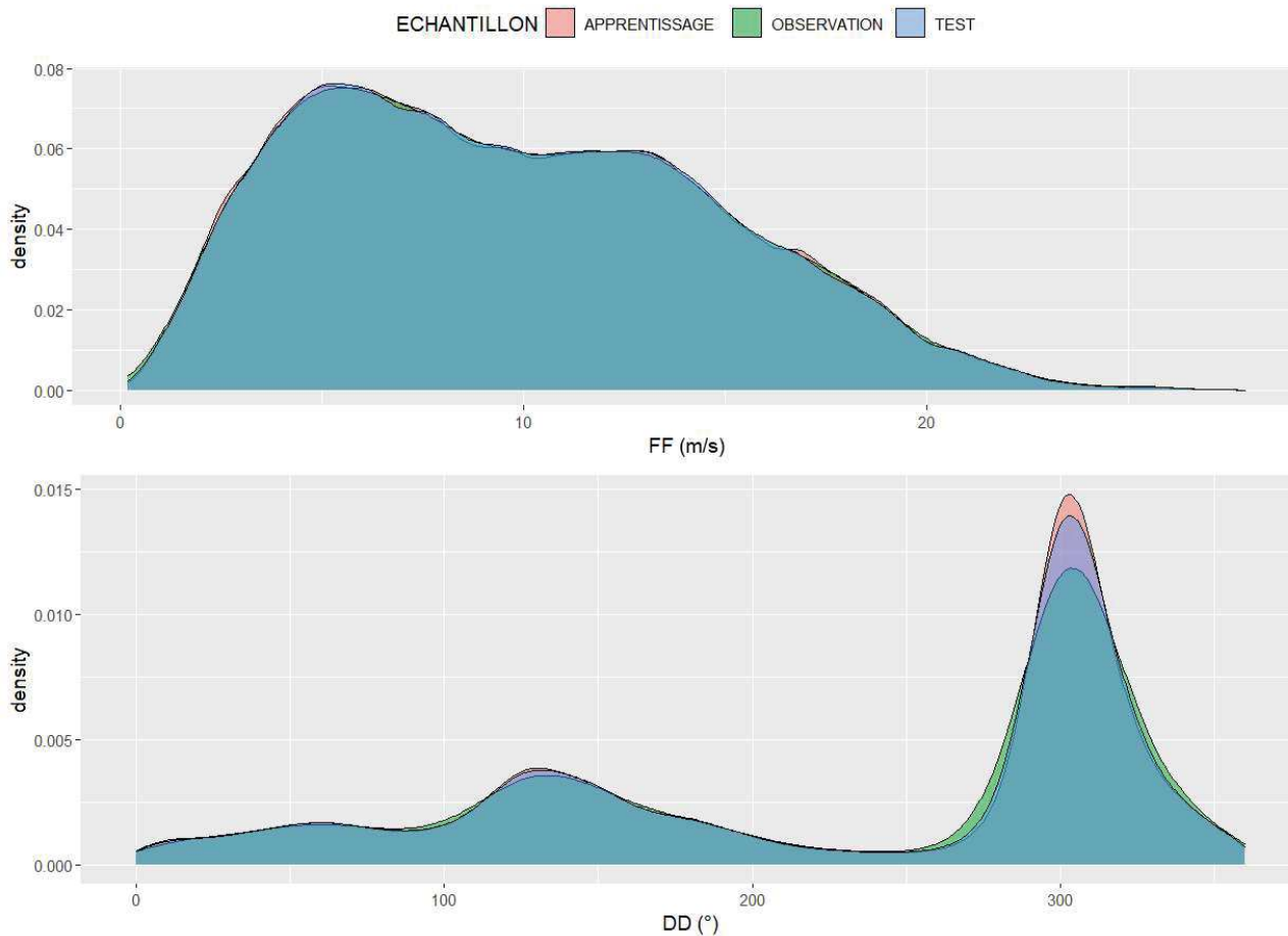
Illustration 3.8: AO6 Méditerranée zone 1 – Distribution de FF (première ligne) et DD (deuxième ligne) pour les échantillons d'apprentissage et de test comparée à celle de l'observation sur la période d'apprentissage (période d'observation)
