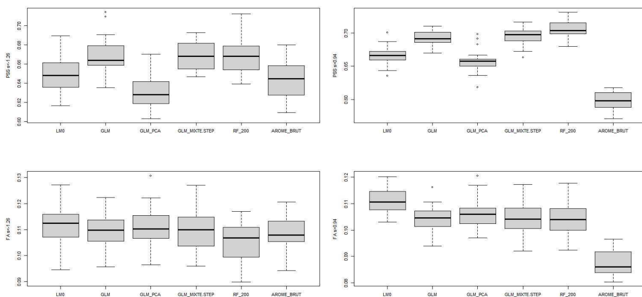
Illustration 8.46: Station de test 1 – U – Modèles linéaires, forêt et AROME - Box-plot PSS et FA pour l'échantillon de test
