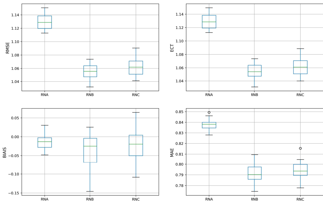
Illustration 8.27: Station de test 1 – FF – Réseau de neurones - Box-plot RMSE, ECT, BIAIS et MAE pour l'échantillon d'apprentissage
