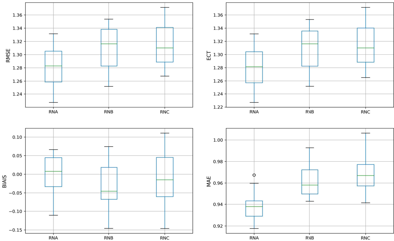
Illustration 8.47: Station de test 1 – V – Réseau de neurones - Box-plot RMSE, ECT, BIAIS et MAE pour l'échantillon de test
