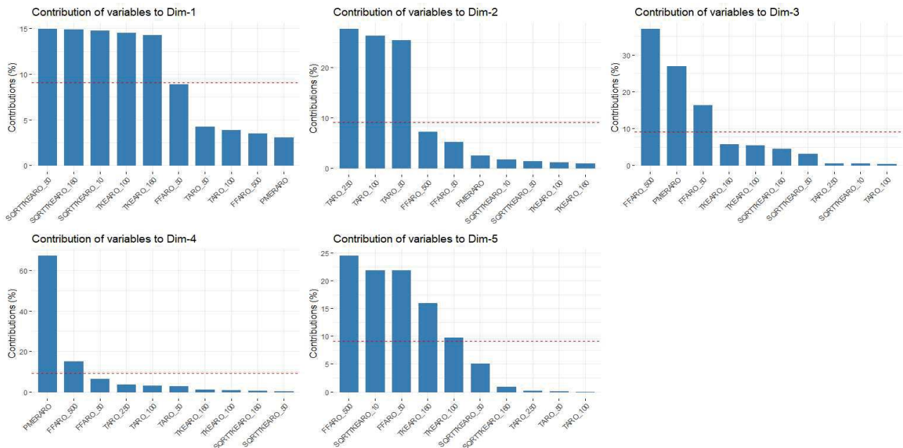
Illustration 8.4: Station de test 1 – FF – Contribution des variables à l'ACP (une figure pour chaque dimension)
