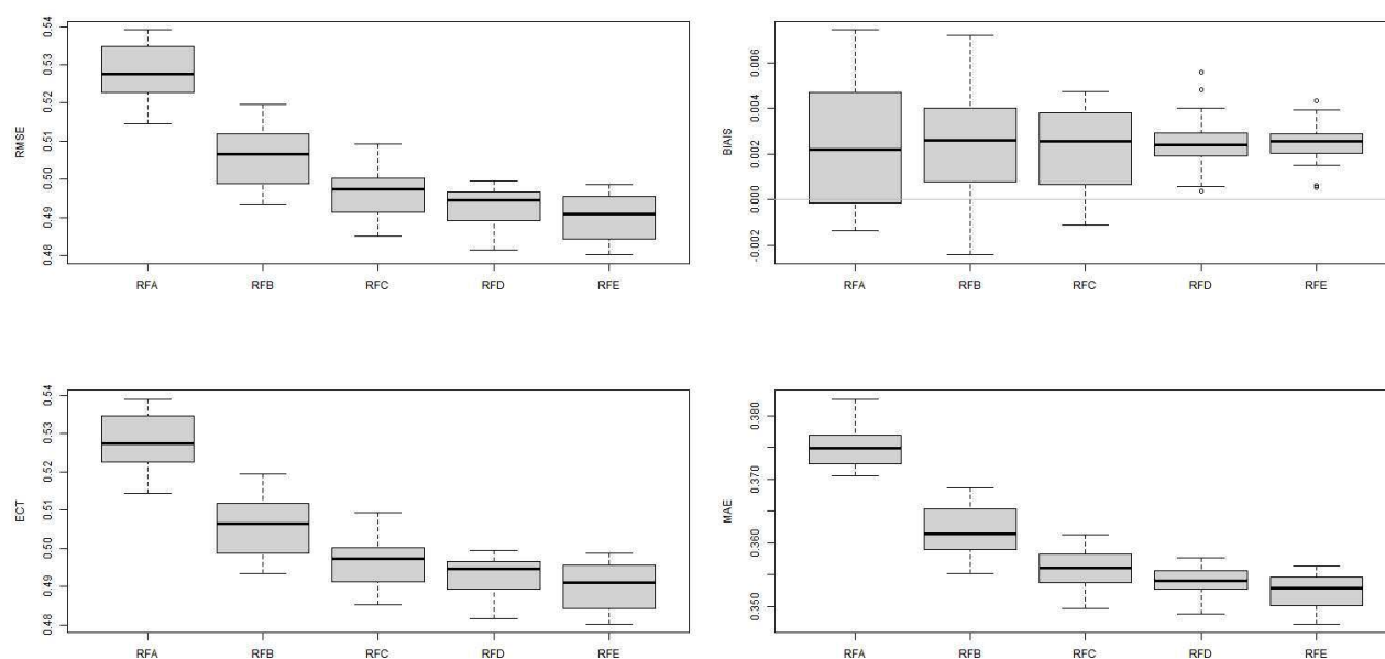
Illustration 8.15: Station de test 1 – FF – Modèles de forêt aléatoire à 20, 50, 100, 200 et 500 arbres - Box-plot RMSE (haut gauche), ECT (bas gauche), BIAIS (haut droite) et MAE (bas droite) pour l'échantillon d'apprentissage
