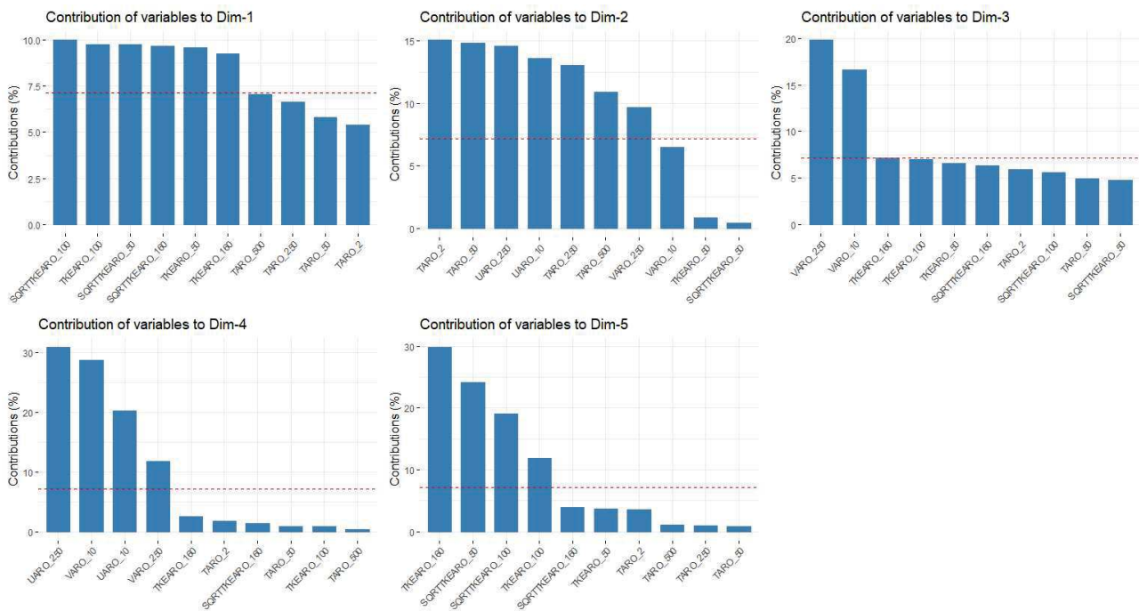
Illustration 3.25: AO6 Méditerranée zone 1 – DD – Contribution des variables à l'ACP (une figure pour chaque dimension)
