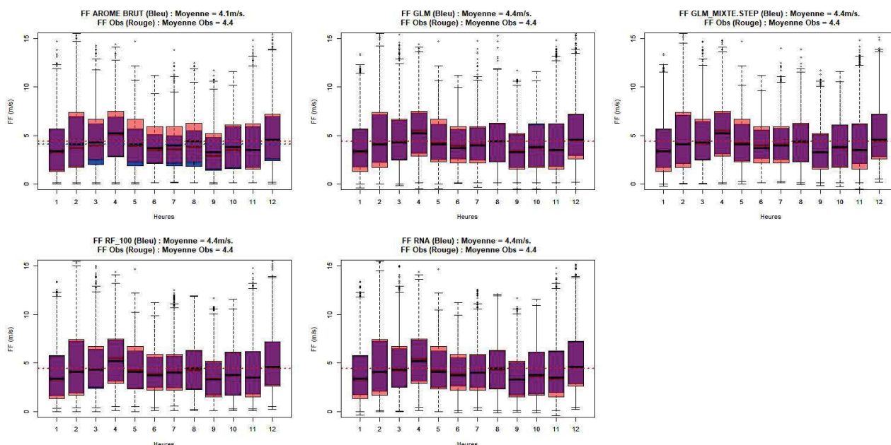
Illustration 8.35: Station de test 1 – FF – Cycle annuel des modèles statistiques (bleu) superposé aux observations (rouge)
