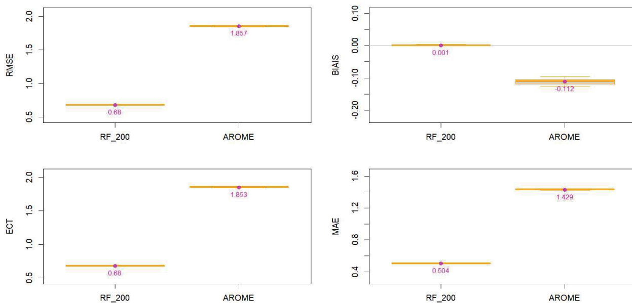
Illustration 3.21: AO6 Méditerranée zone 1 – V – Modèle de forêt aléatoire à 200 arbres - Box-plot RMSE (haut gauche), ECT (bas gauche), BIAIS (haut droite) et MAE (bas droite) pour l'échantillon d'apprentissage. La valeur en magenta sur chaque boîte à moustaches correspond à la moyenne des 20 échantillons.
