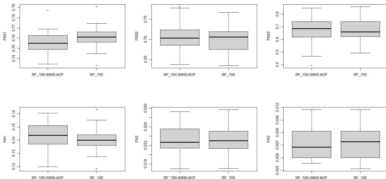
Illustration 8.22: Station de test 1 – FF – Modèles de forêt aléatoire à 100 arbres avec et sans ACP - Box-plot PSS (première ligne pss > 3 m/s, pss > 9 m/s et pss > 12 m/s) et FA (deuxième ligne fa > 3 m/s, fa > 9 m/s et fa > 12 m/s) pour l'échantillon de test
