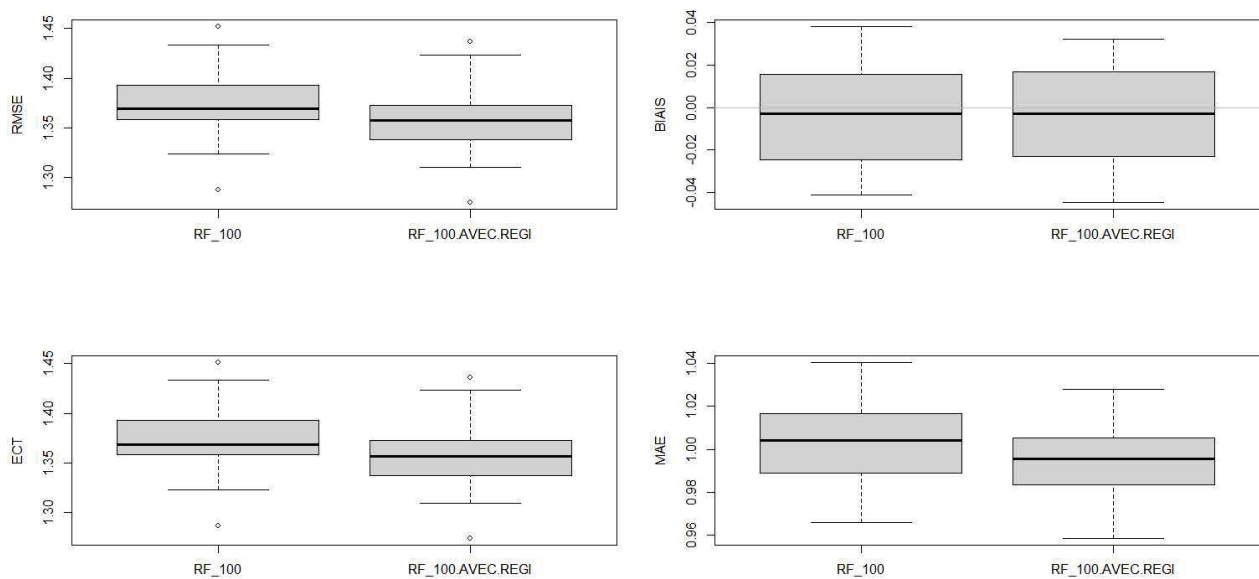
Illustration 8.38: Station de test 2 – FF – Modèles de forêt aléatoire à 100 arbres avec et sans prédicteurs de régimes de temps - Box-plot RMSE (haut gauche), ECT (bas gauche), BIAIS (haut droite) et MAE (bas droite) pour l'échantillon de test
