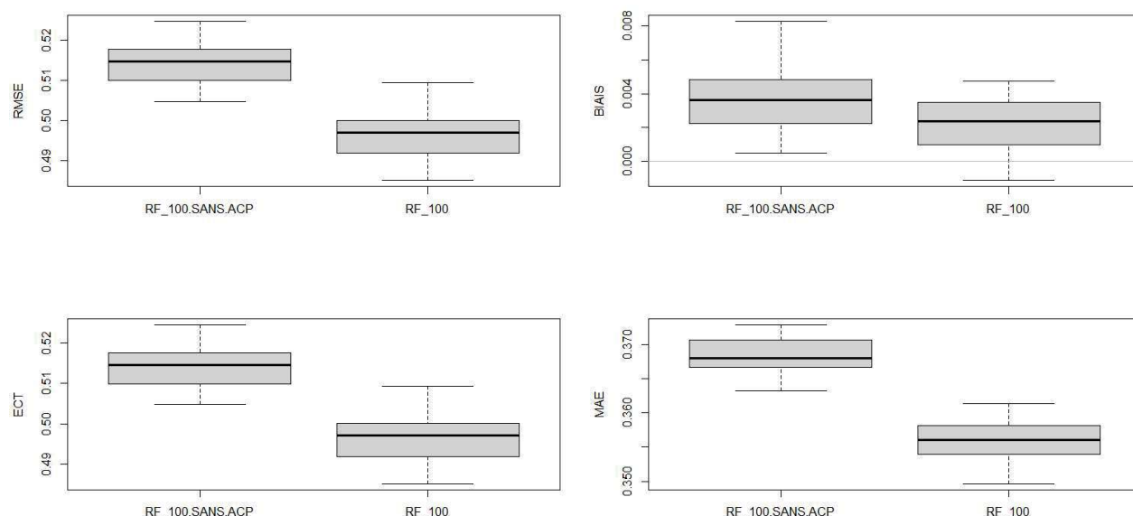
Illustration 8.19: Station de test 1 – FF – Modèles de forêt aléatoire à 100 arbres avec et sans ACP - Box-plot RMSE (haut gauche), ECT (bas gauche), BIAIS (haut droite) et MAE (bas droite) pour l'échantillon d'apprentissage
