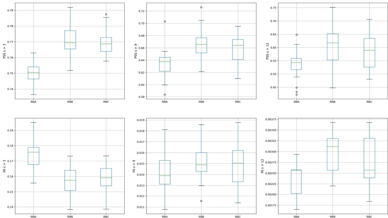
Illustration 8.28: Station de test 1 – FF – Réseau de neurones - Box-plot PSS et FA pour l'échantillon d'apprentissage
