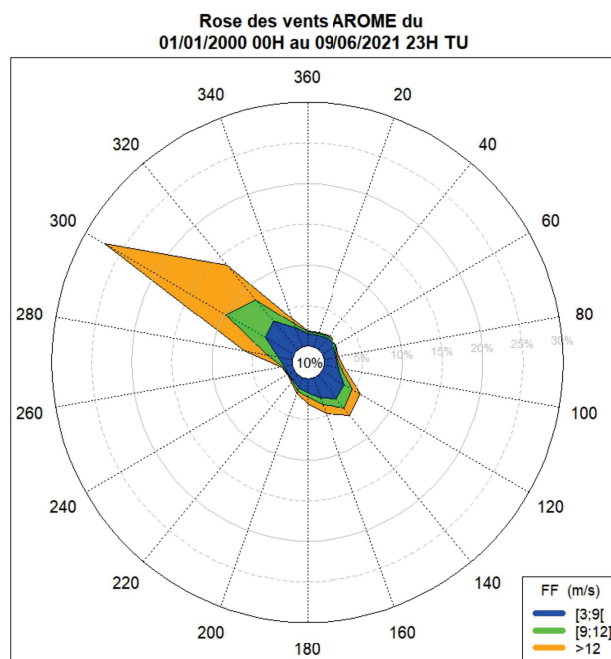
Illustration 4.7: AO6 Méditerranée zone 1 – Roses des vents sur la période d'extension du 01/01/2000 00H TU au 09/06/2021 23H TU : à gauche on retrouve la rose de l'extension statistique et à droite la rose d'AROME.
