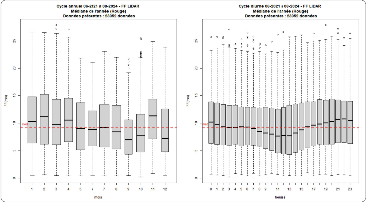
Illustration 3.4: AO6 Méditerranée zone 1 – FF – Distribution du vent permettant de déterminer le cycle saisonnier (gauche) et le cycle diurne (droite)
