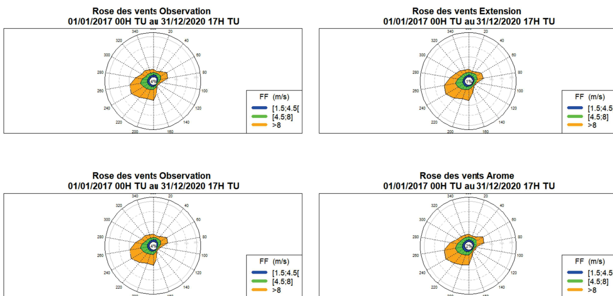
Illustration 8.53: Station de test 2 – Roses des vents finales de l'extension entre l'année 2017 et 2020 (sans les données d'apprentissage de l'année 2018)
