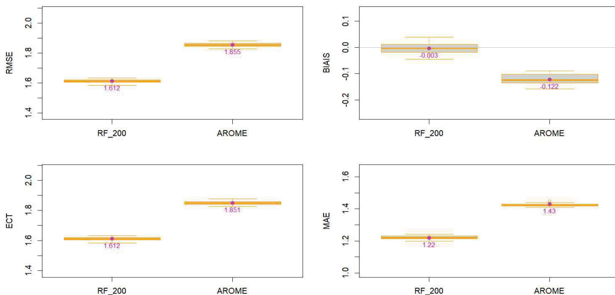
Illustration 3.23: AO6 Méditerranée zone 1 – V – Modèle de forêt aléatoire à 200 arbres - Box-plot RMSE, ECT, BIAIS et MAE pour l'échantillon de test. La valeur en magenta sur chaque boîte à moustaches correspond à la moyenne des 20 échantillons.
