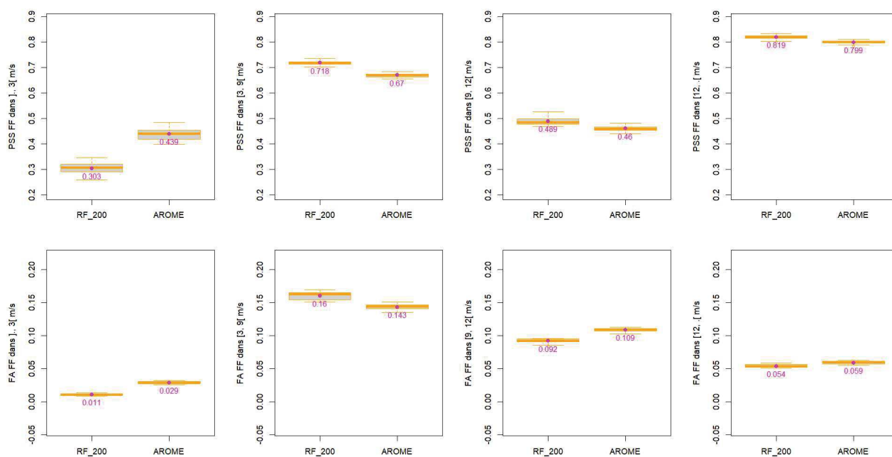
Illustration 3.14: AO6 Méditerranée zone 1 – FF – Modèle de forêt aléatoire - Box-plot PSS et FA pour l'échantillon de test. La valeur en magenta sur chaque boîte à moustaches correspond à la moyenne des 20 échantillons.
