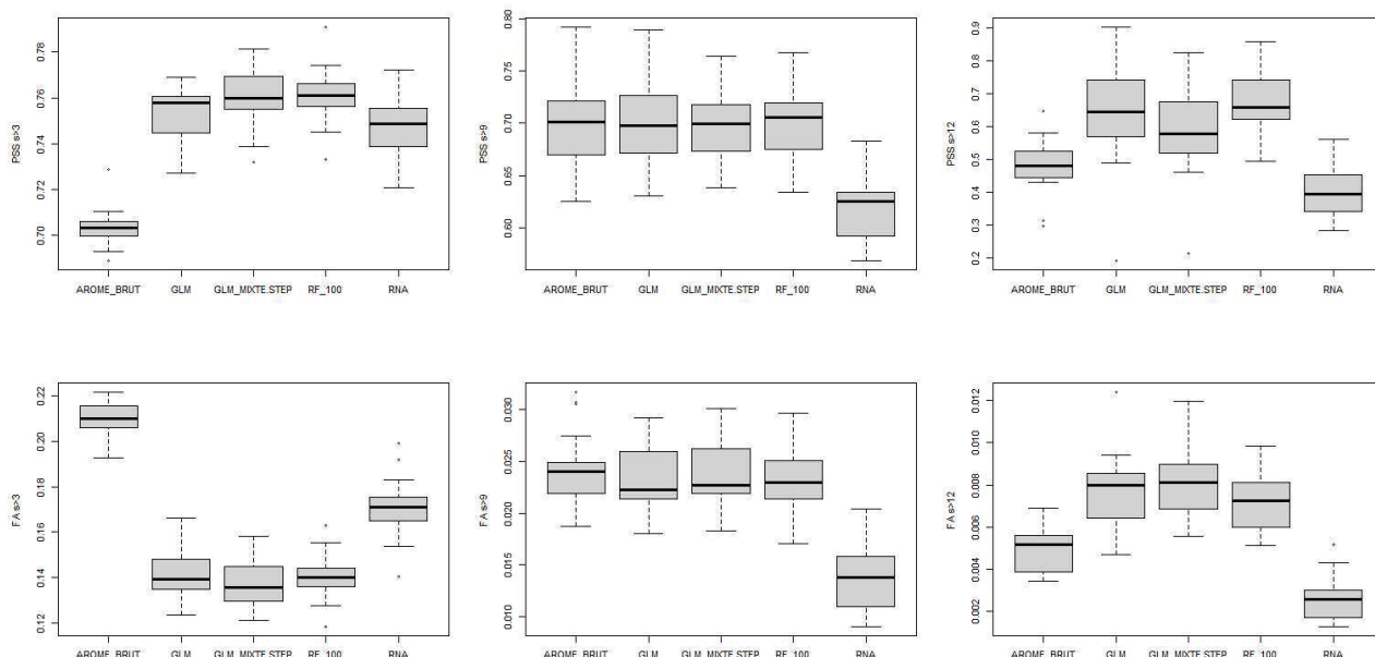
Illustration 8.32: Station de test 1 – FF – Comparaison inter-modèles - Box-plot PSS (première ligne pss > 3 m/s, pss > 9 m/s et pss > 12 m/s) et FA (deuxième ligne fa > 3 m/s, fa > 9 m/s et fa > 12 m/s) pour l'échantillon de test
