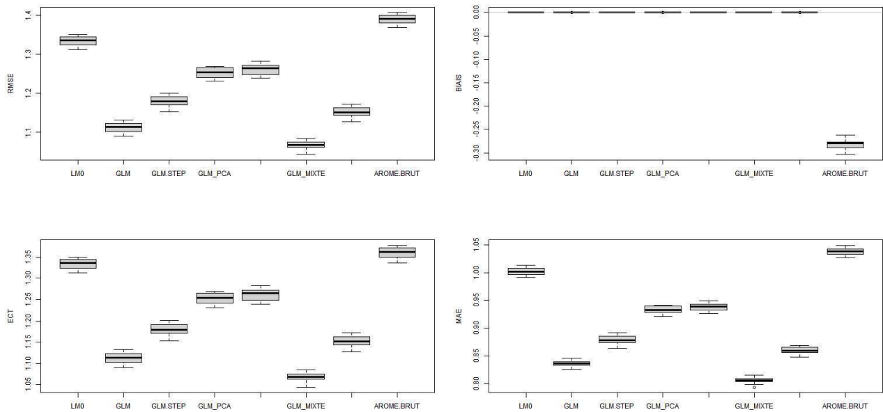
Illustration 8.11: Station de test 1 – FF – Modèles linéaires et AROME.BRUT - Box-plot RMSE (haut gauche), ECT (bas gauche), BIAIS (haut droite) et MAE (bas droite) pour l'échantillon d'apprentissage
