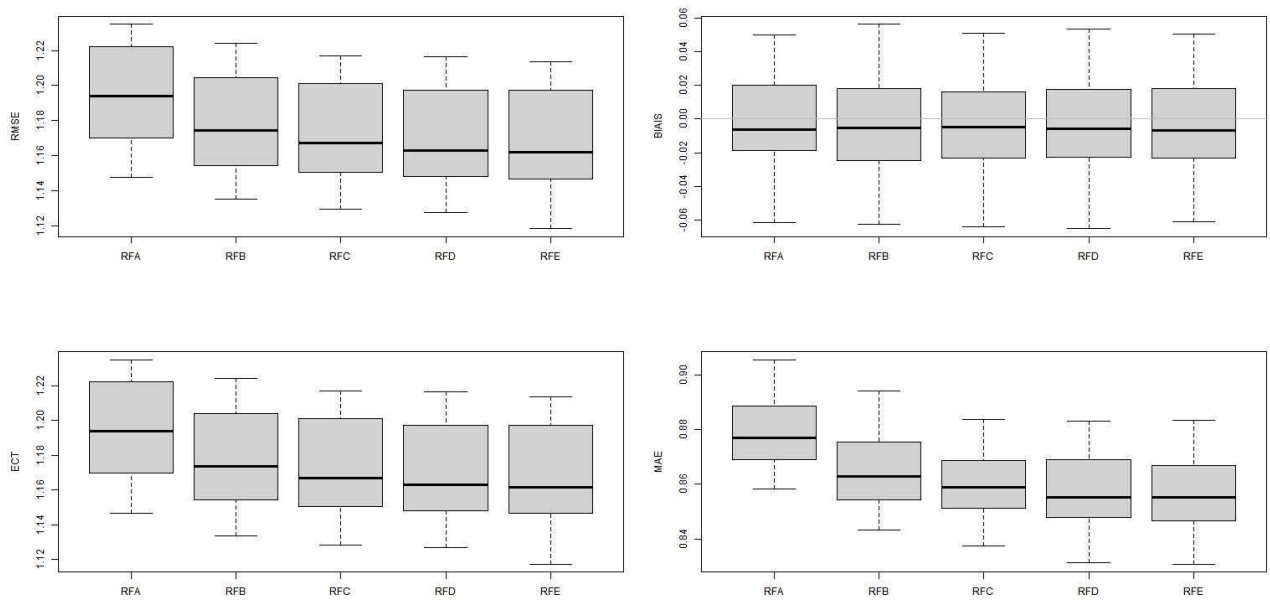
Illustration 8.17: Station de test 1 – FF – Modèles de forêt aléatoire - Box-plot RMSE, ECT, BIAIS et MAE pour l'échantillon de test
