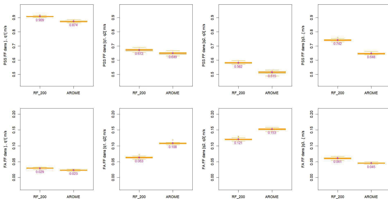
Illustration 3.24: AO6 Méditerranée zone 1 – V – Modèle de forêt aléatoire à 200 arbres - Box-plot PSS et FA pour l'échantillon de test. La valeur en magenta sur chaque boîte à moustaches correspond à la moyenne des 20 échantillons.
