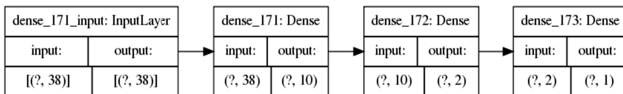
Illustration 8.23: Station de test 1 – Architecture du réseau conservé pour la modélisation de FF
