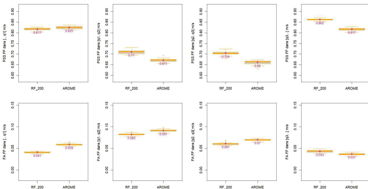
Illustration 3.20: AO6 Méditerranée zone 1 – U – Modèle de forêt aléatoire à 200 arbres - Box-plot PSS et FA pour l'échantillon de test. La valeur en magenta sur chaque boîte à moustaches correspond à la moyenne des 20 échantillons.
