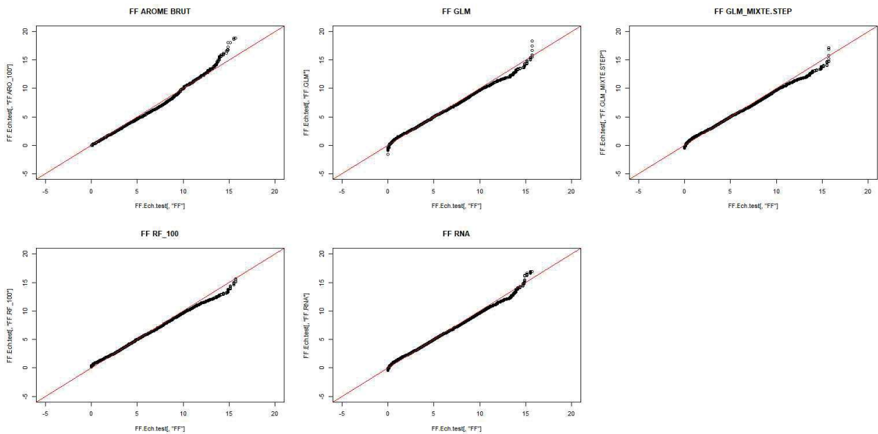
Illustration 8.33: Station de test 1 – FF – QQ-Plot de FF pour les modèles GLM, GLM_MIXTE.STEP, RF_100, RNA et AROME
