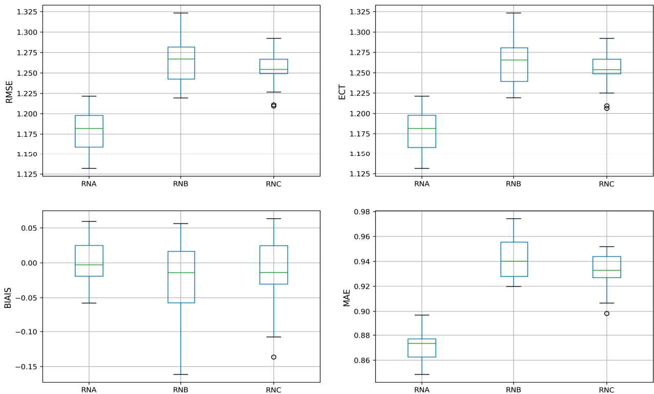
Illustration 8.29: Station de test 1 – FF – Réseau de neurones - Box-plot RMSE, ECT, BIAIS et MAE pour l'échantillon de test
