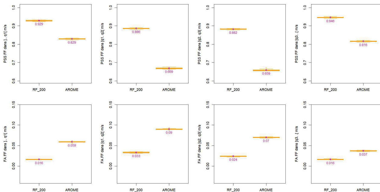
Illustration 3.18: AO6 Méditerranée zone 1 – U – Modèle de forêt aléatoire à 200 arbres - Box-plot PSS (première ligne PSS U \in ] , q_1[ m/s , PSS U \in [q_1, q_2[ m/s , PSS U \in [q_2, q_3[ m/s et PSS U \in [q_3, .[ m/s ) et FA (deuxième ligne FA U \in ] , q_1[ m/s , FA U \in [q_1, q_2[ m/s , FA U \in [q_2, q_3[ m/s et FA U \in [q_3, .[ m/s ) pour l'échantillon d'apprentissage. La valeur en magenta sur chaque boîte à moustaches correspond à la moyenne des 20 échantillons.
