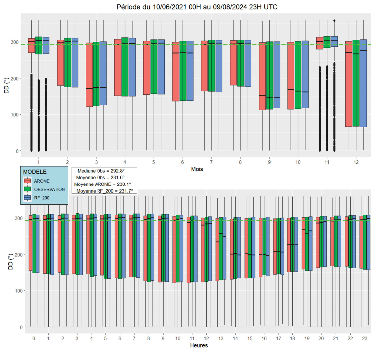
Illustration 4.2: AO6 Méditerranée zone 1 – DD – Restitution des cycles de DD sur la période d'observation (du 10/06/2021 00H au 09/08/2024 23H). Sur la première ligne on retrouve le cycle annuel et sur la deuxième ligne le cycle diurne. La ligne discontinue verte traversant les boxplots désigne la médiane de l'observation sur la période d'observation.
