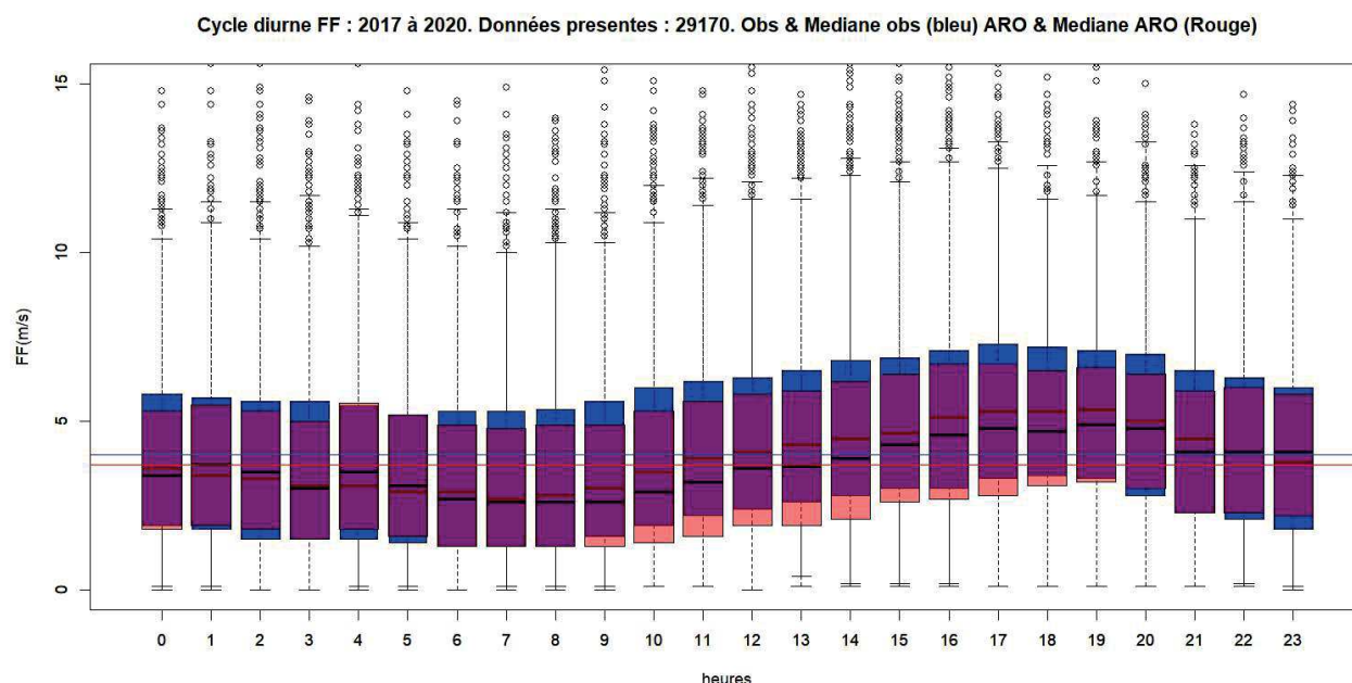
Illustration 8.2: Station de test 1 – Cycle diurne de la force du vent observée (bleu) et AROME (rouge) de 2017 à 2020.
