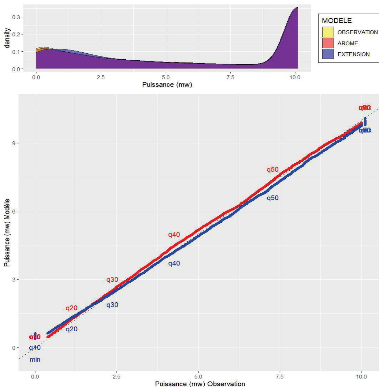
Illustration 4.5: AO6 Méditerranée zone 1 – QQ-Plot des données de puissances sur la période d'observation pour l'extension statistique (bleu) et AROME (rouge).
