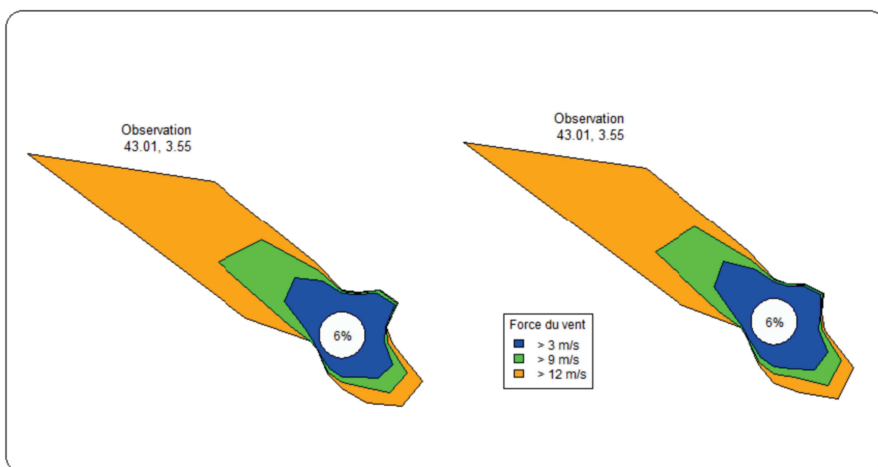
Illustration 6.1: AO6 Méditerranée zone 1 – Roses des vents du point d'observation – de gauche à droite on retrouve respectivement les roses de la campagne 1 (10/06/2021 00H TU au 30/09/2022 23 TU) et de la campagne « 1 et 2 » (du 10/06/2021 00H TU au 09/08/2024 23H TU).
