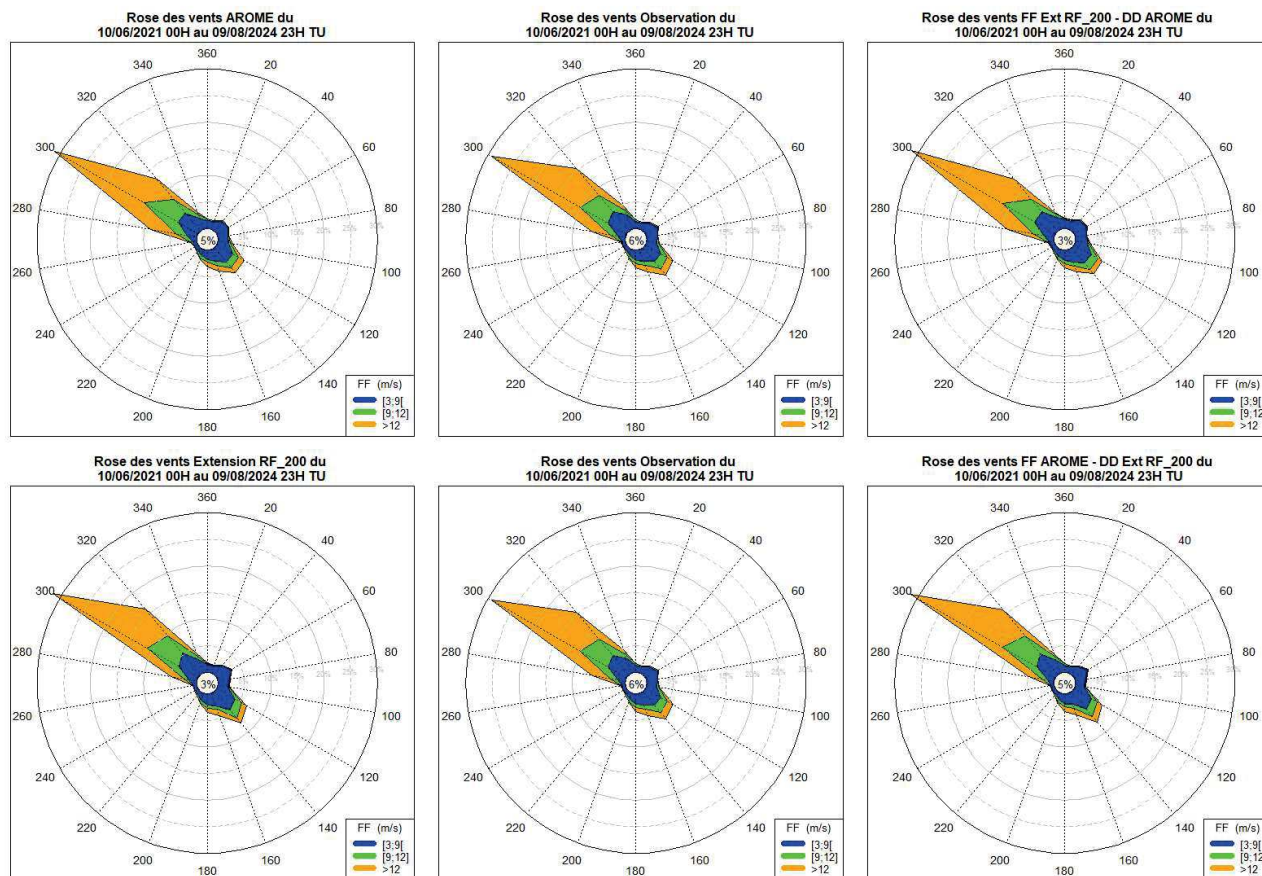
Illustration 4.3: AO6 Méditerranée zone 1 – Roses des vents sur la période d'observation (du 10/06/2021 00H au 09/08/2024 23H) : sur la 1ère colonne (de haut en bas) on retrouve la rose AROME et celle de l'extension ; sur la 2ème colonne on retrouve la rose de l'observation. Les deux vignettes de cette colonne sont identiques et ont été dupliquées par soucis de lisibilité ; et sur la 3ème colonne (de haut en bas) on retrouve respectivement les roses issues de FF Extension et DD AROME, FF AROME et DD Extension
