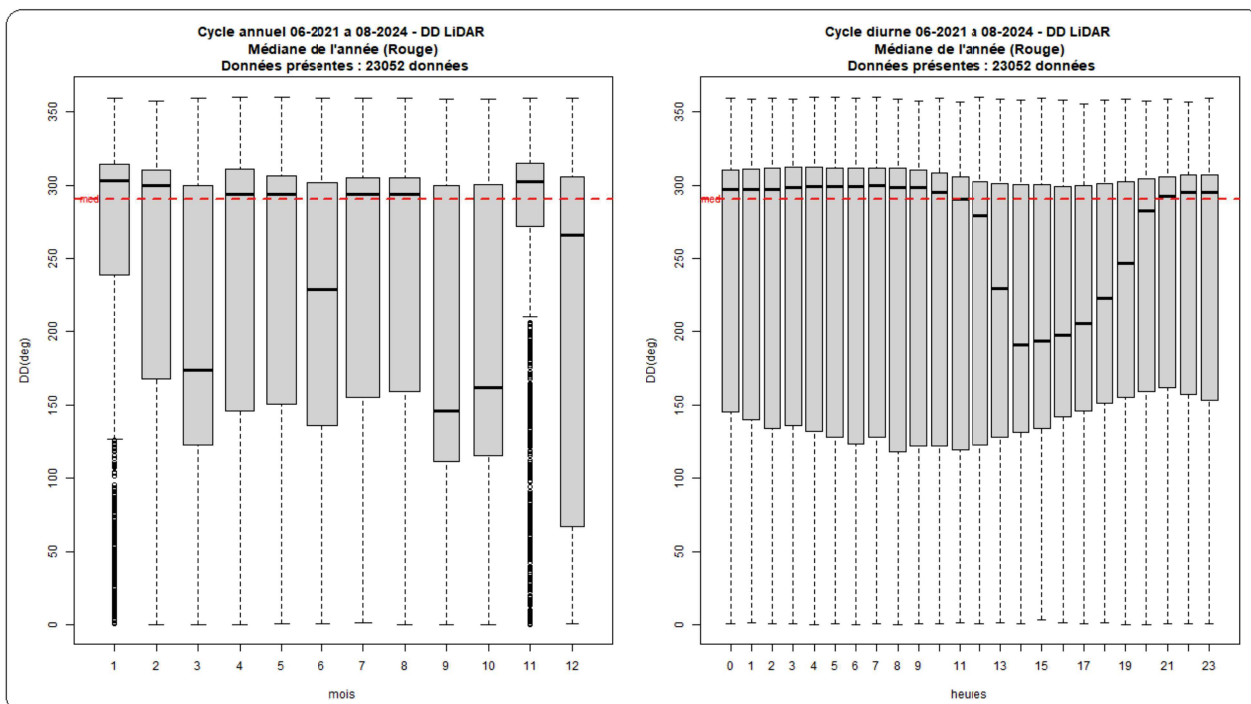
Illustration 3.7: AO6 Méditerranée zone 1 – DD – Distribution du vent permettant de déterminer le cycle saisonnier (graphique à gauche) et cycle diurne (graphique à droite)
