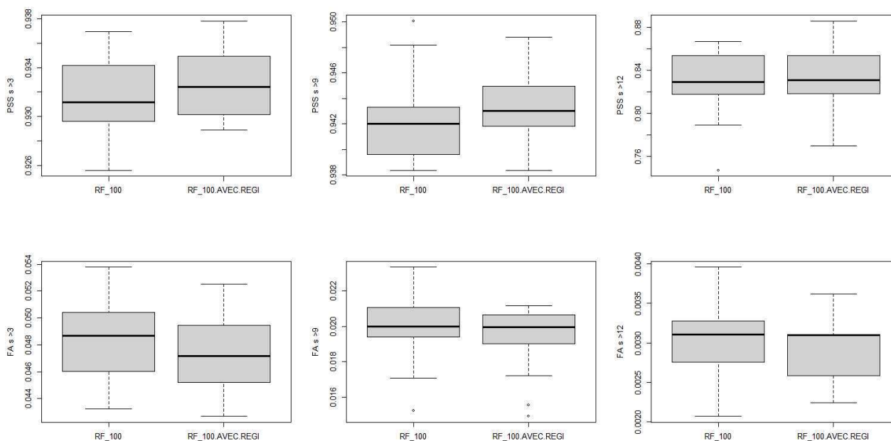
Illustration 8.37: Station de test 2 – FF – Modèles de forêt aléatoire à 100 arbres avec et sans prédicteurs de régimes de temps - Box-plot PSS (première ligne pss > 3 m/s, pss > 9 m/s et pss > 12 m/s) et FA (deuxième ligne fa > 3 m/s, fa > 9 m/s et fa > 12 m/s) pour l'échantillon d'apprentissage
