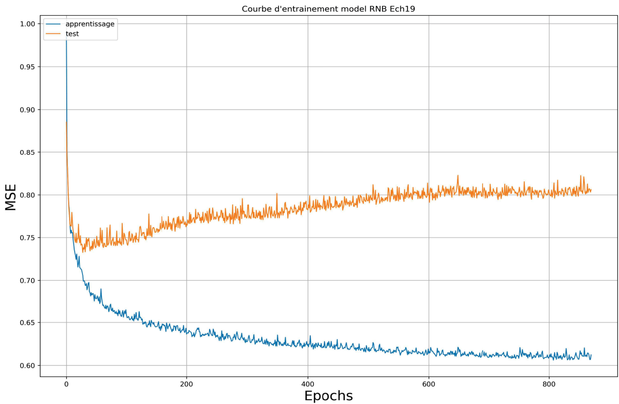
Illustration 8.25: Station de test 1 – FF – Courbe d'entraînement - modèles RNB avec l'optimizer Adam
