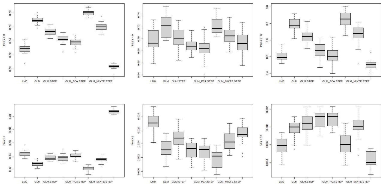
Illustration 8.12: Station de test 1 – FF – Modèles linéaires et AROME.BRUT - Box-plot PSS (première ligne pss > 3 m/s, pss > 9 m/s et pss > 12 m/s noté respectivement pss1, pss2 et pss3) et FA (deuxième ligne fa > 3 m/s, fa > 9 m/s et fa > 12 m/s notée respectivement fa1, fa2 et fa3) pour l'échantillon d'apprentissage
