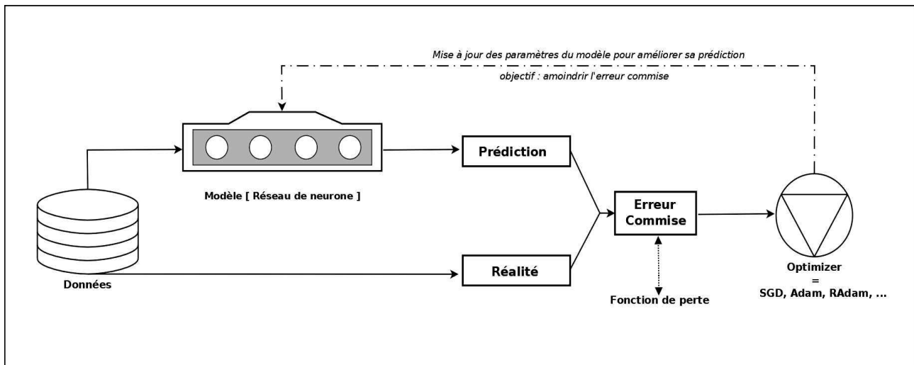
Illustration 7.2: Processus de fonctionnement de la fonction de perte et de la mise à jour des paramètres du réseau
