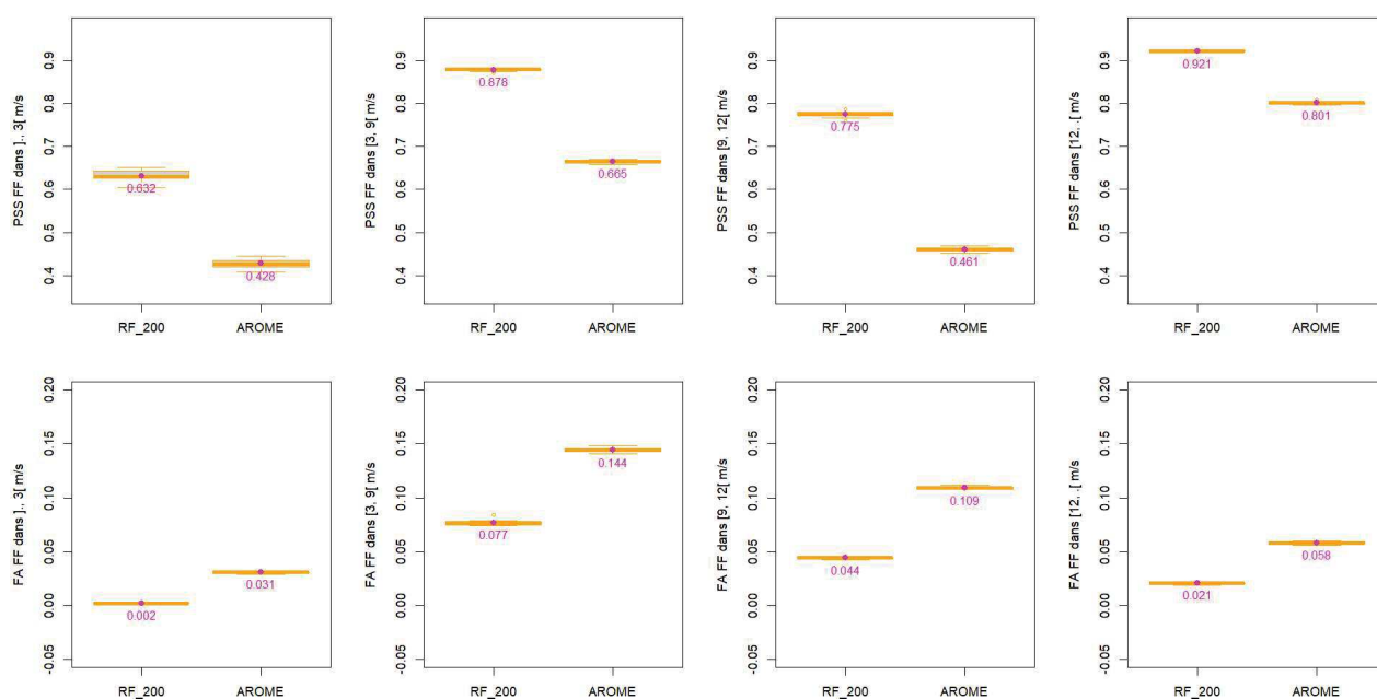
Illustration 3.12: AO6 Méditerranée zone 1 – FF – Modèle de forêt aléatoire à 200 arbres - Box-plot PSS (première ligne PSS FF \in ]., 3[ \text{ m/s} , PSS FF \in [3, 9[ \text{ m/s} , PSS FF \in [9, 12[ \text{ m/s} et PSS FF \in [12, .[ \text{ m/s} ) et FA (deuxième ligne FA FF \in ]., 3[ \text{ m/s} , FA FF \in [3, 9[ \text{ m/s} , FA FF \in [9, 12[ \text{ m/s} et FA FF \in [12, .[ \text{ m/s} ) pour l'échantillon d'apprentissage. La valeur en magenta sur chaque boîte à moustaches correspond à la moyenne des 20 échantillons.
