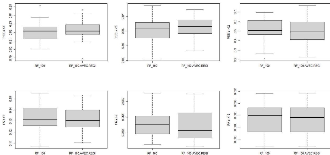
Illustration 8.39: Station de test 2 – FF – Modèles de forêt aléatoire à 100 arbres avec et sans prédicteurs de régimes de temps - Box-plot PSS (première ligne pss > 3 m/s, pss > 9 m/s et pss > 12 m/s) et FA (deuxième ligne fa > 3 m/s, fa > 9 m/s et fa > 12 m/s) pour l'échantillon de test
