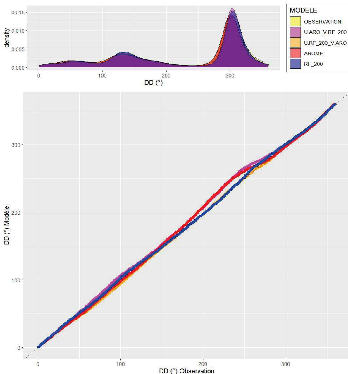
Illustration 3.26: AO6 Méditerranée zone 1 – DD – QQ-Plots de la reconstitution de DD avec combinaison de U et V sur l'échantillon de test concaténé.
