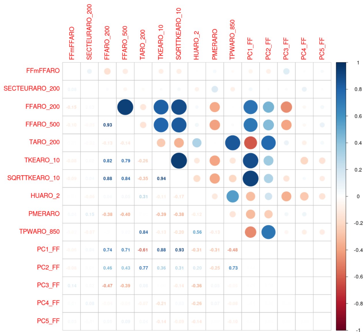
Illustration 8.11 : AO4 Barfleur – 200 M – Variables explicatives finales (avec les composantes principales de l'ACP) pour la prédiction de FF
