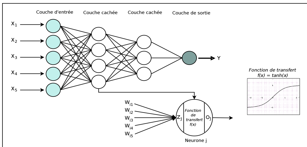
Illustration 6.1 : Réseau de neurones multicouches
