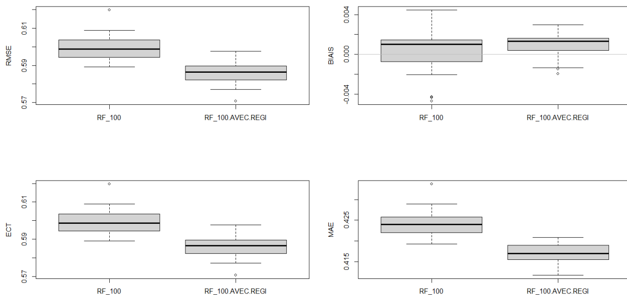
Illustration 7.36 : Station de test 2 – FF – Modèles de forêt aléatoire à 100 arbres avec et sans prédicteurs de régimes de temps - Box-plot RMSE (haut gauche), ECT (bas gauche), BIAIS (haut droite) et MAE (bas droite) pour l'échantillon d'apprentissage
