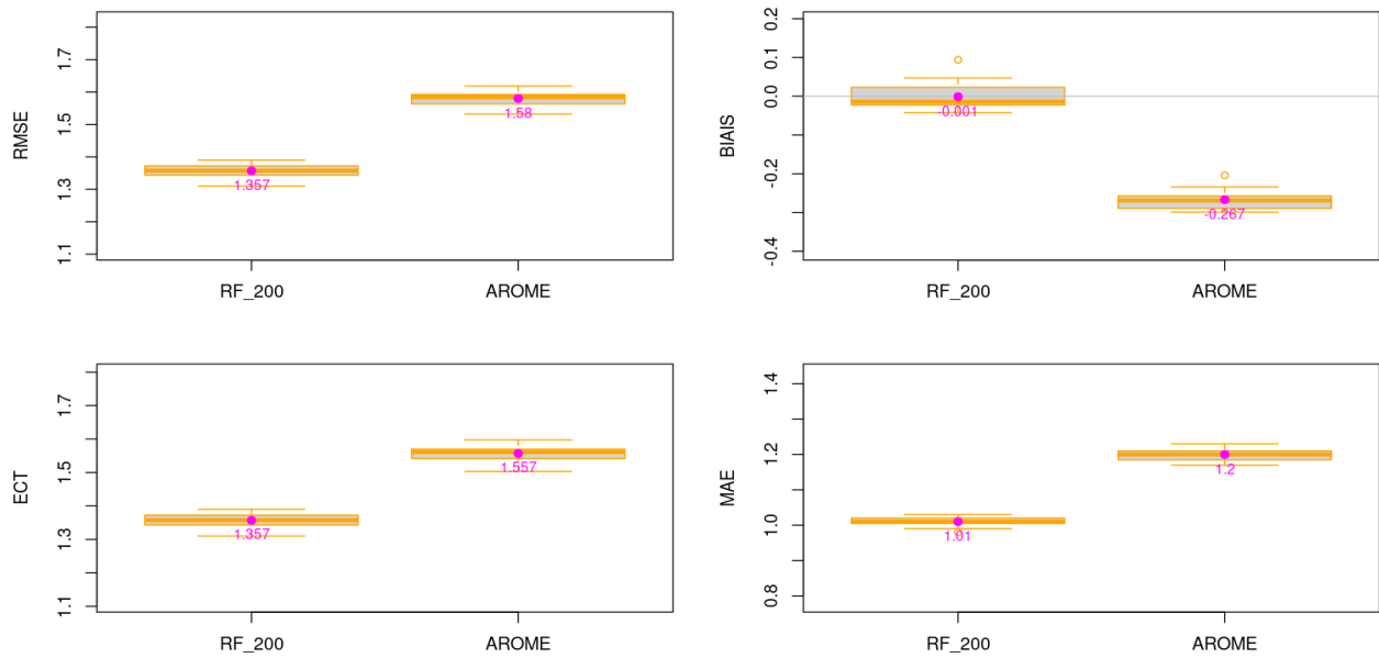
Illustration 3.23 : BNO – V – Niveau 100 m – Modèle de forêt aléatoire à 200 arbres - Box-plot RMSE, ECT, BIAIS et MAE pour l'échantillon de test. La valeur en magenta sur chaque boîte à moustaches correspond à la moyenne des 20 échantillons.
