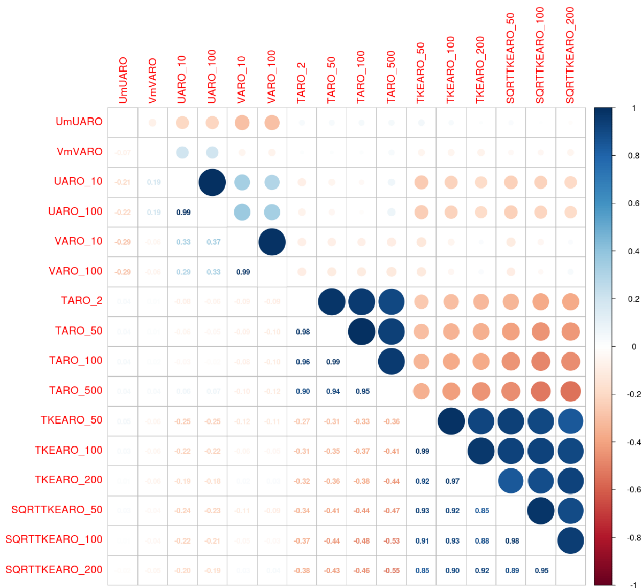
Illustration 8.41 : AO4 Barfleur – 200 M – Deuxième groupe (variables de l'ACP) pour la prédiction de DD
