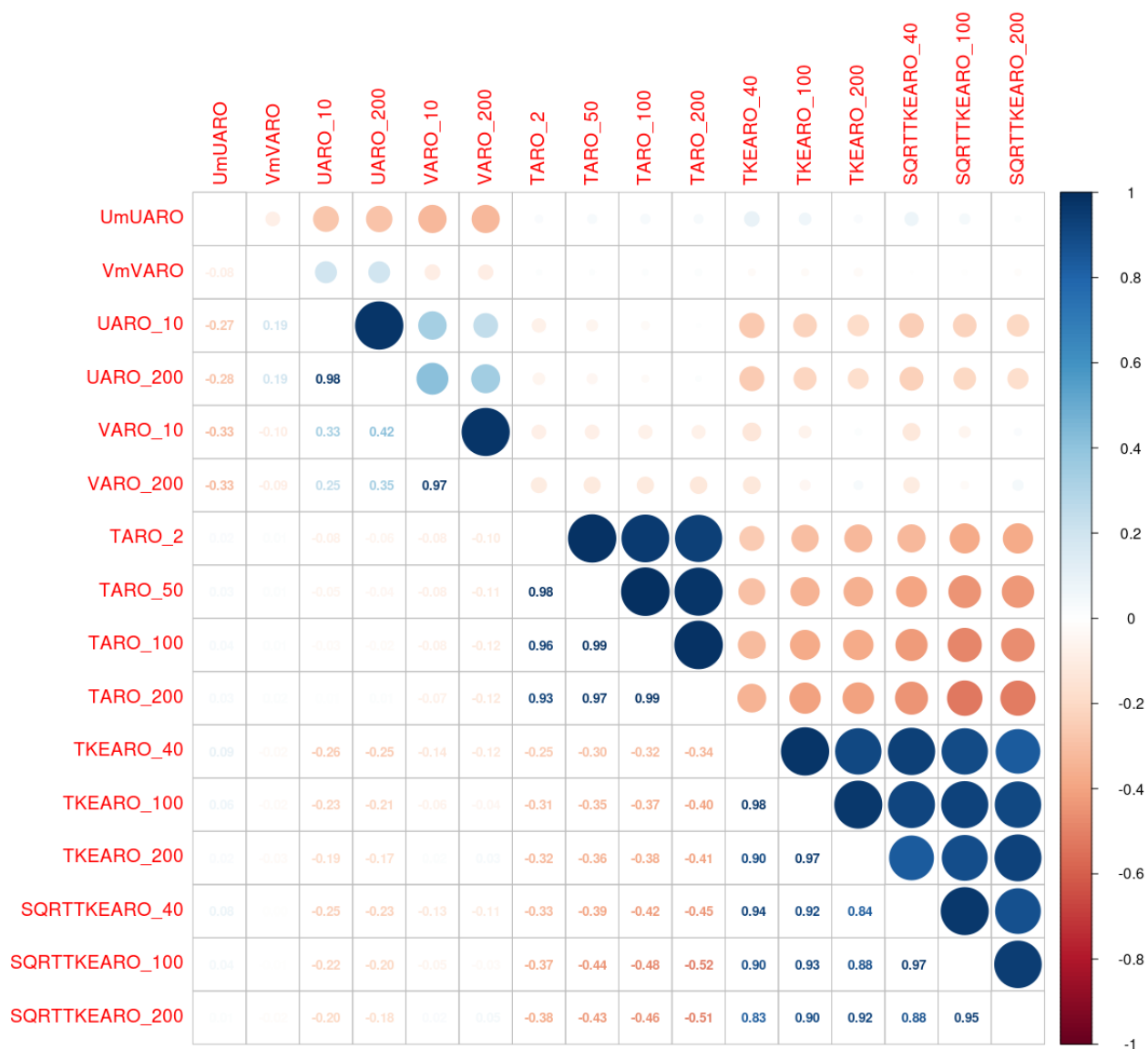
Illustration 8.35 : AO4 Barfleur – 40 M – Deuxième groupe (variables de l'ACP) pour la prédiction de DD
