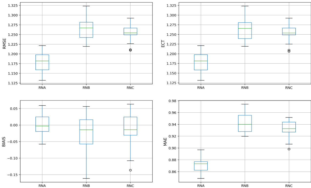
Illustration 7.29 : Station de test 1 – FF – Réseau de neurones - Box-plot RMSE, ECT, BIAIS et MAE pour l'échantillon de test
