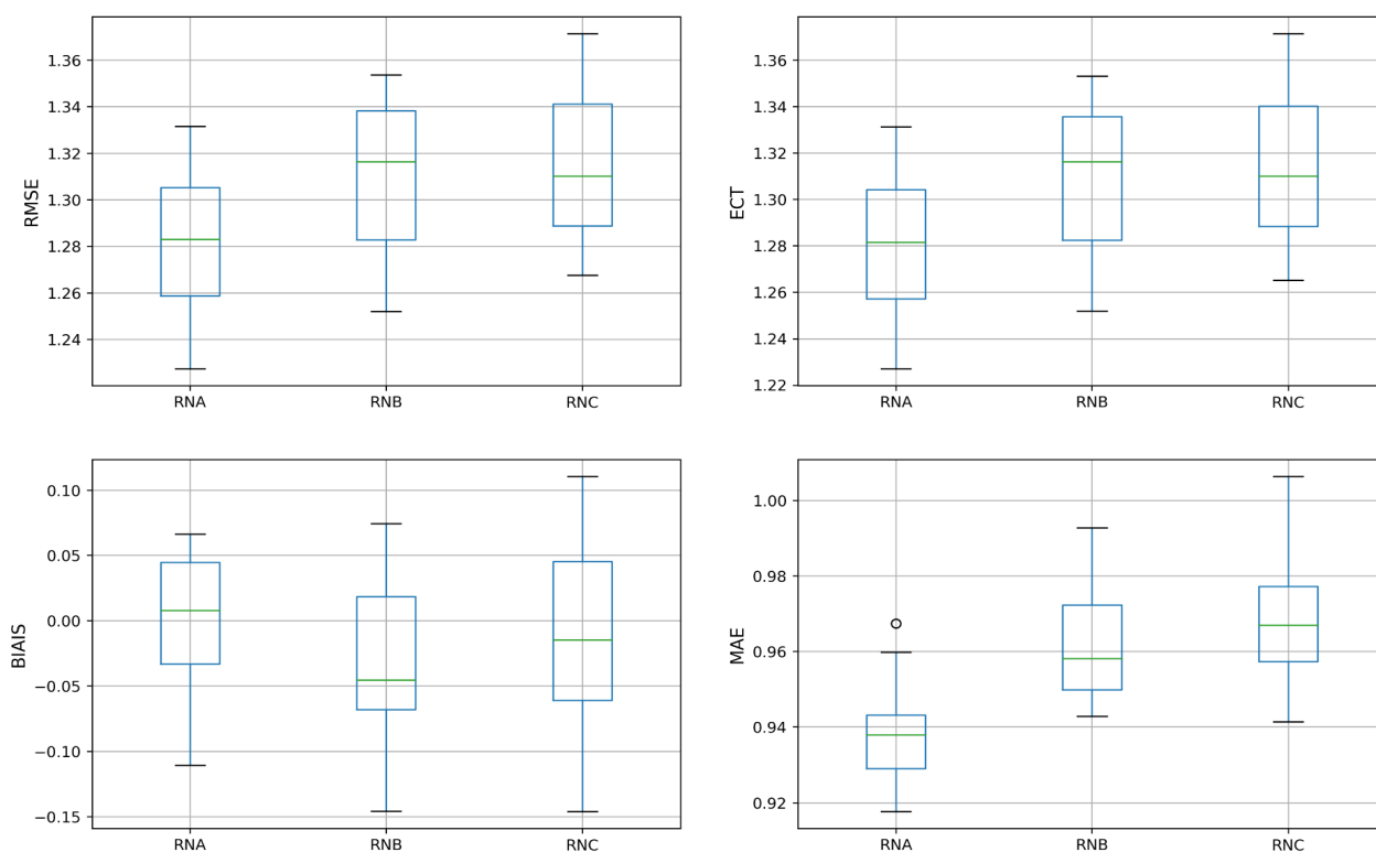
Illustration 7.47 : Station de test 1 – V – Réseau de neurones - Box-plot RMSE, ECT, BIAIS et MAE pour l'échantillon de test
