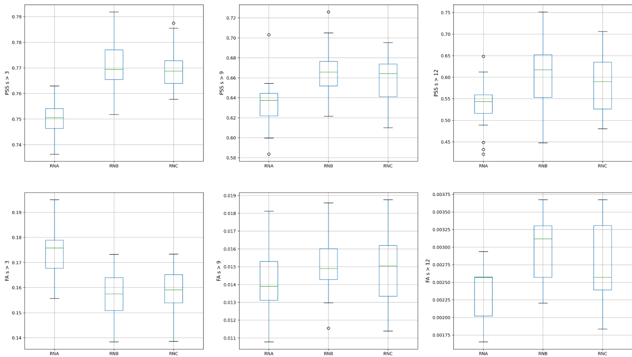
Illustration 7.28 : Station de test 1 – FF – Réseau de neurones - Box-plot PSS et FA pour l'échantillon d'apprentissage
