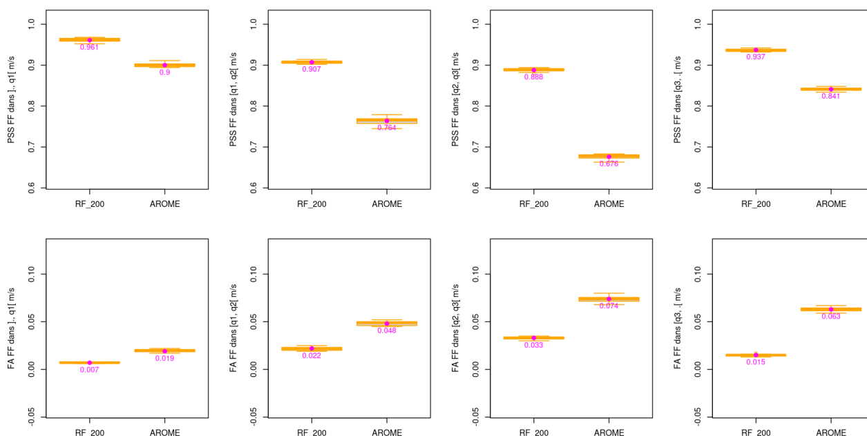
Illustration 3.18 : BNO – U – Niveau 100 m – Modèle de forêt aléatoire à 200 arbres - Box-plot PSS (première ligne PSS U \in ., q_1[ m/s , PSS U \in [q_1, q_2[ m/s , PSS U \in [q_2, q_3[ m/s et PSS U \in [q_3, .[ m/s ) et FA (deuxième ligne FA U \in ., q_1[ m/s , FA U \in [q_1, q_2[ m/s , FA U \in [q_2, q_3[ m/s et FA U \in [q_3, .[ m/s ) pour l'échantillon d'apprentissage. La valeur en magenta sur chaque boîte à moustaches correspond à la moyenne des 20 échantillons.
