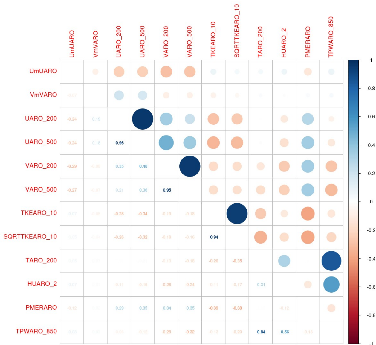
Illustration 8.39 : AO4 Barfleur – 200 M – Premier groupe (variables explicatives conservées pour la sélection finale) pour la prédiction de DD
