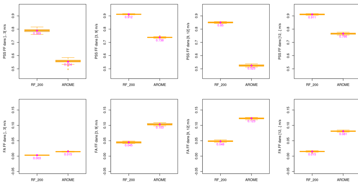
Illustration 3.12 : BNO – FF – Niveau 100 m – Modèle de forêt aléatoire à 200 arbres - Box-plot PSS (première ligne PSS FF \in ] , 3[ m/s , PSS FF \in [3, 9[ m/s , PSS FF \in [9, 12[ m/s et PSS FF \in [12, .[ m/s ) et FA (deuxième ligne FA FF \in ] , 3[ m/s , FA FF \in [3, 9[ m/s , FA FF \in [9, 12[ m/s et FA FF \in [12, .[ m/s ) pour l'échantillon d'apprentissage. La valeur en magenta sur chaque boîte à moustaches correspond à la moyenne des 20 échantillons.
