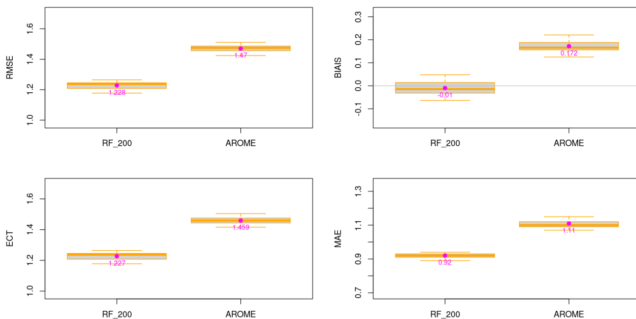
Illustration 3.13 : BNO – FF – Niveau 100 m – Modèle de forêt aléatoire - Box-plot RMSE, ECT, BIAIS et MAE pour l'échantillon de test. La valeur en magenta sur chaque boîte à moustaches correspond à la moyenne des 20 échantillons.
