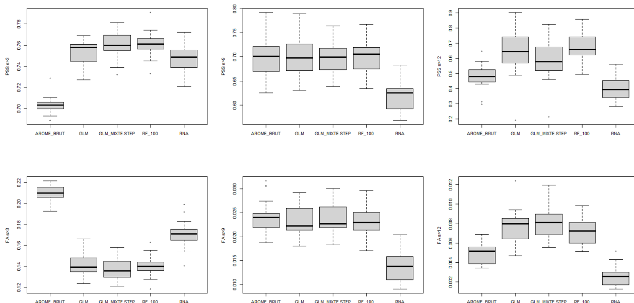
Illustration 7.32 : Station de test 1 – FF – Comparaison inter-modèles - Box-plot PSS (première ligne pss > 3 m/s, pss > 9 m/s et pss > 12 m/s) et FA (deuxième ligne fa > 3 m/s, fa > 9 m/s et fa > 12 m/s) pour l'échantillon de test
