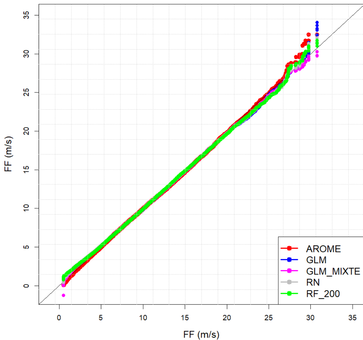
Illustration 8.28 : AO5 Bretagne Sud – 200 M – FF – QQ-Plot de FF pour les modèles GLM, GLM_MIXTE, RF_200, RNA et AROME
