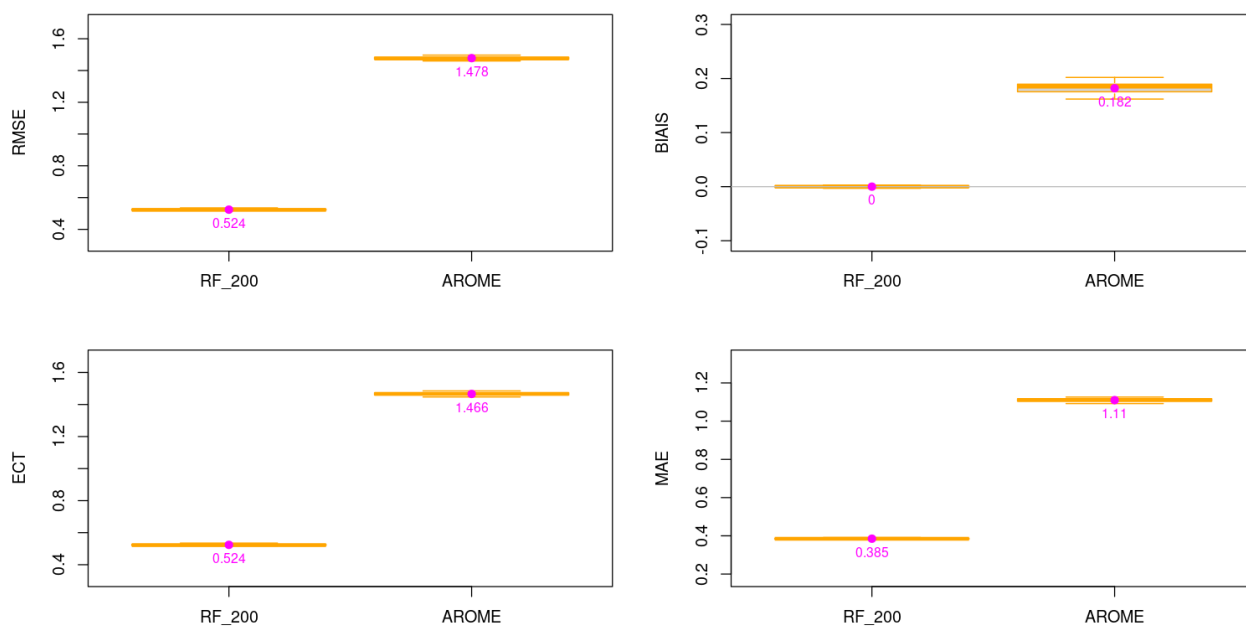
Illustration 3.11 : BNO – FF – Niveau 100 m – Modèle de forêt aléatoire à 200 arbres - Box-plot RMSE (haut gauche), ECT (bas gauche), BIAIS (haut droite) et MAE (bas droite) pour l'échantillon d'apprentissage. La valeur en magenta sur chaque boîte à moustaches correspond à la moyenne des 20 échantillons.
