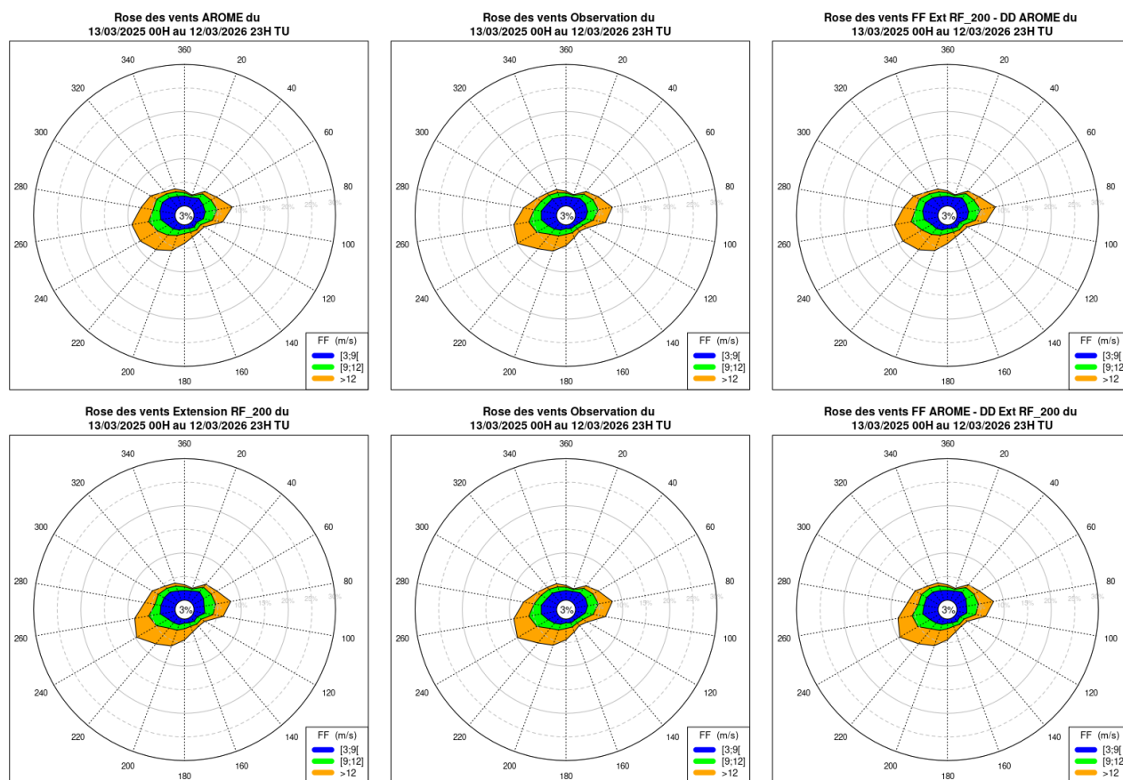
Illustration 4.9 : BNO – Roses des vents sur la période d'observation pour le niveau 200 m (du 13/03/2025 00H au 12/03/2026 23H) : sur la 1 re colonne (de haut en bas) on retrouve la rose AROME et celle de l'extension ; sur la 2 e colonne on retrouve la rose de l'observation. Les deux vignettes de cette colonne sont identiques et ont été dupliquées par soucis de lisibilité ; et sur la 3 e colonne (de haut en bas) on retrouve respectivement les roses issues de FF Extension et DD AROME, FF AROME et DD Extension
