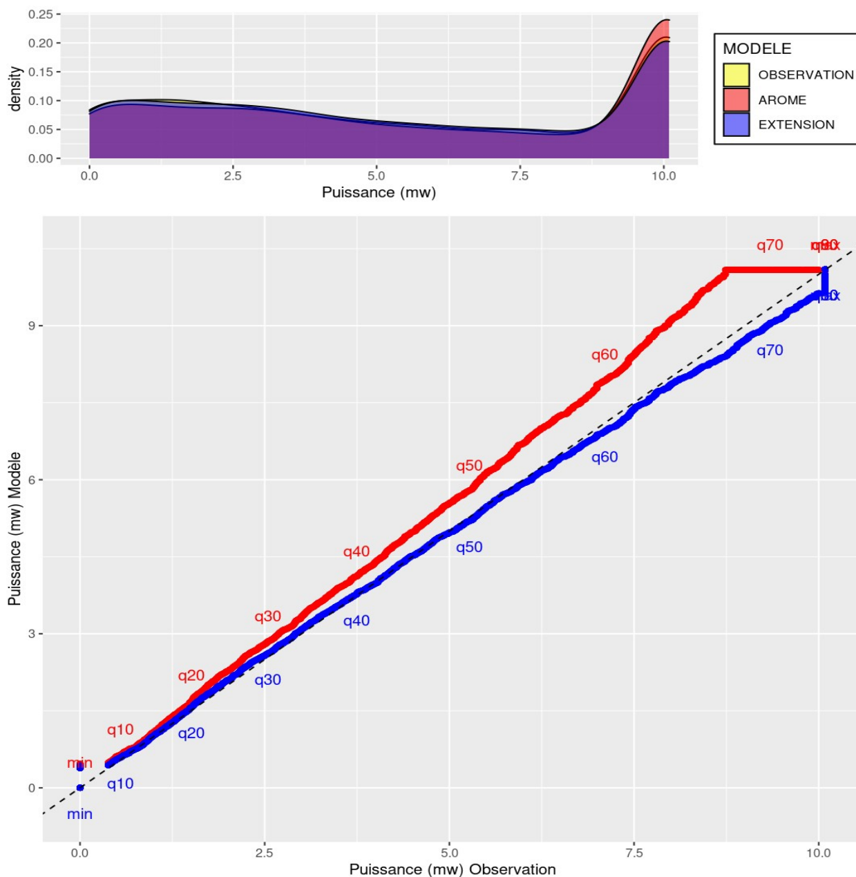
Illustration 4.16 : BNO – QQ-Plot des données de puissances de l'extension statistique (bleu) et AROME (rouge) sur la période d'observation pour le niveau 40 m.
