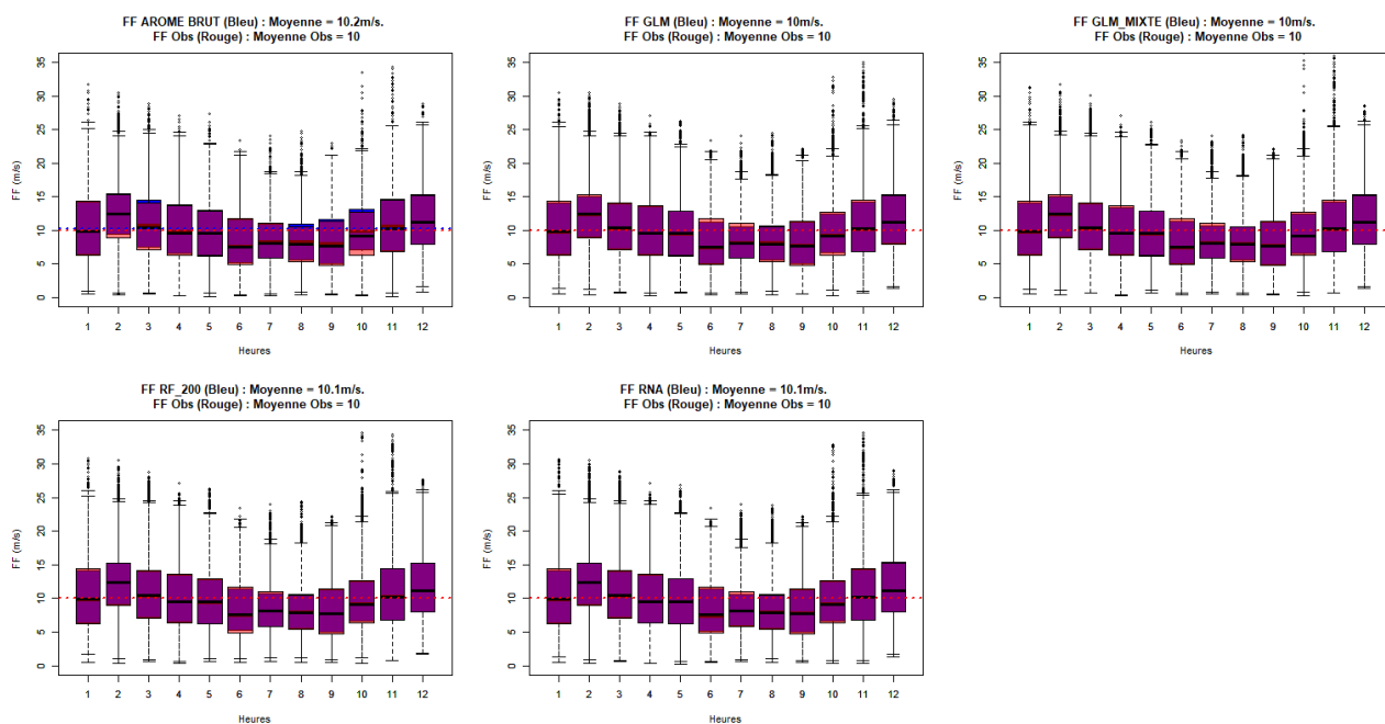
Illustration 8.31 : AO4 Barfleur – 200 M – FF – Cycle annuel des modèles statistiques (bleu) superposé aux observations (rouge)
