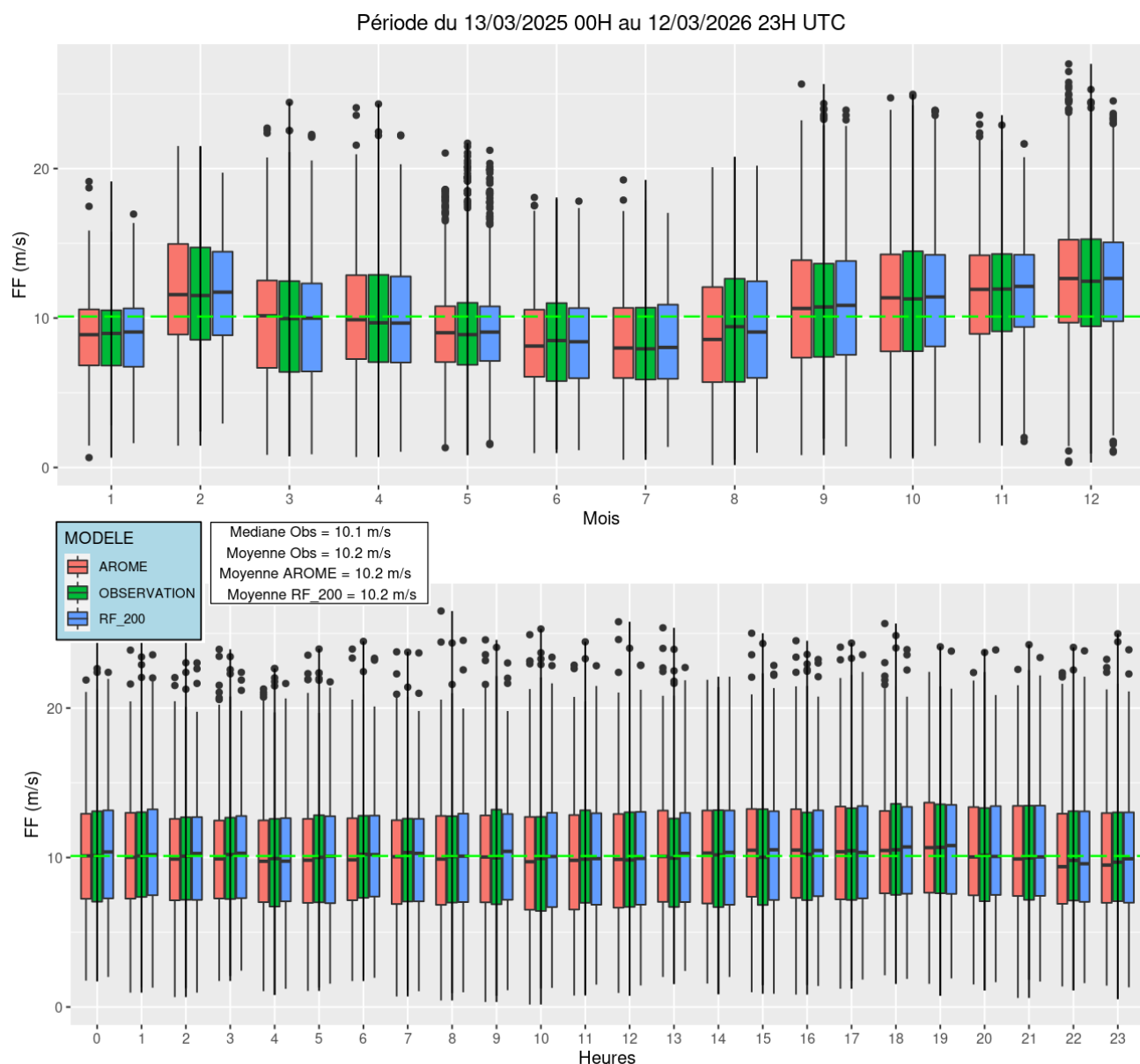
Illustration 4.3 : BNO – FF – Restitution des cycles de FF sur la période d'observation pour le niveau 200 m (du 13/03/2025 00H au 12/03/2026 23H). Sur la première ligne on retrouve le cycle annuel et sur la deuxième ligne le cycle diurne. La ligne discontinue verte traversant les boxplots désigne la médiane de l'observation sur la période d'observation.
