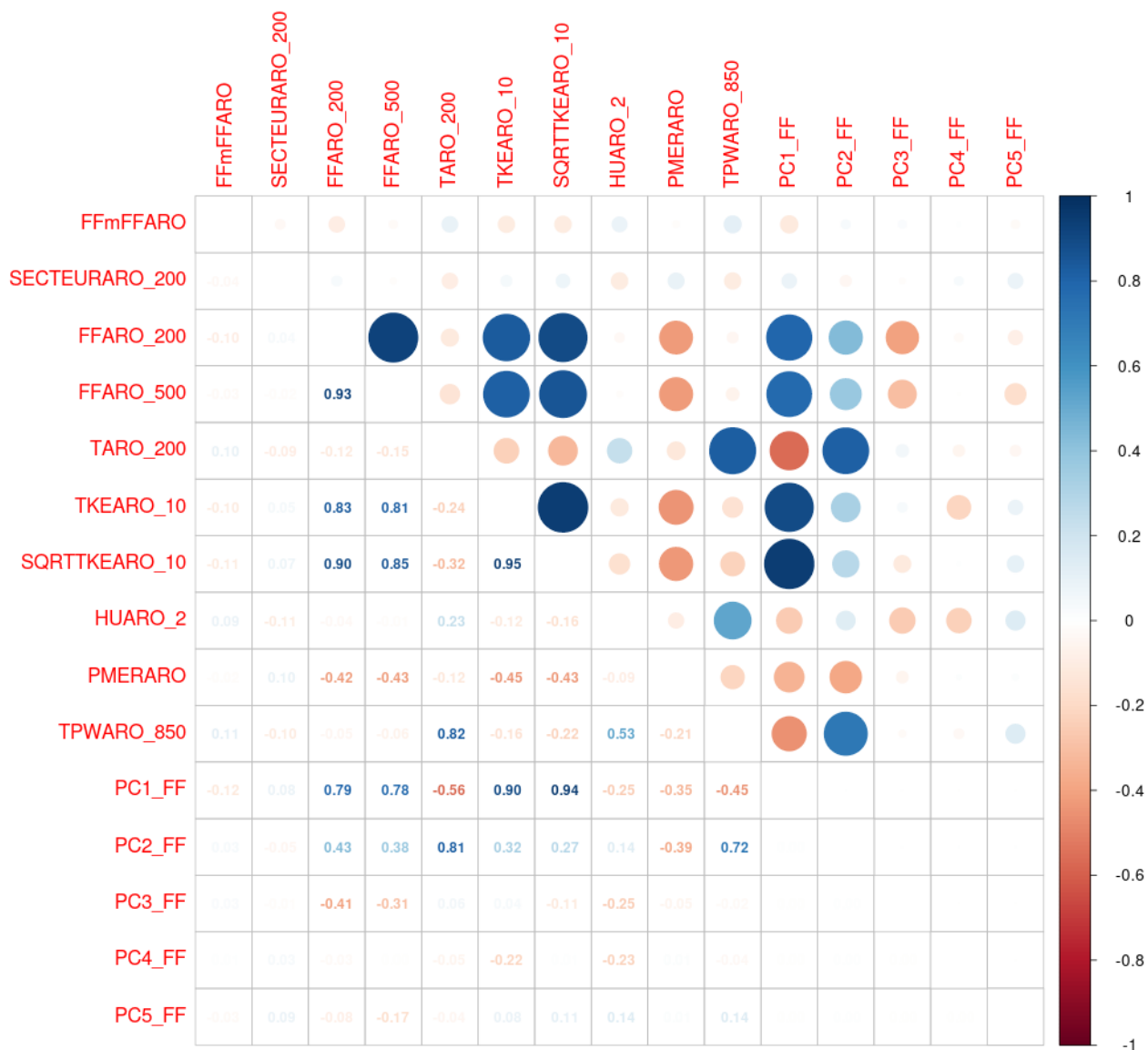
Illustration 8.12 : AO5 Bretagne Sud – 200 M – Variables explicatives finales (avec les composantes principales de l'ACP) pour la prédiction de FF
