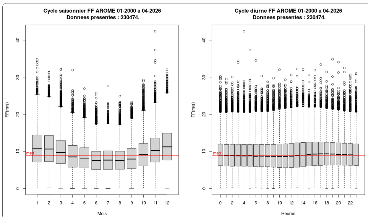
Illustration 3.5: BNO – FF – Niveau 100 m – Distribution du vent mensuelle (graphique de gauche) et horaire (graphique de droite) à partir des données climatologiques (AROME 01/2000 à 04/2026)
