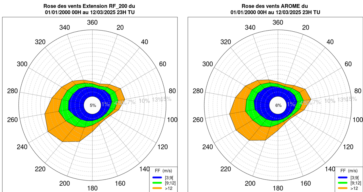
Illustration 4.24 : BNO – Roses des vents sur la période d'extension pour le niveau 200 m (du 01/01/2000 00H TU au 12/03/2025 23H TU). À gauche on retrouve la rose de l'extension statistique et à droite la rose d'AROME.
