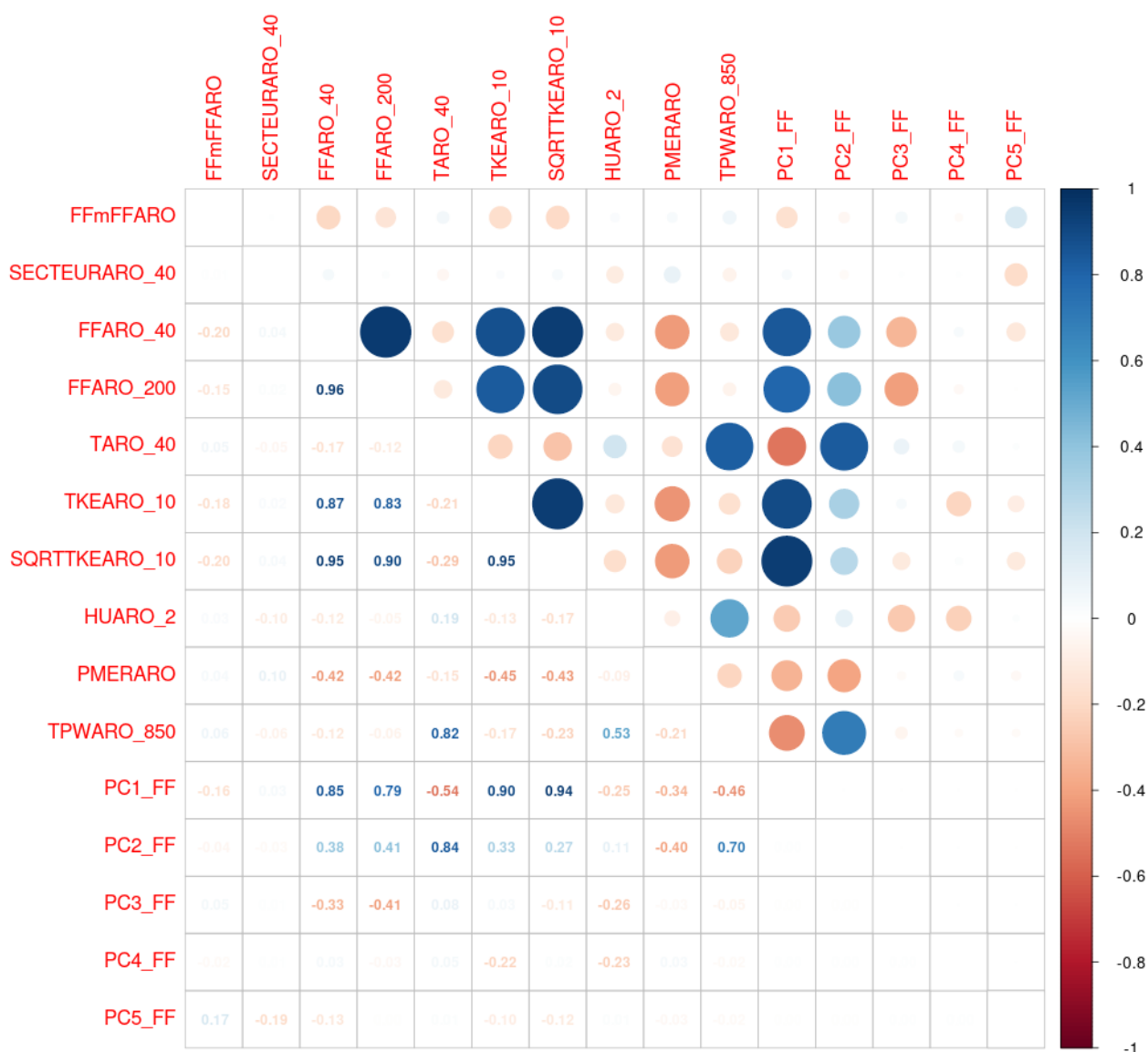
Illustration 8.6 : AO5 Bretagne Sud – 40 M – Variables explicatives finales (avec les composantes principales de l'ACP) pour la prédiction de FF
