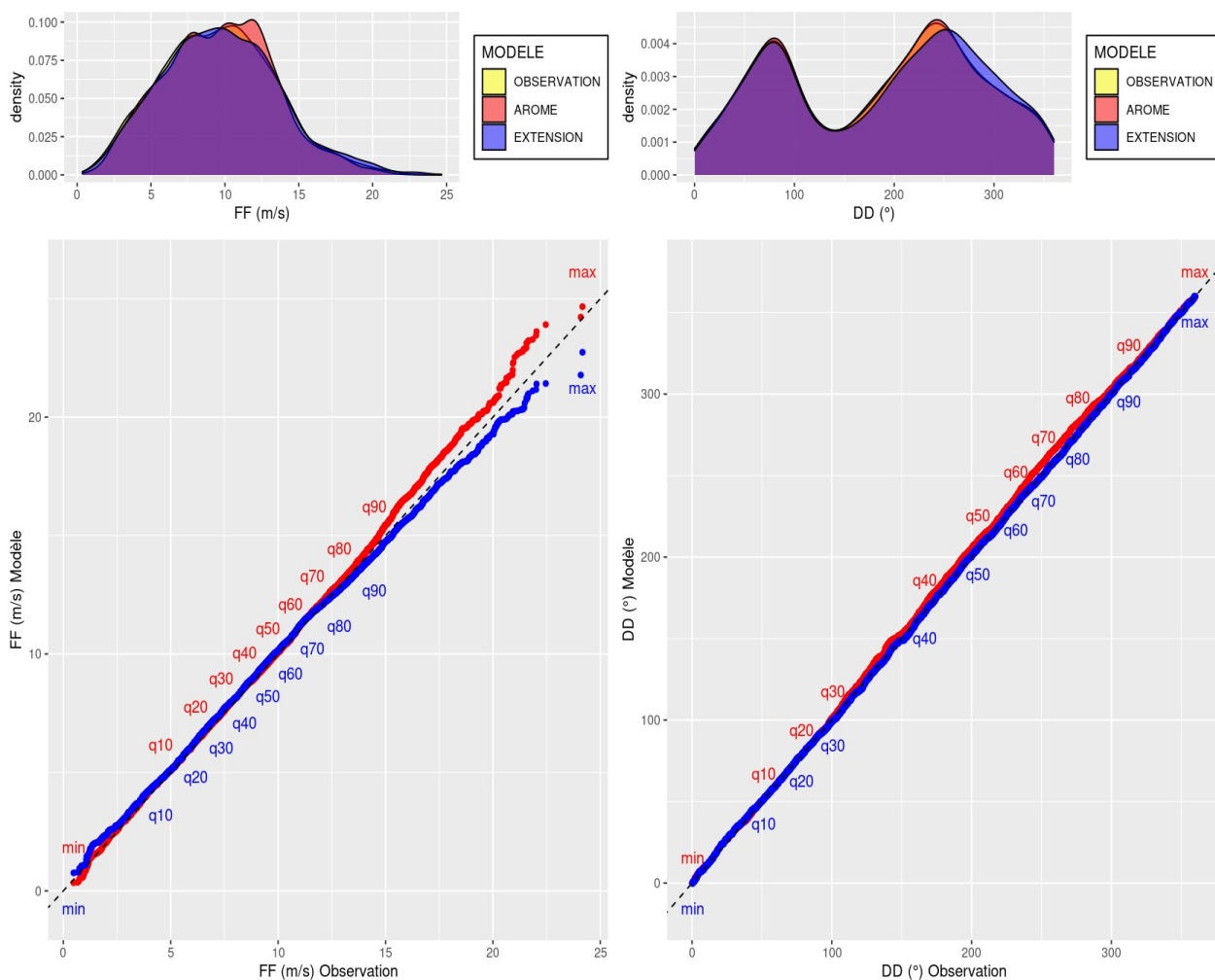
Illustration 4.8 : BNO – QQPlots FF et DD sur la période d'observation pour le niveau 100 m . En rouge : AROME, en bleu : extension statistique.
