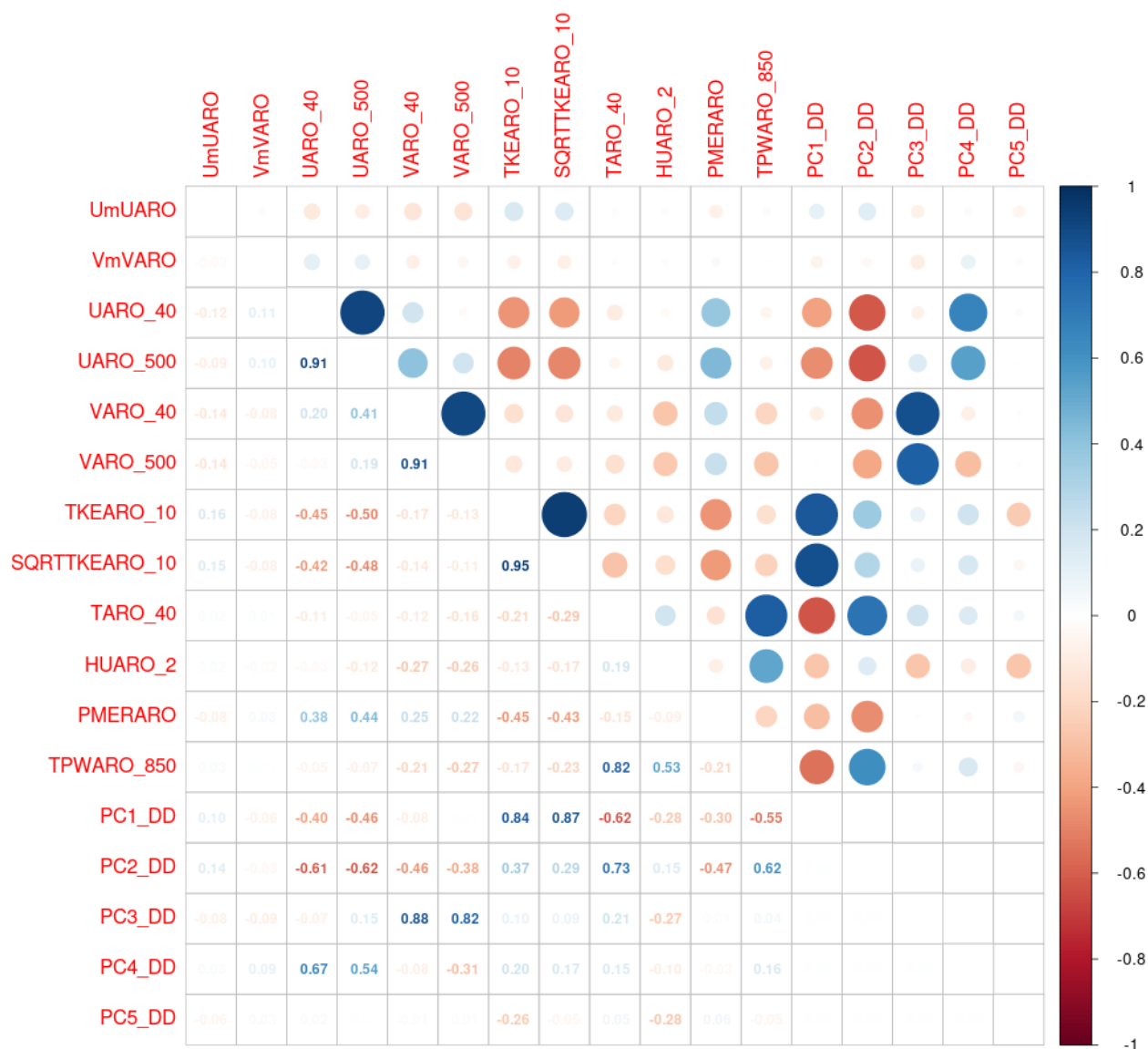
Illustration 8.38 : AO5 Bretagne Sud – 40 M – Variables explicatives finales (avec les composantes principales de l'ACP) pour la prédiction de DD
