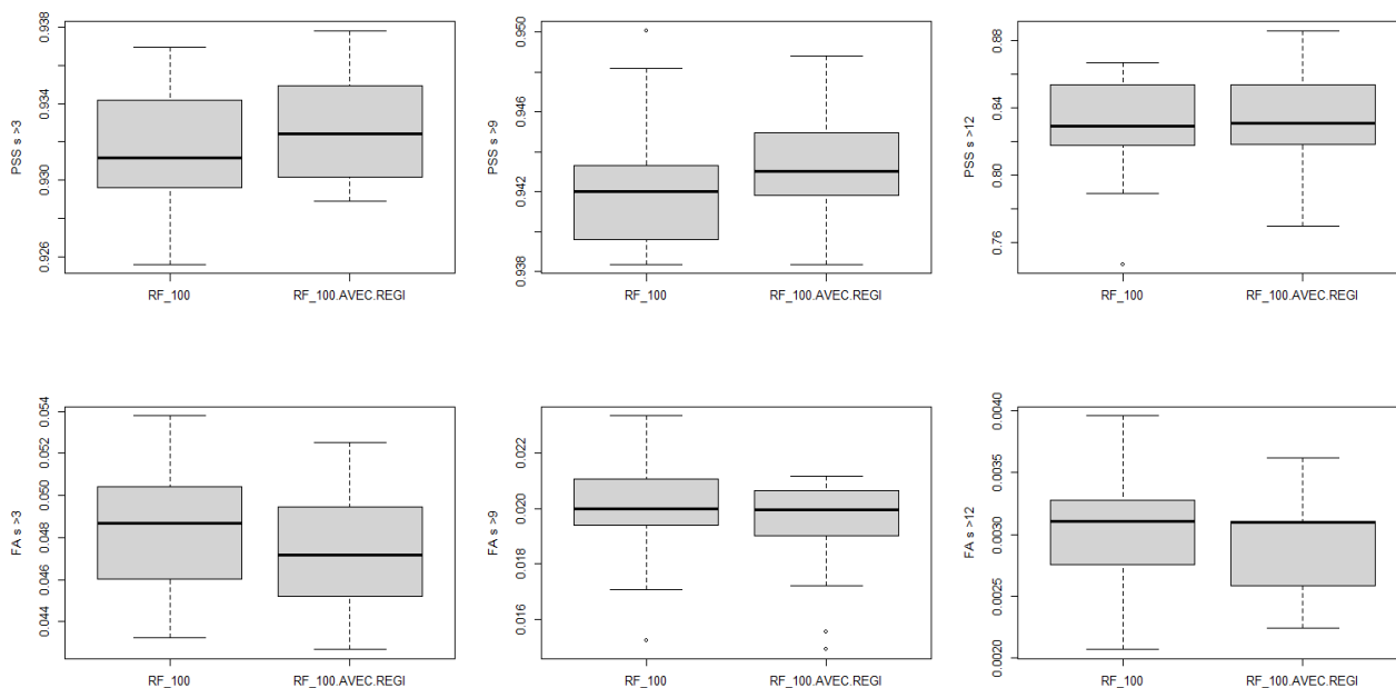
Illustration 7.37 : Station de test 2 – FF – Modèles de forêt aléatoire à 100 arbres avec et sans prédicteurs de régimes de temps - Box-plot PSS (première ligne pss > 3 m/s, pss > 9 m/s et pss > 12 m/s) et FA (deuxième ligne fa > 3 m/s, fa > 9 m/s et fa > 12 m/s) pour l'échantillon d'apprentissage
