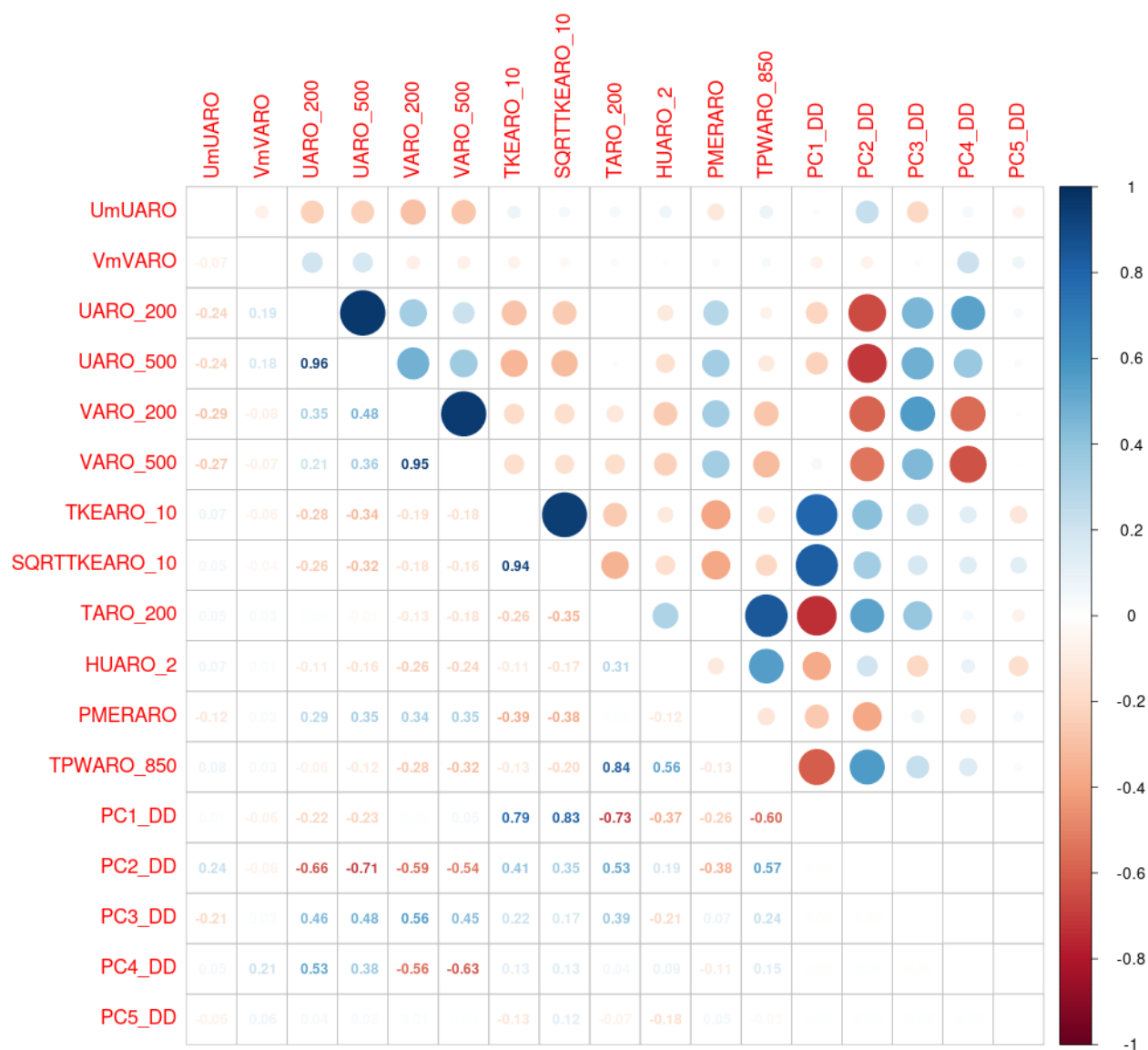
Illustration 8.43 : AO4 Barfleur – 200 M – Variables explicatives finales (avec les composantes principales de l'ACP) pour la prédiction de DD
