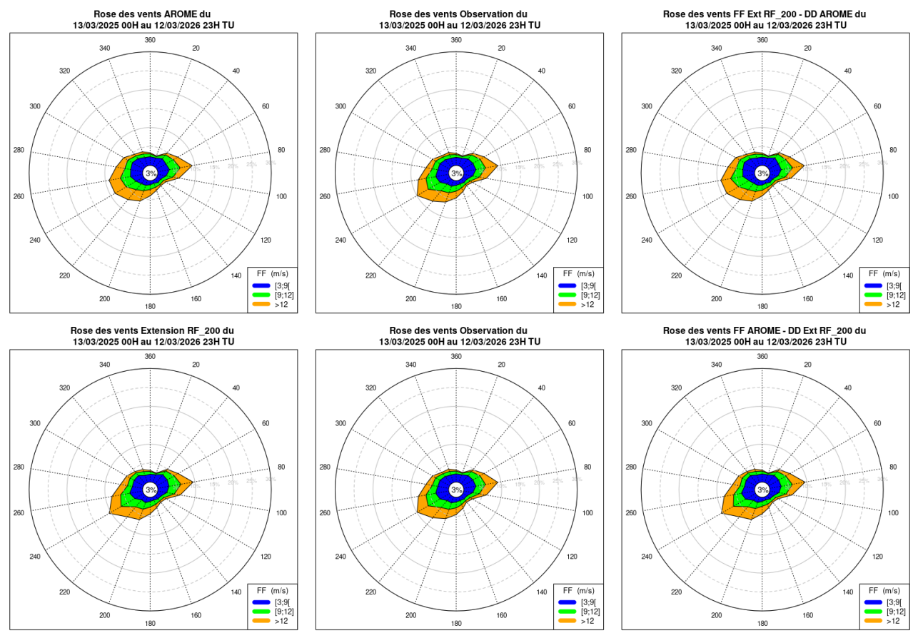
Illustration 4.7 : BNO – Roses des vents sur la période d'observation pour le niveau 100 m (du 13/03/2025 00H au 12/03/2026 23H) : sur la 1 re colonne (de haut en bas) on retrouve la rose AROME et celle de l'extension ; sur la 2 e colonne on retrouve la rose de l'observation. Les deux vignettes de cette colonne sont identiques et ont été dupliquées par soucis de lisibilité ; et sur la 3 e colonne (de haut en bas) on retrouve respectivement les roses issues de FF Extension et DD AROME, FF AROME et DD Extension
