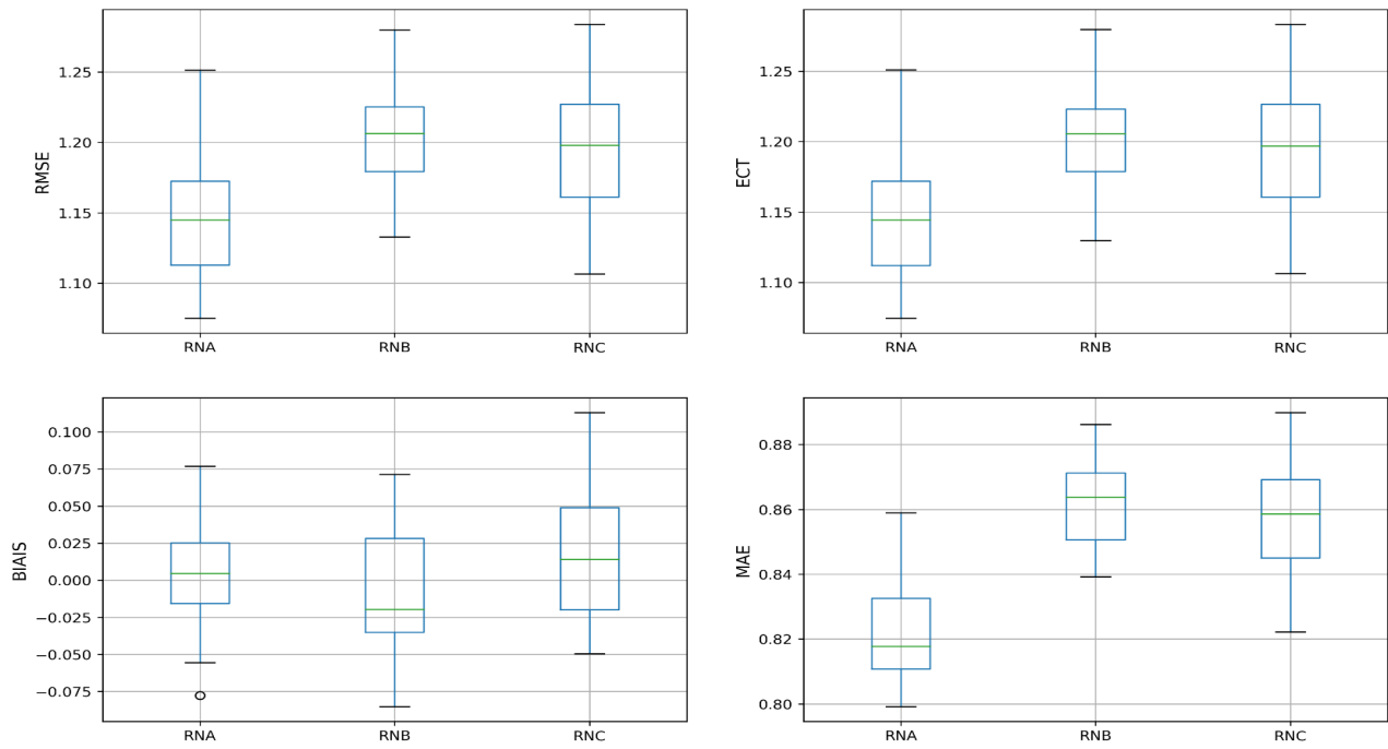
Illustration 7.43 : Station de test 1 – U – Réseau de neurones - Box-plot RMSE, ECT, BIAIS et MAE pour l'échantillon de test
