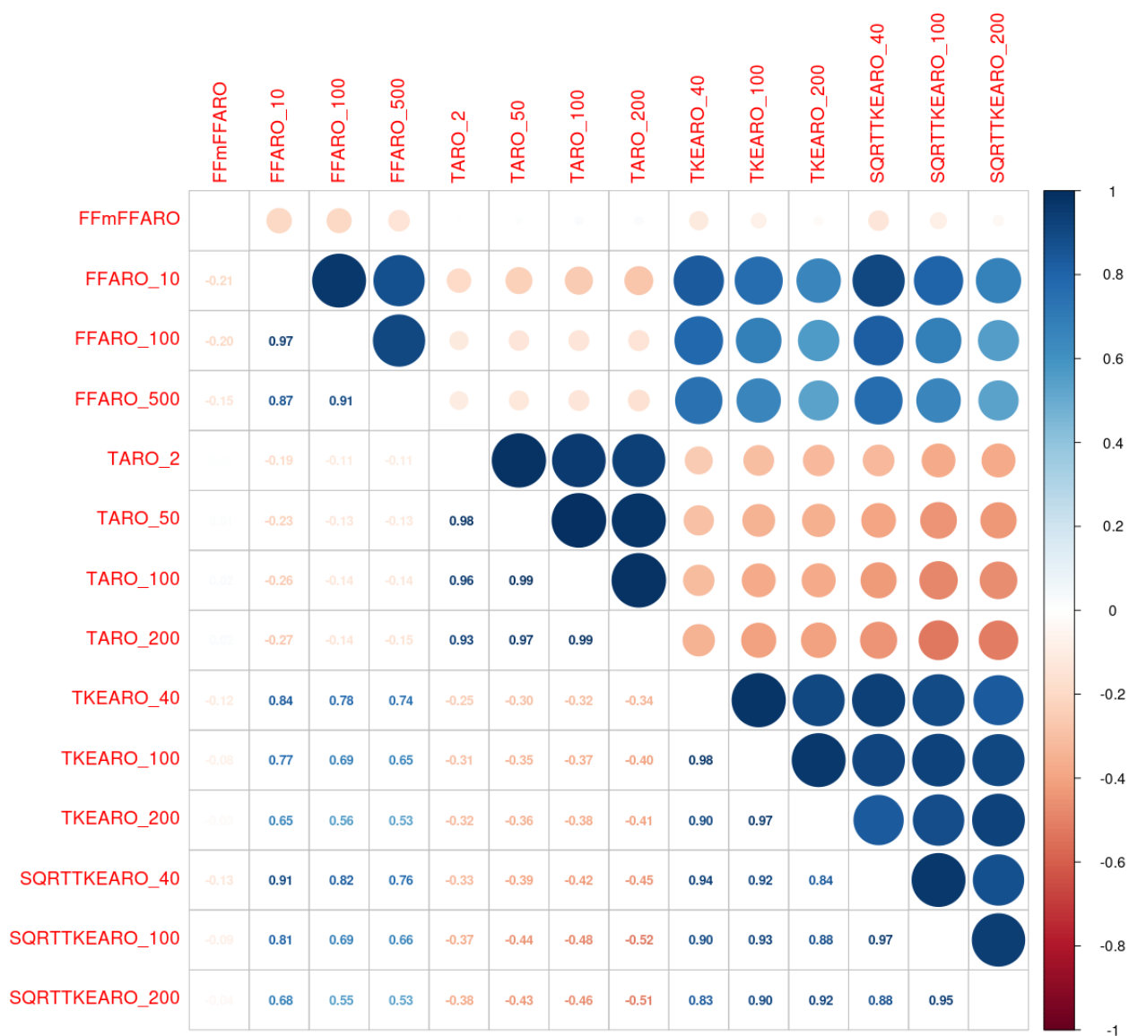
Illustration 8.3 : AO4 Barfleur – 40 M – Deuxième groupe (variables de l'ACP) pour la prédiction de FF
