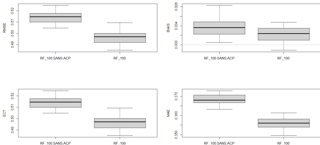
Illustration 7.19 : Station de test 1 – FF – Modèles de forêt aléatoire à 100 arbres avec et sans ACP - Box-plot RMSE (haut gauche), ECT (bas gauche), BIAIS (haut droite) et MAE (bas droite) pour l'échantillon d'apprentissage
