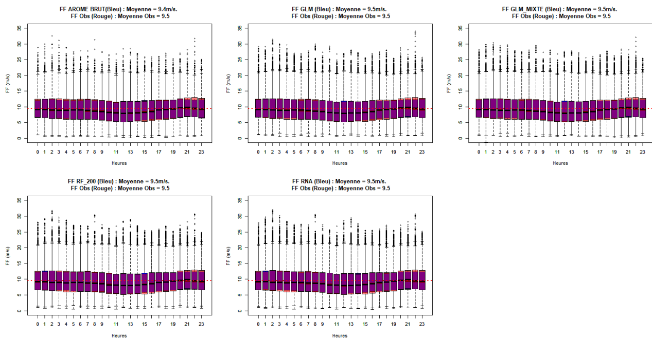
Illustration 8.30 : AO5 Bretagne Sud – 200 M – FF – Cycle diurne des modèles statistiques (bleu) superposé aux observations (rouge)
