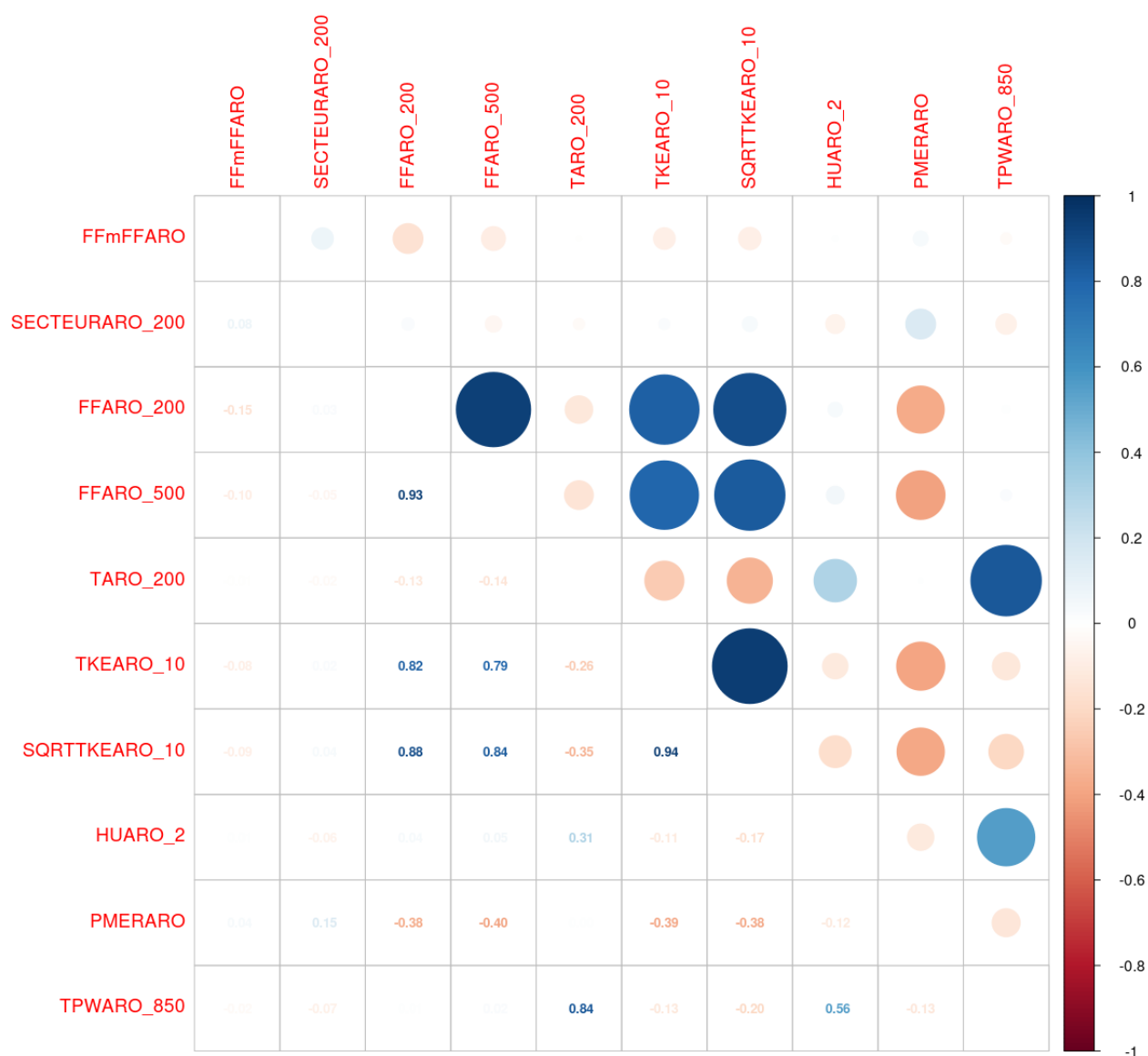
Illustration 8.7 : AO4 Barfleur – 200 M – Premier groupe (variables explicatives conservées pour la sélection finale) pour la prédiction de FF
