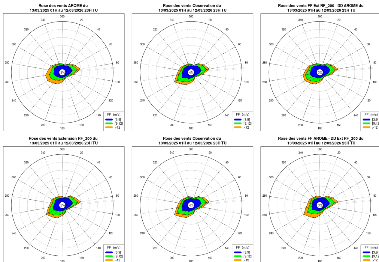
Illustration 4.11 : BNO – Roses des vents sur la période d'observation pour le niveau 40 m (du 13/03/2025 00H au 12/03/2026 23H) : sur la 1 re colonne (de haut en bas) on retrouve la rose AROME et celle de l'extension ; sur la 2 e colonne on retrouve la rose de l'observation. Les deux vignettes de cette colonne sont identiques et ont été dupliquées par soucis de lisibilité ; et sur la 3 e colonne (de haut en bas) on retrouve respectivement les roses issues de FF Extension et DD AROME, FF AROME et DD Extension
