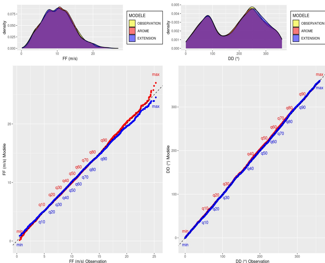
Illustration 4.10 : BNO – QQPlots FF et DD sur la période d'observation pour le niveau 200 m . En rouge : AROME, en bleu : extension statistique.
