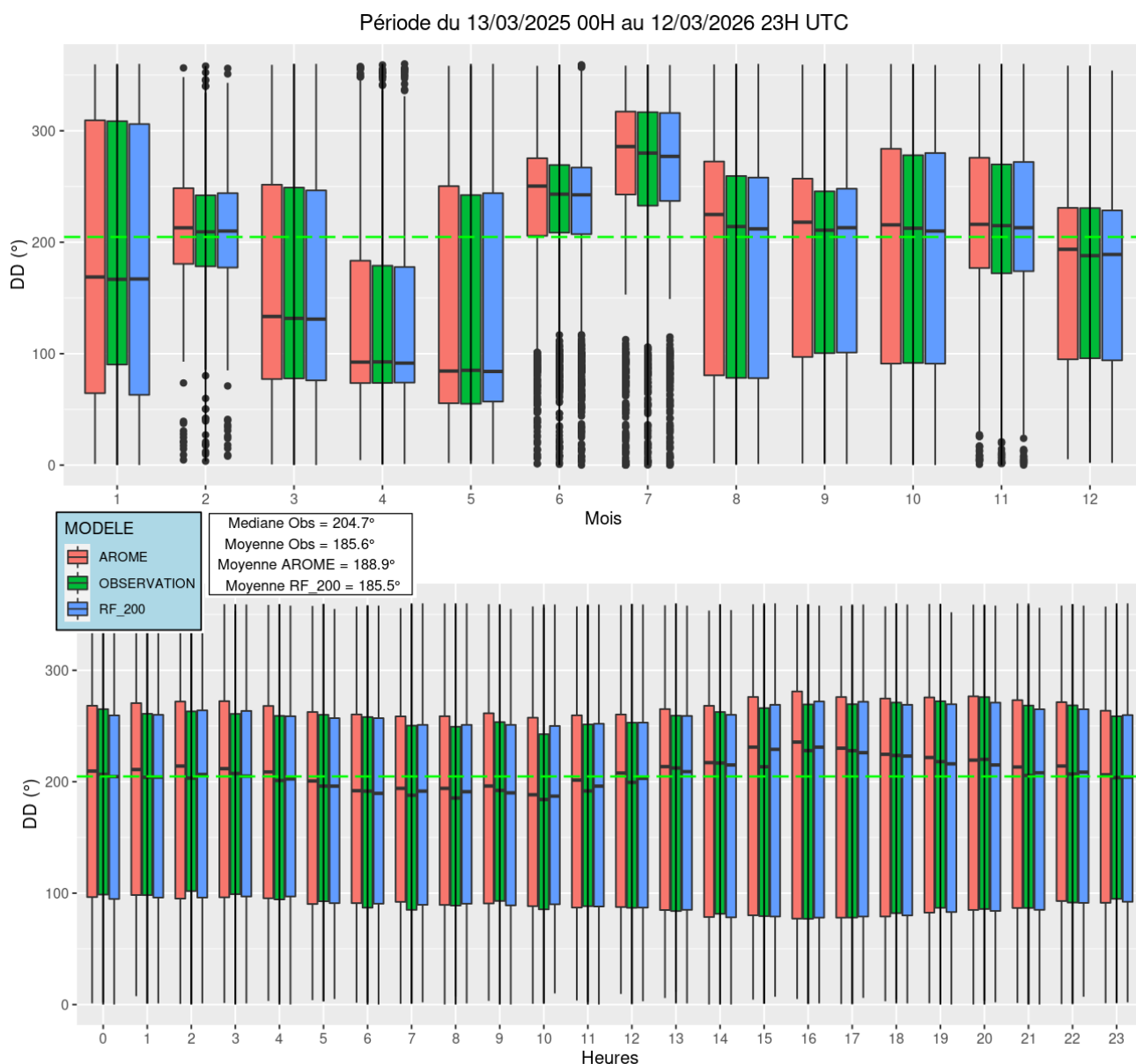
Illustration 4.2 : BNO – DD – Restitution des cycles de DD sur la période d'observation pour le niveau 100 m (du 13/03/2025 00H au 12/03/2026 23H). Sur la première ligne on retrouve le cycle annuel et sur la deuxième ligne le cycle diurne. La ligne discontinue verte traversant les boxplots désigne la médiane de l'observation sur la période d'observation.
