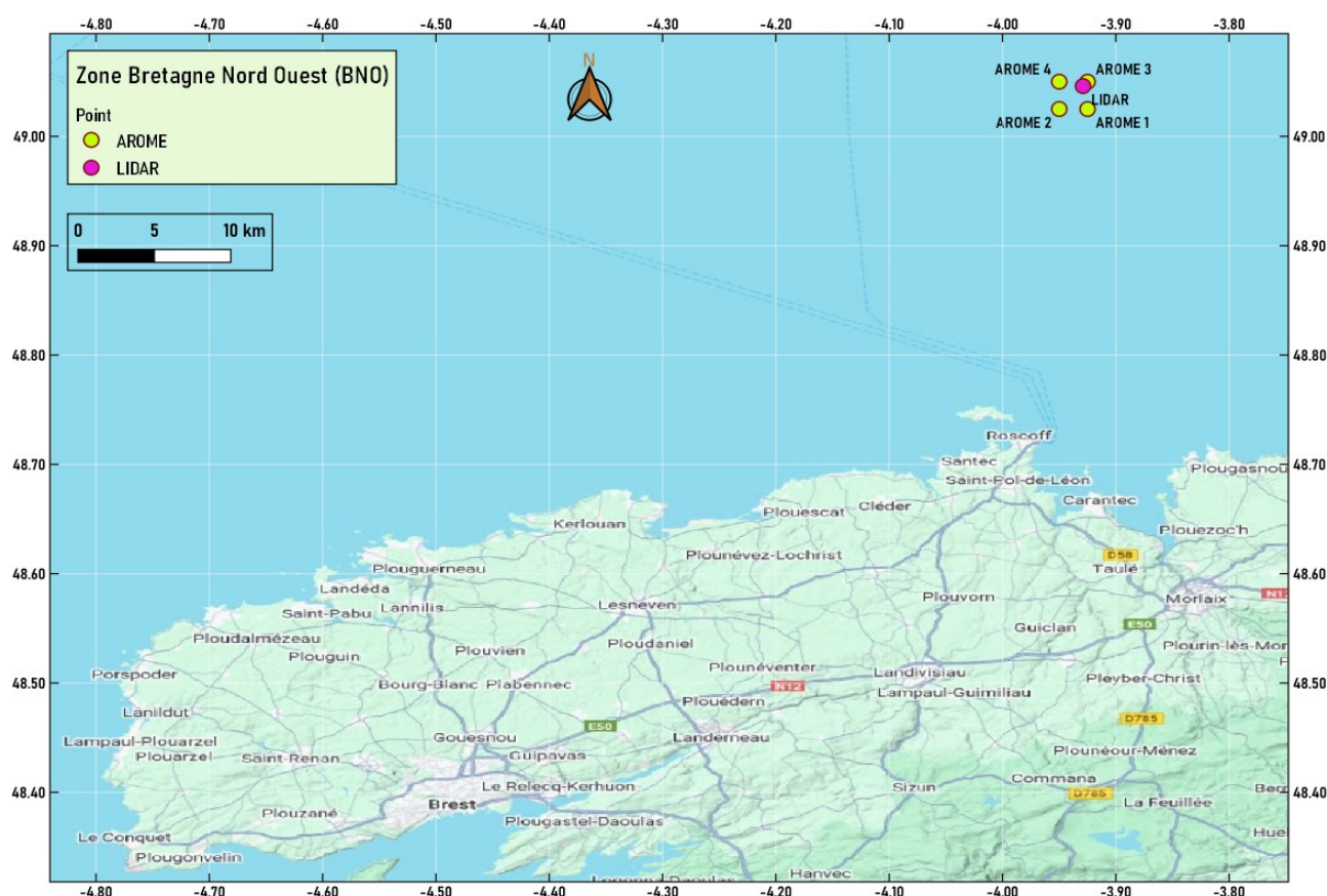
Illustration 3.2: Localisation du site de la zone BNO - Point d'observation LiDAR (en magenta) et points AROME (en jaune)
