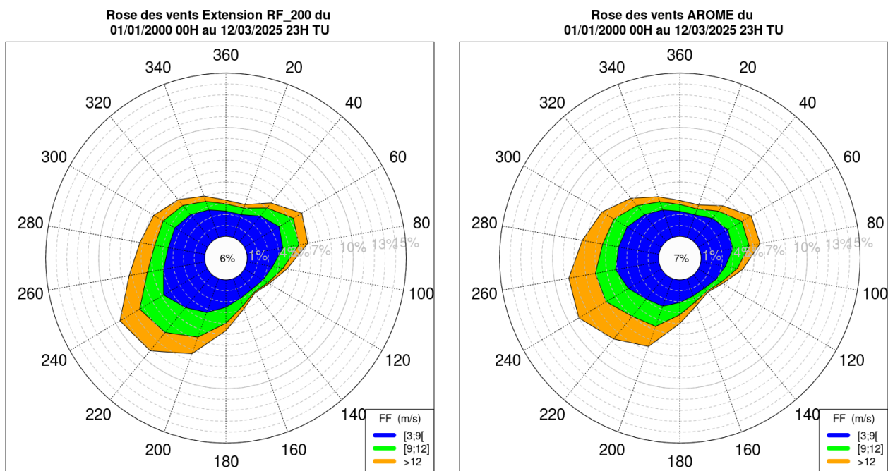
Illustration 4.25 : BNO – Roses des vents sur la période d'extension pour le niveau 40 m (du 01/01/2000 00H TU au 12/03/2025 23H TU). À gauche on retrouve la rose de l'extension statistique et à droite la rose d'AROME.
