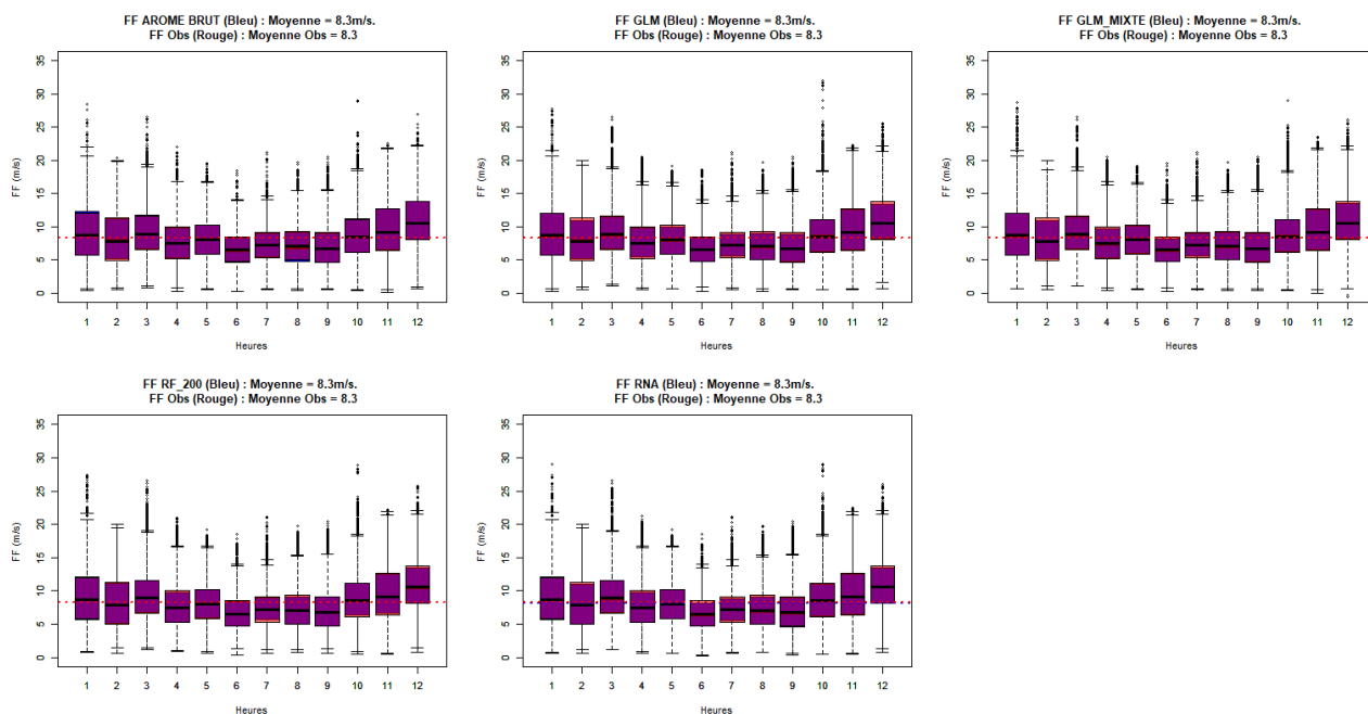
Illustration 8.22 : AO5 Bretagne Sud – 40 M – FF – Cycle annuel des modèles statistiques (bleu) superposé aux observations (rouge)
