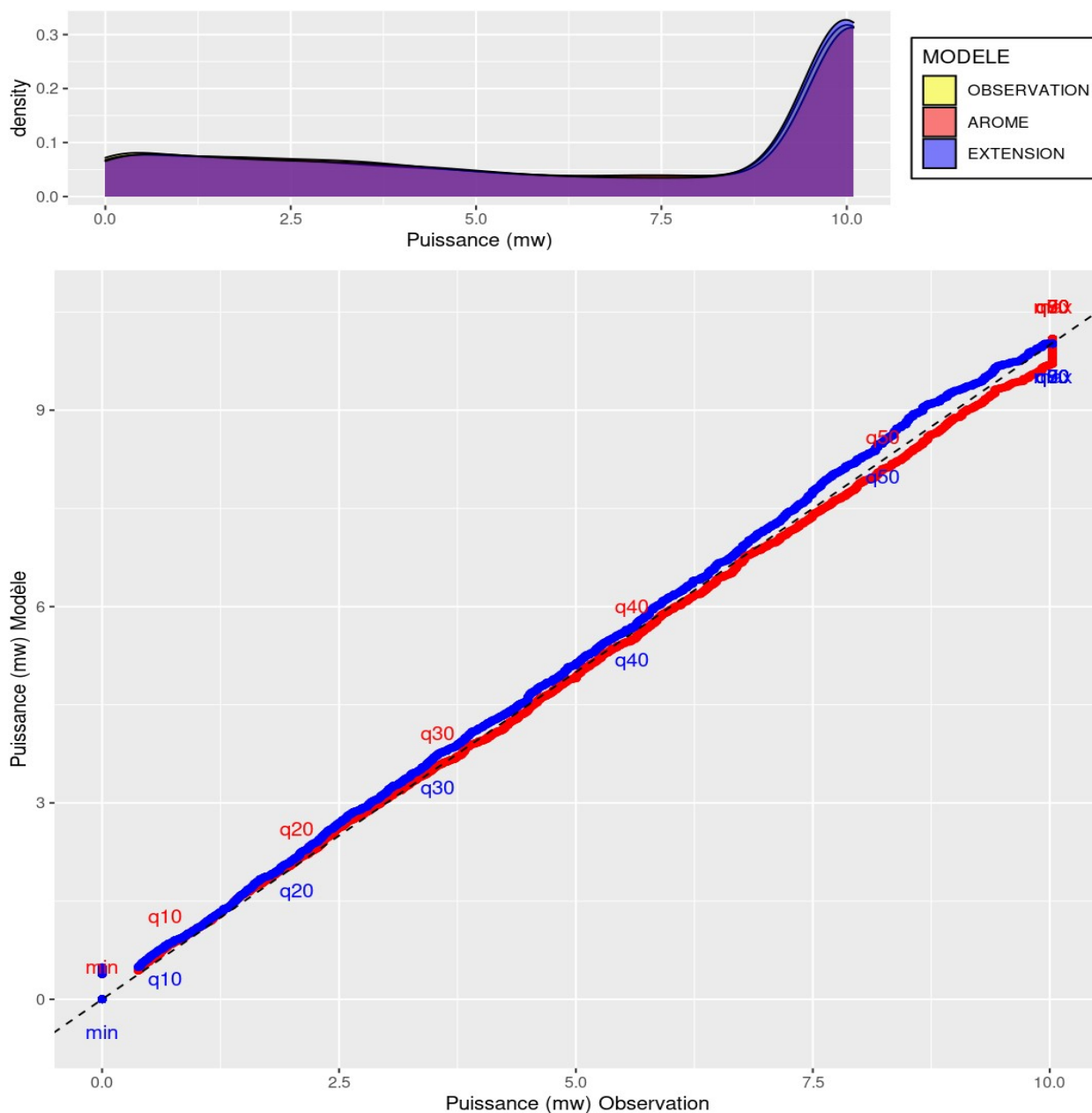
Illustration 4.14 : BNO – QQ-Plot des données de puissances de l'extension statistique (bleu) et AROME (rouge) sur la période d'observation pour le niveau 200 m.
