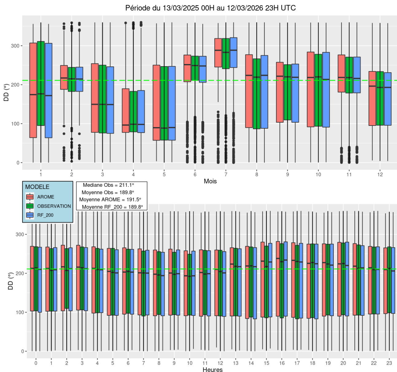
Illustration 4.4 : BNO – DD – Restitution des cycles de DD sur la période d'observation pour le niveau 200 m (du 13/03/2025 00H au 12/03/2026 23H). Sur la première ligne on retrouve le cycle annuel et sur la deuxième ligne le cycle diurne. La ligne discontinue verte traversant les boxplots désigne la médiane de l'observation sur la période d'observation.
