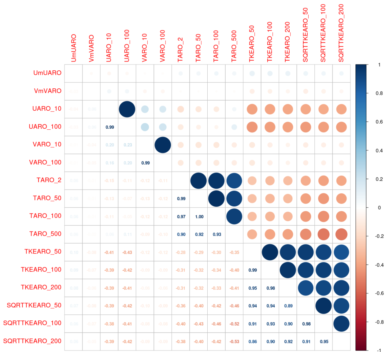
Illustration 8.42 : AO5 Bretagne Sud – 200 M – Deuxième groupe (variables de l'ACP) pour la prédiction de DD
