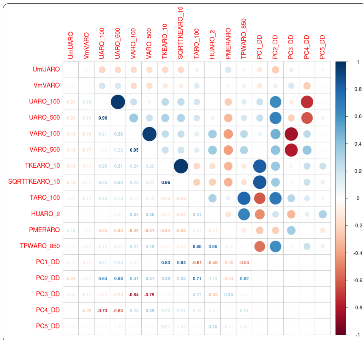
Illustration 3.6 : BNO – DD – Niveau 100 m – Corrélation entre les variables à expliquer UmUARO et VmVARO et les variables explicatives. En haut : sous forme de bulles. En bas : chiffré (0 : absence de corrélation, 1 ou -1 : forte corrélation).
