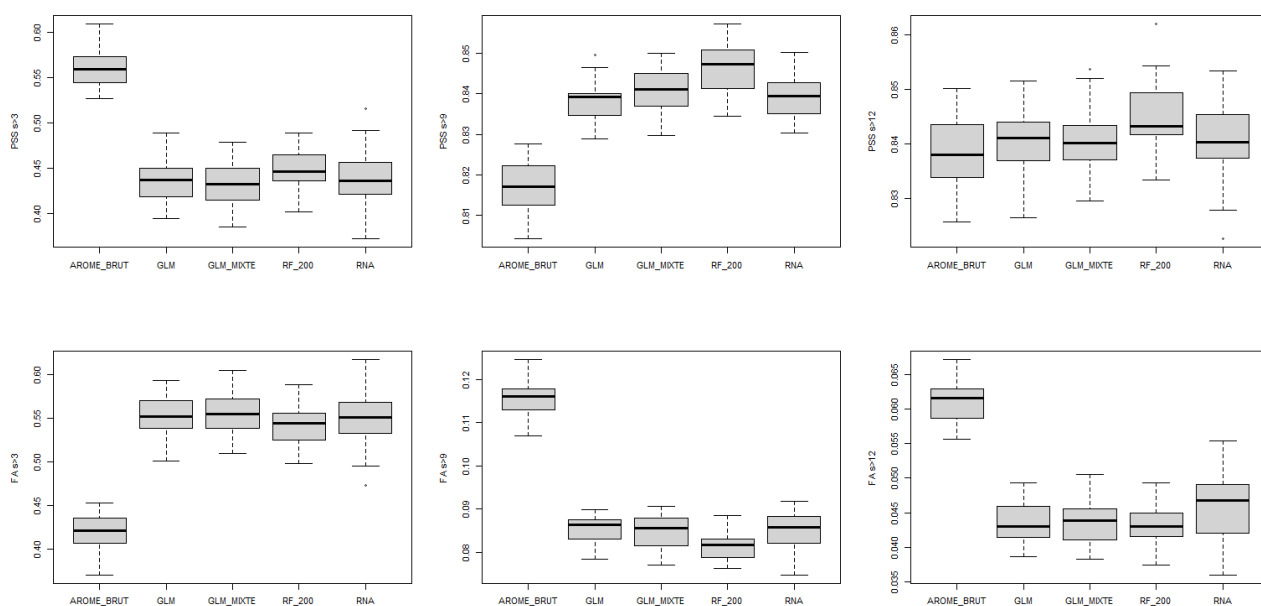
Illustration 8.25 : AO4 Barfleur – 200 M – FF – Comparaison inter-modèles - Box-plot PSS (première ligne pss FF > 3 m/s, pss FF > 9 m/s et pss FF > 12 m/s) et FA (deuxième ligne fa FF > 3 m/s, fa FF > 9 m/s et fa FF > 12 m/s) pour l'échantillon de test
