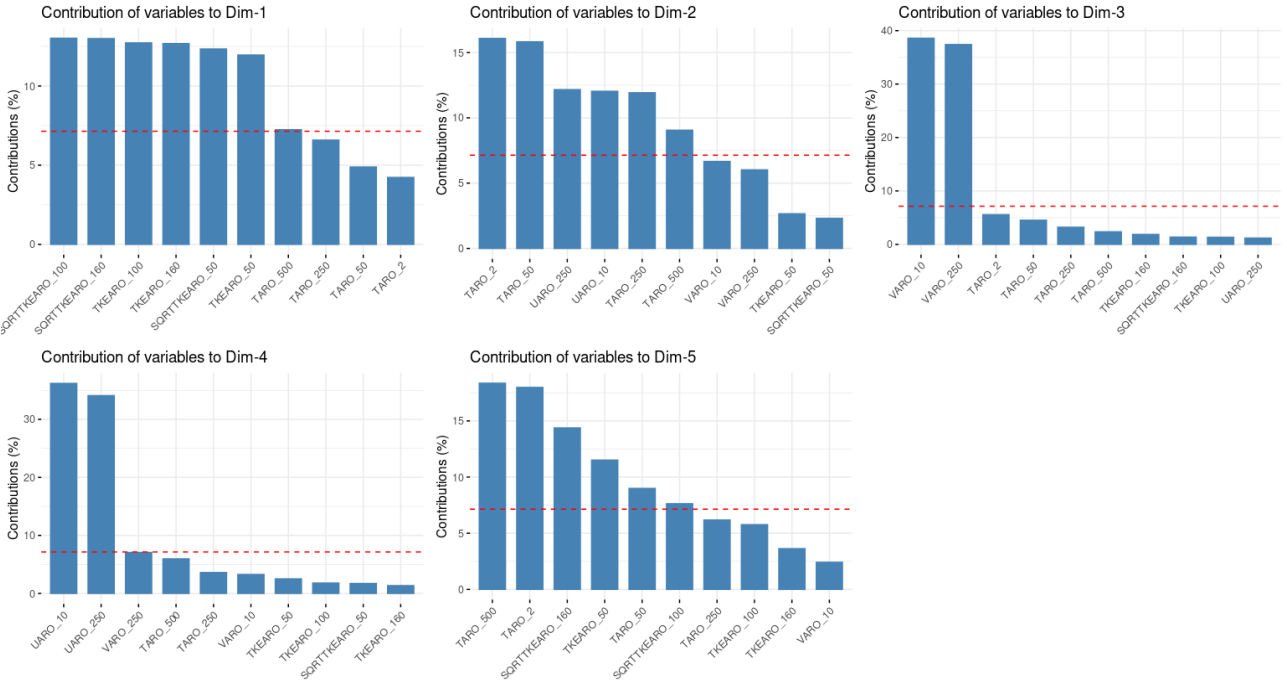
Illustration 3.25 : BNO – DD – Niveau 100 m – Contribution des variables à l'ACP (une figure pour chaque dimension)
