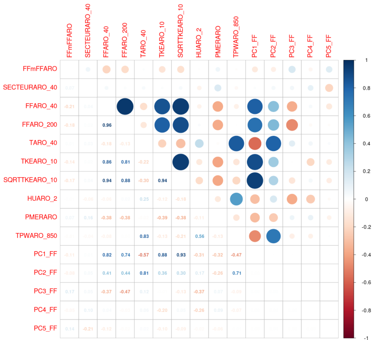
Illustration 8.5 : AO4 Barfleur – 40 M – Variables explicatives finales (avec les composantes principales de l'ACP) pour la prédiction de FF
