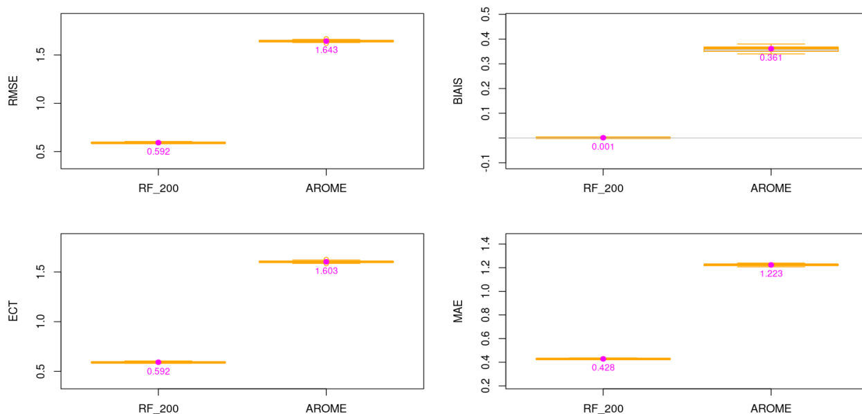
Illustration 3.17 : BNO – U – Niveau 100 m – Modèle de forêt aléatoire à 200 arbres - Box-plot RMSE (haut gauche), ECT (bas gauche), BIAIS (haut droite) et MAE (bas droite) pour l'échantillon d'apprentissage. La valeur en magenta sur chaque boîte à moustaches correspond à la moyenne des 20 échantillons.
