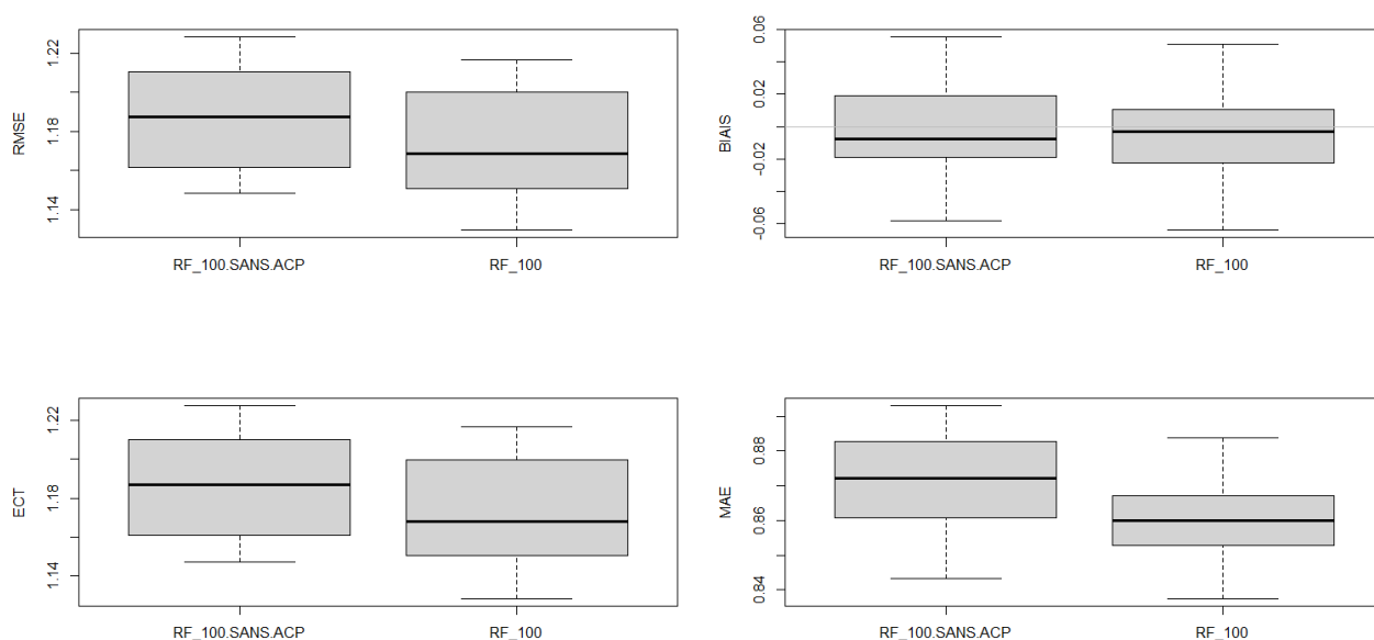
Illustration 7.21 : Station de test 1 – FF – Modèles de forêt aléatoire à 100 arbres avec et sans ACP - Box-plot RMSE (haut gauche), ECT (bas gauche), BIAIS (haut droite) et MAE (bas droite) pour l'échantillon de test
