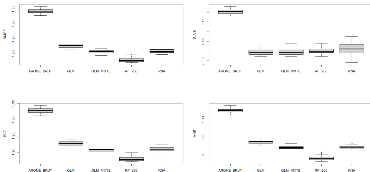
Illustration 8.13 : AO4 Barfleur – 40 M – FF – Comparaison inter-modèles - Box-plot RMSE (haut gauche), ECT (bas gauche), BIAIS (haut droite) et MAE (bas droite) pour l'échantillon de test
