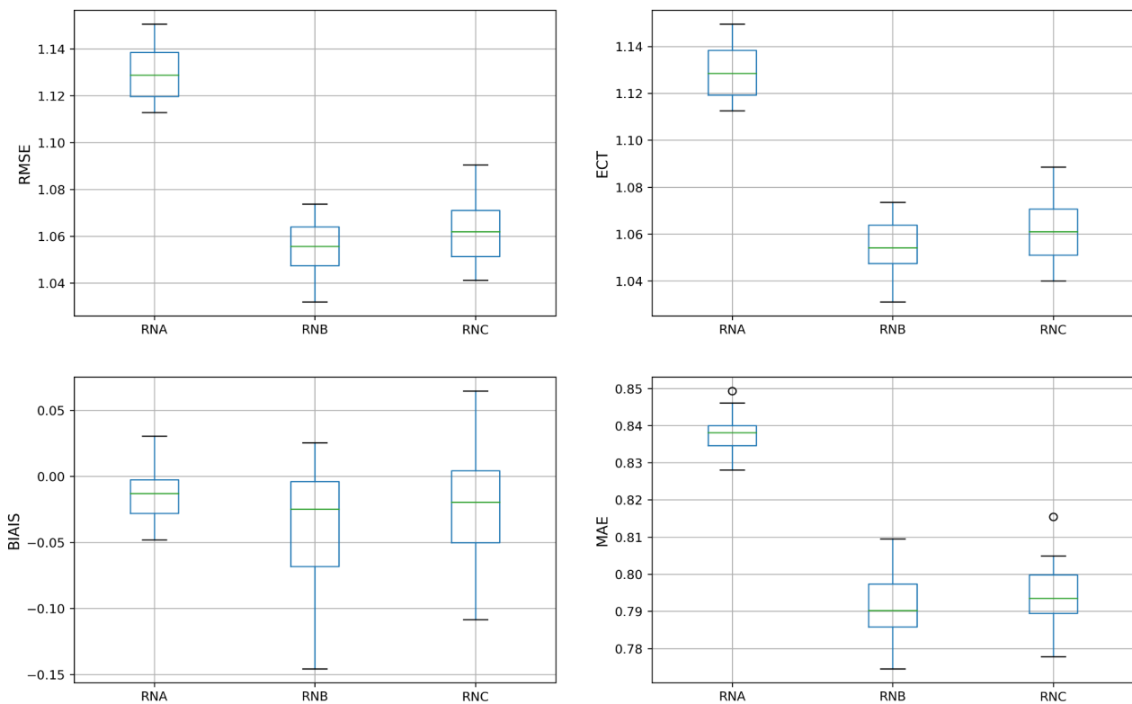
Illustration 7.27 : Station de test 1 – FF – Réseau de neurones - Box-plot RMSE, ECT, BIAIS et MAE pour l'échantillon d'apprentissage
