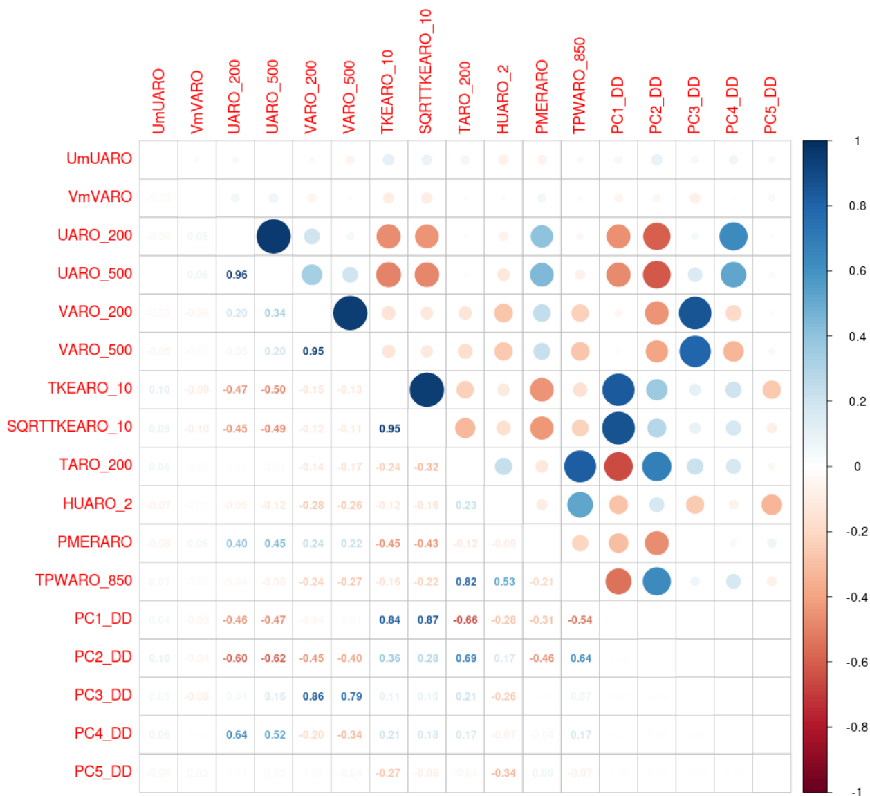
Illustration 8.44 : AO5 Bretagne Sud – 200 M – Variables explicatives finales (avec les composantes principales de l'ACP) pour la prédiction de DD
