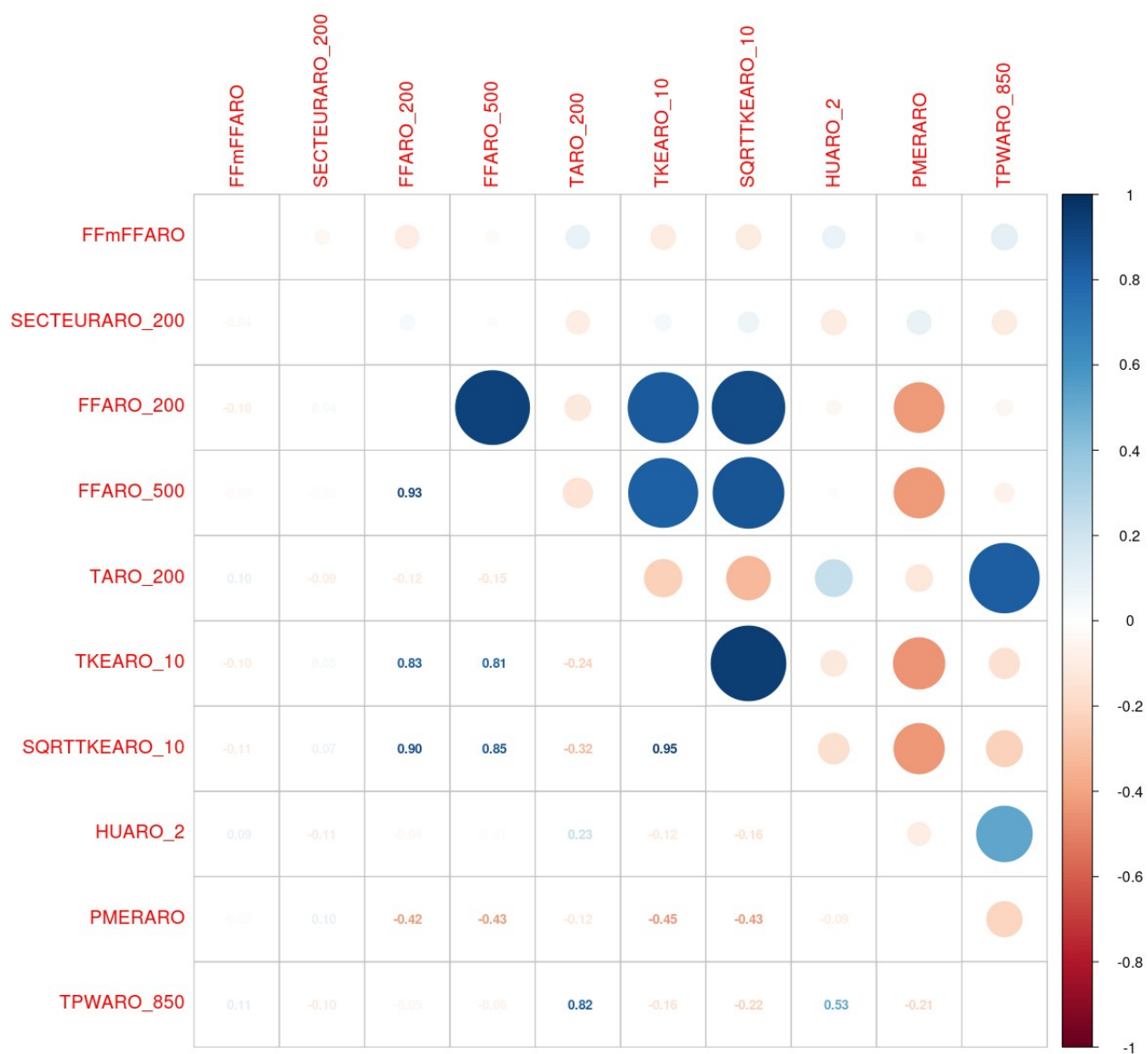
Illustration 8.8 : AO5 Bretagne Sud – 200 M – Premier groupe (variables explicatives conservées pour la sélection finale) pour la prédiction de FF
