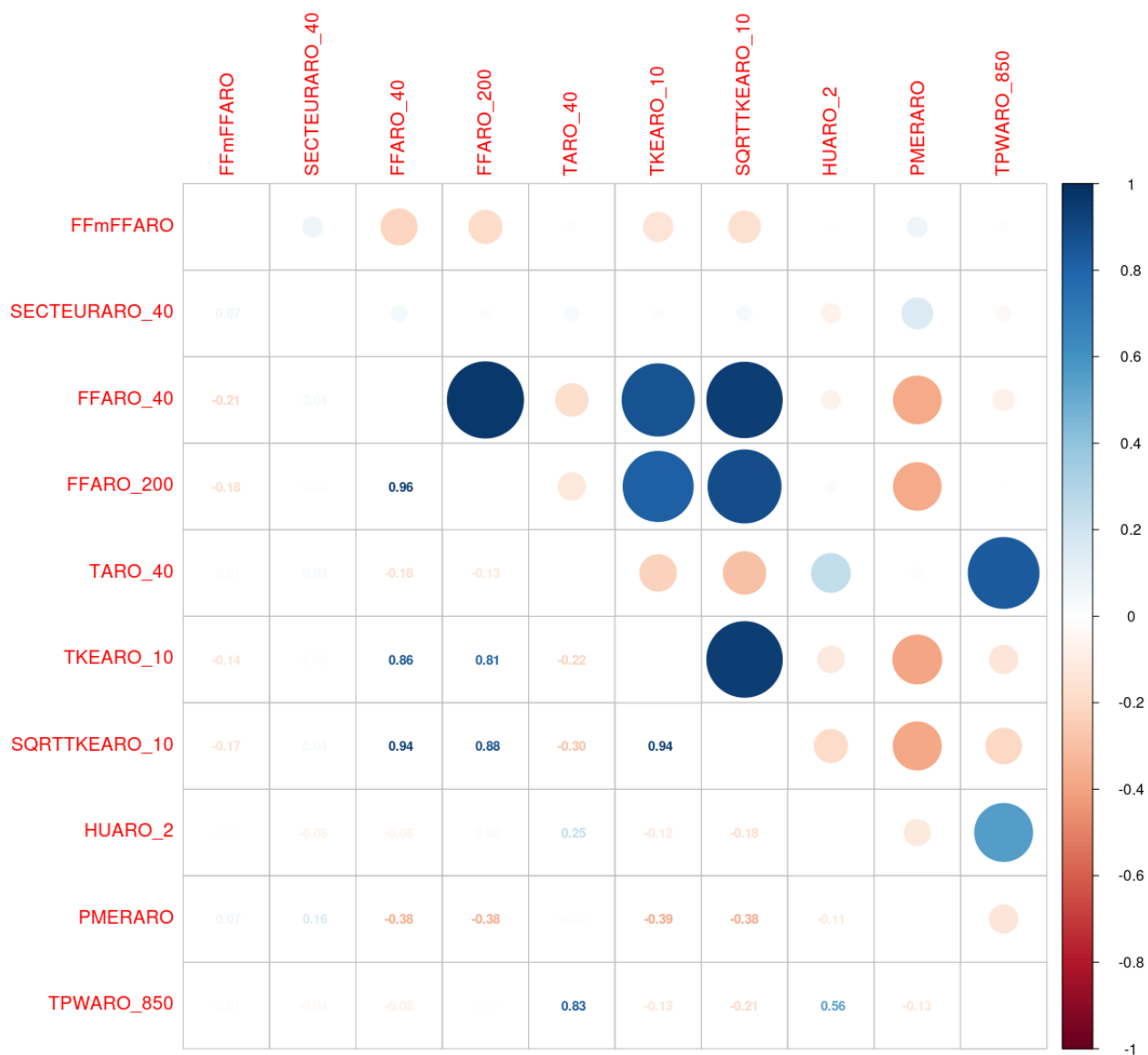
Illustration 8.1 : AO4 Barfleur – 40 M – Premier groupe (variables explicatives conservées pour la sélection finale) pour la prédiction de FF
