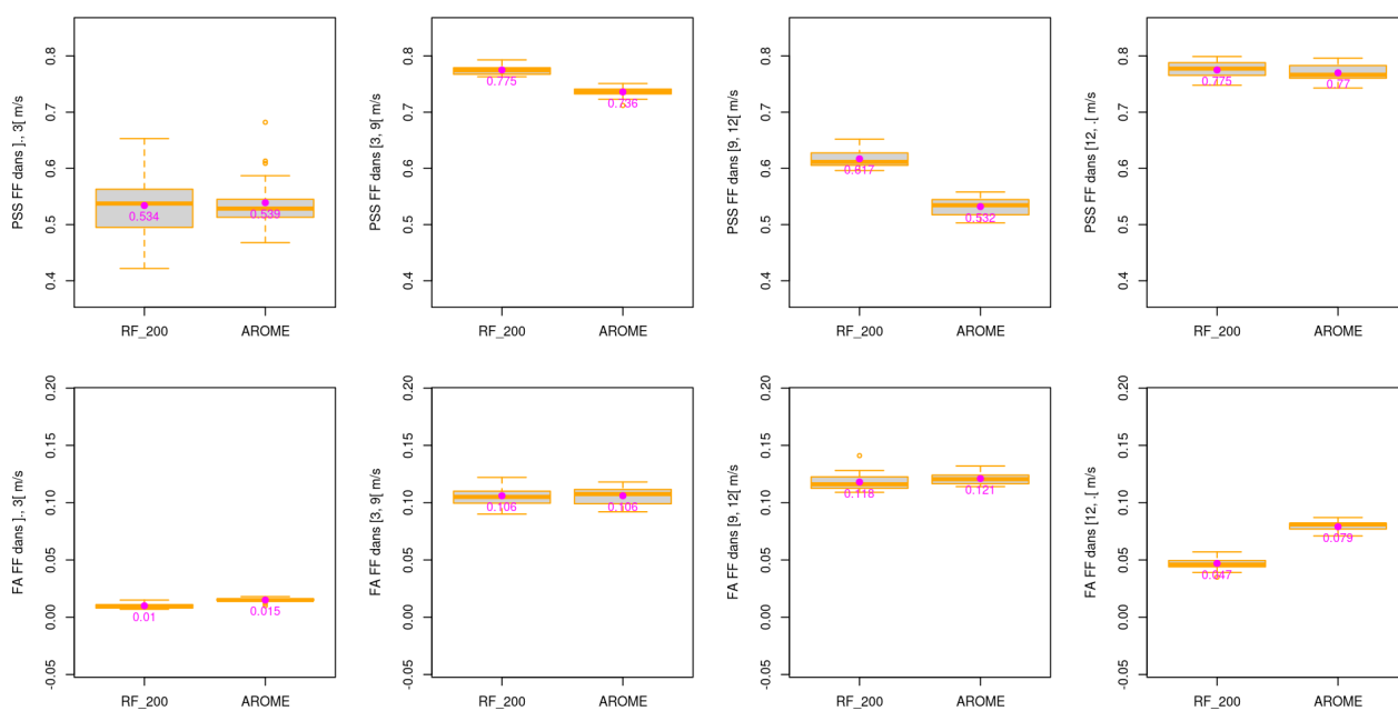
Illustration 3.14 : BNO – FF – Niveau 100 m – Modèle de forêt aléatoire - Box-plot PSS et FA pour l'échantillon de test. La valeur en magenta sur chaque boîte à moustaches correspond à la moyenne des 20 échantillons.
