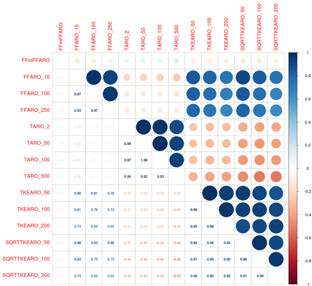
Illustration 8.10 : AO5 Bretagne Sud – 200 M – Deuxième groupe (variables de l'ACP) pour la prédiction de FF
