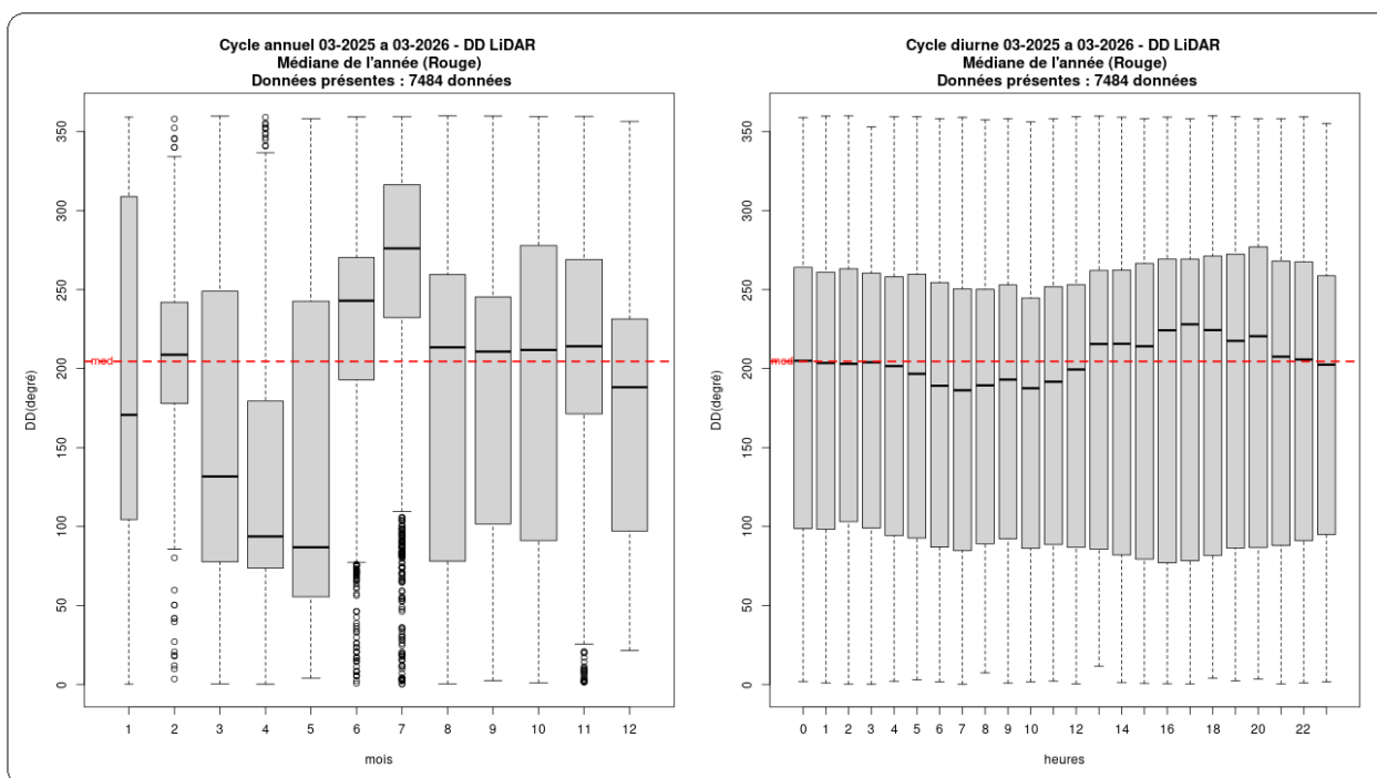
Illustration 3.7 : BNO – DD – Niveau 100 m – Distribution du vent mensuelle (graphique de gauche) et horaire (graphique de droite) à partir des données observées
