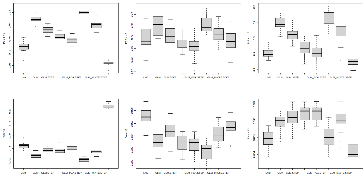
Illustration 7.12 : Station de test 1 – FF – Modèles linéaires et AROME.BRUT - Box-plot PSS (première ligne pss > 3 m/s, pss > 9 m/s et pss > 12 m/s noté respectivement pss1, pss2 et pss3) et FA (deuxième ligne fa > 3 m/s, fa > 9 m/s et fa > 12 m/s notée respectivement fa1, fa2 et fa3) pour l'échantillon d'apprentissage
