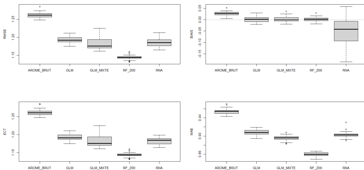
Illustration 8.14 : AO5 Bretagne Sud – 40 M – FF – Comparaison inter-modèles - Box-plot RMSE (haut gauche), ECT (bas gauche), BIAIS (haut droite) et MAE (bas droite) pour l'échantillon de test
