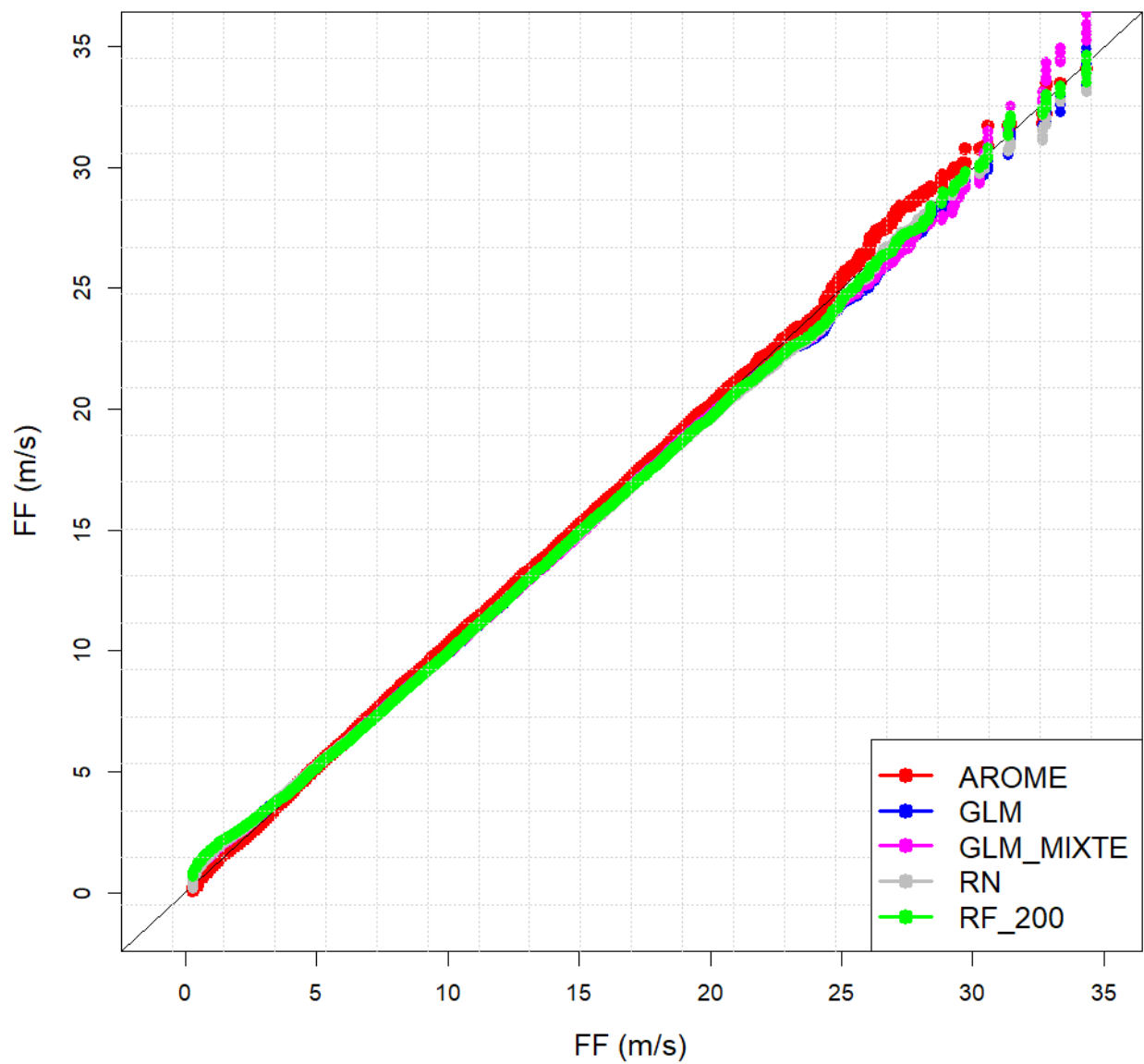
Illustration 8.27 : AO4 Barfleur – 200 M – FF – QQ-Plot de FF pour les modèles GLM, GLM_MIXTE, RF_200, RNA et AROME
