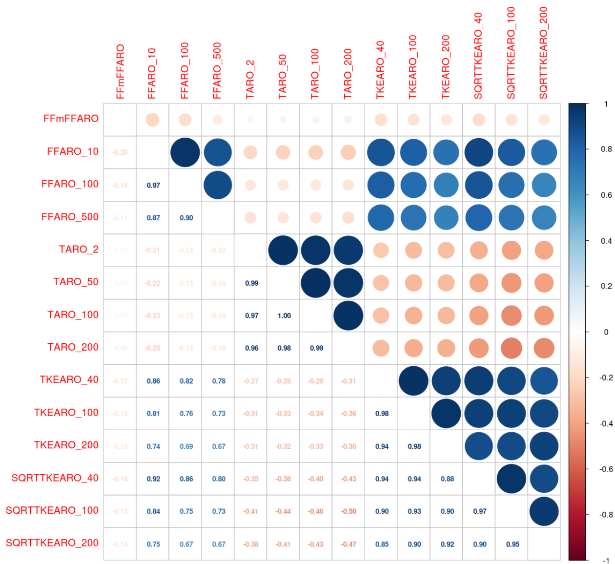
Illustration 8.4 : AO5 Bretagne Sud – 40 M – Deuxième groupe (variables de l'ACP) pour la prédiction de FF
