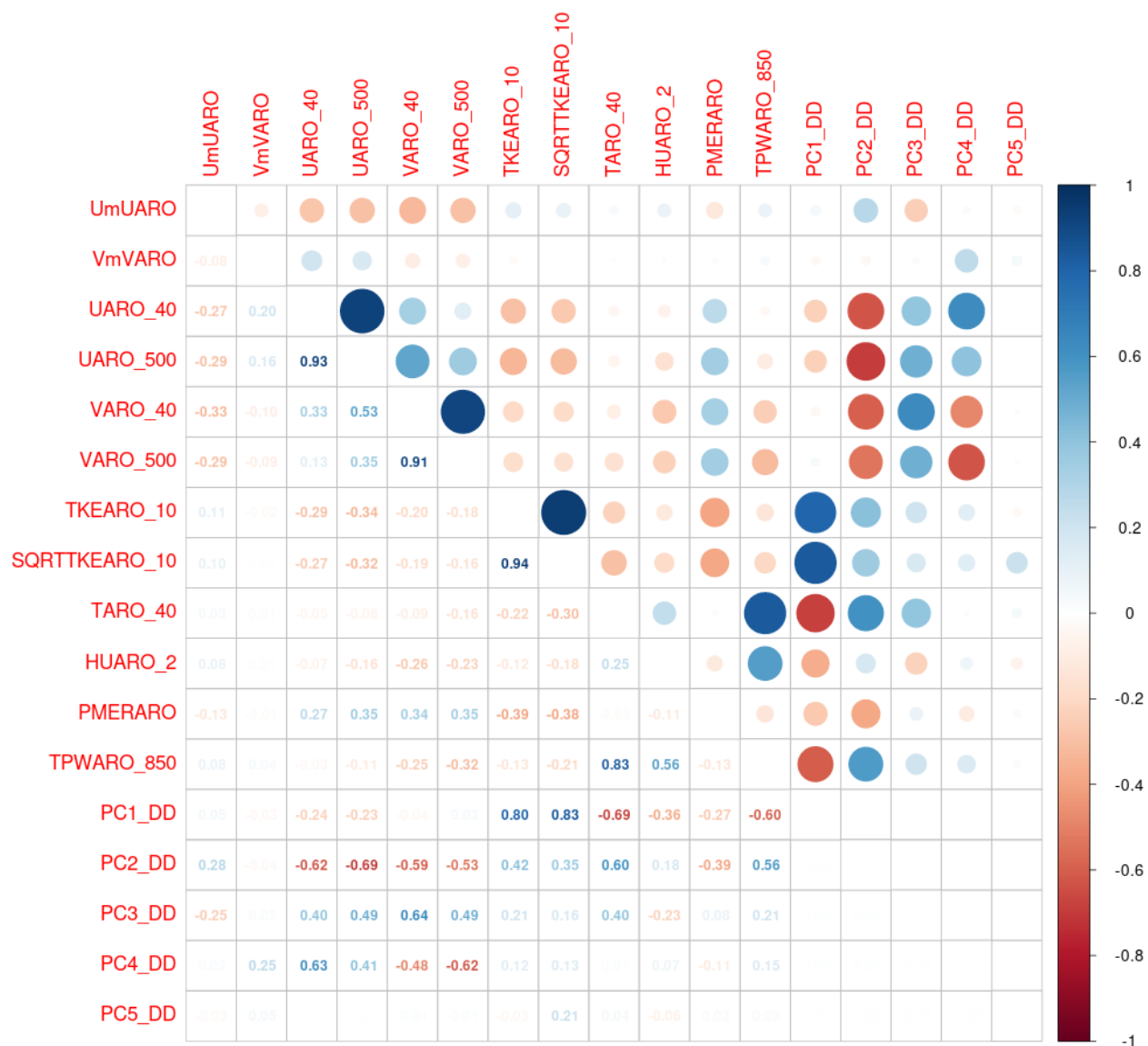
Illustration 8.37 : AO4 Barfleur – 40 M – Variables explicatives finales (avec les composantes principales de l'ACP) pour la prédiction de DD
