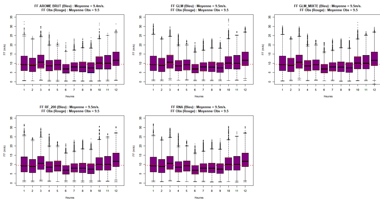
Illustration 8.32 : AO5 Bretagne Sud – 200 M – FF – Cycle annuel des modèles statistiques (bleu) superposé aux observations (rouge)
