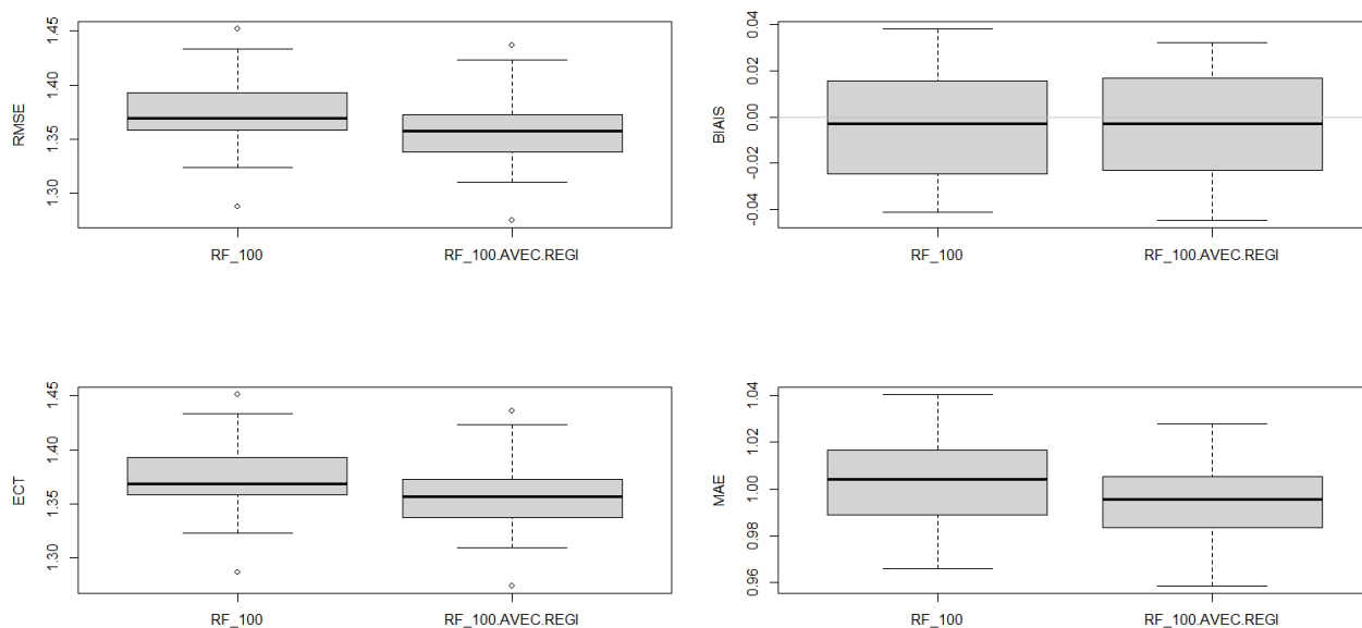
Illustration 7.38 : Station de test 2 – FF – Modèles de forêt aléatoire à 100 arbres avec et sans prédicteurs de régimes de temps - Box-plot RMSE (haut gauche), ECT (bas gauche), BIAIS (haut droite) et MAE (bas droite) pour l'échantillon de test
