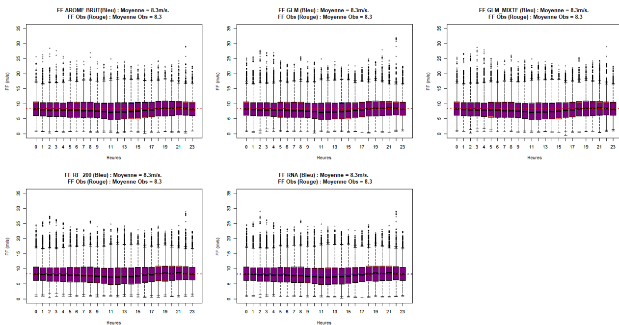
Illustration 8.20 : AO5 Bretagne Sud – 40 M – FF – Cycle diurne des modèles statistiques (bleu) superposé aux observations (rouge)
