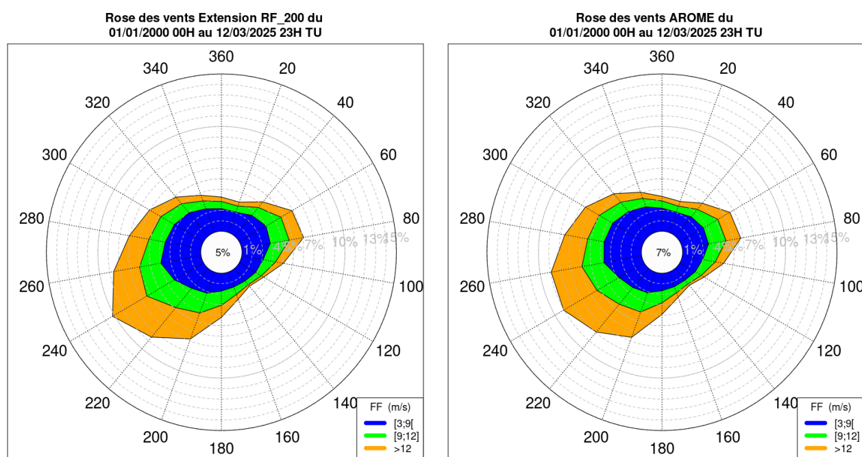
Illustration 4.23 : BNO – Roses des vents sur la période d'extension pour le niveau 100 m (du 01/01/2000 00H TU au 12/03/2025 23H TU). À gauche on retrouve la rose de l'extension statistique et à droite la rose d'AROME.
