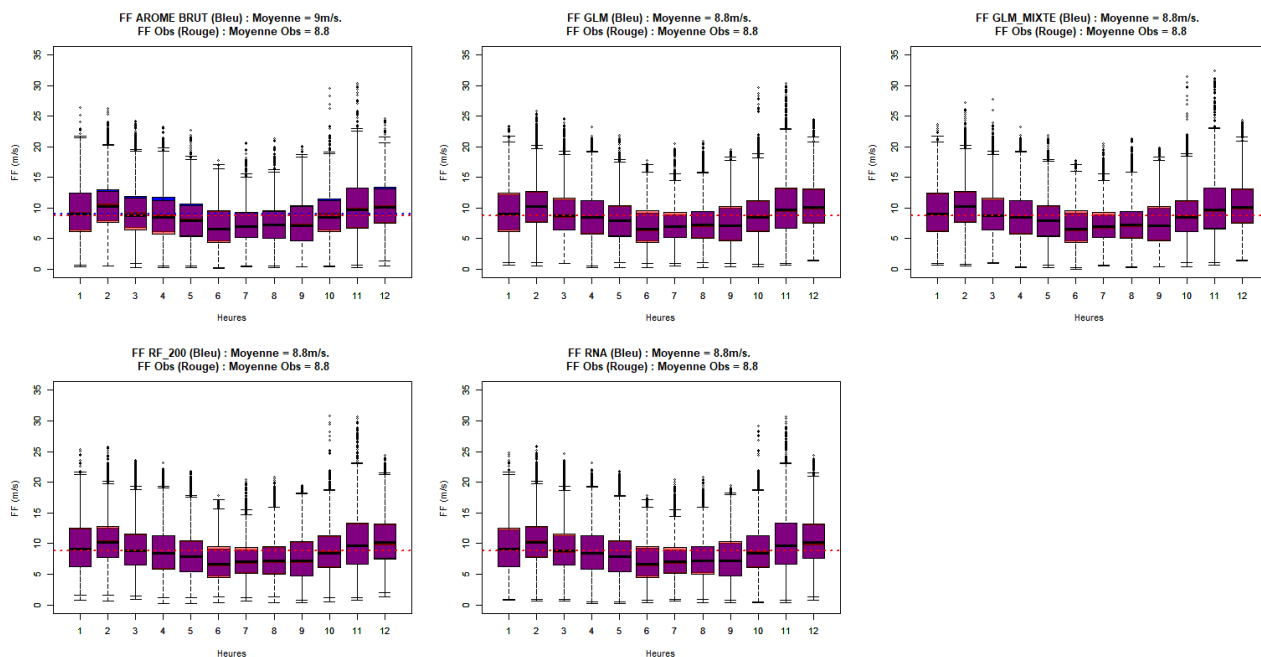
Illustration 8.21 : AO4 Barfleur – 40 M – FF – Cycle annuel des modèles statistiques (bleu) superposé aux observations (rouge)
