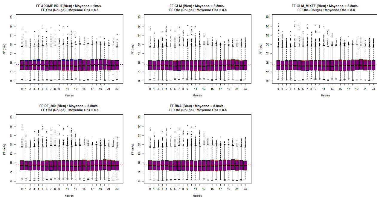
Illustration 8.19 : AO4 Barfleur – 40 M – FF – Cycle diurne des modèles statistiques (bleu) superposé aux observations (rouge)
