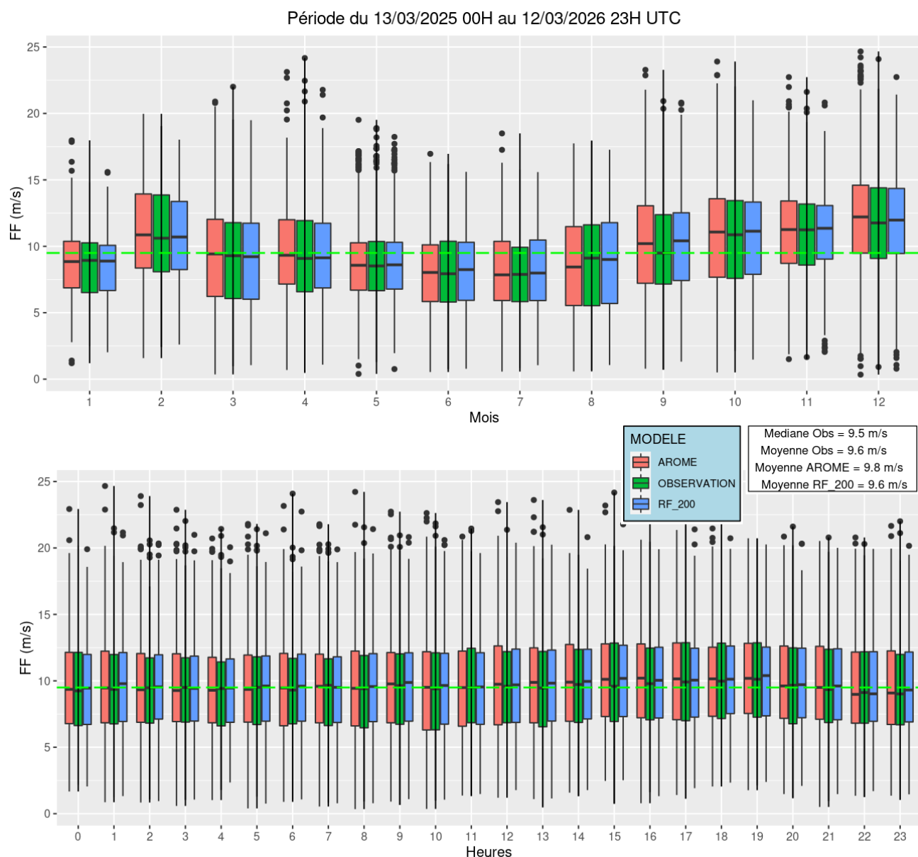
Illustration 4.1 : BNO – FF – Restitution des cycles de FF sur la période d'observation pour le niveau 100 m (du 13/03/2025 00H au 12/03/2026 23H). Sur la première ligne on retrouve le cycle annuel et sur la deuxième ligne le cycle diurne. La ligne discontinue verte traversant les boxplots désigne la médiane de l'observation sur la période d'observation.
