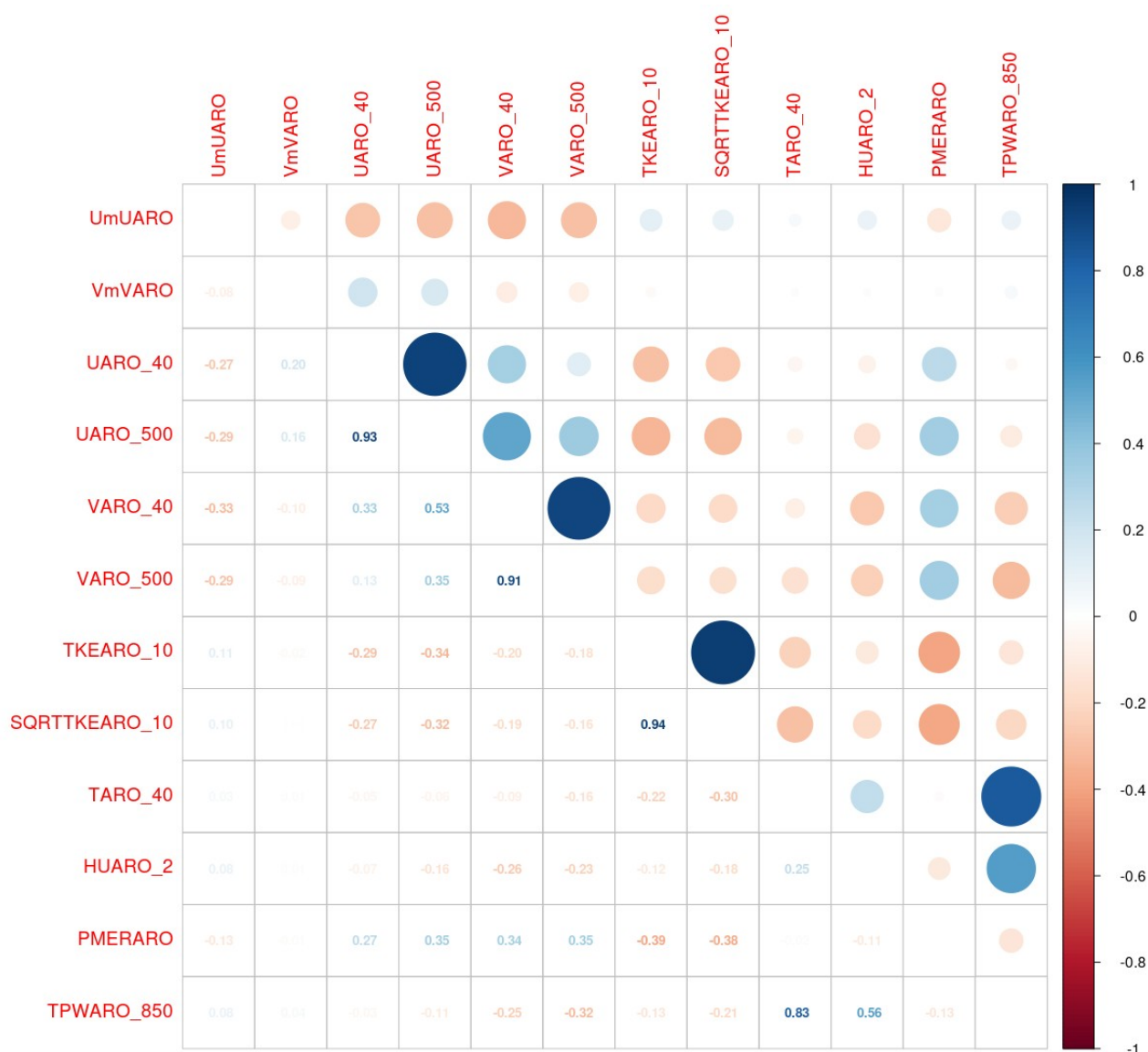
Illustration 8.33 : AO4 Barfleur – 40 M – Premier groupe (variables explicatives conservées pour la sélection finale) pour la prédiction de DD
