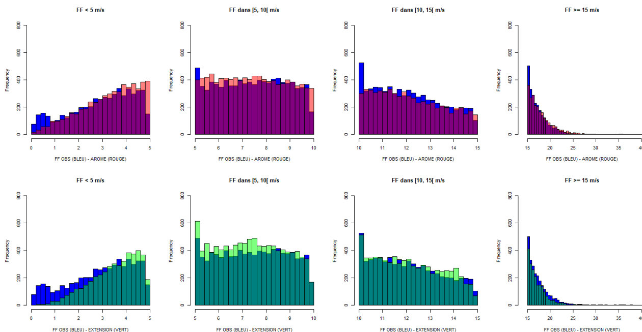
Illustration 7.55 : Station de test 2 – Histogrammes de FF par classe de vent par pas de 5 m/s pour les années 2017 à 2020 (sans les données d'apprentissage de l'année 2018). En haut, observations (bleu) comparées à AROME (rouge). En bas, observations (bleu) comparées à l'extension (vert).
