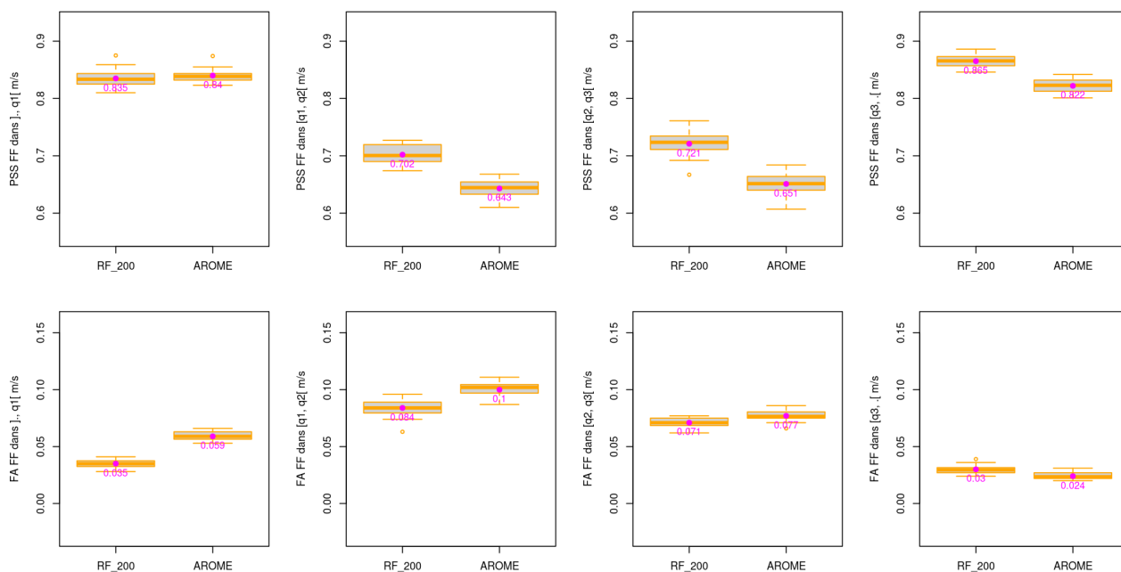
Illustration 3.24 : BNO – V – Niveau 100 m – Modèle de forêt aléatoire à 200 arbres - Box-plot PSS et FA pour l'échantillon de test. La valeur en magenta sur chaque boîte à moustaches correspond à la moyenne des 20 échantillons.
