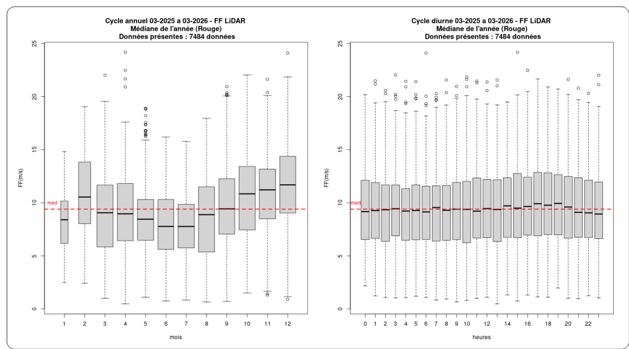
Illustration 3.4 : BNO – FF – Niveau 100 m – Distribution du vent mensuelle (graphique de gauche) et horaire (graphique de droite) à partir des données observées
