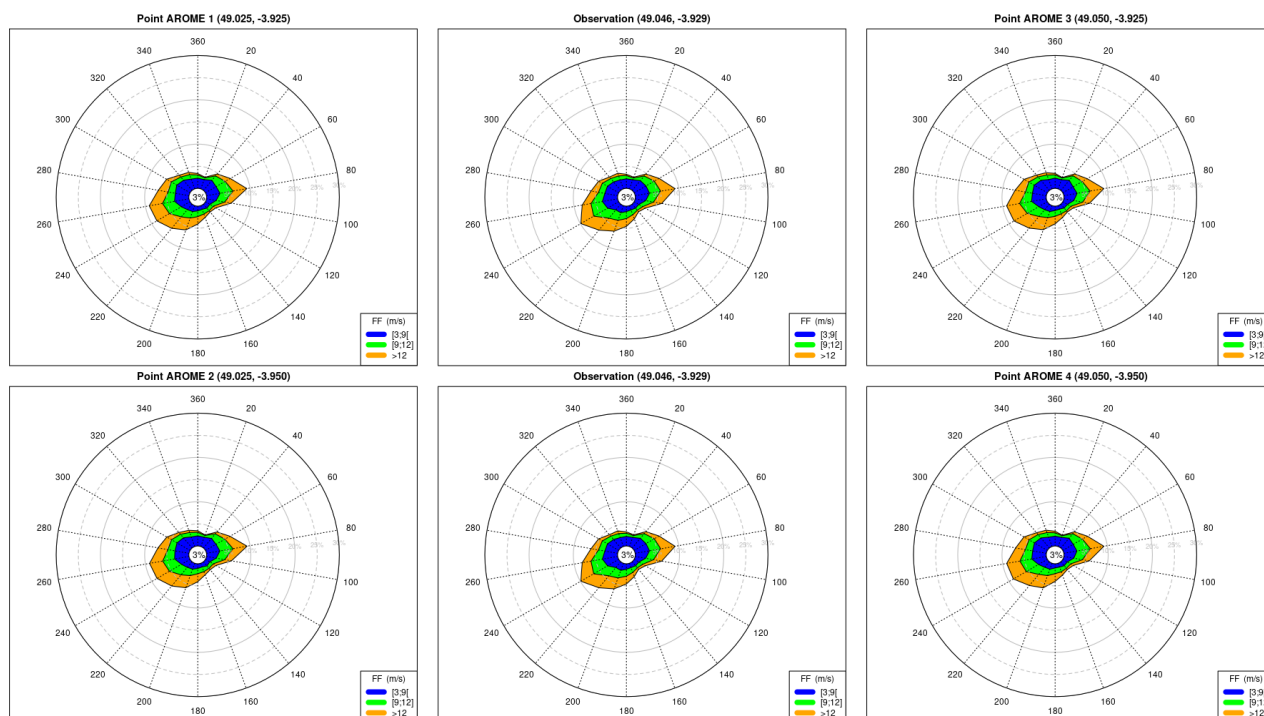
Illustration 3.1: BNO – Choix du point AROME de référence – Roses des vents du point d'observation (en double au milieu) et des 4 points AROME voisins calculées pendant la période de mesure pour le niveau 100 m
