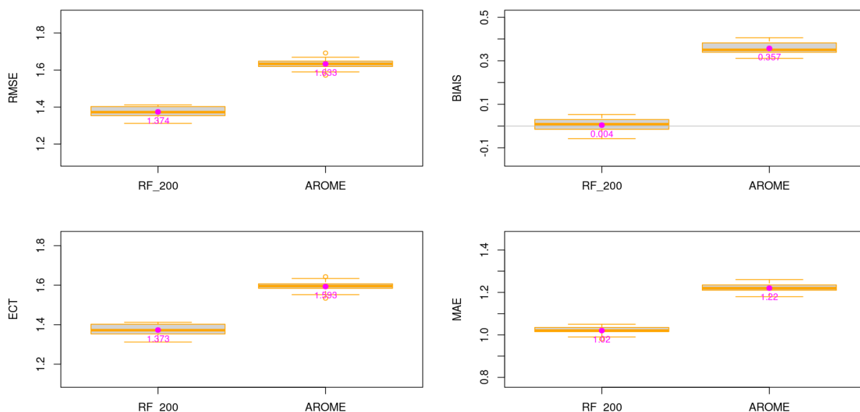
Illustration 3.19 : BNO – U – Niveau 100 m – Modèle de forêt aléatoire à 200 arbres - Box-plot RMSE, ECT, BIAIS et MAE pour l'échantillon de test. La valeur en magenta sur chaque boîte à moustaches correspond à la moyenne des 20 échantillons.
