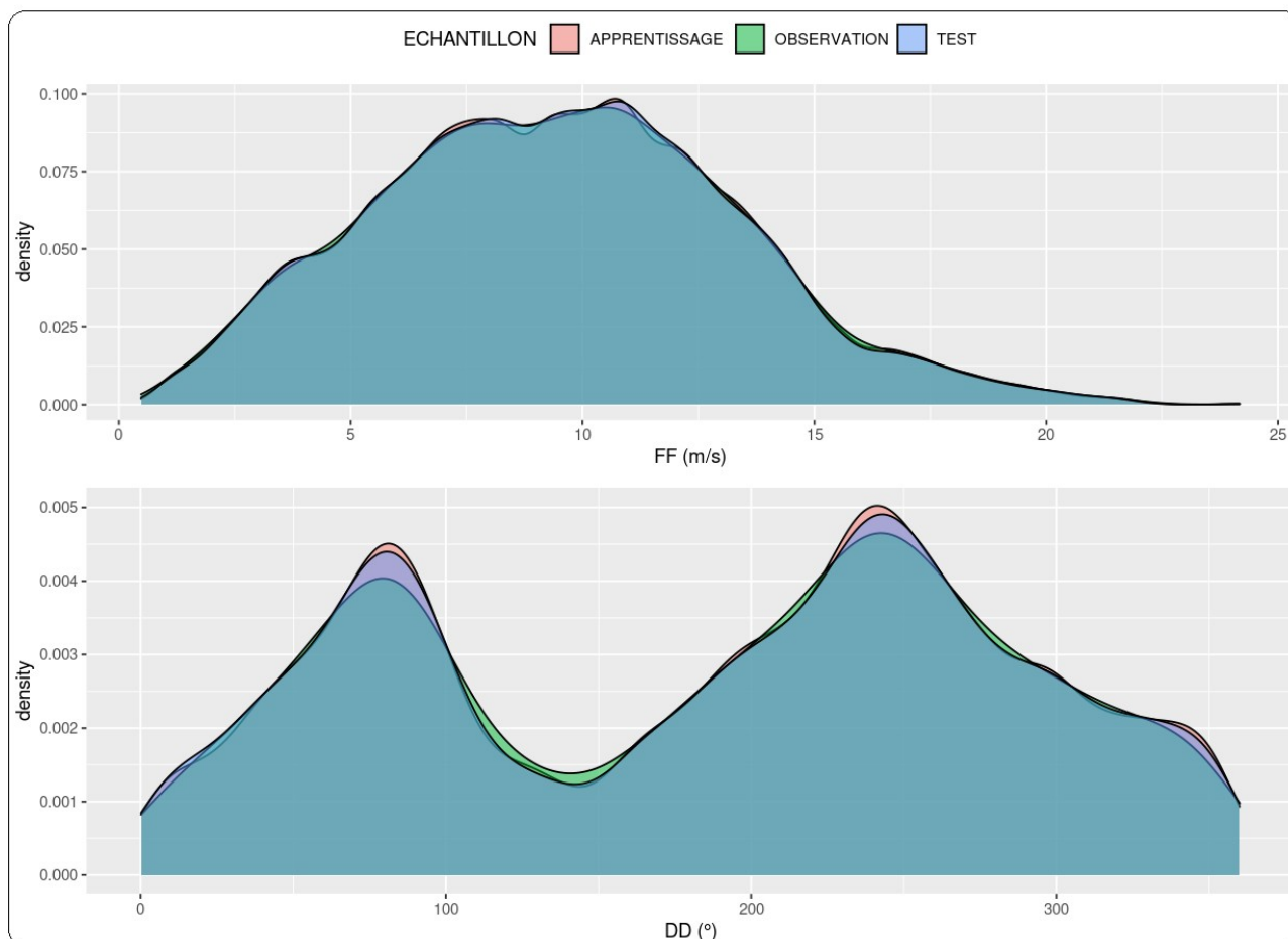
Illustration 3.8 : BNO – Distribution de FF (première ligne) et DD (deuxième ligne) pour les échantillons d'apprentissage et de test comparée à celle de l'observation sur la période d'apprentissage (période d'observation) pour le niveau 100 m
