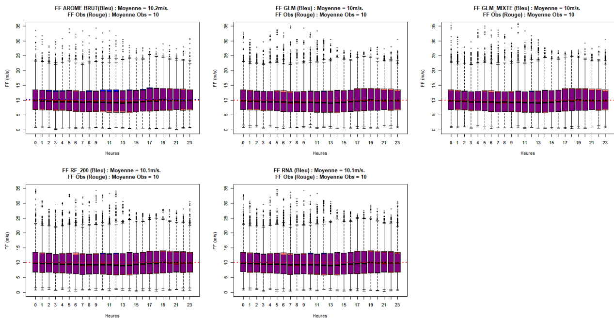
Illustration 8.29 : AO4 Barfleur – 200 M – FF – Cycle diurne des modèles statistiques (bleu) superposé aux observations (rouge)
