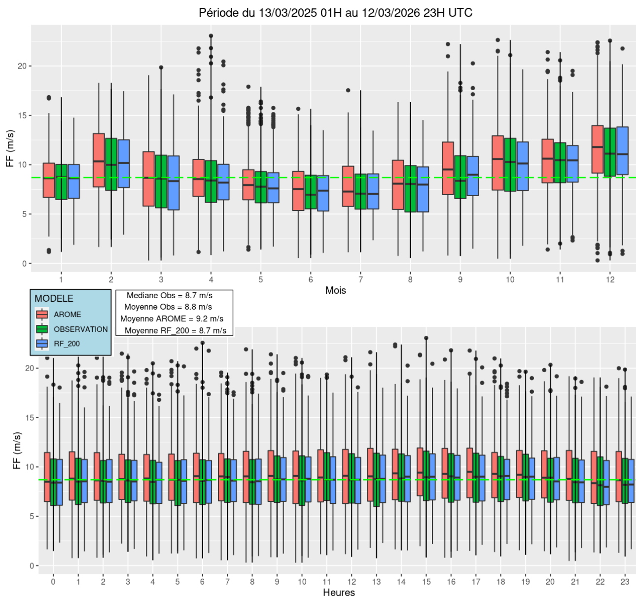
Illustration 4.5 : BNO – FF – Restitution des cycles de FF sur la période d'observation pour le niveau 40 m (du 13/03/2025 00H au 12/03/2026 23H). Sur la première ligne on retrouve le cycle annuel et sur la deuxième ligne le cycle diurne. La ligne discontinue verte traversant les boxplots désigne la médiane de l'observation sur la période d'observation.
