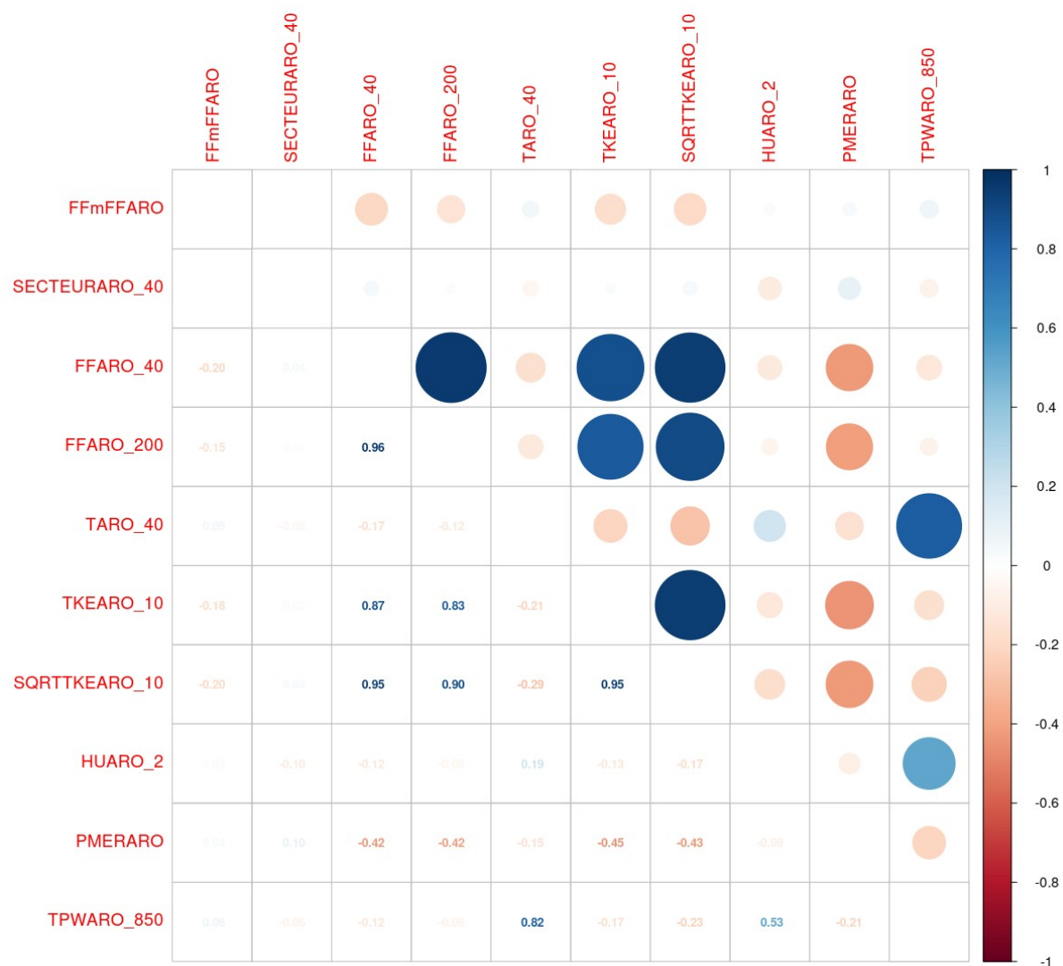
Illustration 8.2 : AO5 Bretagne Sud – 40 M – Premier groupe (variables explicatives conservées pour la sélection finale) pour la prédiction de FF
