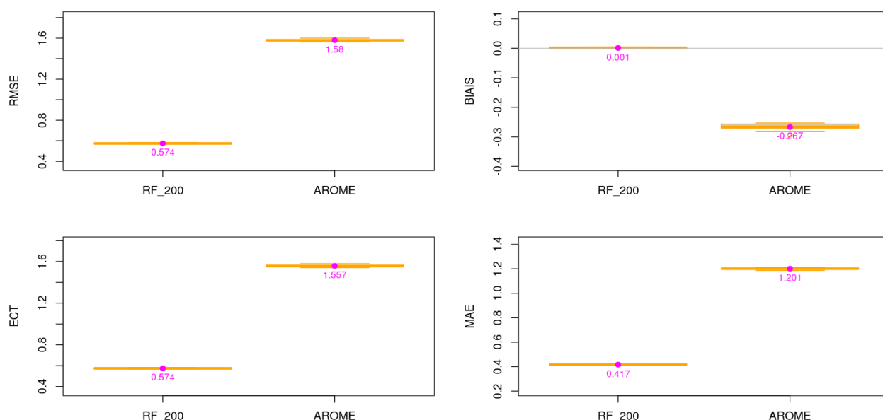
Illustration 3.21 : BNO – V – Niveau 100 m – Modèle de forêt aléatoire à 200 arbres - Box-plot RMSE (haut gauche), ECT (bas gauche), BIAIS (haut droite) et MAE (bas droite) pour l'échantillon d'apprentissage. La valeur en magenta sur chaque boîte à moustaches correspond à la moyenne des 20 échantillons.
