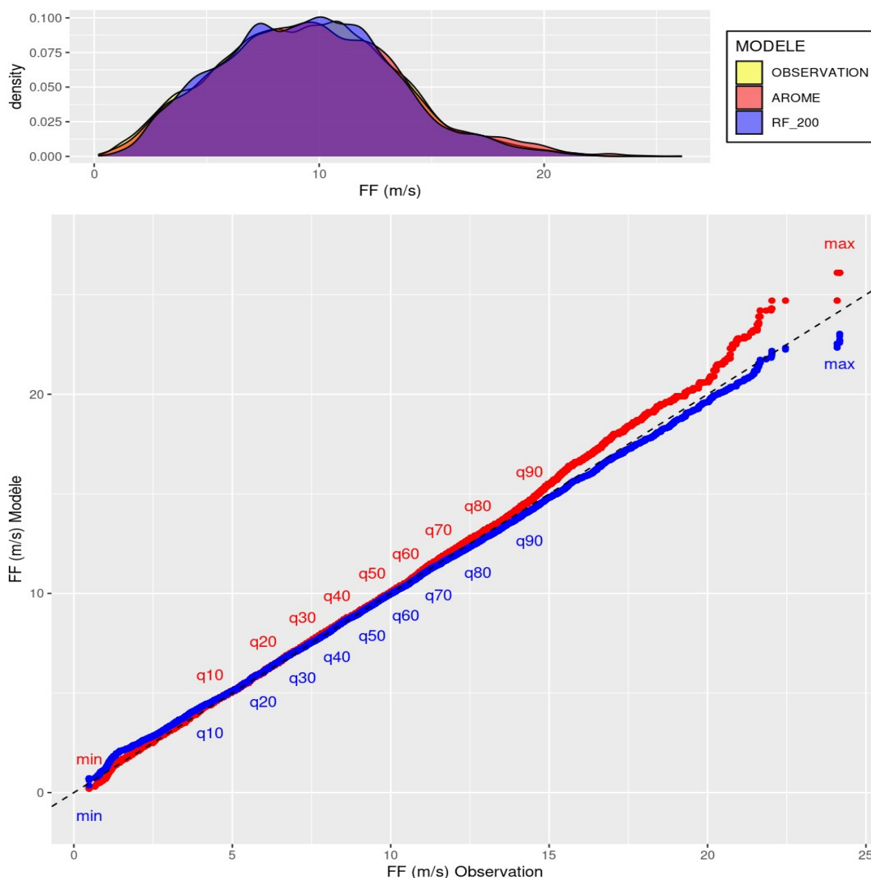
Illustration 3.16 : BNO – FF – QQ-Plots sur l'échantillon de test concaténé pour le niveau 100 m. En rouge : AROME, en bleu : RF_200.
