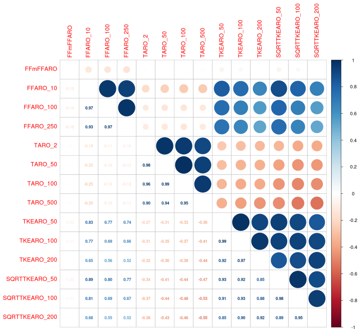
Illustration 8.9 : AO4 Barfleur – 200 M – Deuxième groupe (variables de l'ACP) pour la prédiction de FF
