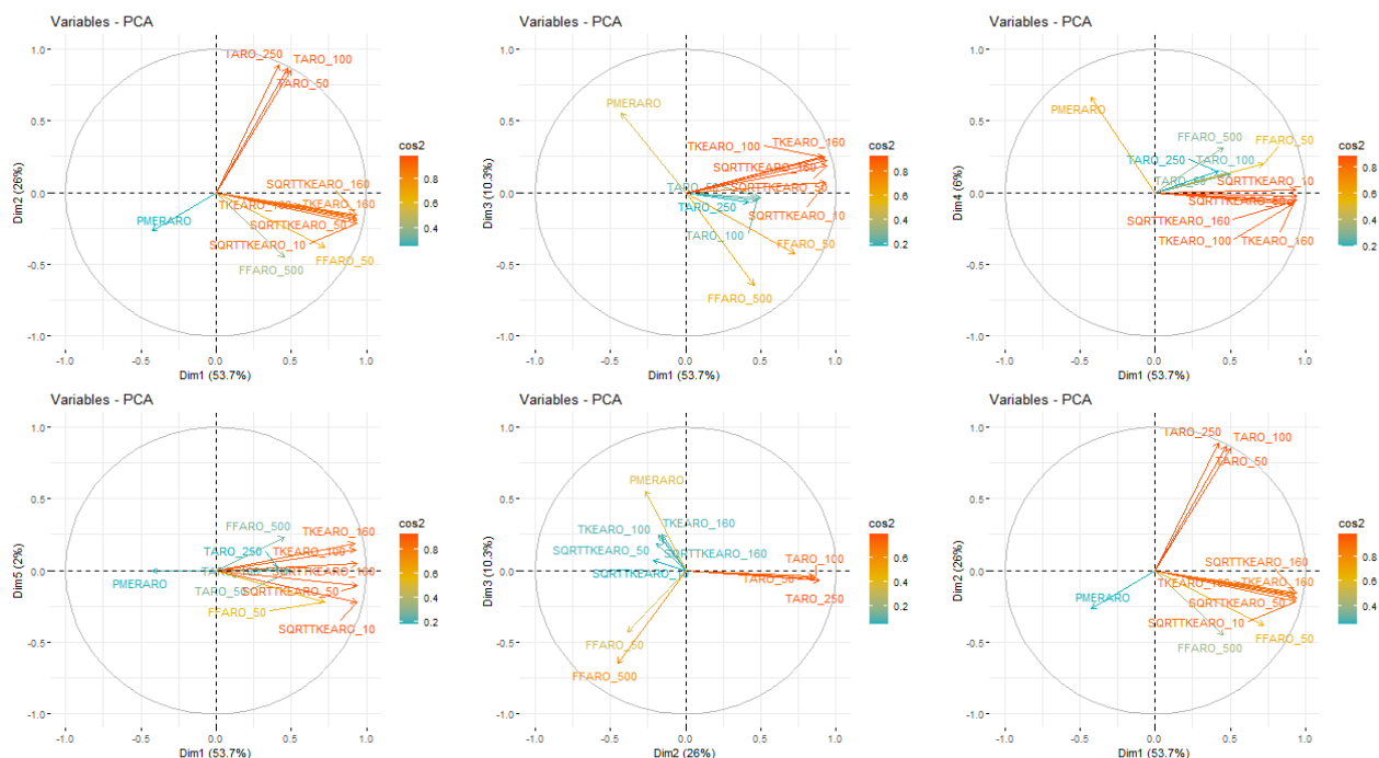
Illustration 7.5 : Station de test 1 – FF – Représentation des variables sur les plans factoriels de l'ACP (première partie des plans) : première ligne dimension 1-2, dimension 1-3 et dimension 1-4 ; deuxième ligne dimension 1-5, dimension 2-3, et dimension 1-2 (à nouveau)
