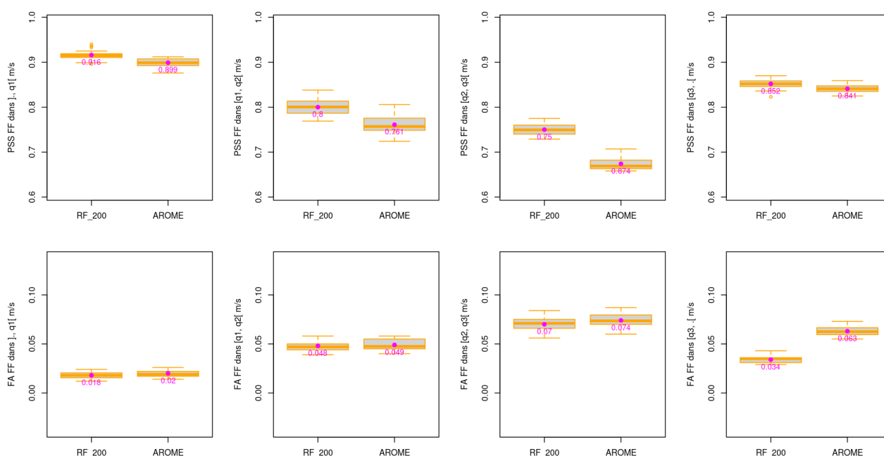
Illustration 3.20 : BNO – U – Niveau 100 m – Modèle de forêt aléatoire à 200 arbres - Box-plot PSS et FA pour l'échantillon de test. La valeur en magenta sur chaque boîte à moustaches correspond à la moyenne des 20 échantillons.
