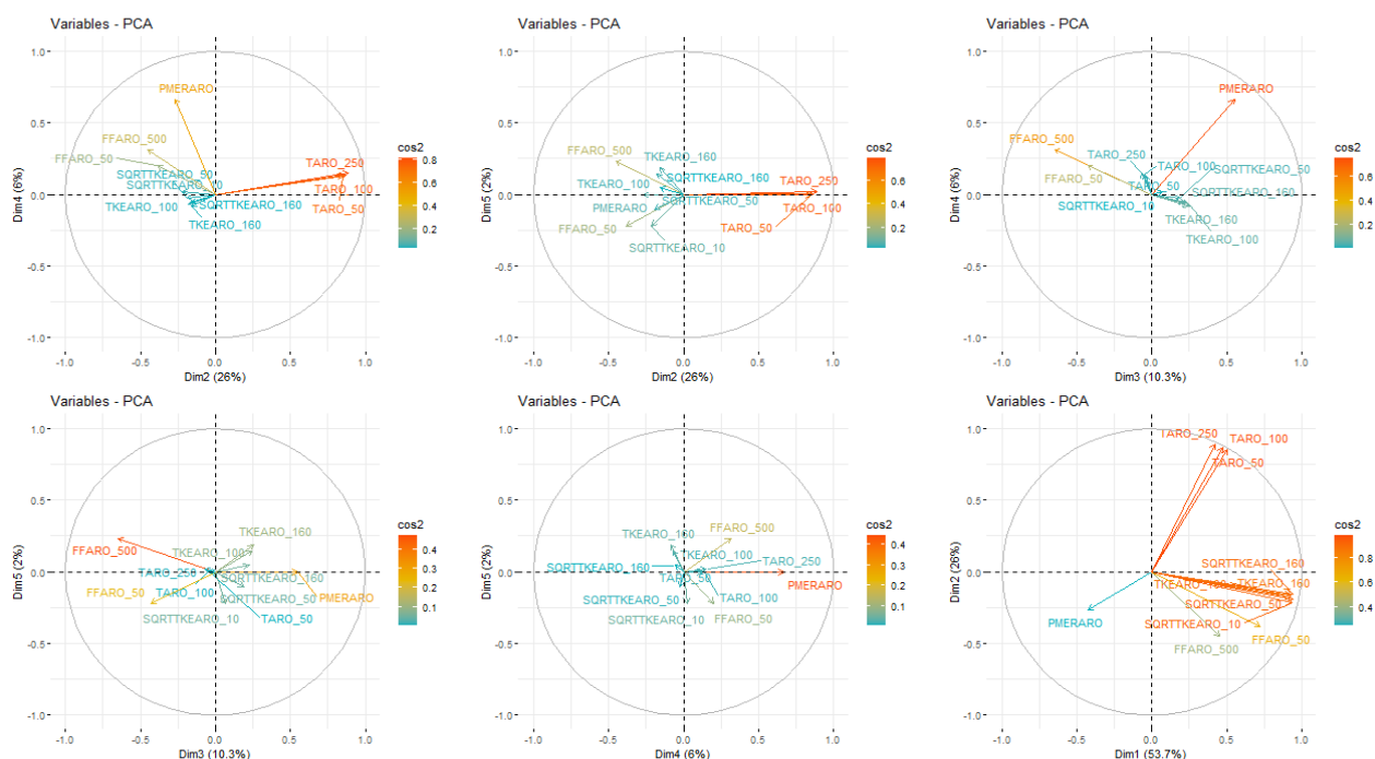
Illustration 7.6 : Station de test 1 – FF – Représentation des variables sur les plans factoriels de l'ACP (deuxième partie des plans) : première ligne dimension 2-4, dimension 2-5 et dimension 3-4 ; deuxième ligne dimension 3-5, dimension 4-5, et dimension 1-2
