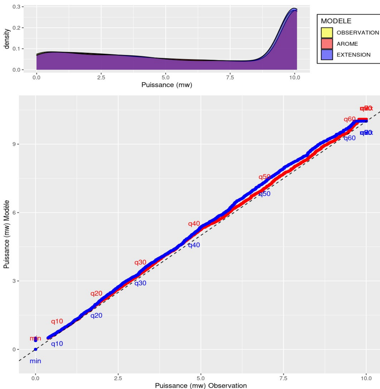
Illustration 4.13 : BNO – QQ-Plot des données de puissances de l'extension statistique (bleu) et AROME (rouge) sur la période d'observation pour le niveau 100 m.
