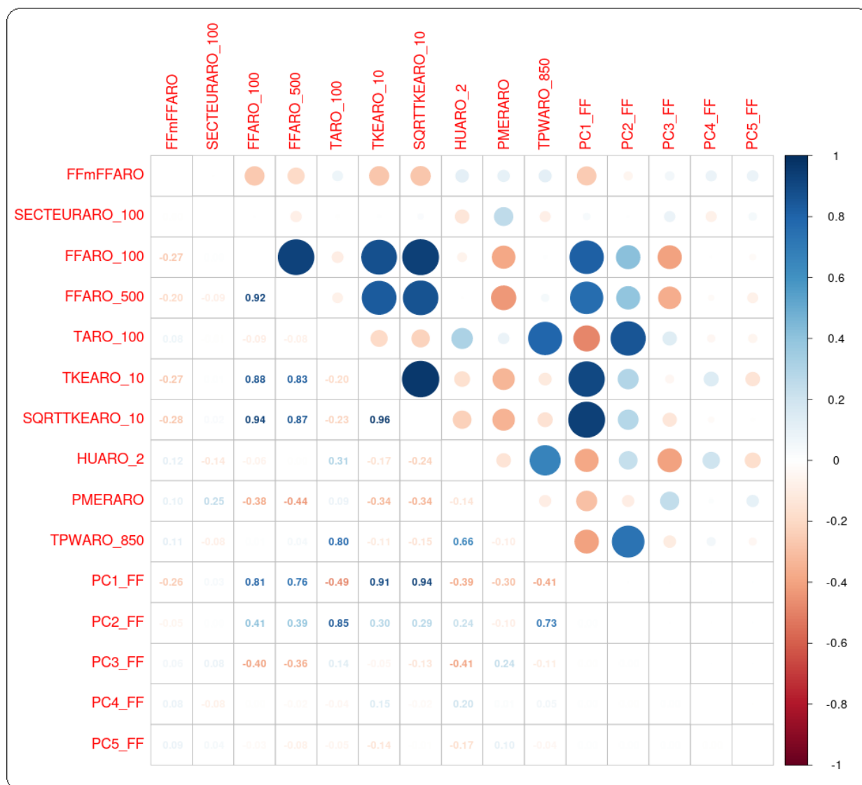
Illustration 3.3 : BNO – FF – Niveau 100 m - Corrélation entre la variable à expliquer FFmFFARO et les variables explicatives. En haut : sous forme de bulles. En bas : chiffré (0 : absence de corrélation, 1 ou -1 : forte corrélation)
