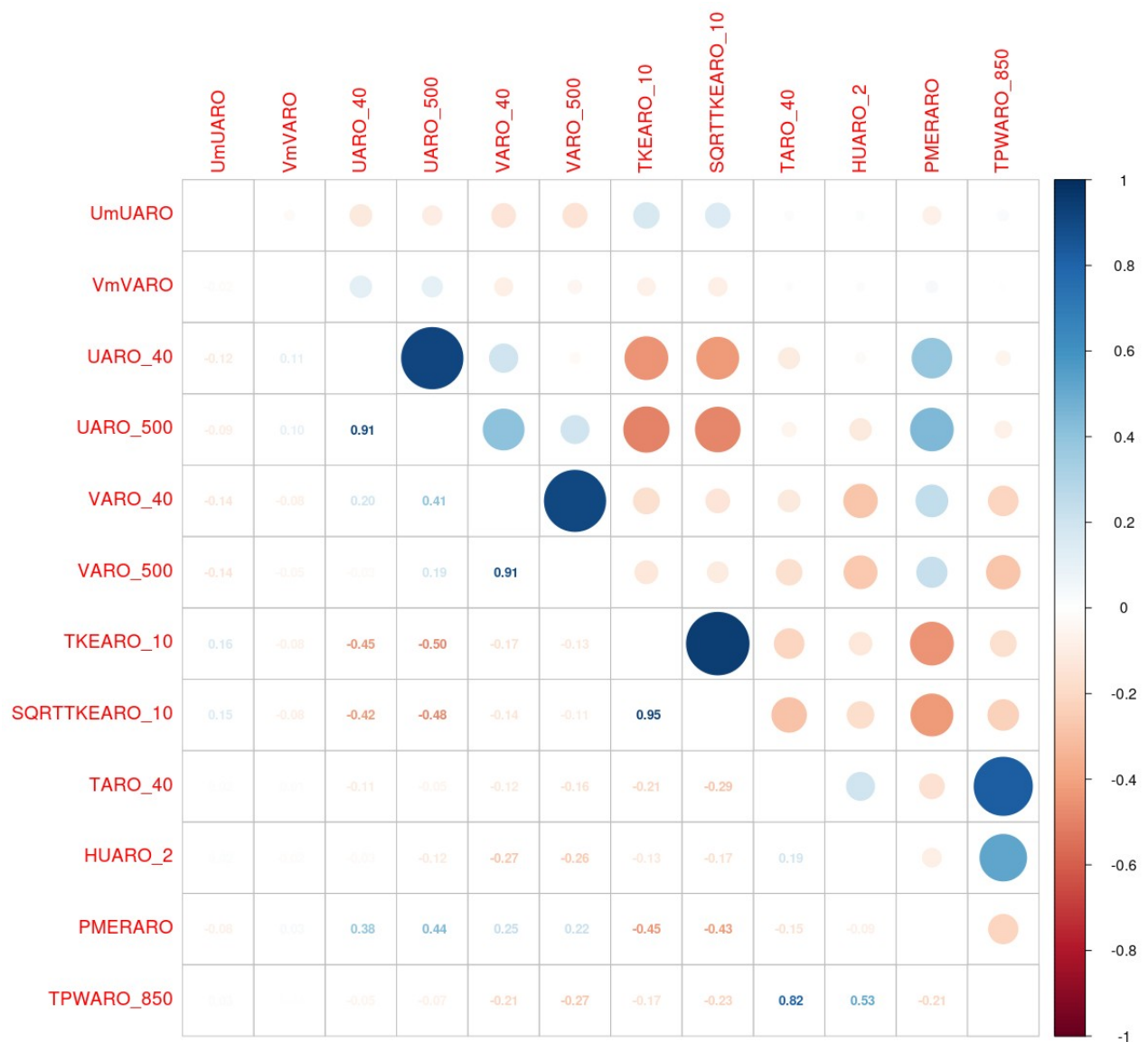
Illustration 8.34 : AO5 Bretagne Sud – 40 M – Premier groupe (variables explicatives conservées pour la sélection finale) pour la prédiction de DD
