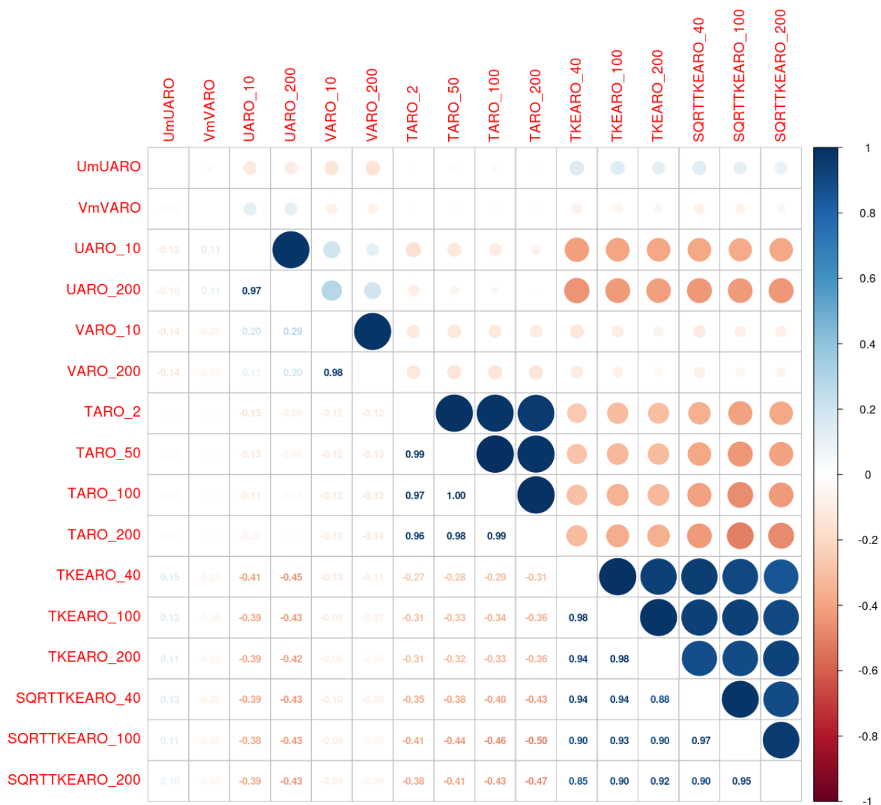
Illustration 8.36 : AO5 Bretagne Sud – 40 M – Deuxième groupe (variables de l'ACP) pour la prédiction de DD
