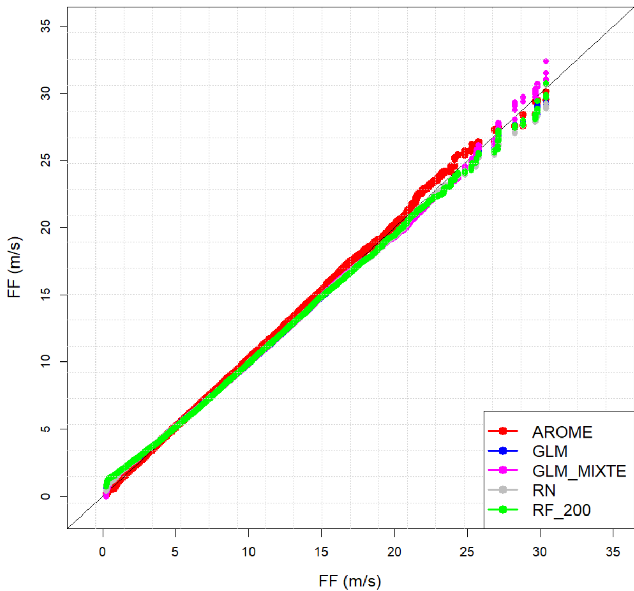
Illustration 8.17 : AO4 Barfleur – 40 M – FF – QQ-Plot de FF pour les modèles GLM, GLM_MIXTE, RF_200, RNA et AROME
