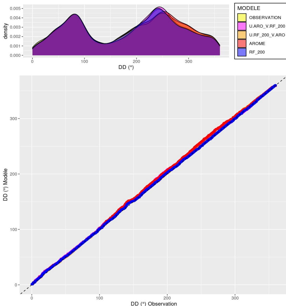
Illustration 3.26 : BNO – DD – QQ-Plots de la reconstitution de DD avec combinaison de U et V sur l'échantillon de test concaténé. En violet : U.ARO V.RF_200, en orange : U.RF_200 V.ARO, en rouge : AROME, en bleu : RF_200.
