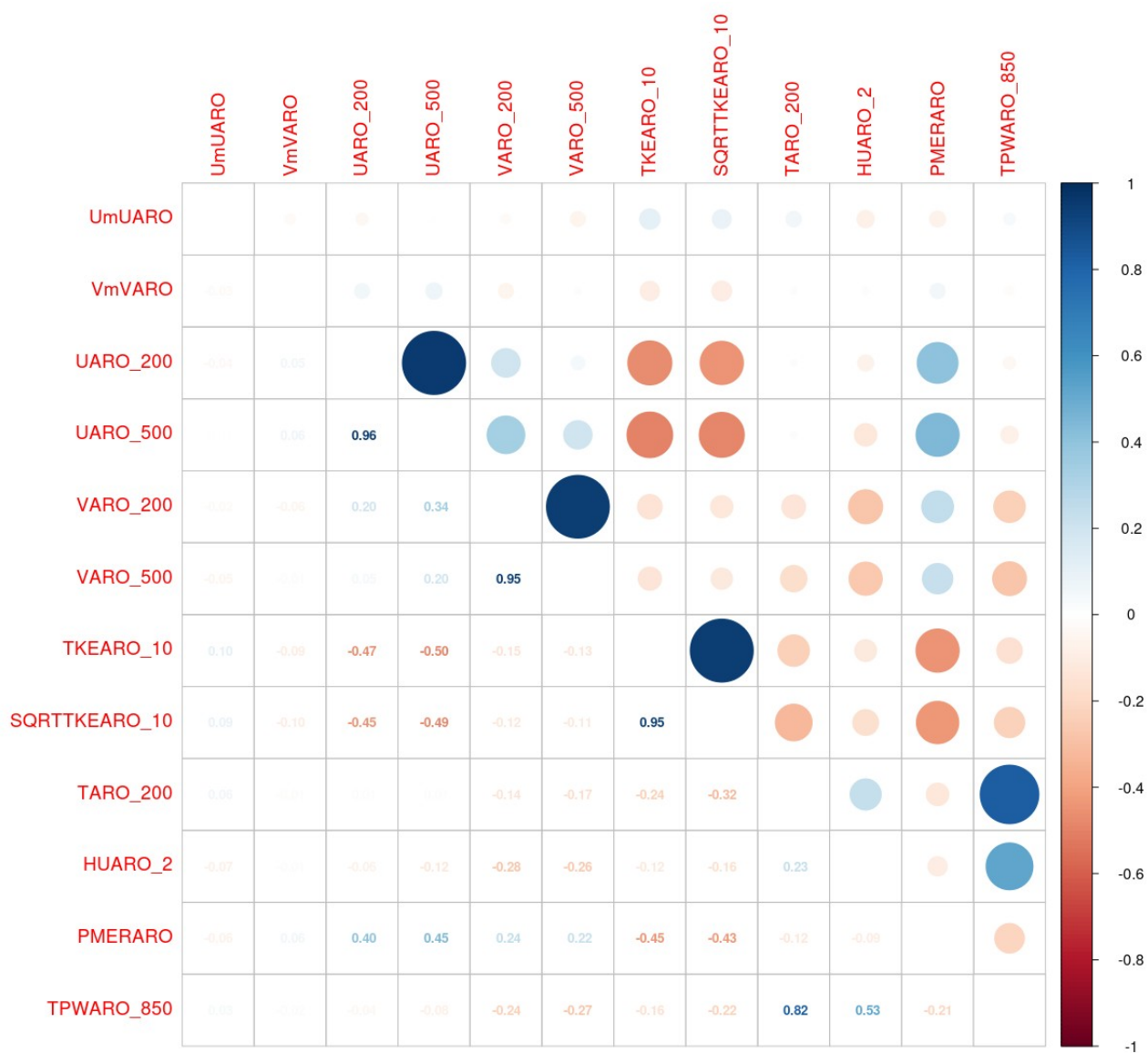
Illustration 8.40 : AO5 Bretagne Sud – 200 M – Premier groupe (variables explicatives conservées pour la sélection finale) pour la prédiction de DD
