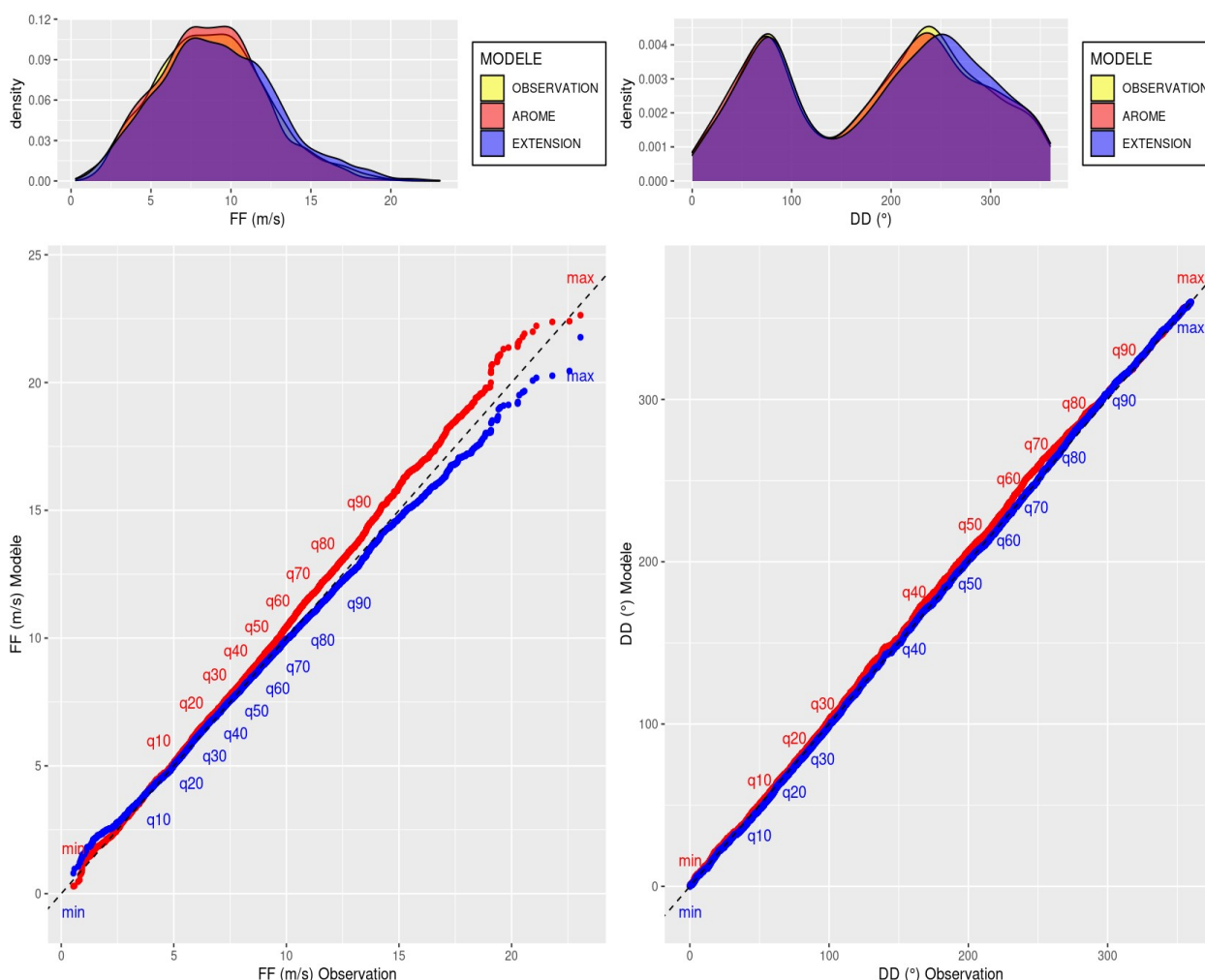
Illustration 4.12 : BNO – QQPlots FF et DD sur la période d'observation pour le niveau 40 m . En rouge : AROME, en bleu : extension statistique.
