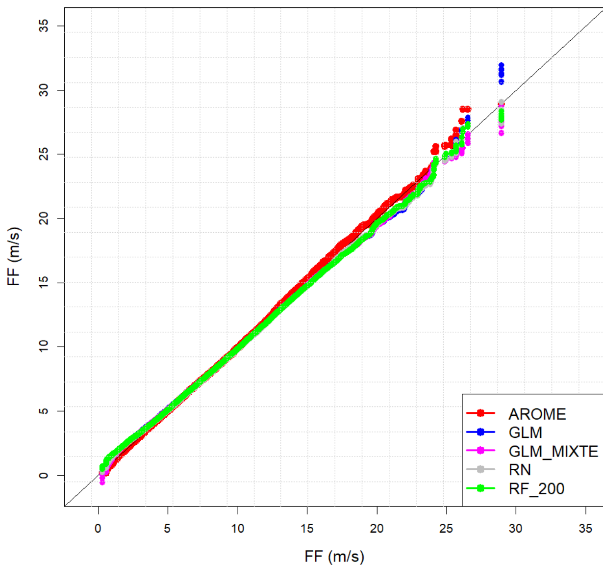
Illustration 8.18 : AO5 Bretagne Sud – 40 M – FF – QQ-Plot de FF pour les modèles GLM, GLM_MIXTE, RF_200, RNA et AROME
