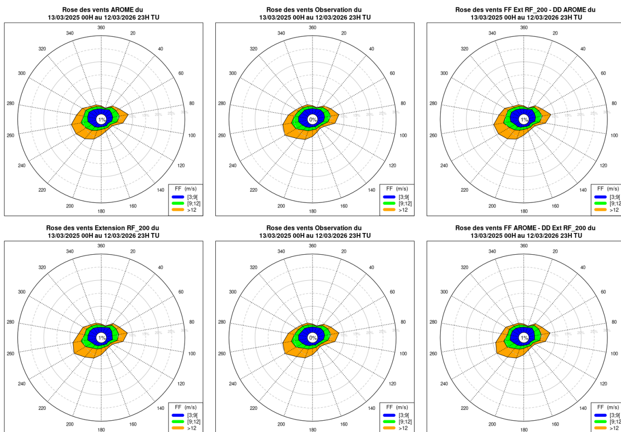
Illustration 4.15 : BNO – Roses des vents partielles (excluant les forces de vent FF < 3 m/s) sur la période d'observation pour le niveau 200 m (du 13/03/2025 00H au 12/03/2026 23H) : sur la 1 re colonne (de haut en bas) on retrouve la rose AROME et celle de l'extension ; sur la 2 e colonne on retrouve la rose de l'observation. Les deux vignettes de cette colonne sont identiques et ont été dupliquées par soucis de lisibilité ; et sur la 3 e colonne (de haut en bas) on retrouve respectivement les roses issues de FF Extension et DD AROME, FF AROME et DD Extension
