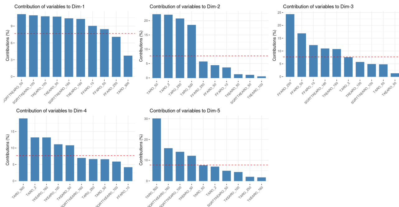
Illustration 3.15 : BNO – FF – Niveau 100 m – Contribution des variables à l'ACP (une figure pour chaque dimension)
