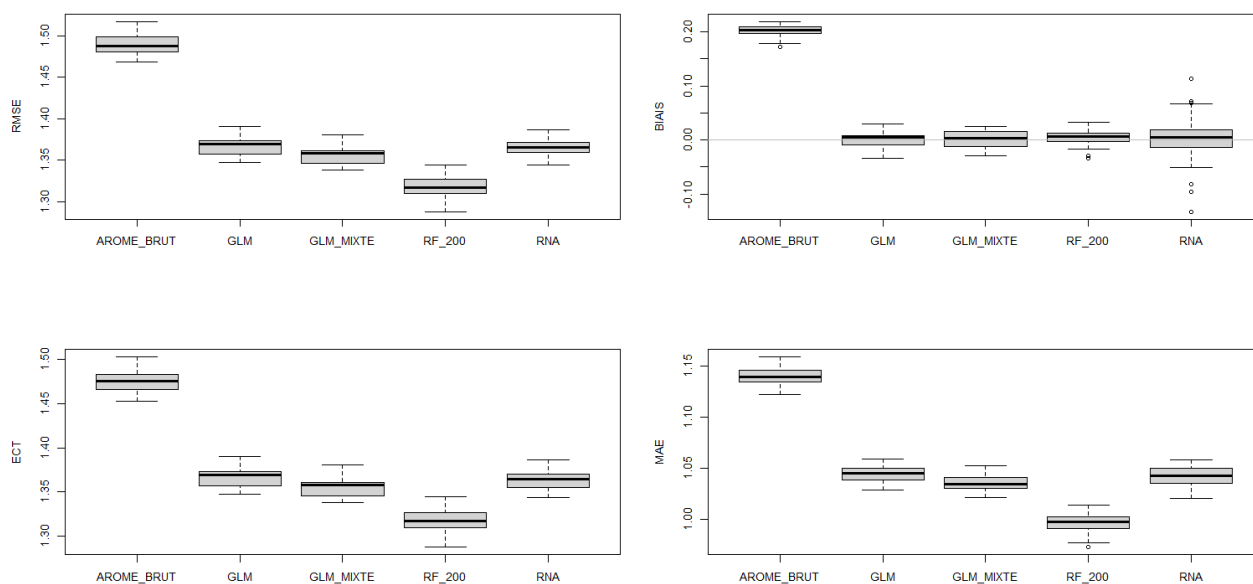
Illustration 8.23 : AO4 Barfleur – 200 M – FF – Comparaison inter-modèles - Box-plot RMSE (haut gauche), ECT (bas gauche), BIAIS (haut droite) et MAE (bas droite) pour l'échantillon de test
