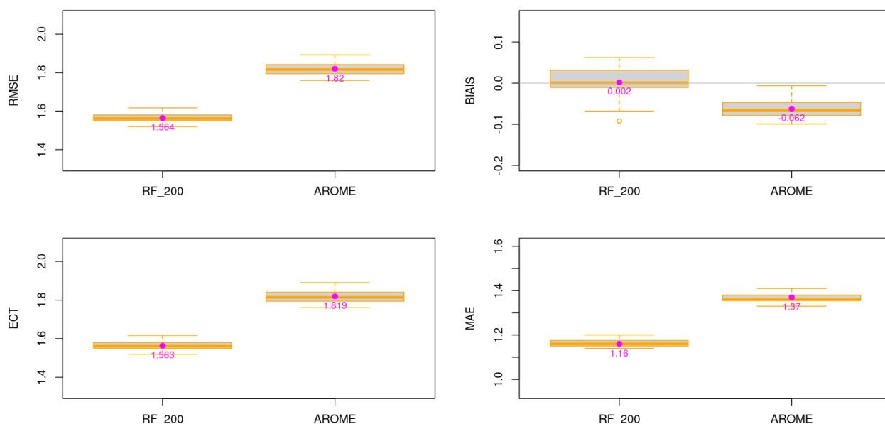
Illustration 3.20 : GLE – U – Niveau 100 m – Modèle de forêt aléatoire à 200 arbres - Box-plot RMSE, ECT, BIAIS et MAE pour l'échantillon de test. La valeur en magenta sur chaque boîte à moustaches correspond à la moyenne des 20 échantillons.
