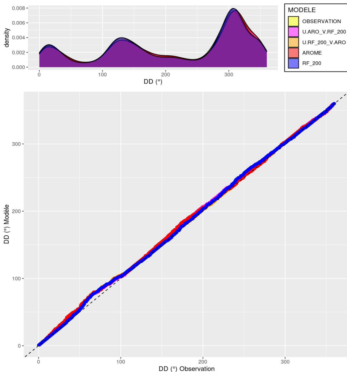
Illustration 3.27 : GLE – DD – QQ-Plots de la reconstitution de DD avec combinaison de U et V sur l'échantillon de test concaténé. En violet : U.ARO V.RF_200, en orange : U.RF_200 V.ARO, en rouge : AROME, en bleu : RF_200.
