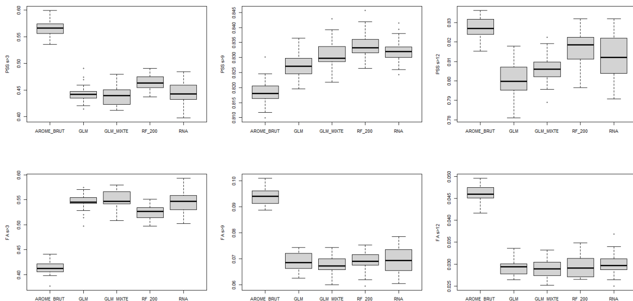
Illustration 8.15 : AO4 Barfleur – 40 M – FF – Comparaison inter-modèles - Box-plot PSS (première ligne pss FF > 3 m/s, pss FF > 9 m/s et pss FF > 12 m/s) et FA (deuxième ligne fa FF > 3 m/s, fa FF > 9 m/s et fa FF > 12 m/s) pour l'échantillon de test
