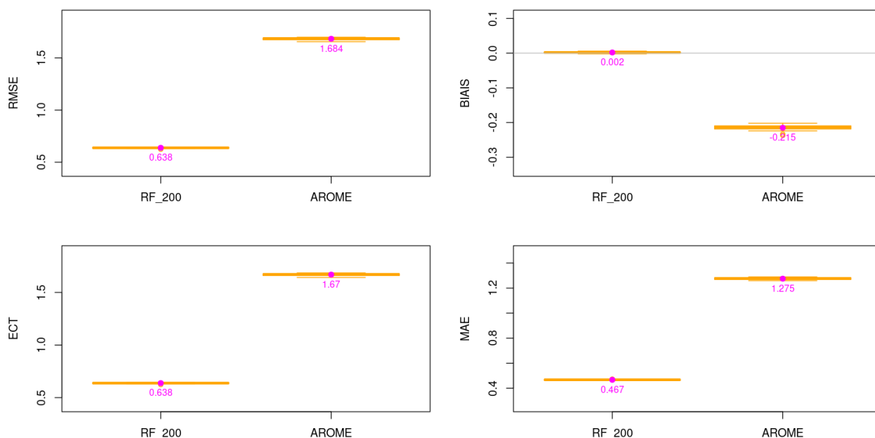
Illustration 3.12 : GLE – FF – Niveau 100 m – Modèle de forêt aléatoire à 200 arbres - Box-plot RMSE (haut gauche), ECT (bas gauche), BIAIS (haut droite) et MAE (bas droite) pour l'échantillon d'apprentissage. La valeur en magenta sur chaque boîte à moustaches correspond à la moyenne des 20 échantillons.
