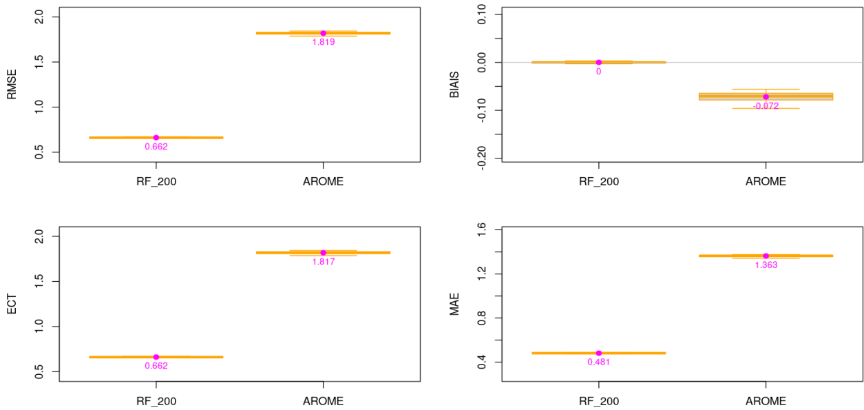
Illustration 3.18 : GLE – U – Niveau 100 m – Modèle de forêt aléatoire à 200 arbres - Box-plot RMSE (haut gauche), ECT (bas gauche), BIAIS (haut droite) et MAE (bas droite) pour l'échantillon d'apprentissage. La valeur en magenta sur chaque boîte à moustaches correspond à la moyenne des 20 échantillons.
