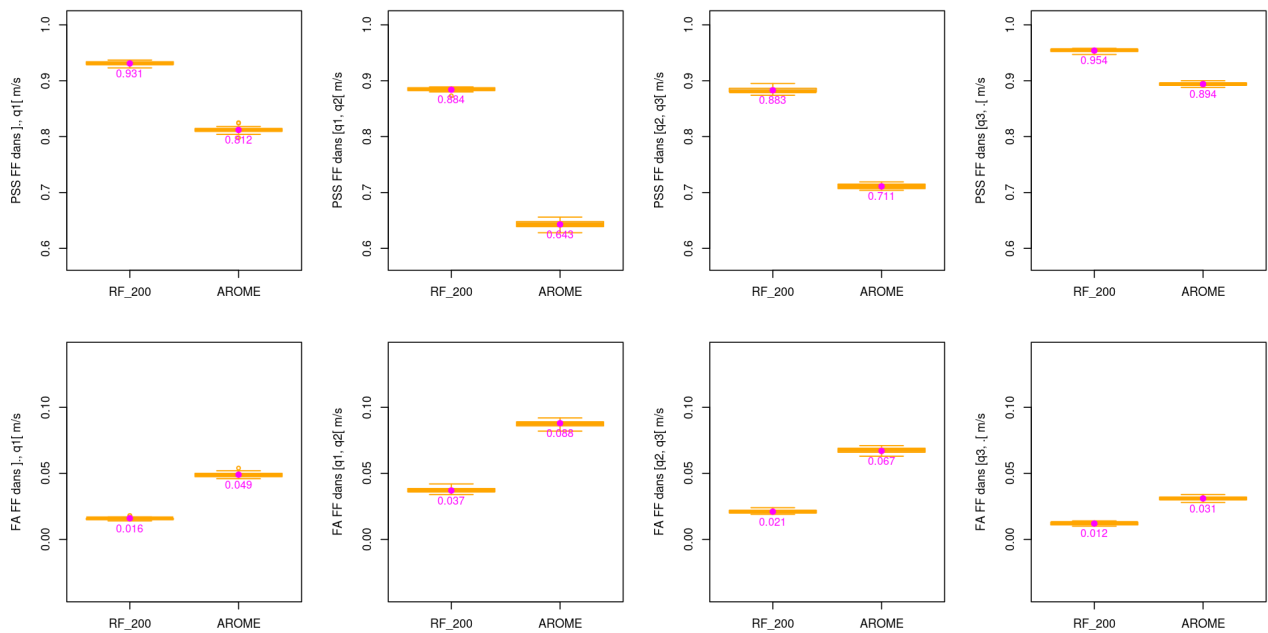
Illustration 3.23 : GLE – V – Niveau 100 m – Modèle de forêt aléatoire à 200 arbres - Box-plot PSS (première ligne PSS V \in [q_1, q_2] m/s, PSS V \in [q_2, q_3] m/s et PSS V \in [q_3, q_4] m/s) et FA (deuxième ligne FA V \in [q_1, q_2] m/s, FA V \in [q_2, q_3] m/s et FA V \in [q_3, q_4] m/s) pour l'échantillon d'apprentissage. La valeur en magenta sur chaque boîte à moustaches correspond à la moyenne des 20 échantillons.
