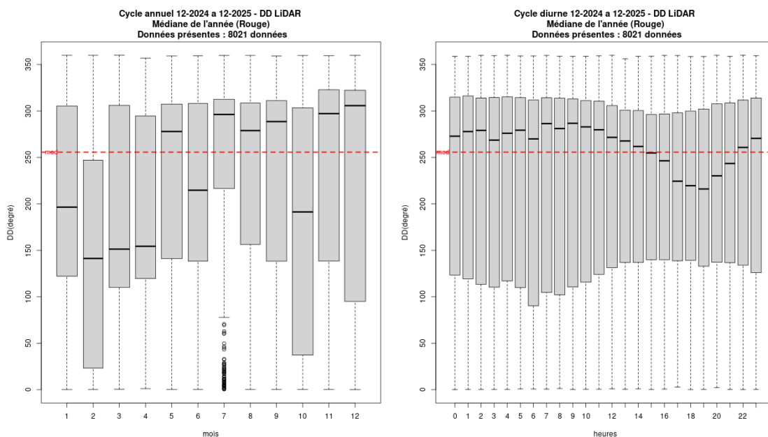
Illustration 3.7 : GLE – DD – Niveau 100 m – Distribution du vent mensuelle (graphique de gauche) et horaire (graphique de droite) à partir des données observées
