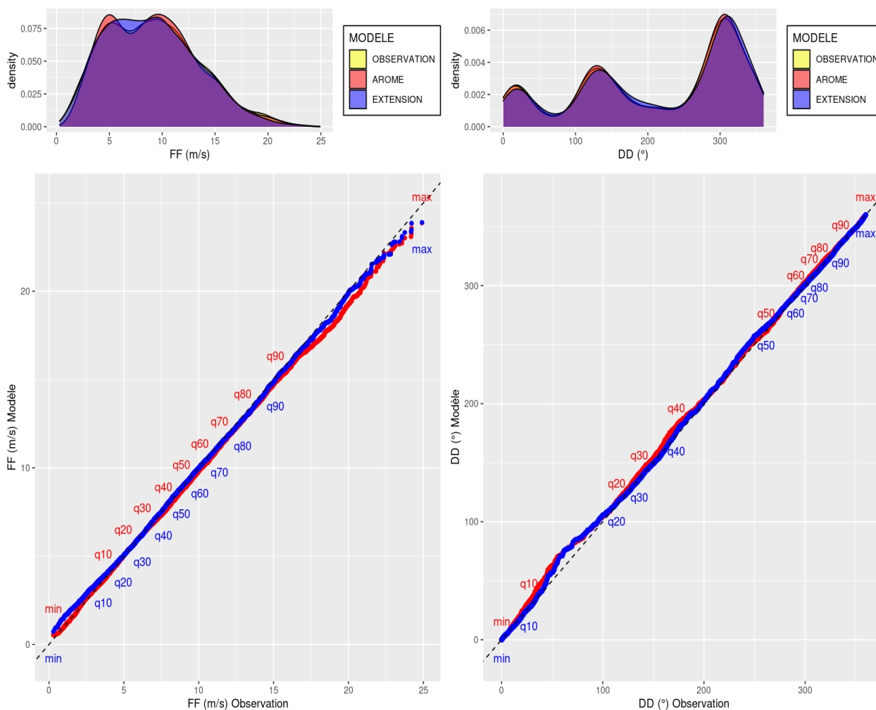
Illustration 4.12 : GLE – QQPlots FF et DD sur la période d'observation pour le niveau 40 m . En rouge : AROME, en bleu : extension statistique.
