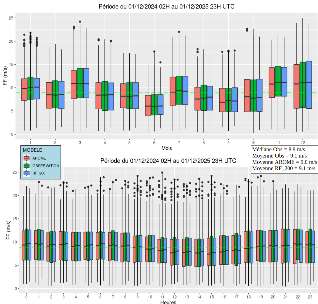
Illustration 4.5 : GLE – FF – Restitution des cycles de FF sur la période d'observation pour le niveau 40 m (du 01/12/2024 02H au 01/12/2025 23H). Sur la première ligne on retrouve le cycle annuel et sur la deuxième ligne le cycle diurne. La ligne discontinue verte traversant les boxplots désigne la médiane de l'observation sur la période d'observation.
