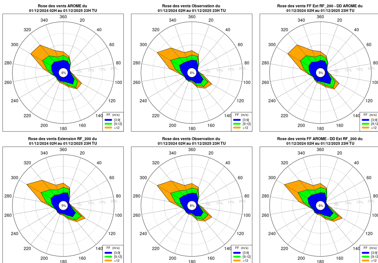
Illustration 4.11 : GLE – Roses des vents sur la période d'observation pour le niveau 40 m (du 01/12/2024 02H au 01/12/2025 23H) : sur la 1 re colonne (de haut en bas) on retrouve la rose AROME et celle de l'extension ; sur la 2 e colonne on retrouve la rose de l'observation. Les deux vignettes de cette colonne sont identiques et ont été dupliquées par soucis de lisibilité ; et sur la 3 e colonne (de haut en bas) on retrouve respectivement les roses issues de FF Extension et DD AROME, FF AROME et DD Extension
