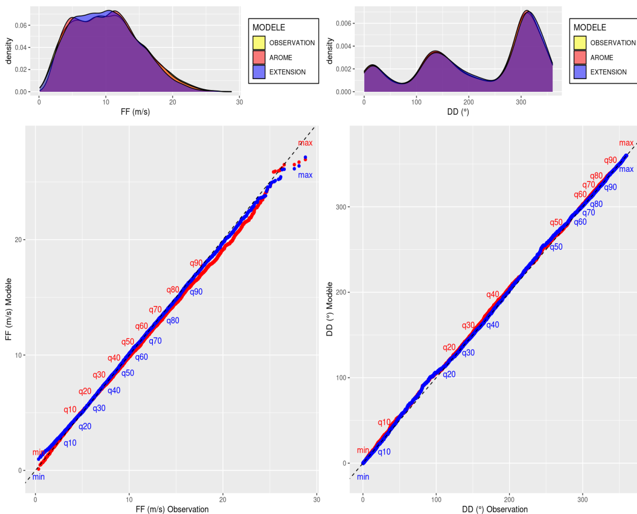
Illustration 4.10 : GLE – QQPlots FF et DD sur la période d'observation pour le niveau 200 m . En rouge : AROME, en bleu : extension statistique.
