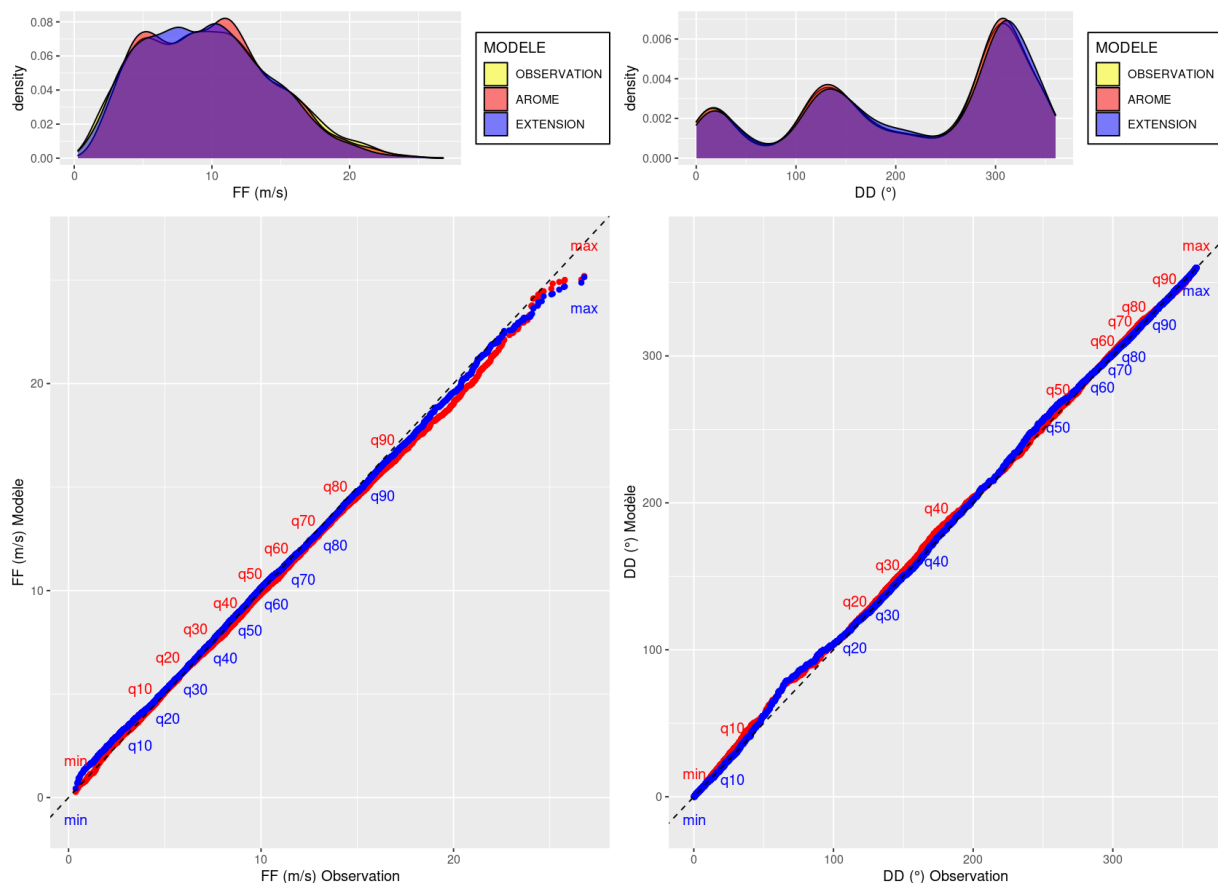
Illustration 4.8 : GLE – QQPlots FF et DD sur la période d'observation pour le niveau 100 m . En rouge : AROME, en bleu : extension statistique.
