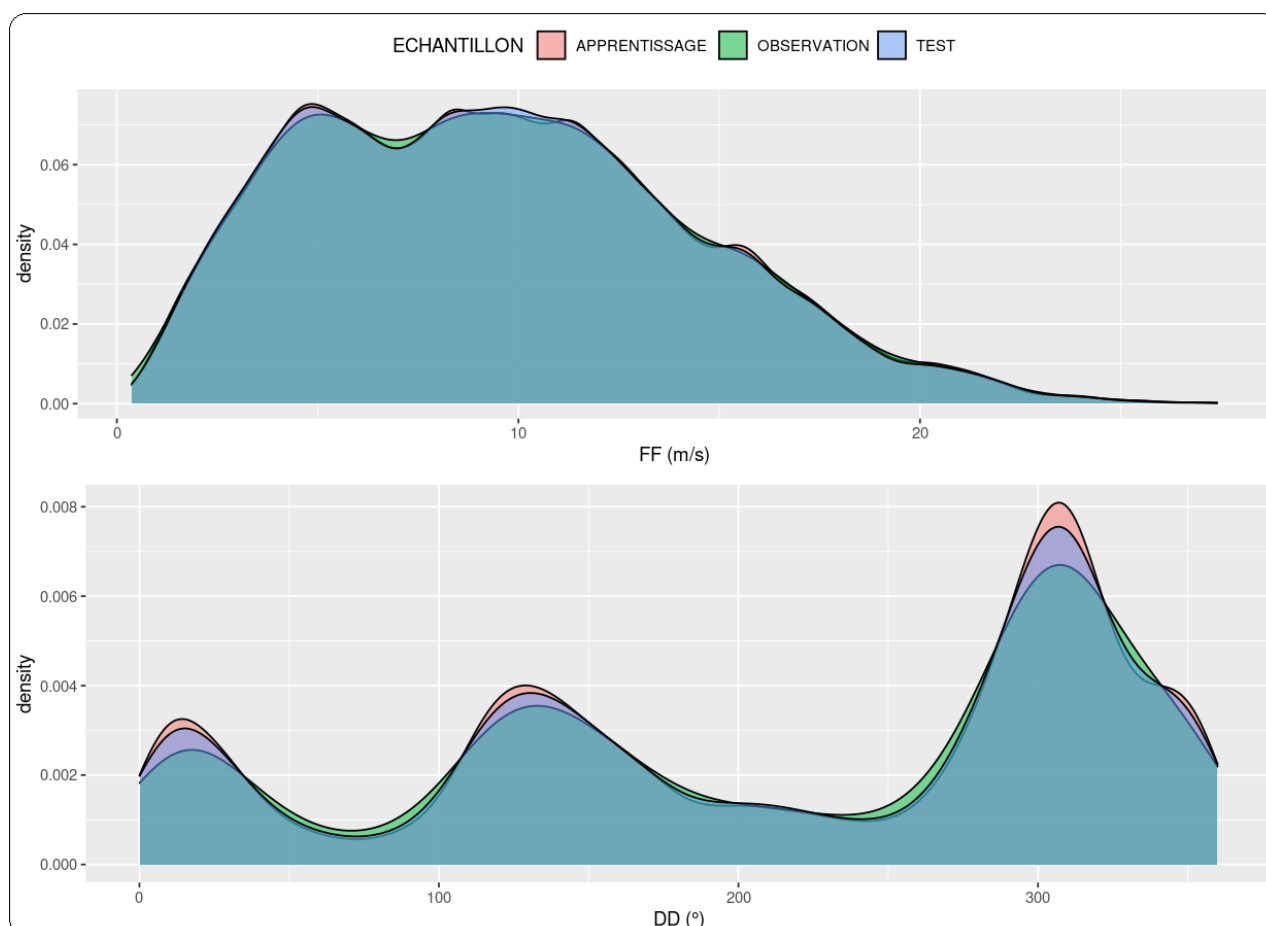
Illustration 3.9 : GLE – Distribution de FF (première ligne) et DD (deuxième ligne) pour les échantillons d'apprentissage et de test comparée à celle de l'observation sur la période d'apprentissage (période d'observation) pour le niveau 100 m
