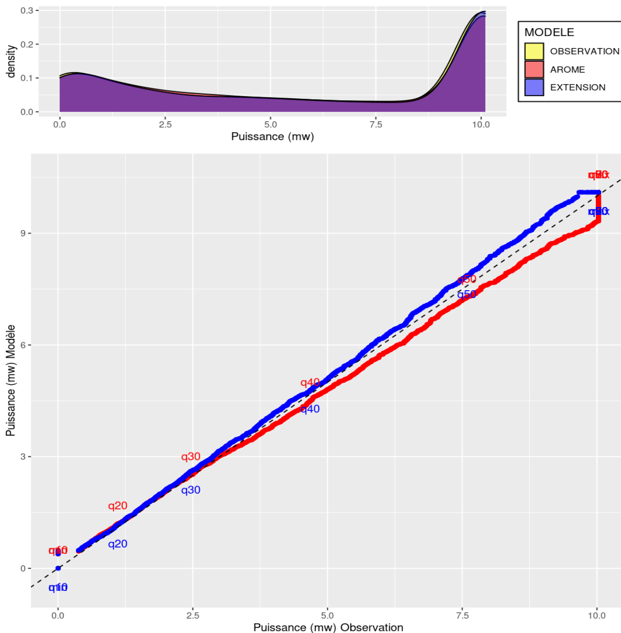
Illustration 4.15 : GLE – QQ-Plot des données de puissances de l'extension statistique (bleu) et AROME (rouge) sur la période d'observation pour le niveau 200 m.
