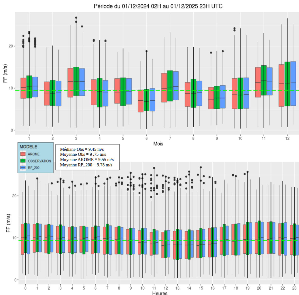
Illustration 4.1 : GLE – FF – Restitution des cycles de FF sur la période d'observation pour le niveau 100 m (du 01/12/2024 02H au 01/12/2025 23H). Sur la première ligne on retrouve le cycle annuel et sur la deuxième ligne le cycle diurne. La ligne discontinue verte traversant les boxplots désigne la médiane de l'observation sur la période d'observation.
