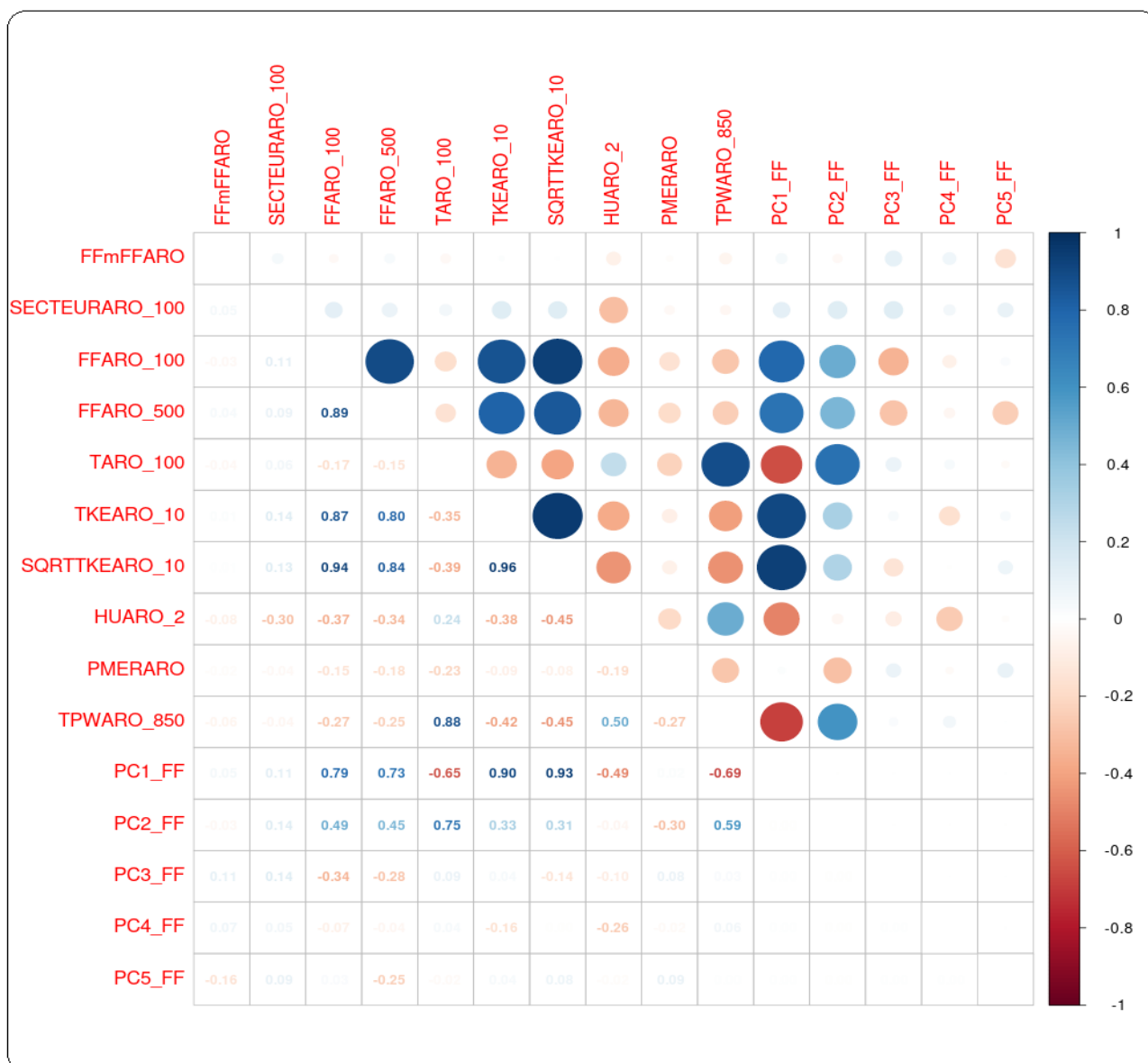
Illustration 3.3 : GLE – FF – Niveau 100 m - Corrélation entre la variable à expliquer FFmFFARO et les variables explicatives. En haut : sous forme de bulles. En bas : chiffré (0 : absence de corrélation, 1 ou -1 : forte corrélation)
