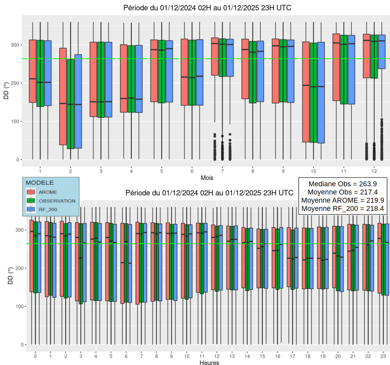
Illustration 4.4 : GLE – DD – Restitution des cycles de DD sur la période d'observation pour le niveau 200 m (du 01/12/2024 02H au 01/12/2025 23H).. Sur la première ligne on retrouve le cycle annuel et sur la deuxième ligne le cycle diurne. La ligne discontinue verte traversant les boxplots désigne la médiane de l'observation sur la période d'observation.
