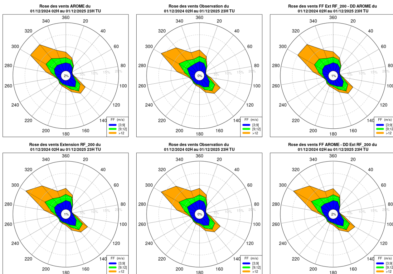
Illustration 4.14 : GLE – Roses des vents partielles (excluant les forces de vent FF < 3 m/s) sur la période d'observation (du 01/12/2024 02H au 01/12/2025 23H) pour le niveau 100 m : sur la 1 re colonne (de haut en bas) on retrouve la rose AROME et celle de l'extension ; sur la 2 e colonne on retrouve la rose de l'observation. Les deux vignettes de cette colonne sont identiques et ont été dupliquées par soucis de lisibilité ; et sur la 3 e colonne (de haut en bas) on retrouve respectivement les roses issues de FF Extension et DD AROME, FF AROME et DD Extension
