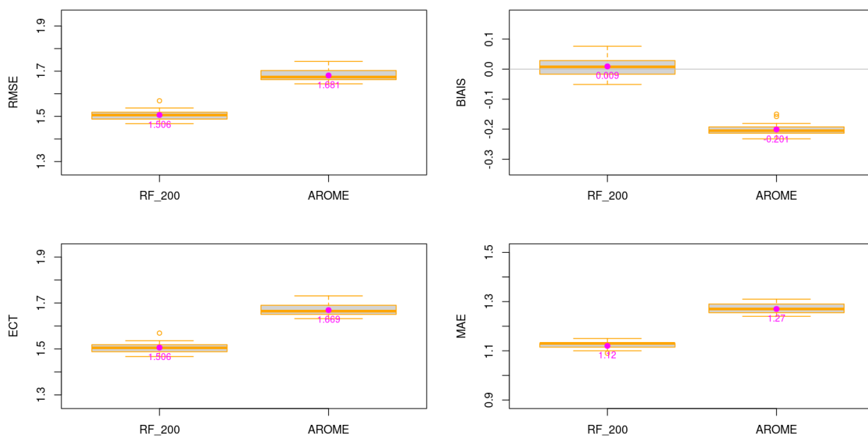
Illustration 3.14 : GLE – FF – Niveau 100 m – Modèle de forêt aléatoire - Box-plot RMSE, ECT, BIAIS et MAE pour l'échantillon de test. La valeur en magenta sur chaque boîte à moustaches correspond à la moyenne des 20 échantillons.
