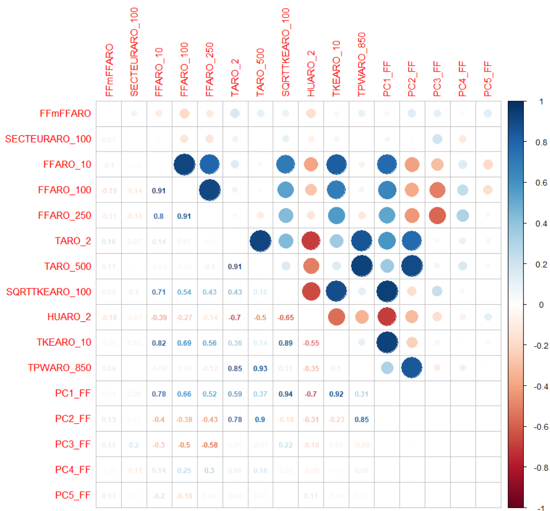
Illustration 7.9 : Station de test 1 – Variables explicatives finales (avec les composantes principales de l'ACP) pour la prédiction de FF
