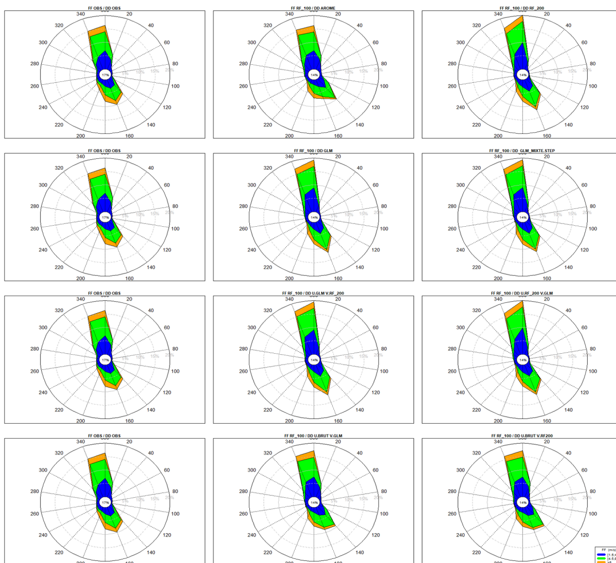
Illustration 7.51 : Station de test 1 – Roses des vents issues des combinaisons de U et V des modèles statistiques: sur la 1 re colonne l'observation ; sur la 2 e colonne (de haut en bas) on retrouve DD AROME brut (U.BRUT et V.BRUT), DD GLM (U.GLM et V.GLM), U.GLM et V.RF_200, U.BRUT et V.GLM; et sur la 3 e colonne on retrouve DD RF_200 (U.RF_200, V.RF_200), DD GLM MIXTE.STEP (U.GLM MIXTE.STEP, V.GLM MIXTE.STEP), U.RF_200 et V.GLM, U.BRUT et V.RF_200
