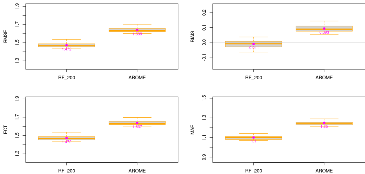
Illustration 3.24 : GLE – V – Niveau 100 m – Modèle de forêt aléatoire à 200 arbres - Box-plot RMSE, ECT, BIAIS et MAE pour l'échantillon de test. La valeur en magenta sur chaque boîte à moustaches correspond à la moyenne des 20 échantillons.
