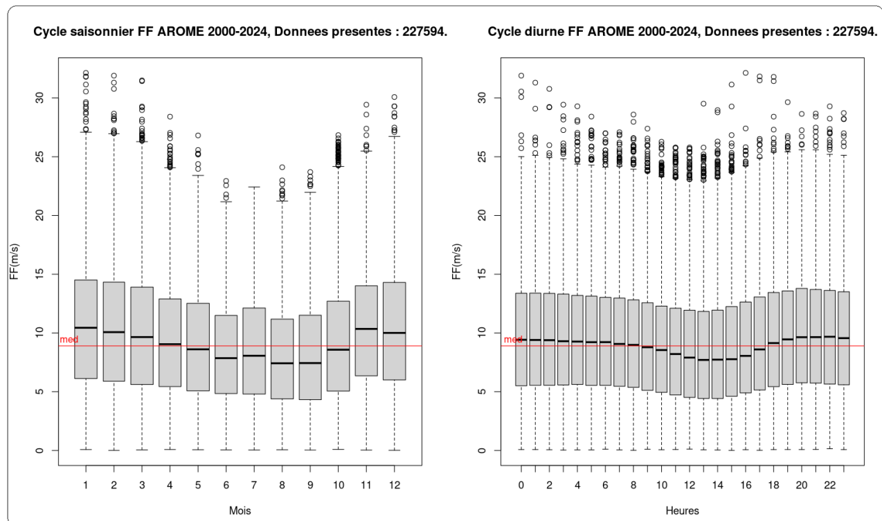
Illustration 3.5: GLE – FF – Niveau 100 m – Distribution du vent mensuelle (graphique de gauche) et horaire (graphique de droite) à partir des données climatologiques (AROME 2000 à 2024) permettant de déterminer les cycles saisonnier et diurne
