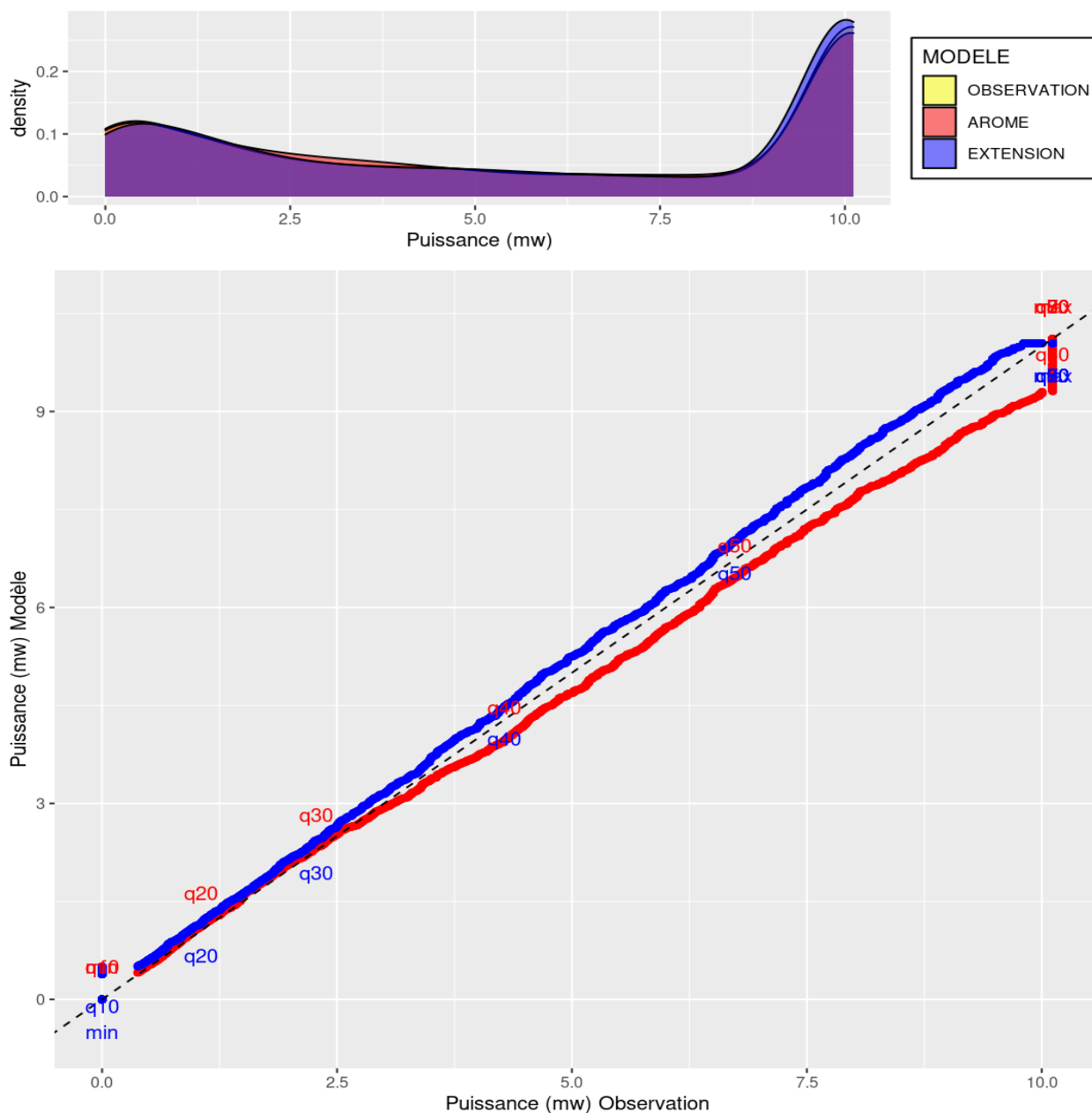
Illustration 4.13 : GLE – QQ-Plot des données de puissances de l'extension statistique (bleu) et AROME (rouge) sur la période d'observation pour le niveau 100 m.
