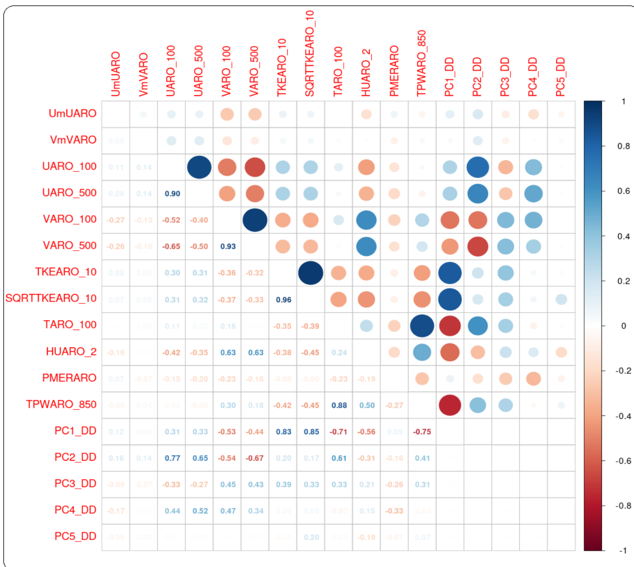
Illustration 3.6 : GLE – DD – Niveau 100 m – Corrélation entre les variables à expliquer UmUARO et VmVARO et les variables explicatives. En haut : sous forme de bulles. En bas : chiffré (0 : absence de corrélation, 1 ou -1 : forte corrélation).
