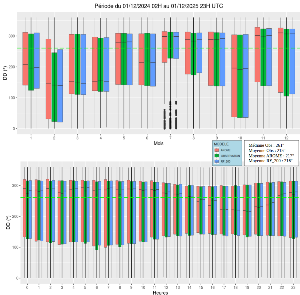
Illustration 4.2 : GLE – DD – Restitution des cycles de DD sur la période d'observation pour le niveau 100 m (du 01/12/2024 02H au 01/12/2025 23H). Sur la première ligne on retrouve le cycle annuel et sur la deuxième ligne le cycle diurne. La ligne discontinue verte traversant les boxplots désigne la médiane de l'observation sur la période d'observation.
