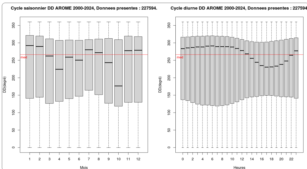
Illustration 3.8 : GLE – DD – Niveau 100 m – Distribution du vent permettant de déterminer le cycle saisonnier (graphique de gauche) et cycle diurne (graphique de droite) à partir de la climatologie AROME (2000-2024), permettant de déterminer les cycles saisonnier et diurne.
