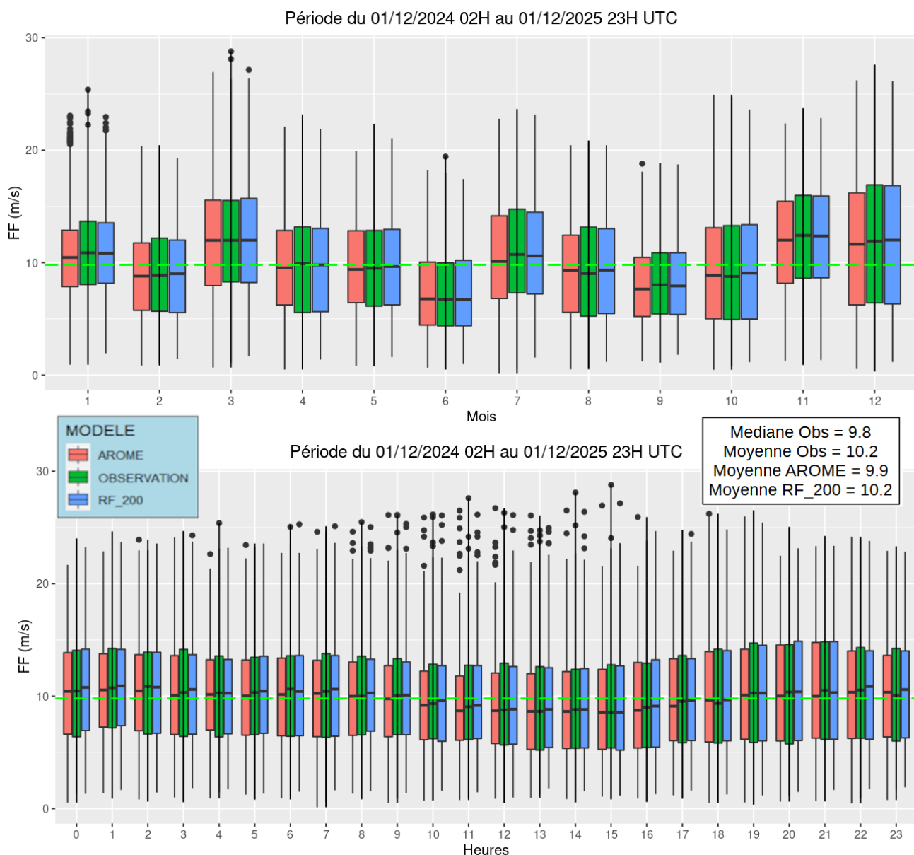
Illustration 4.3 : GLE – FF – Restitution des cycles de FF sur la période d'observation pour le niveau 200 m (du 01/12/2024 02H au 01/12/2025 23H). Sur la première ligne on retrouve le cycle annuel et sur la deuxième ligne le cycle diurne. La ligne discontinue verte traversant les boxplots désigne la médiane de l'observation sur la période d'observation.
