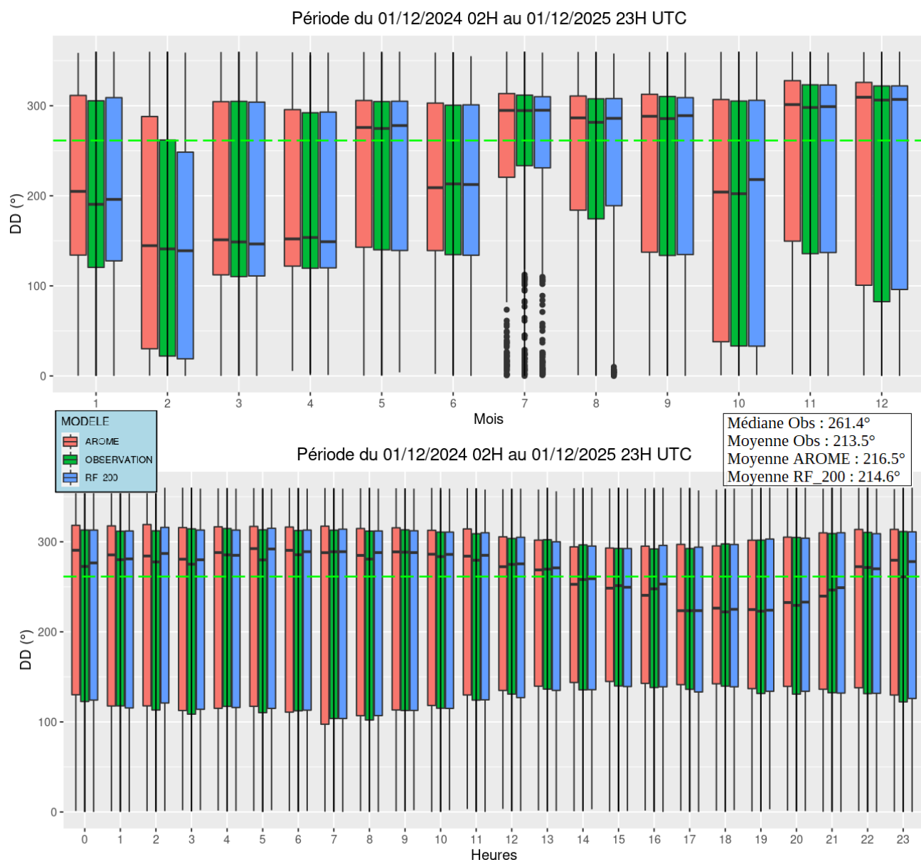
Illustration 4.6 : GLE – DD – Restitution des cycles de DD sur la période d'observation pour le niveau 40 m (du 01/12/2024 02H au 01/12/2025 23H ). Sur la première ligne on retrouve le cycle annuel et sur la deuxième ligne le cycle diurne. La ligne discontinue verte traversant les boxplots désigne la médiane de l'observation sur la période d'observation.
