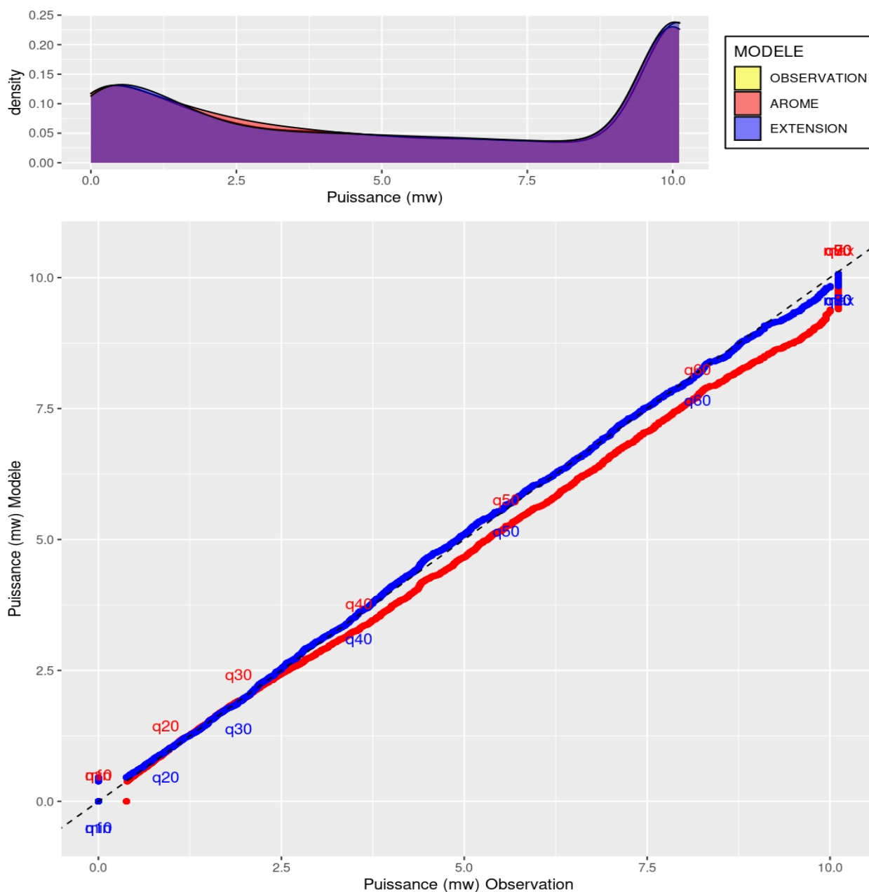
Illustration 4.16 : GLE – QQ-Plot des données de puissances de l'extension statistique (bleu) et AROME (rouge) sur la période d'observation pour le niveau 40 m.
