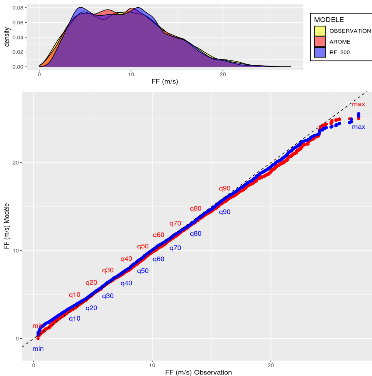
Illustration 3.17 : GLE – FF – QQ-Plots sur l'échantillon de test concaténé pour le niveau 100 m. En rouge : AROME, en bleu : RF_200.
