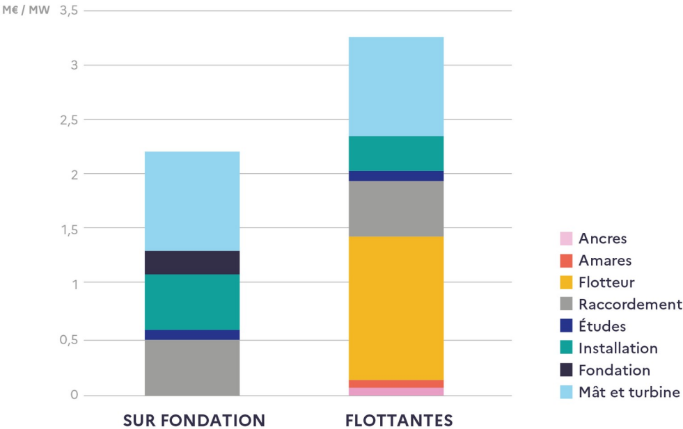
Principaux coûts d'investissement Comparaison entre l'éolien flottant et posé
