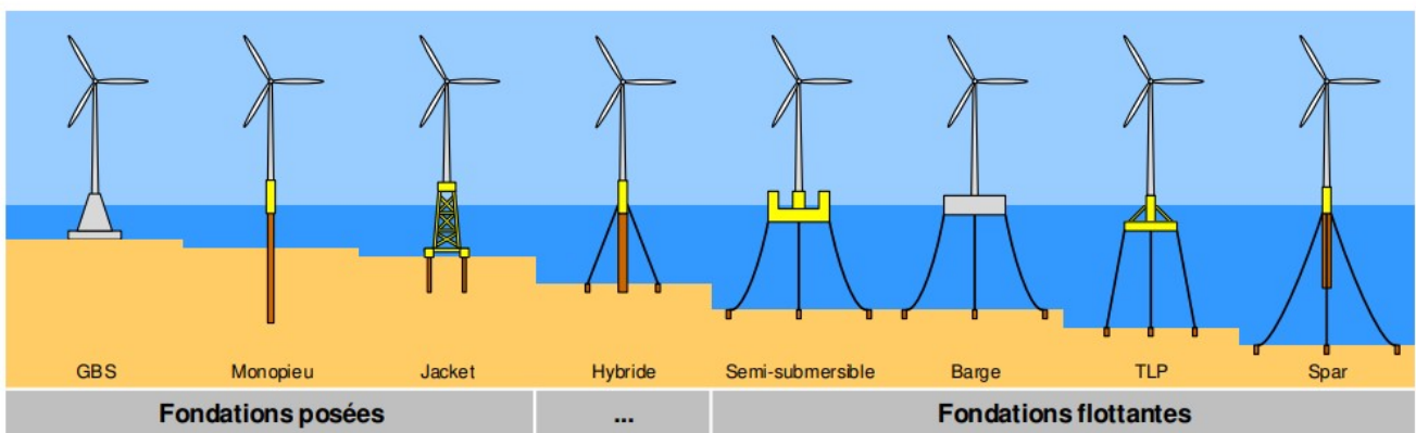
Technologie de fondation d'éoliennes en mer © DNV
