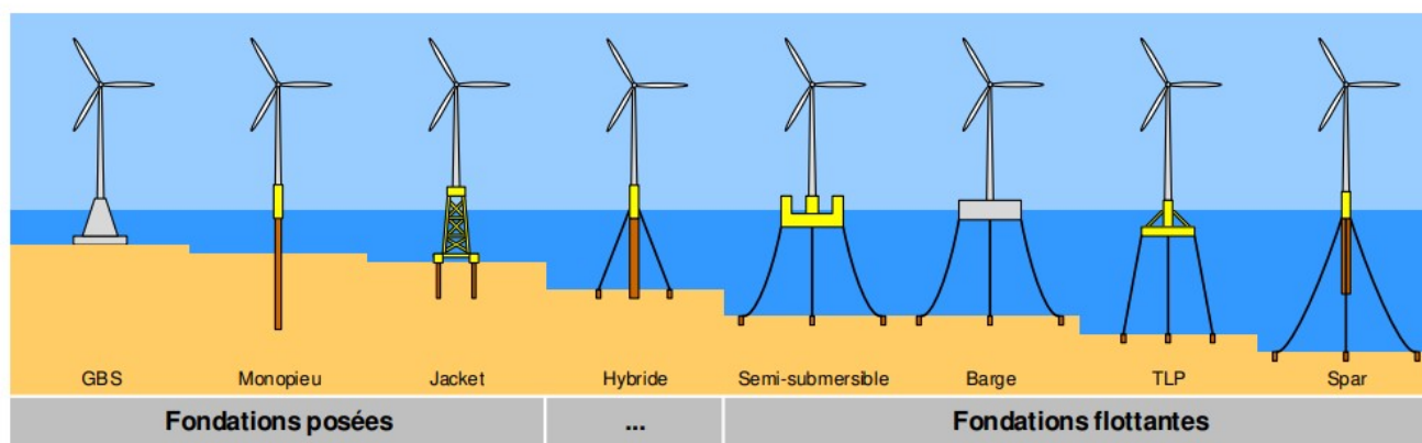
Technologie de fondation d'éoliennes en mer © DNV
