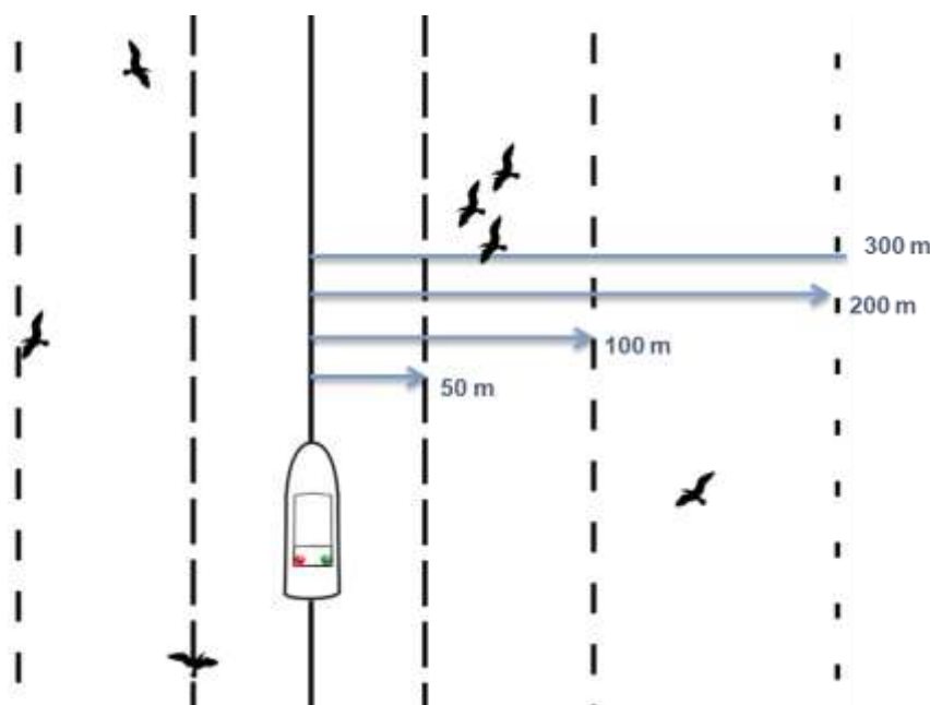
Figure 24 : Schéma simplifié des estimations de densités par strip transect .
